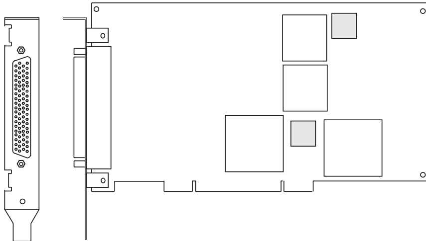
Figura 2. Recurso 2943
