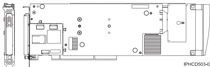
Figura 54. Visualizações lateral e longitudinal do adaptador
