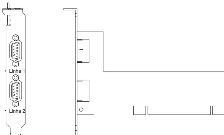
Figura 5. Adaptador PCI EIA-232 Assíncrono de 2 Portas
