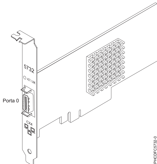
Figura 28. 10 Gigabit Ethernet-CX4 PCI Express(PCIe)
