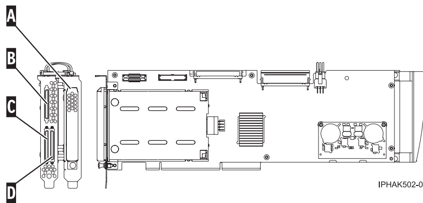
Figura 58. Adaptador 5782
