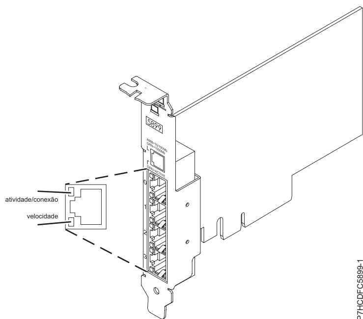
Figura 35. Adaptador
