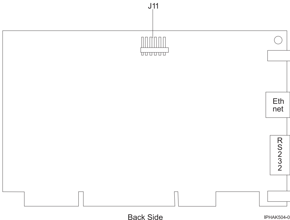
Figura 39. Lado traseiro do adaptador
