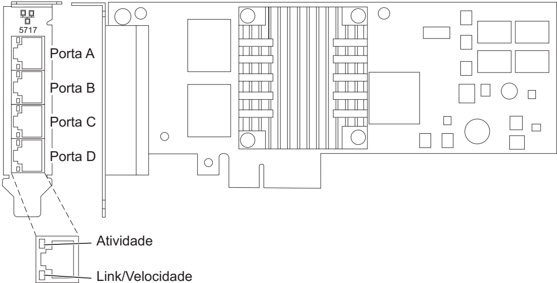
Figura 27. Adaptador PCIe de Base-TX de 4 portas 10/100/1000
