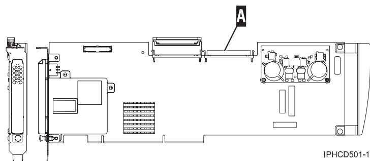
Figura 52. IOA do cache de gravação auxiliar
