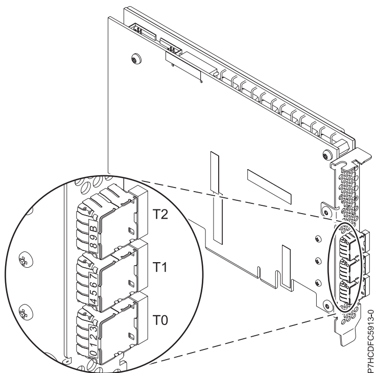
Figura 50. Adaptador ESA3
