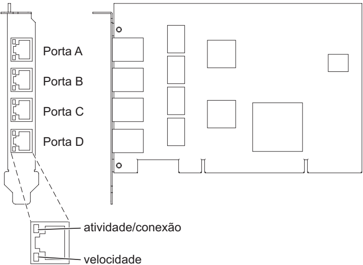
Figura 30. Adaptador PCI-X de Base-TX 10/100/1000 de 4 Portas
