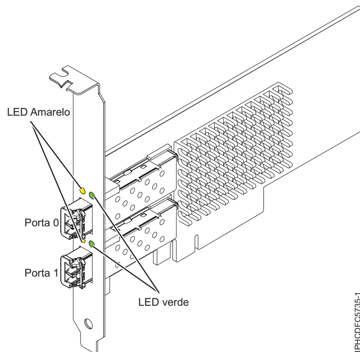
Figura 8. Adaptador 5735
