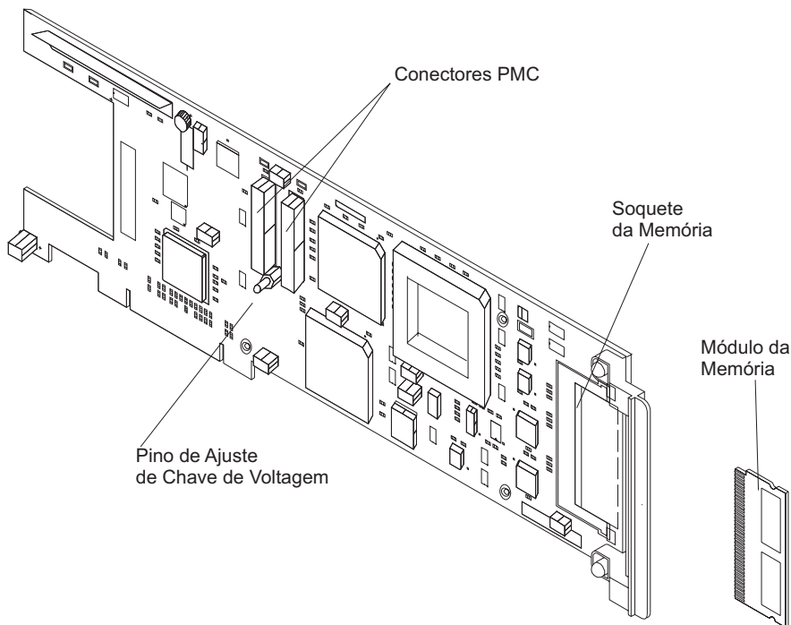
Figura 60. Adaptador PCI base IBM ARTIC960Hx
