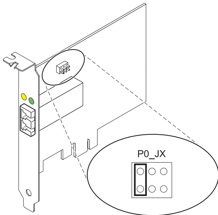
Figura 10. Jumper do ID de dispositivo
