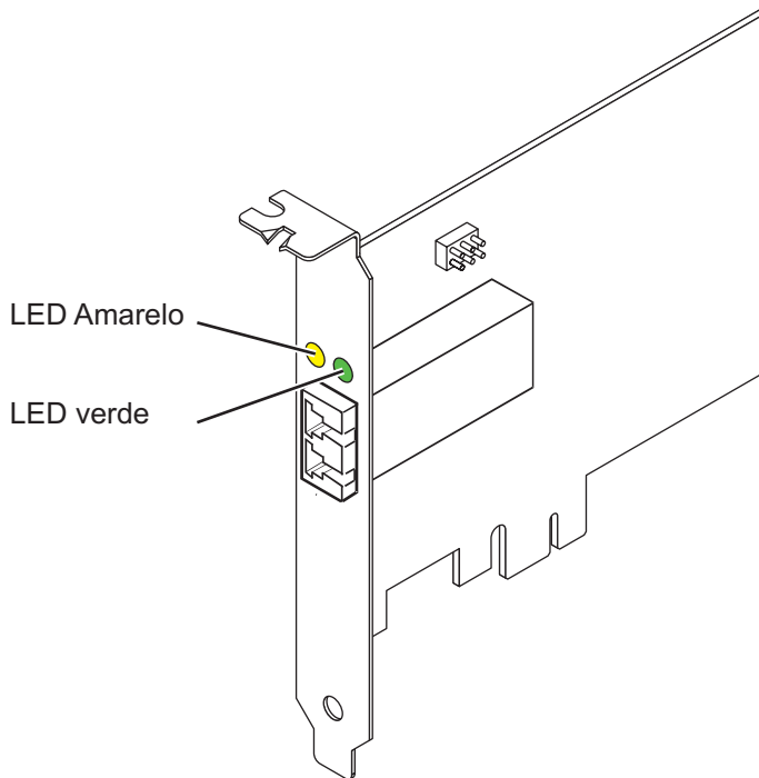
Figura 9. Adaptador 5773
