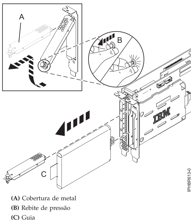
Figura 63. Substituindo a bateria de cache 572F/575C
