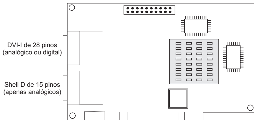
Figura 13. Recurso 2849
