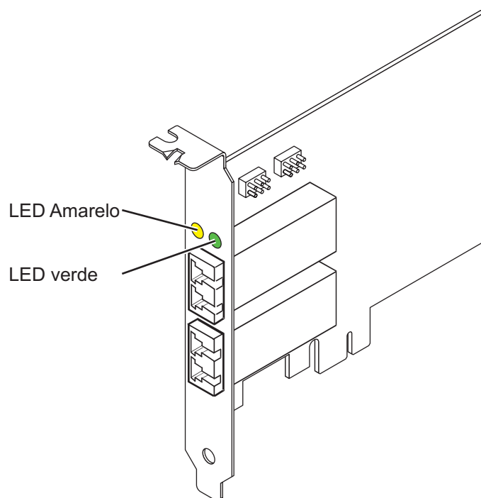
Figura 11. Adaptador 5774
