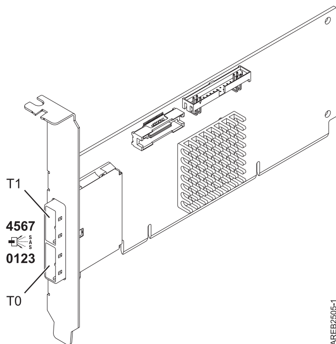
Figura 42. Adaptador PCI-X DDR dual externo – SAS de 4 portas
