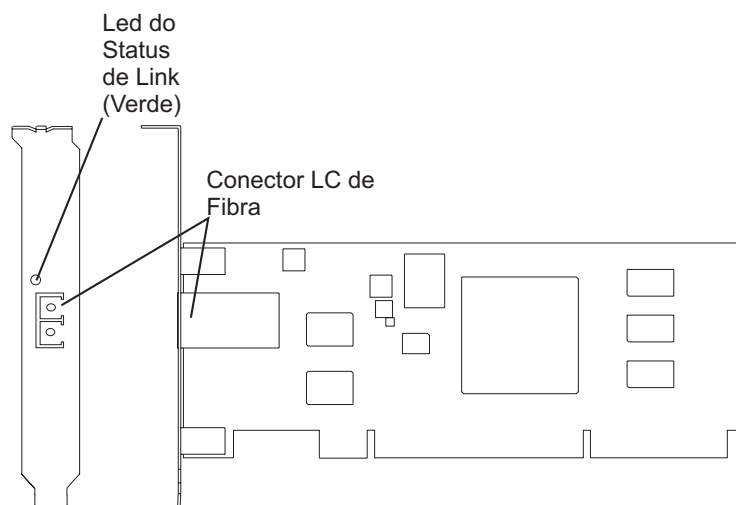
Figura 23. Adaptador PCI-X TOE iSCSI SX de 1 Gigabit
