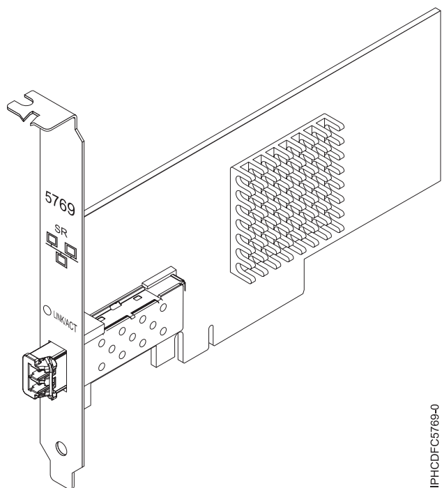
Figura 33. Adaptador PCIe de 10 Gigabits Ethernet-SR
