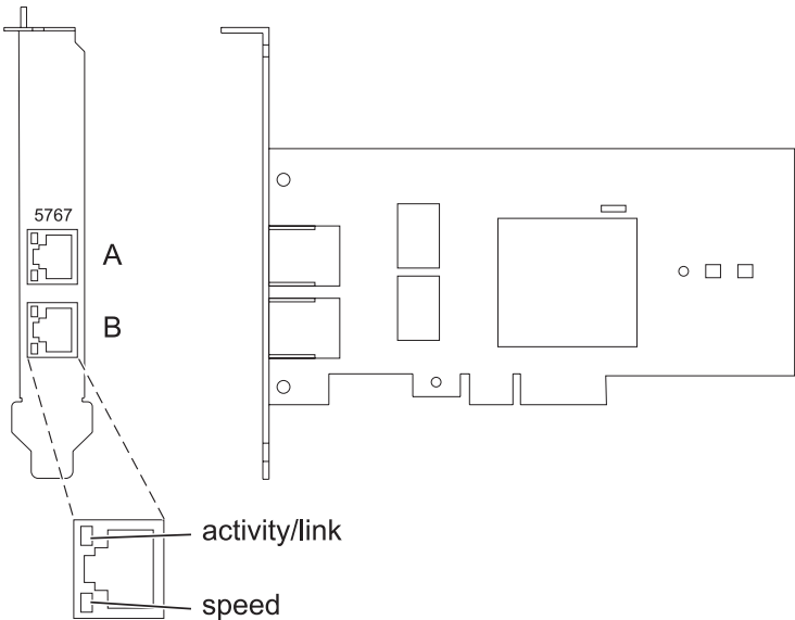
Figura 31. Adaptador PCI Express Ethernet de Base-TX 10/100/1000 de 2 portas
