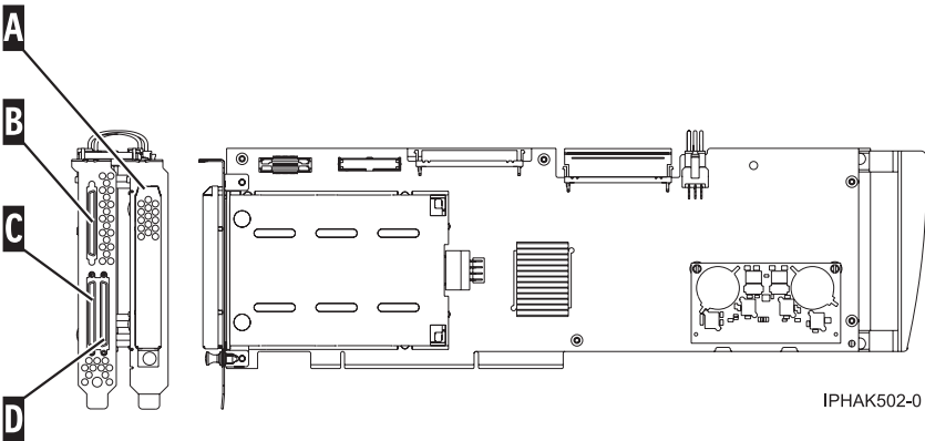
Figura 56. Adaptador
