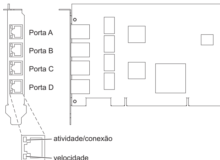
Figura 29. Adaptador PCI-X de Base-TX 10/100/1000 de 4 Portas
