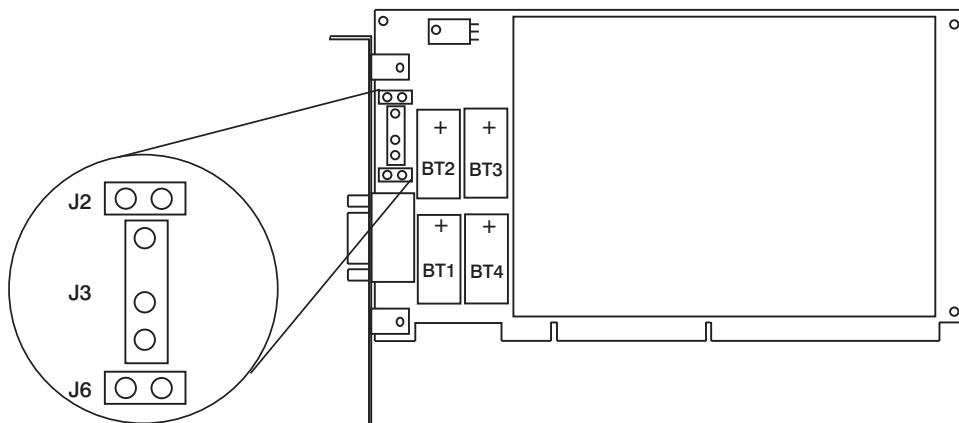
Figura 40. Substituindo baterias do coprocessador
