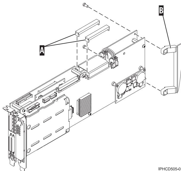
Figura 59. Preparando o adaptador para colocação em um cassete
