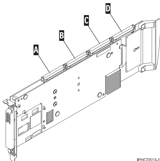
Figura 55. Conectores SCSI do adaptador
