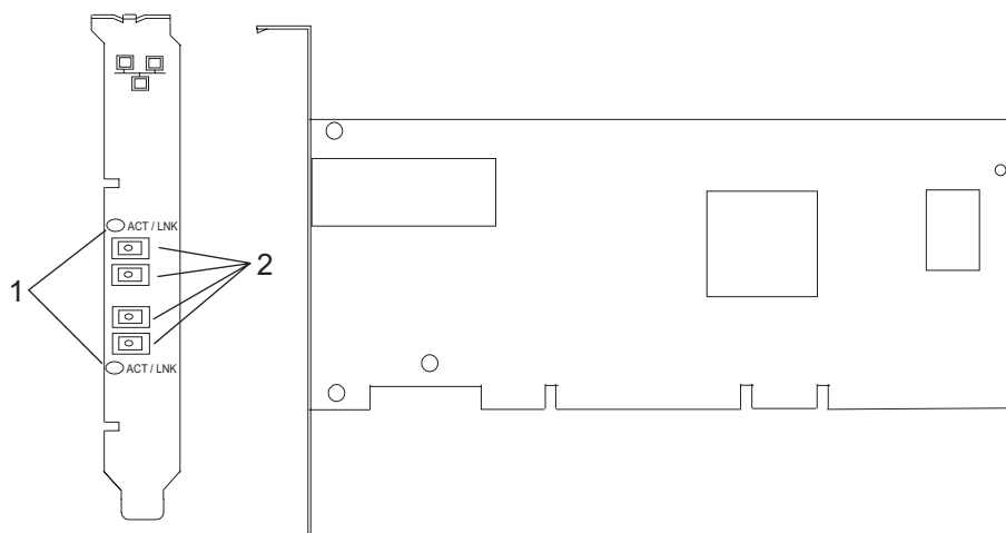
Figura 21. Recurso 5707
