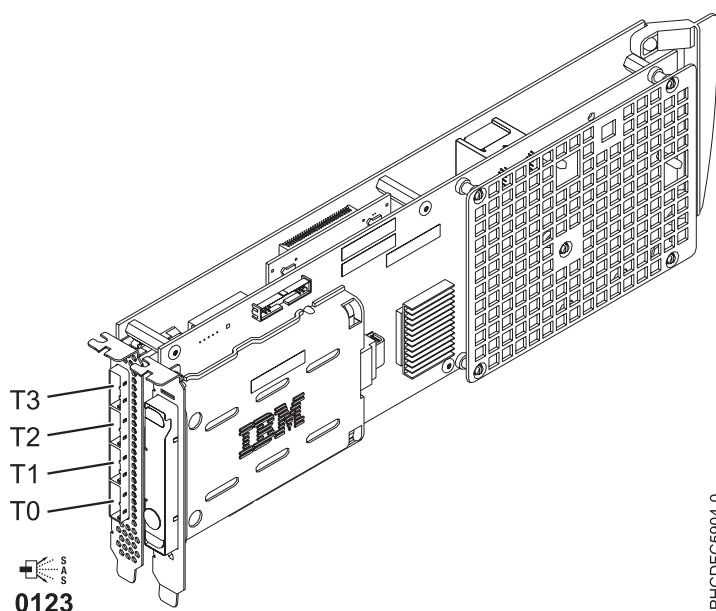
Figura 60. Adaptador PCI-X DDR 1,5GB cache RAID SAS
