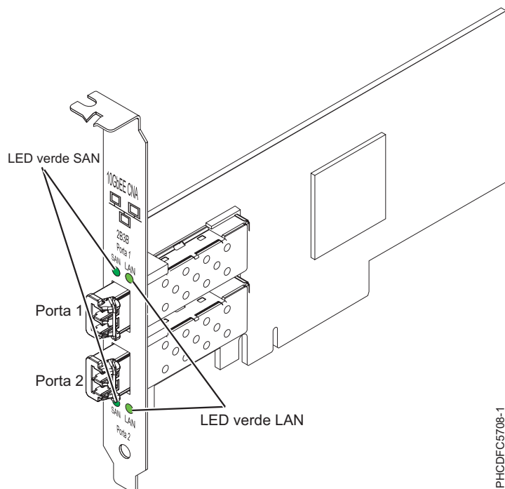
Figura 26. Adaptador Dual Port FCoE PCIe 10 -Gb
