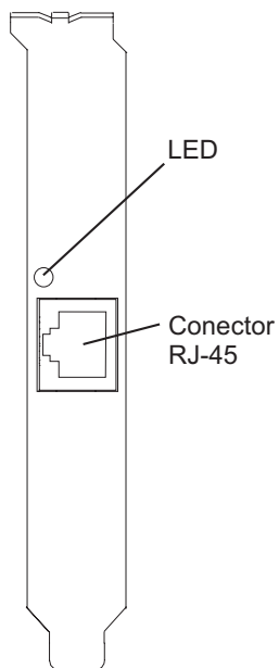
Figura 30. LED no Adaptador PCI-X TOE iSCSI de 1 Gigabit-TX
