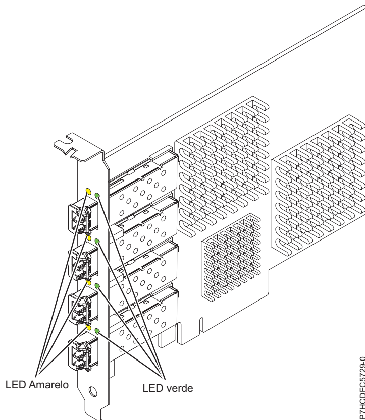
Figura 8. Adaptador FC 5729
