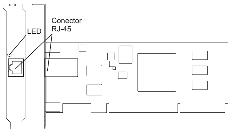
Figura 28. Adaptador PCI-X TOE iSCSI TX de 1 Gigabit
