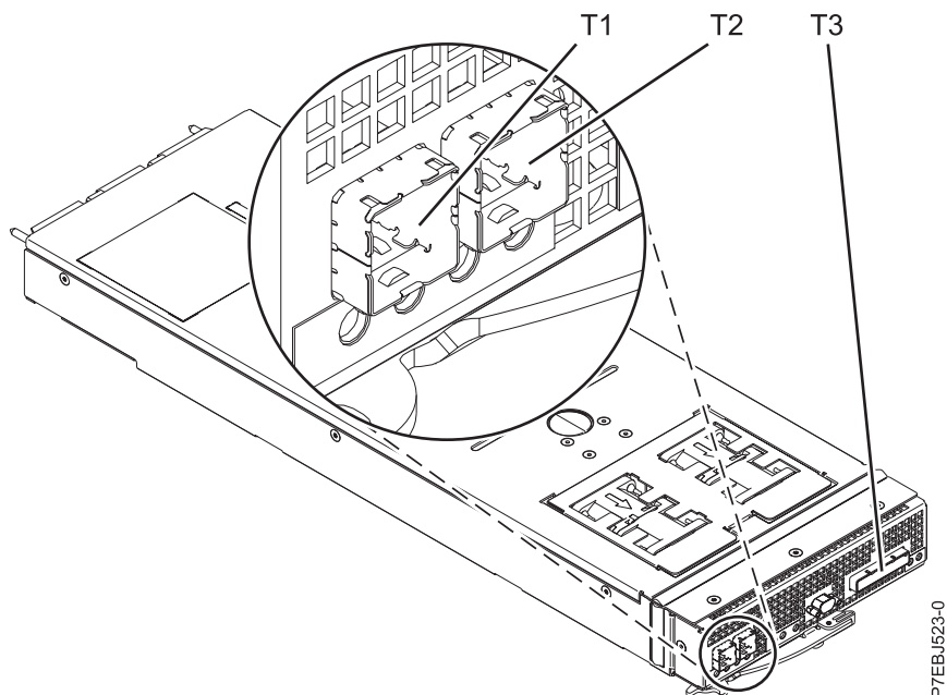
Figura 79. Gabinete SAS RAID de 6Gb x8 com cache de 3,1GB CCIN 57C3 PCIe2
