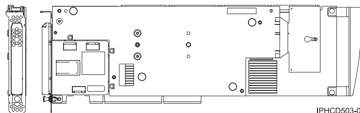
Figura 68. Visualizações lateral e longitudinal do adaptador
