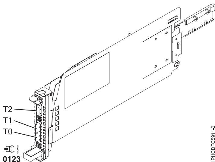
Figura 63. Adaptador SAS para a opção dividir DASD interna
