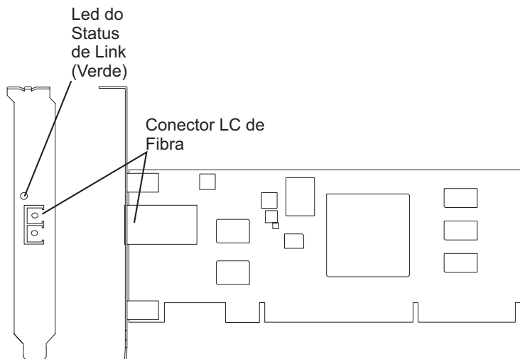
Figura 27. Adaptador PCI-X TOE iSCSI SX de 1 Gigabit
