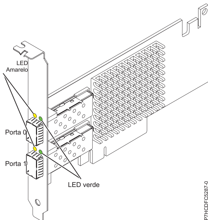
Figura 21. Adaptador SR PCIe2 de 2 portas de 10GbE
