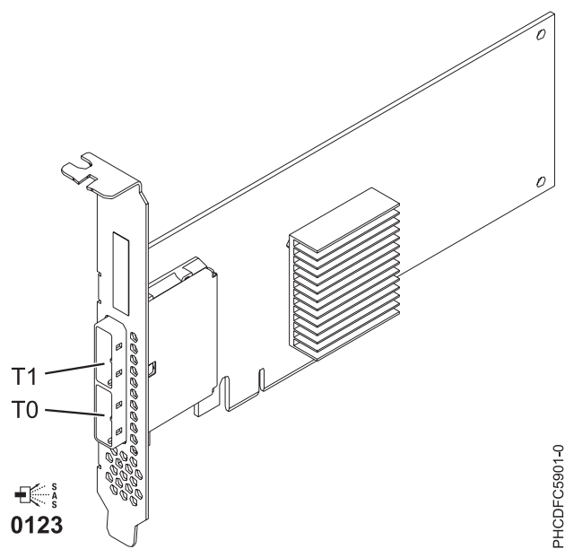
Figura 57. Adaptador SAS x4 - PCIe dual
