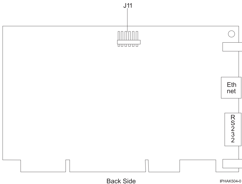
Figura 52. Lado traseiro do adaptador
