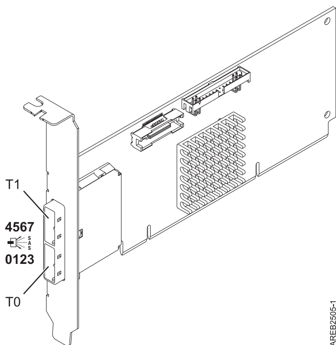
Figura 56. Adaptador PCI-X DDR dual externo – SAS de 4 portas
