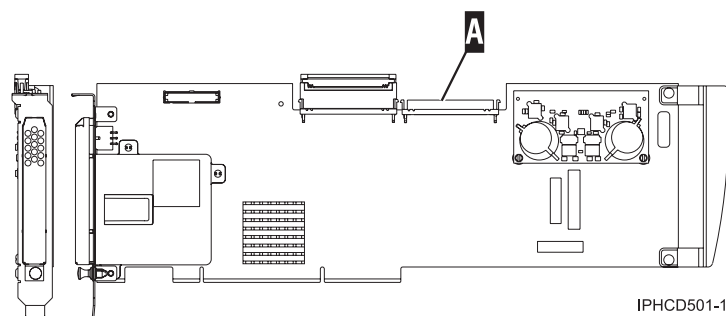
Figura 70. IOA do cache de gravação auxiliar
