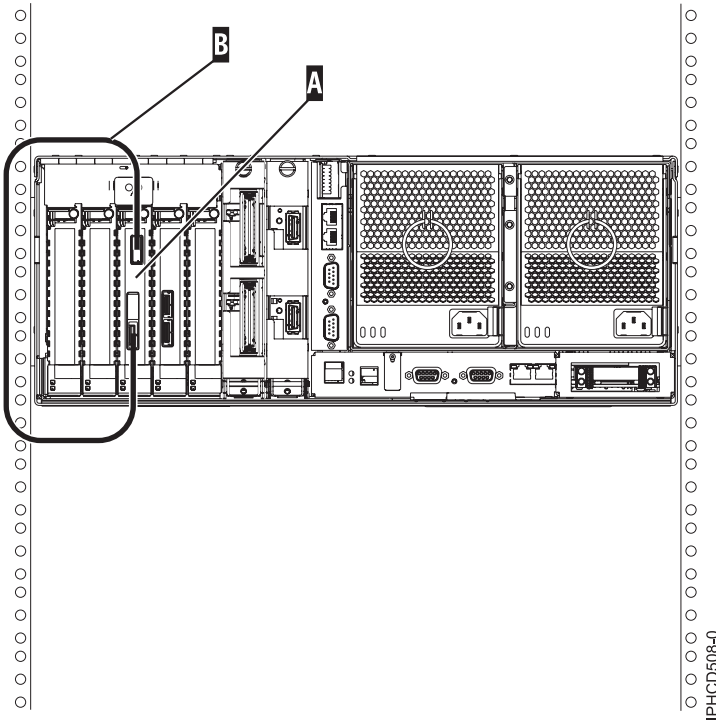
Figura 64. Vista posterior do sistema com o recurso 5911 instalado e cabeado
