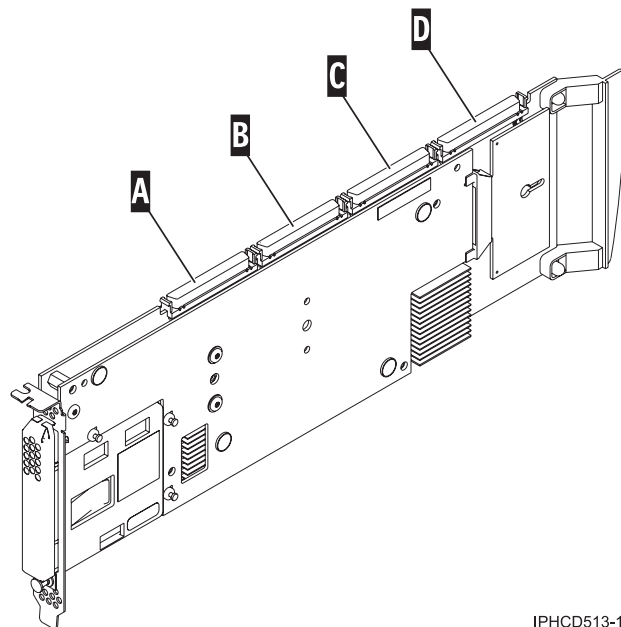
Figura 73. Conectores SCSI do adaptador
