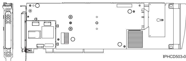
Figura 72. Visualizações lateral e longitudinal do adaptador
