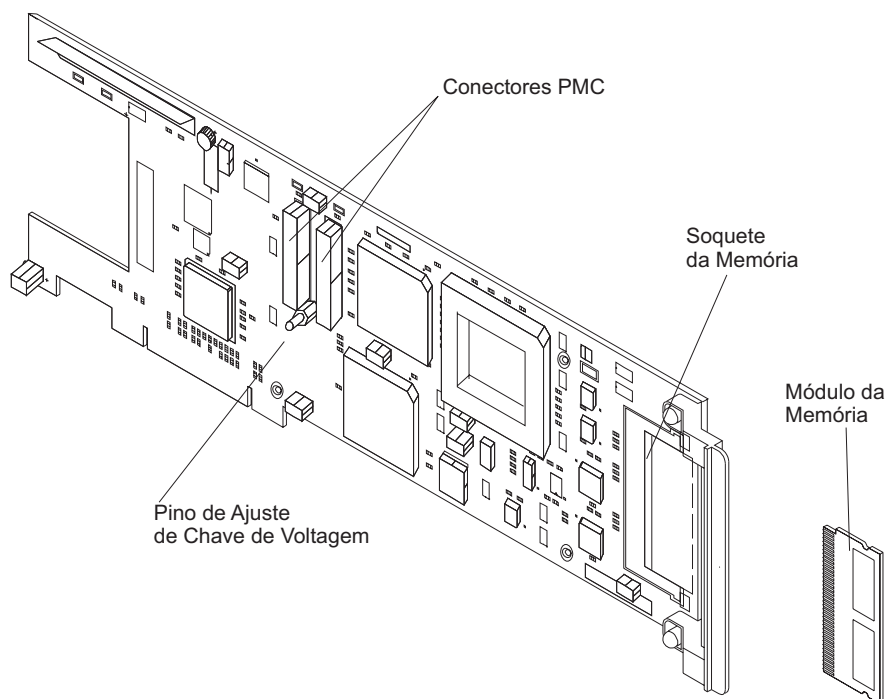
Figura 76. Adaptador PCI base IBM ARTIC960Hx
