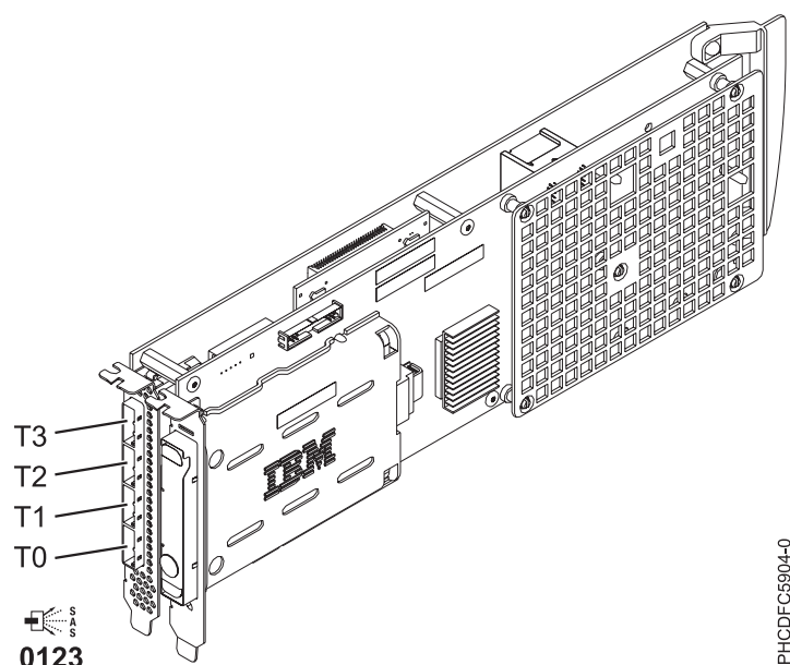
Figura 59. PCI-X Adaptador DDR 1,5GB cache RAID SAS
