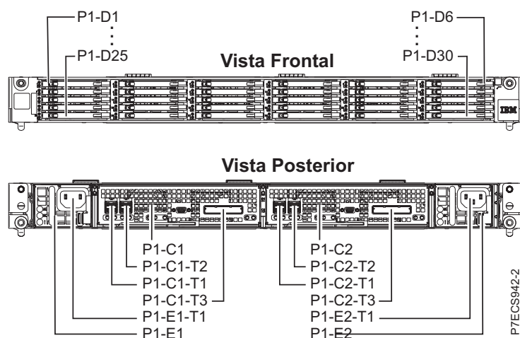
Figura 78. Códigos de colocação do adaptador RAID SAS com cache integrado 3,1GB PCIe2
