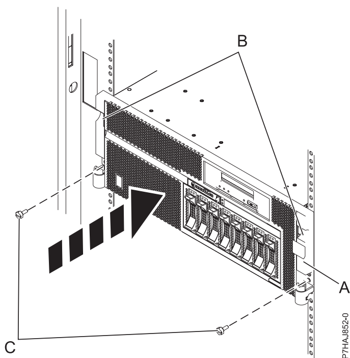
Figura 26. Recolocando os Parafusos de Aperto Manual
