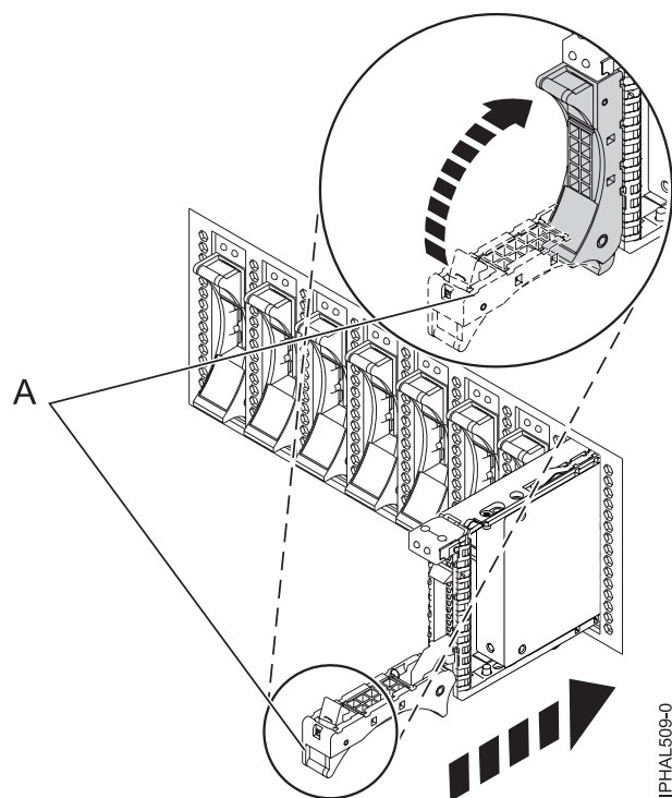
Figura 14. Instalar as Unidades de Disco no Painel Traseiro
