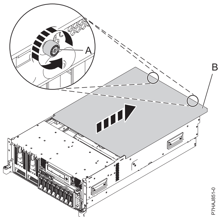
Figura 22. Removendo a Tampa de Acesso de Serviço
