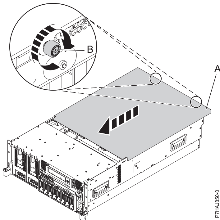
Figura 23. Instalando a Tampa de Acesso de Serviço
