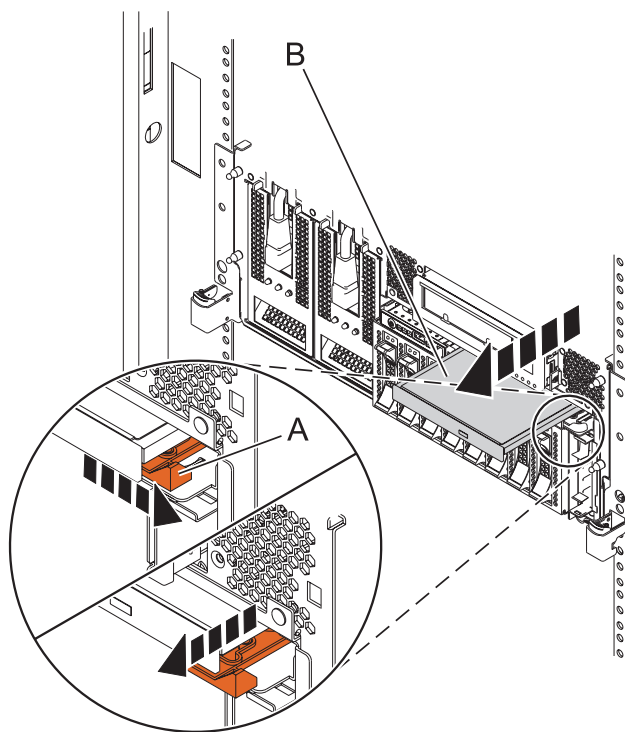
Figura 7. Removendo o dispositivo de mídia do painel traseiro da unidade de disco
