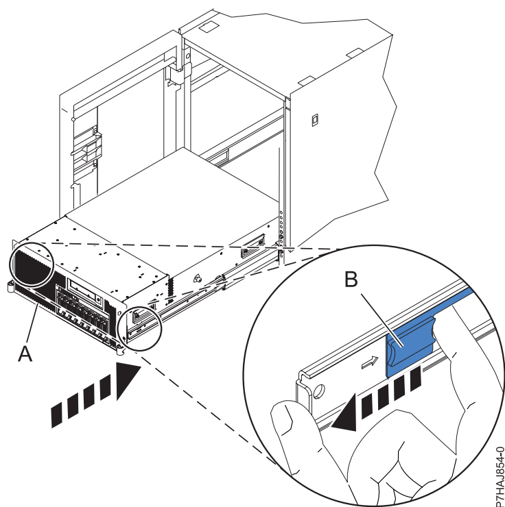
Figura 25. Liberando as Travas de Segurança dos Trilhos
