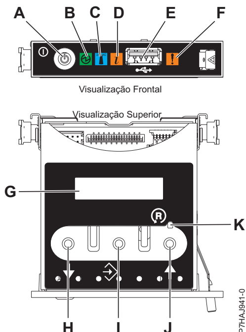
Figura 19. Painel de Controle
