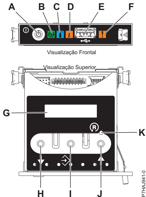
Figura 18. Painel de Controle
