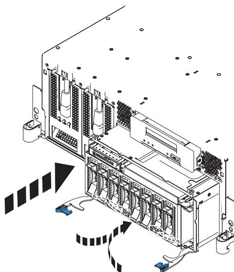
Figura 12. Instalando o Painel Traseiro da Unidade de Disco ocupada em um modelo montado em rack
