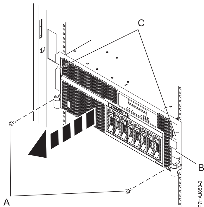
Figura 20. Removendo a Tampa Frontal
