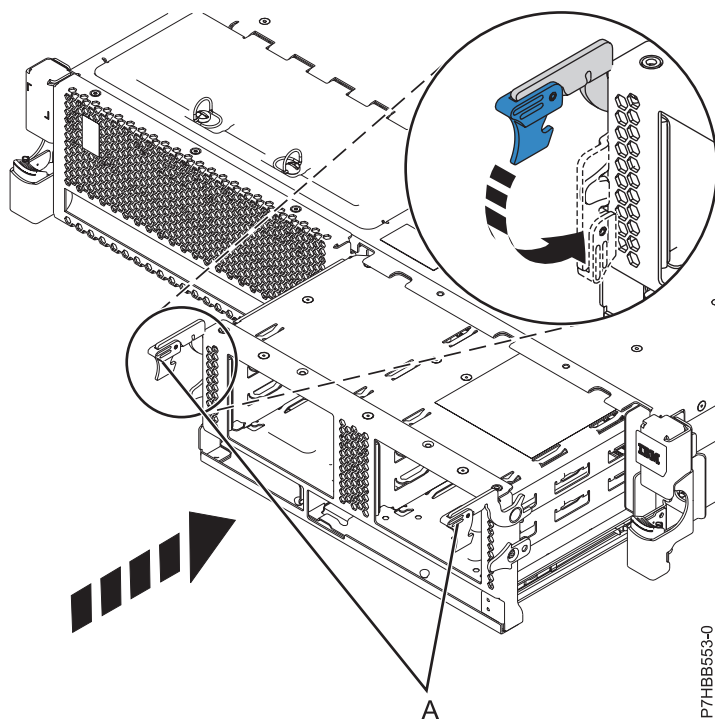
Figura 8. Instalando o Painel Traseiro que Não é Ocupado com Unidades de Disco em um Modelo Montado em Rack
