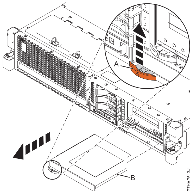
Figura 5. Removendo o dispositivo de mídia SAS do painel traseiro da unidade de disco
