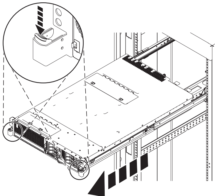
Figura 17. Colocando o Sistema na Posição de Serviço
