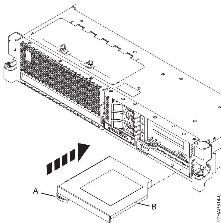
Figura 11. Instalando o Dispositivo de Mídia SAS
