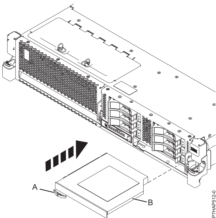
Figura 12. Instalando o Dispositivo de Mídia Fino
