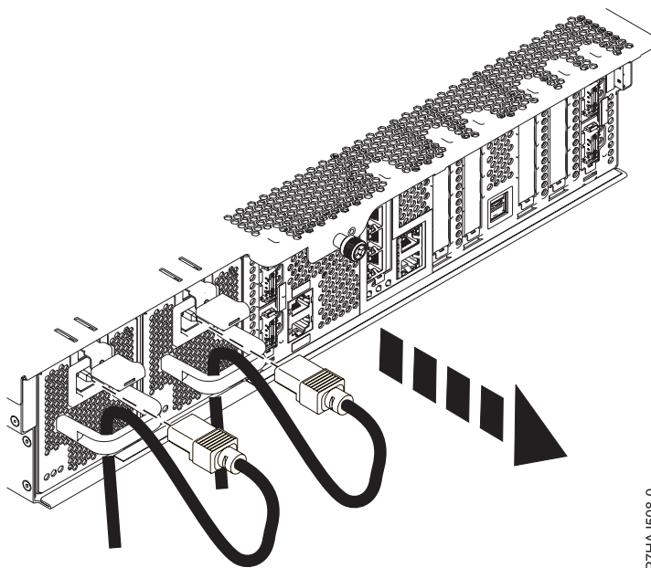
Figura 20. Removendo os Cabos de Energia
