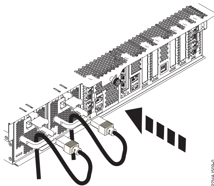
Figura 21. Conectando os Cabos de Energia
