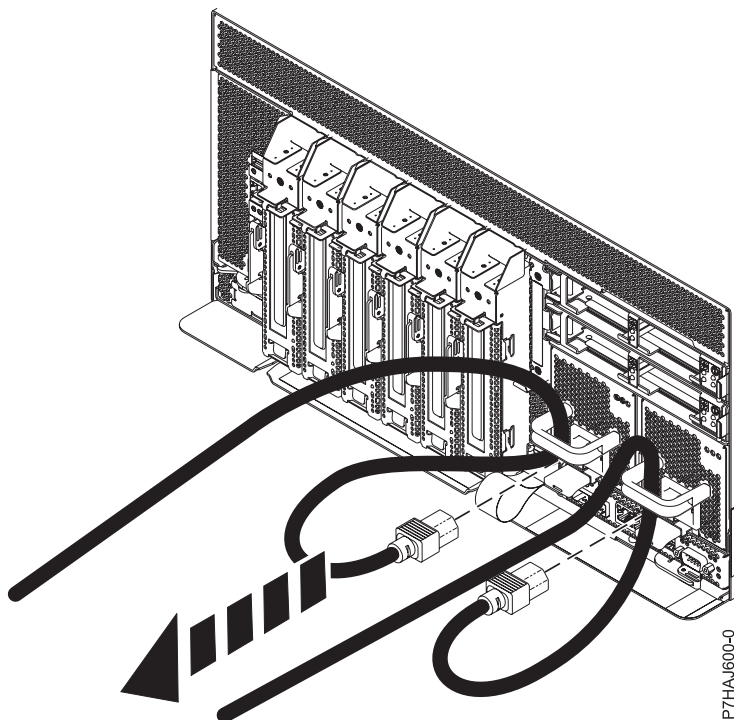
Figura 1. Desconectando os cabos de energia
