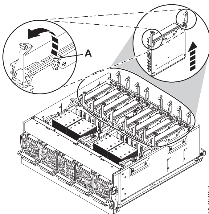
Figura 6. Removendo um riser de memória
