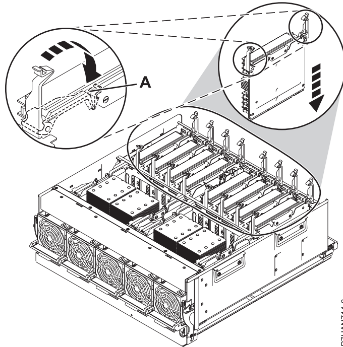
Figura 9. Substituindo um riser de memória
