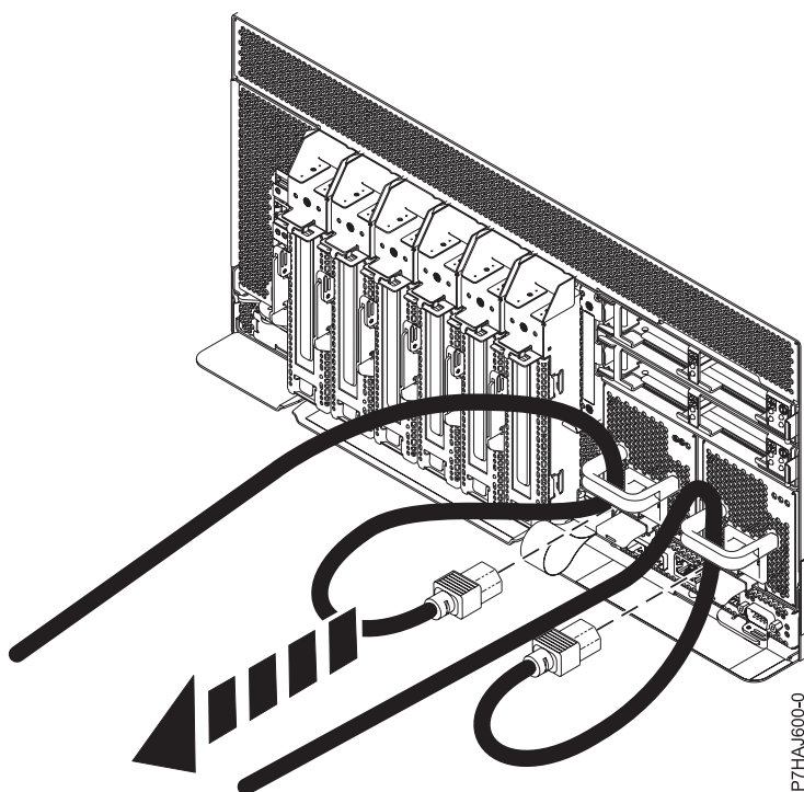
Figura 16. Desconectando os cabos de energia
