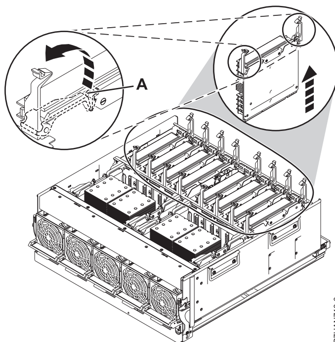
Figura 12. Removendo o riser de memória
