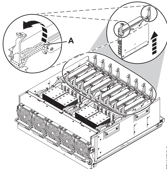
Figura 18. Removendo um riser de memória
