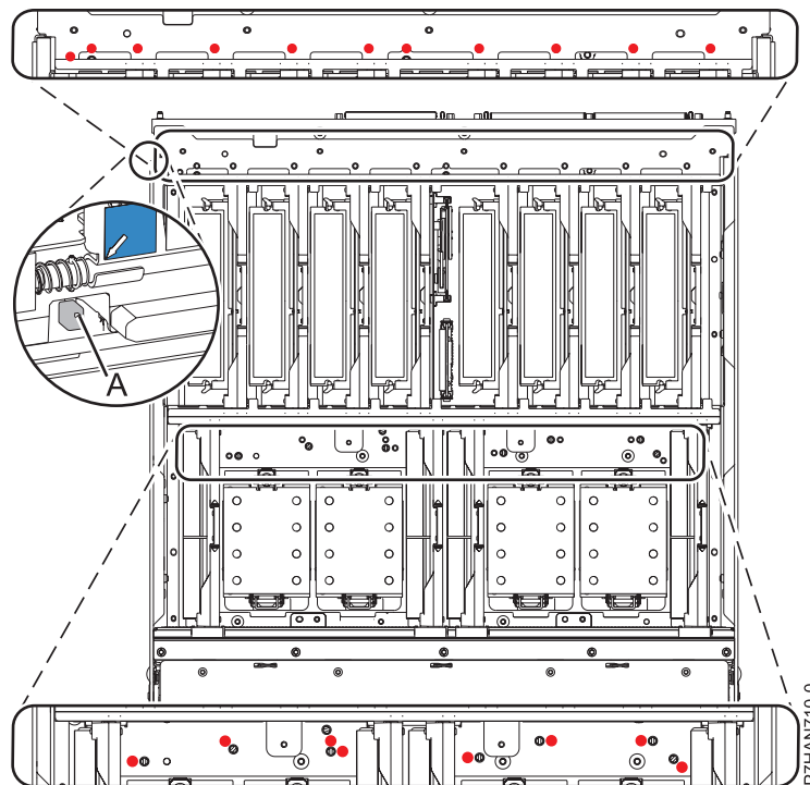
Figura 23. Botão de comando no planar
