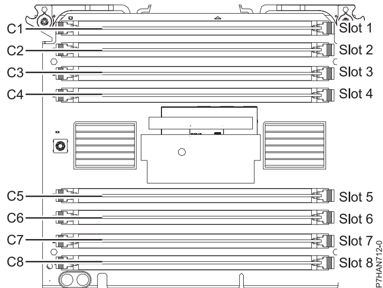
Figura 15. Locais dos slots de módulos de memória para o 8248-L4T,8408-E8D ou 9109-RMD
