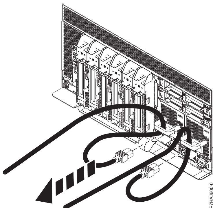
Figura 7. Desconectando os cabos de energia
