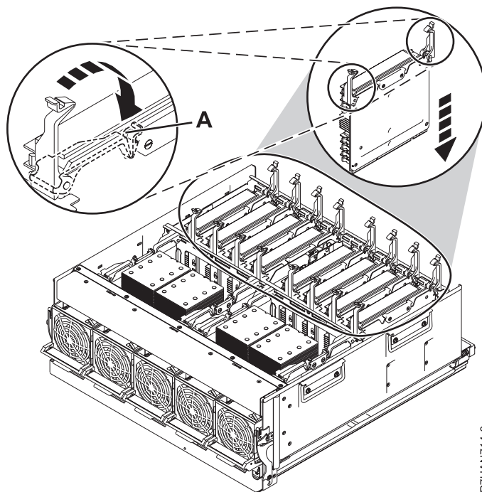
Figura 3. Instalando um riser de memória
