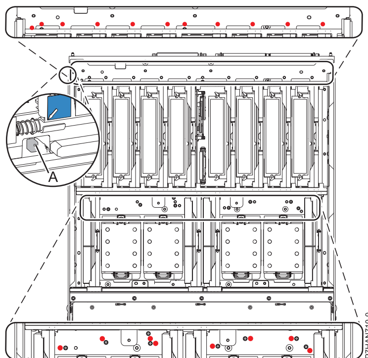
Figura 2. Botão de comando no planar
