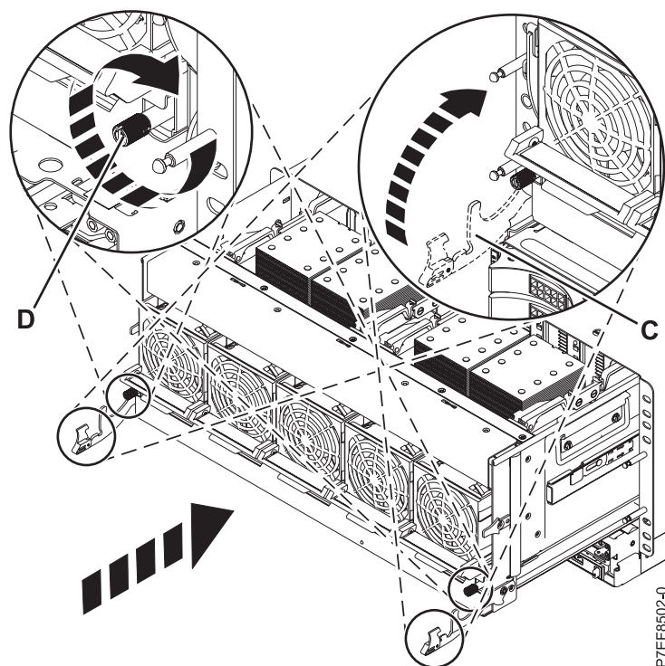
Figura 32. Bloqueando as travas de liberação da unidade de sistema
