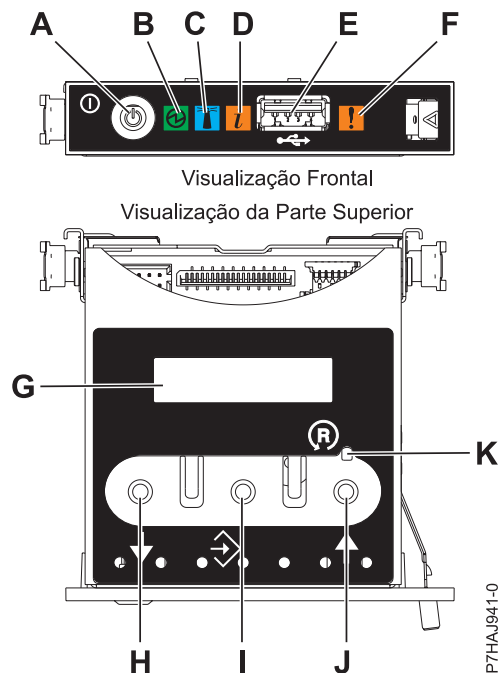
Figura 25. Painel de controle
