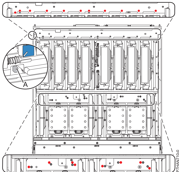
Figura 8. Botão de comando no planar
