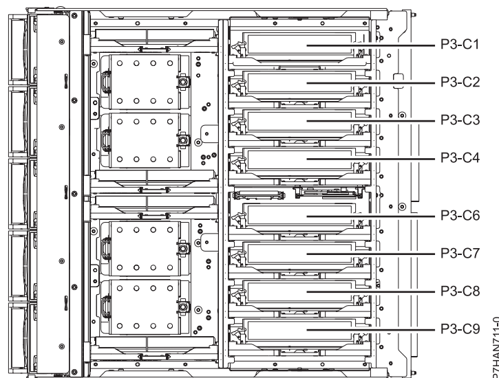
Figura 14. Sequência de plugging do riser de memória
