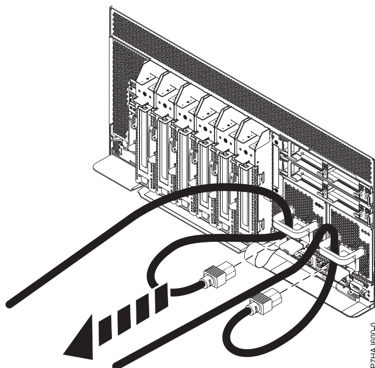
Figura 4. Desconectando os cabos de energia
