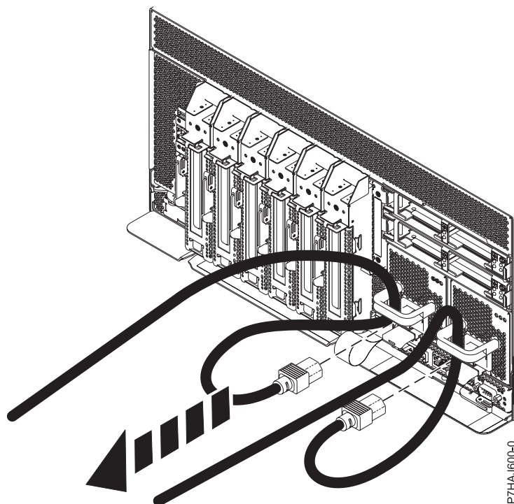
Figura 10. Desconectando os cabos de energia
