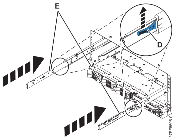
Figura 31. Desbloqueando as travas de segurança do trilho
