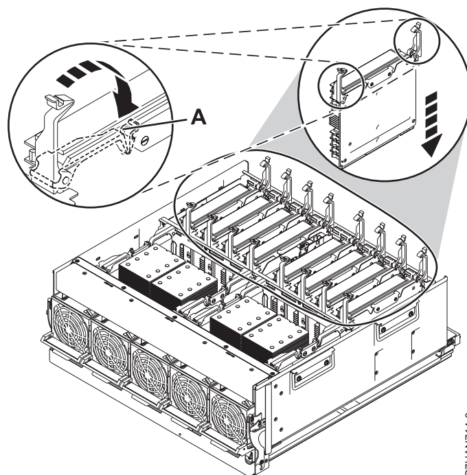
Figura 24. Substituindo um riser de memória
