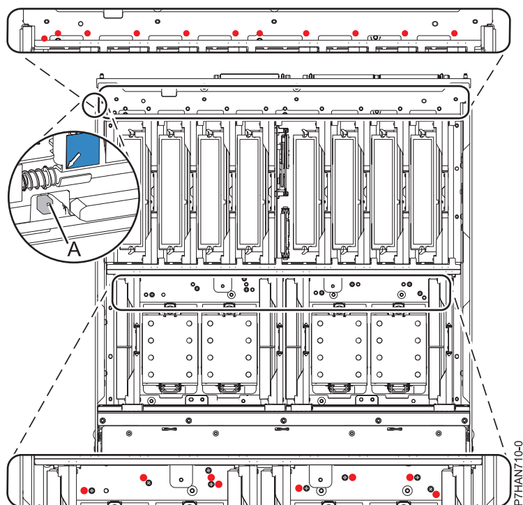
Figura 17. Botão de comando no planar
