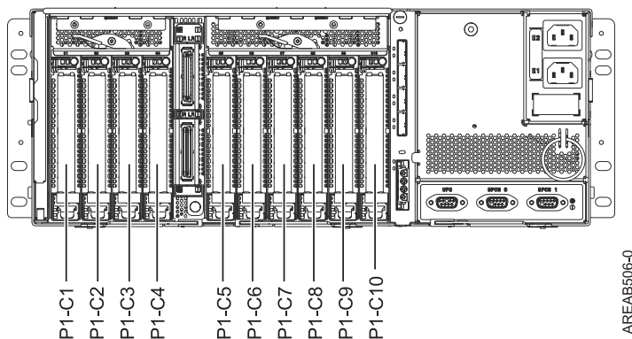
Figura 4. Vista posterior. Esta figura mostra a vista posterior da unidade de expansão.
