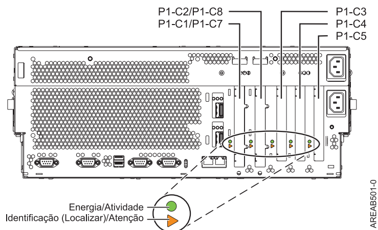
Figura 1. Vista Posterior do Sistema com Códigos de Local. Tabela 4 mostra a vista posterior do sistema com códigos de local para os slots de adaptador PCI e GX.
