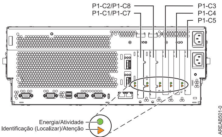
Figura 2. Vista Posterior do Gabinete com Códigos de Local. Tabela 11 mostra a vista posterior da unidade de sistema com os códigos de local para slots PCI e GX+.
