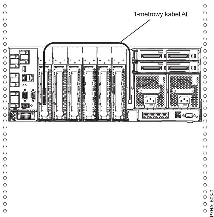
Rysunek 147. Podłączanie adaptera SAS do wewnętrznych gniazd dysków SAS za pośrednictwem zewnętrznego portu SAS systemu
