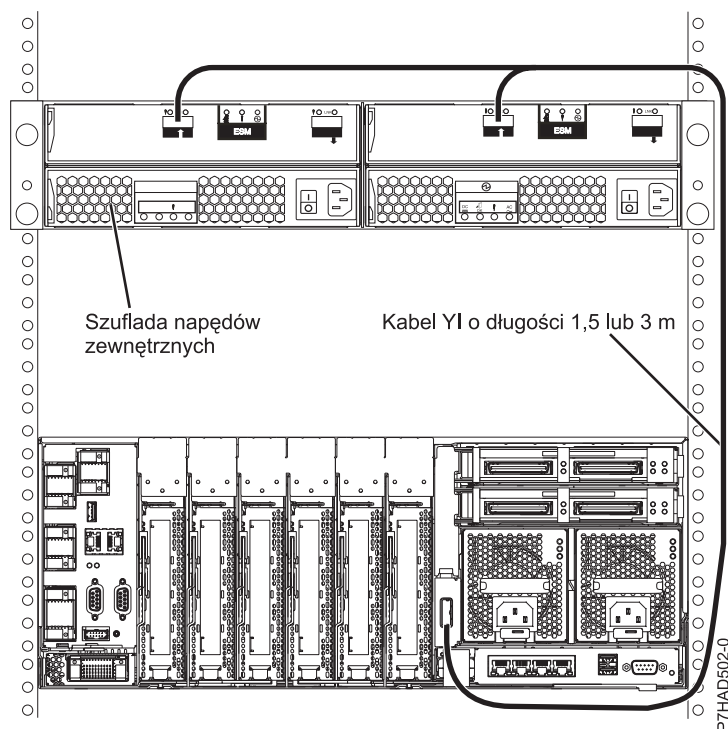
Rysunek 146. Podłączanie zewnętrznego systemowego portu adaptera SAS do szuflady rozszerzeń dysków (modele 9117-MMB i 9179-MHB)
