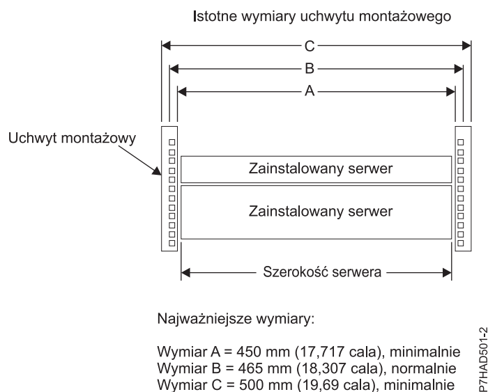
Rysunek 29. Istotne wymiary uchwytu montażowego
