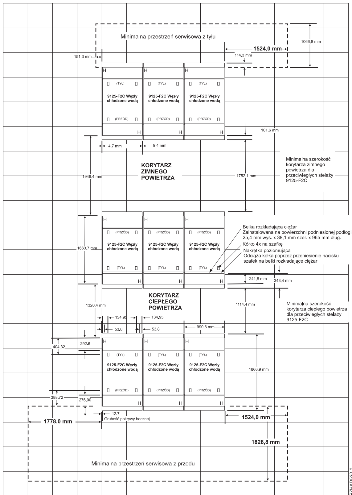
Rysunek 2. Przestrzeń serwisowa w przypadku wielu stelaży - korytarz ciepłego powietrza i korytarz zimnego powietrza
