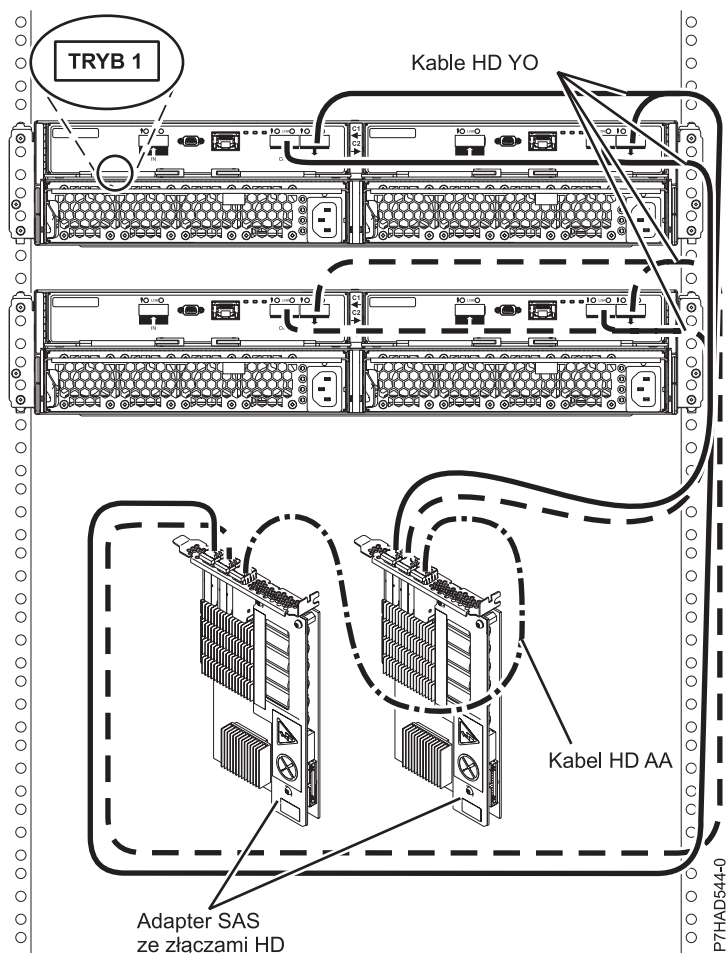
Rysunek 174. Połączenie trybu 1 dwu szuflad 5887 z użyciem złączy HD do dwóch adapterów SAS
