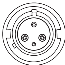
Rysunek 38. Gniazdo typu IEC 60309 P+N+E
