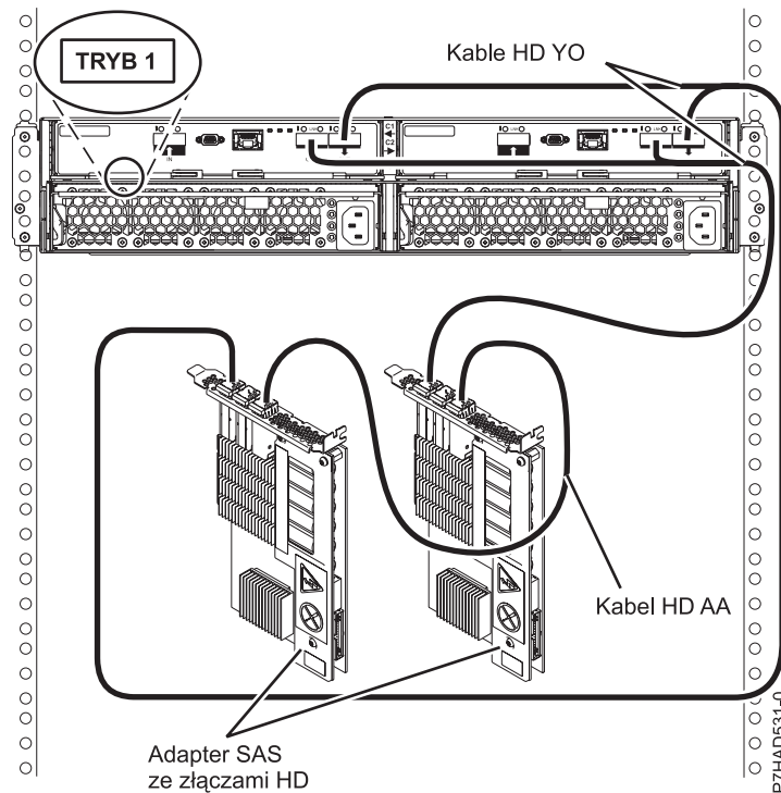
Rysunek 173. Połączenie trybu 1 szuflady 5887 do dwóch adapterów SAS ze złączami HD
