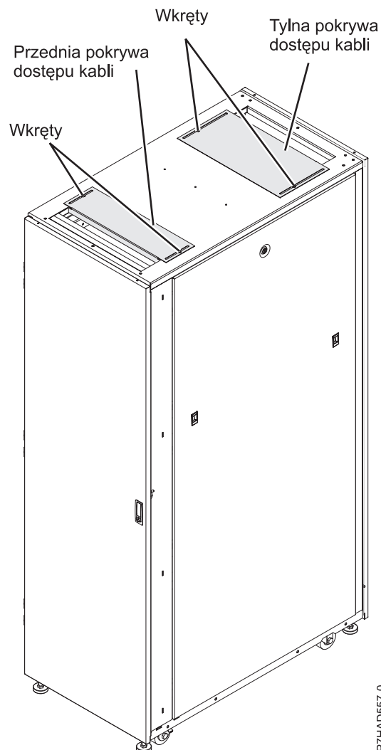
Rysunek 31. Pokrywy dostępu kabli
