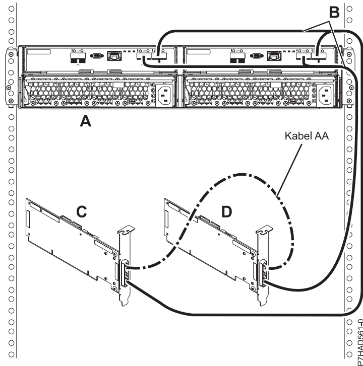
Rysunek 166. Połączenie trybu 2 szuflady 5887 z użyciem kabli YO do dwóch pojedynczych adapterów SAS
