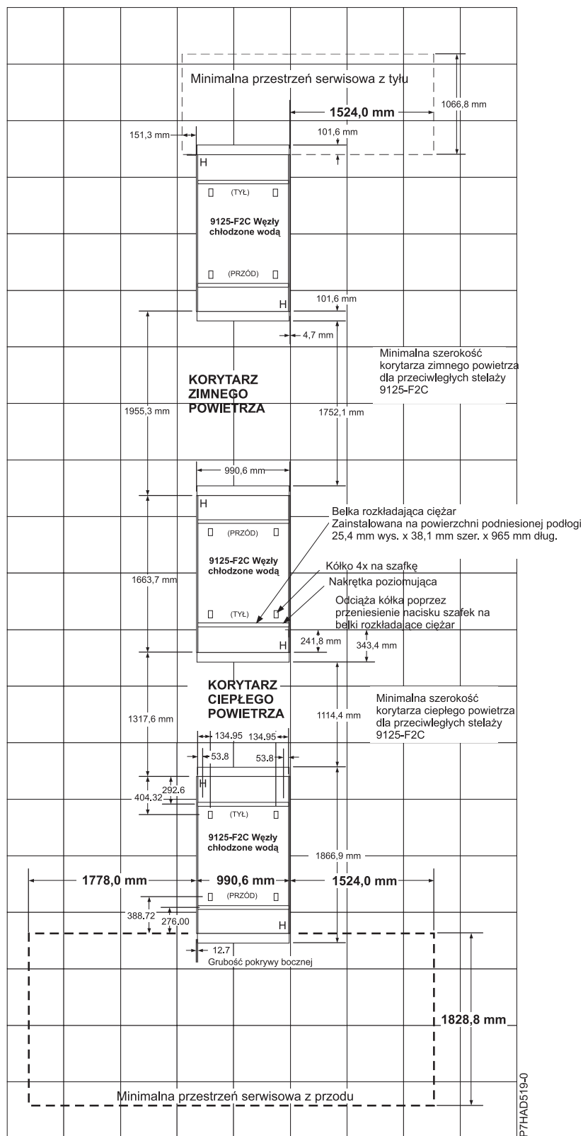
Rysunek 1. Przestrzeń serwisowa w przypadku jednego stelaża - korytarz ciepłego powietrza i korytarz zimnego powietrza
