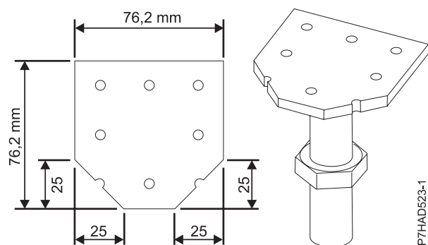
Rysunek 4. Wymiary przyciętych cokołów
