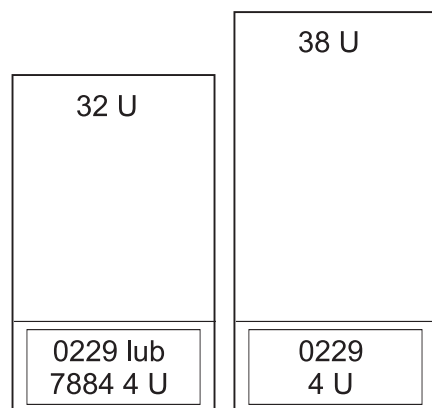
Rysunek 10. Kod opcji 7884: serwery 9406-520 i 9111-520 w stelażu
