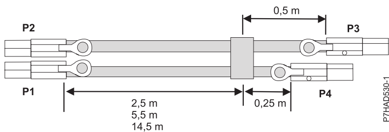
Rysunek 142. Długości kabli w zestawie zewnętrznych kabli X do adapterów SAS
