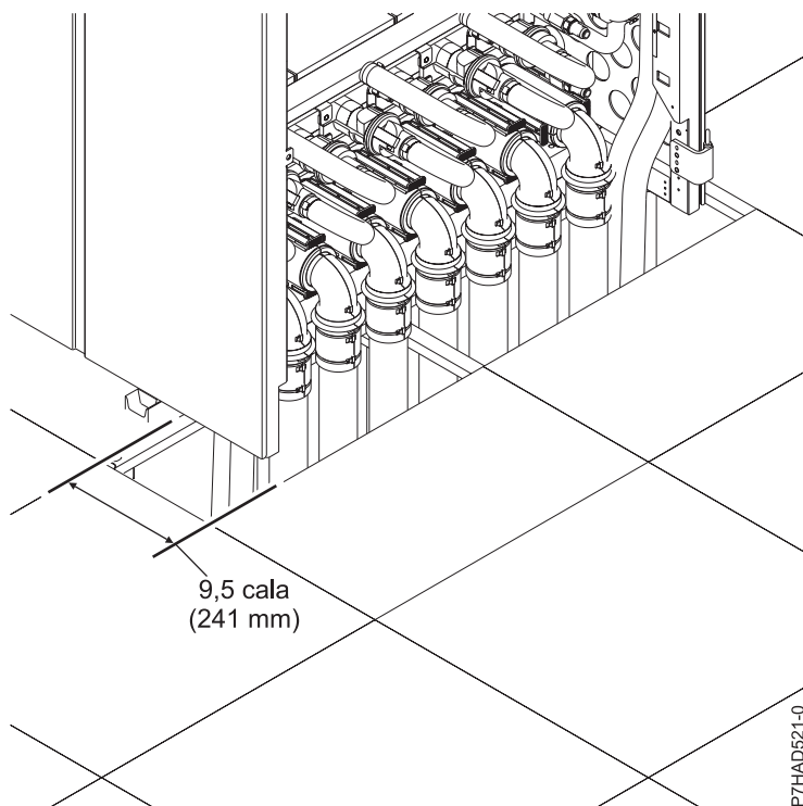
Rysunek 3. Wycięcie w podłodze
