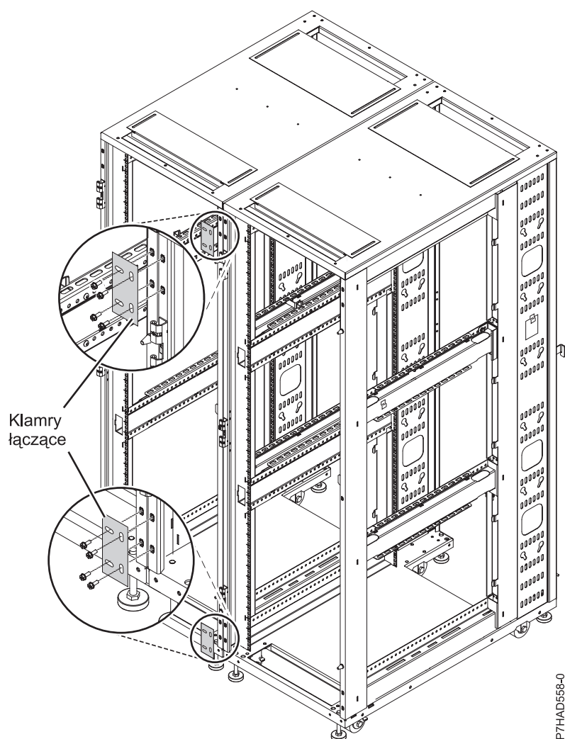
Rysunek 33. Klamry łączące
