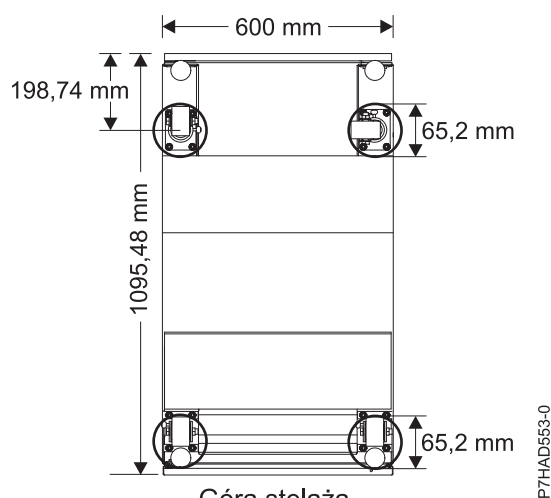
Rysunek 28. Rozmieszczenie kółek
