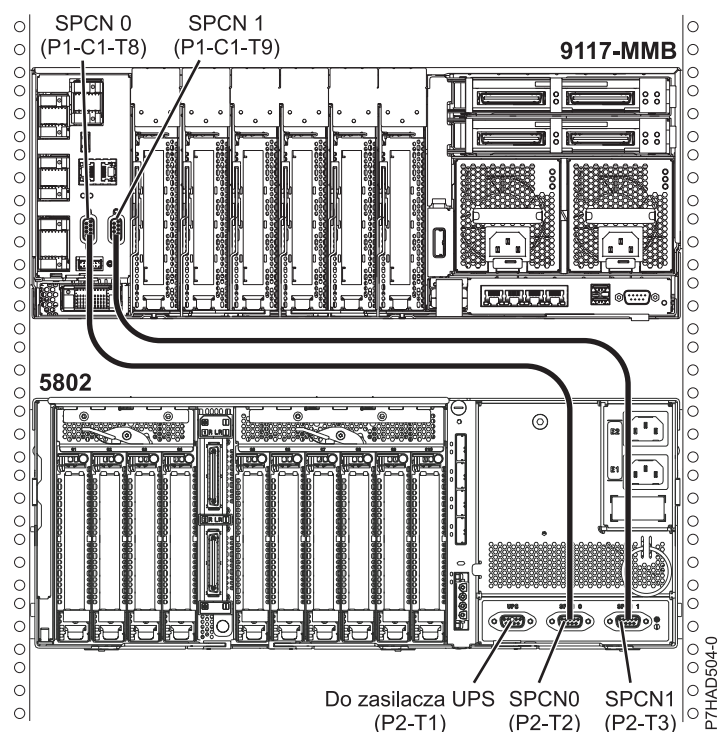
Rysunek 135. Widok z tyłu serwerów 8412-EAD, 9117-MMB, 9117-MMC, 9117-MMD, 9179-MHB, 9179-MHC i 9179-MHD oraz jednostek rozszerzeń 5208 i 5877 - miejsce podłączenia kabli
