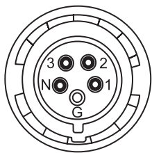
Rysunek 36. Rozmieszczenie wtyków
