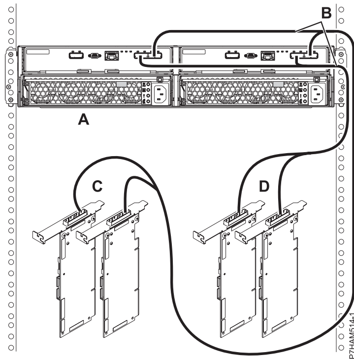
Rysunek 167. Połączenie trybu 2 szuflady 5887 z użyciem kabli X do dwóch par adapterów SAS
