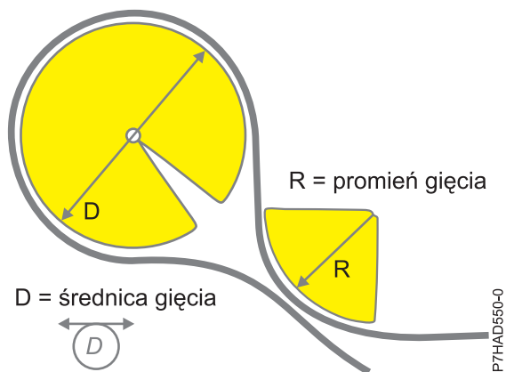
Rysunek 140. Promień gięcia kabla
