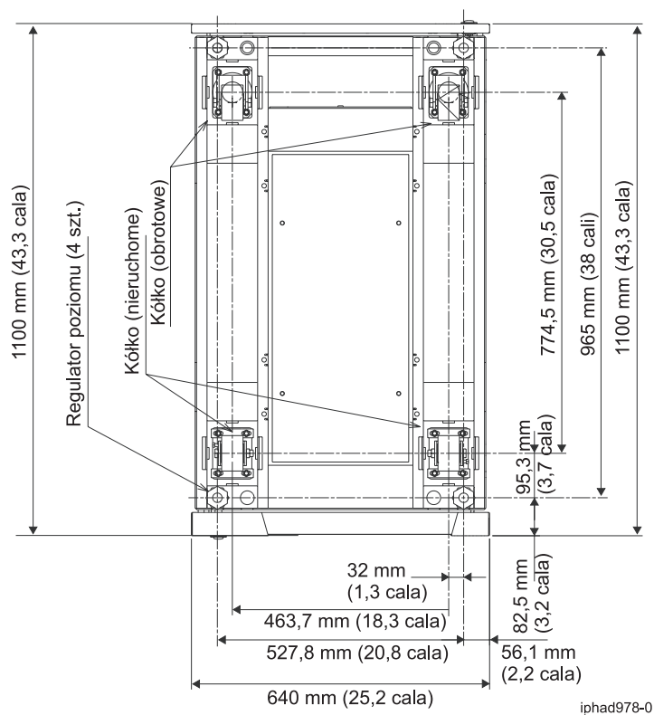
Rysunek 9. Miejsce kółek i regulatora poziomu
