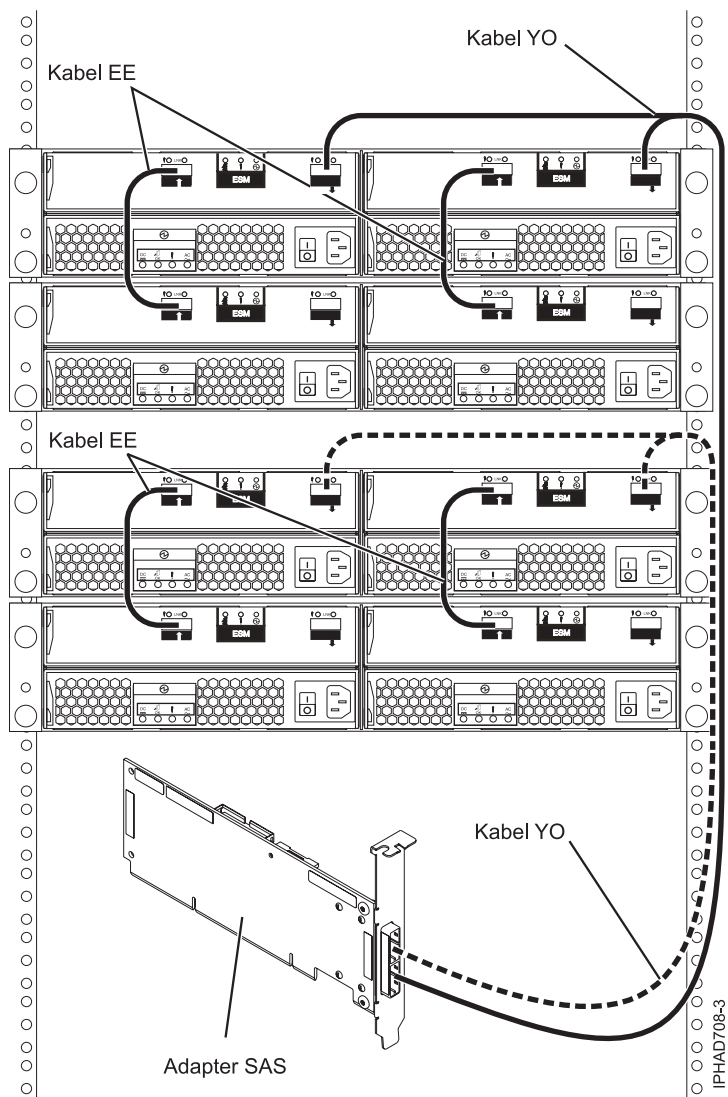
Rysunek 147. Podłączenie adaptera SAS do czterech szuflad rozszerzeń dysków
