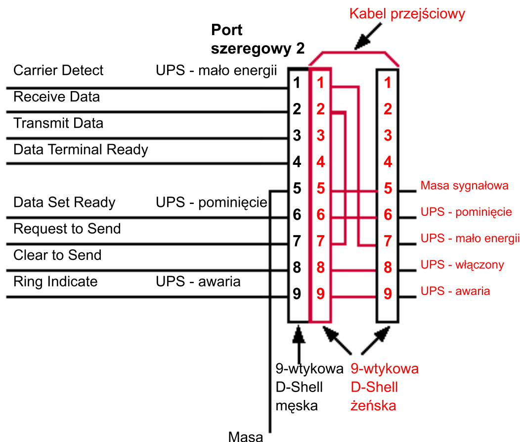
Rysunek 132. Podłączanie kabla 1827
