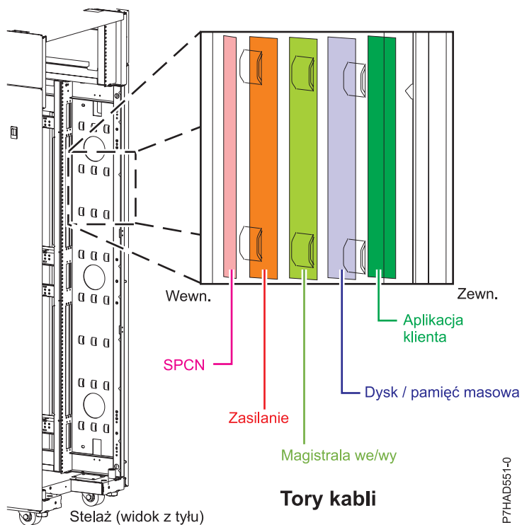
Rysunek 139. Nacięcia mostowe do zarządzania kablami
