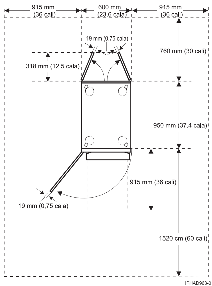
Rysunek 24. Widok planarny stelaży 0555 i 7014-S25
