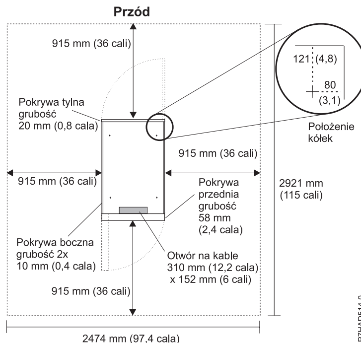
Rysunek 27. Wolne przestrzenie serwisowe i rozmieszczenie kólek w stelażach 7014-T00, 7014-T42 i 0553
