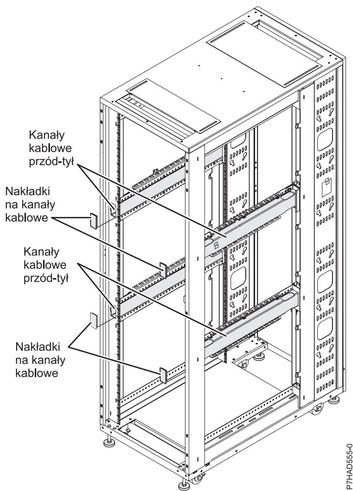
Rysunek 29. Kable wewnątrz stelaża
