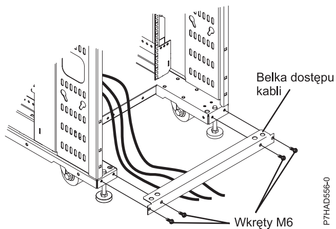
Rysunek 30. Belka dostępu kabli
