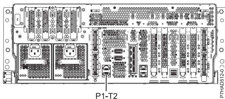
Rysunek 137. Widok z tyłu serwerów 8202-E4B, 8202-E4C, 8202-E4D, 8205-E6B, 8205-E6C i 8205-E6D — miejsce podłączenia kabli
