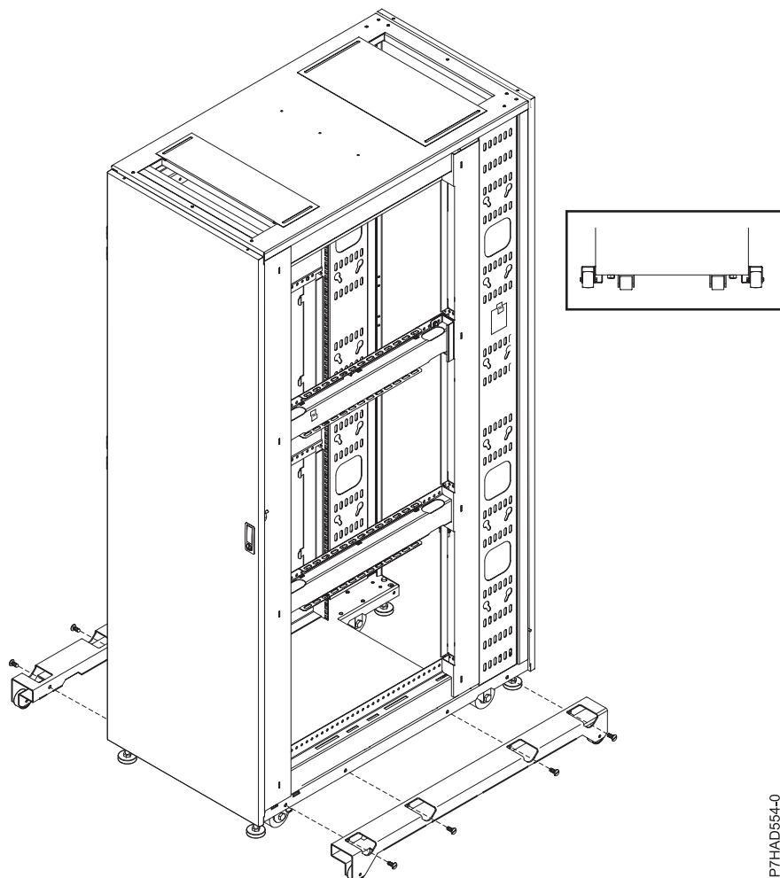
Rysunek 32. Rozmieszczenie wysuwnic
