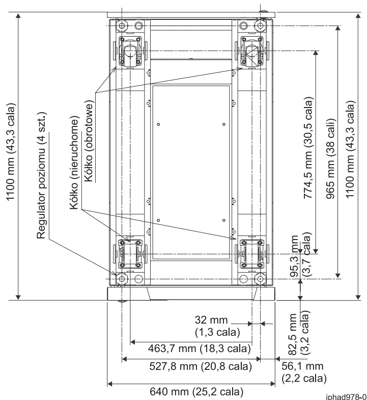
Rysunek 26. Miejsce kółek i regulatora poziomu
