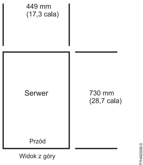
Rysunek 1. Widok planarny serwerów stelażowych 8202-E4B, 8202-E4C, 8202-E4D, 8205-E6B, 8205-E6C i 8205-E6D
