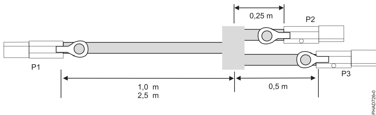
Rysunek 140. Długości kabli w zestawie zewnętrznych kabli Y1 do adapterów SAS
