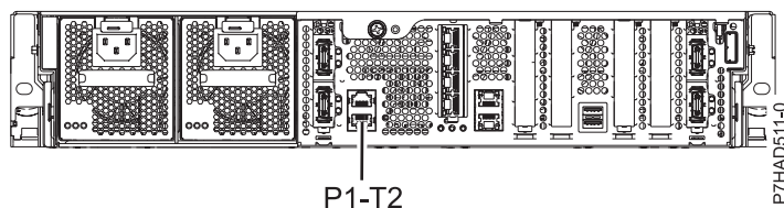
Rysunek 132. Widok z tyłu serwerów 8231-E2B, 8231-E1C, 8231-E1D, 8231-E2C, 8231-E2D i 8268-E1D - miejsce podłączenia kabli
