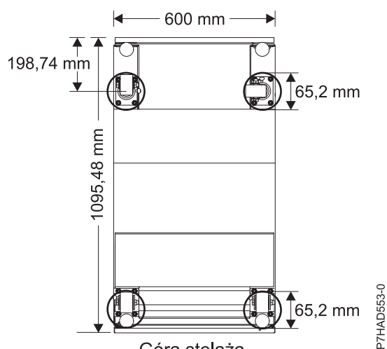
Rysunek 24. Rozmieszczenie kółek
