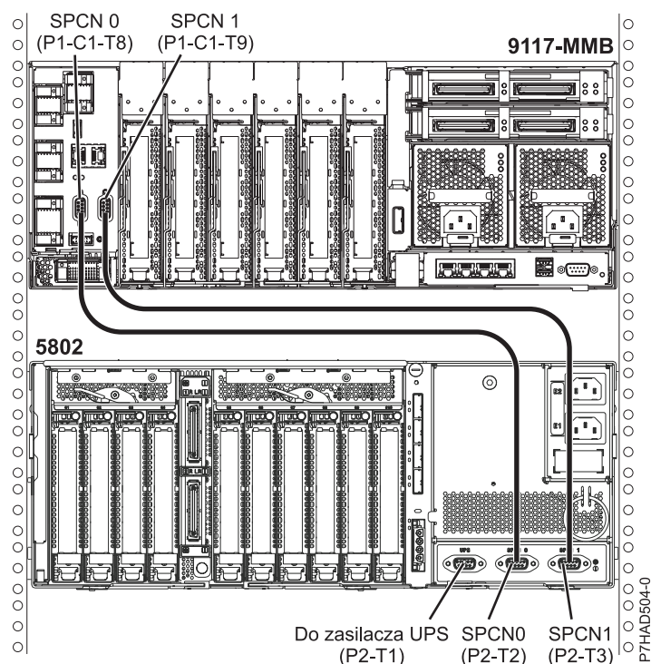
Rysunek 131. Widok z tyłu serwerów 8412-EAD, 9117-MMB, 9117-MMC, 9117-MMD, 9179-MHB, 9179-MHC i 9179-MHD oraz jednostek rozszerzeń 5208 i 5877 - miejsce podłączenia kabli
