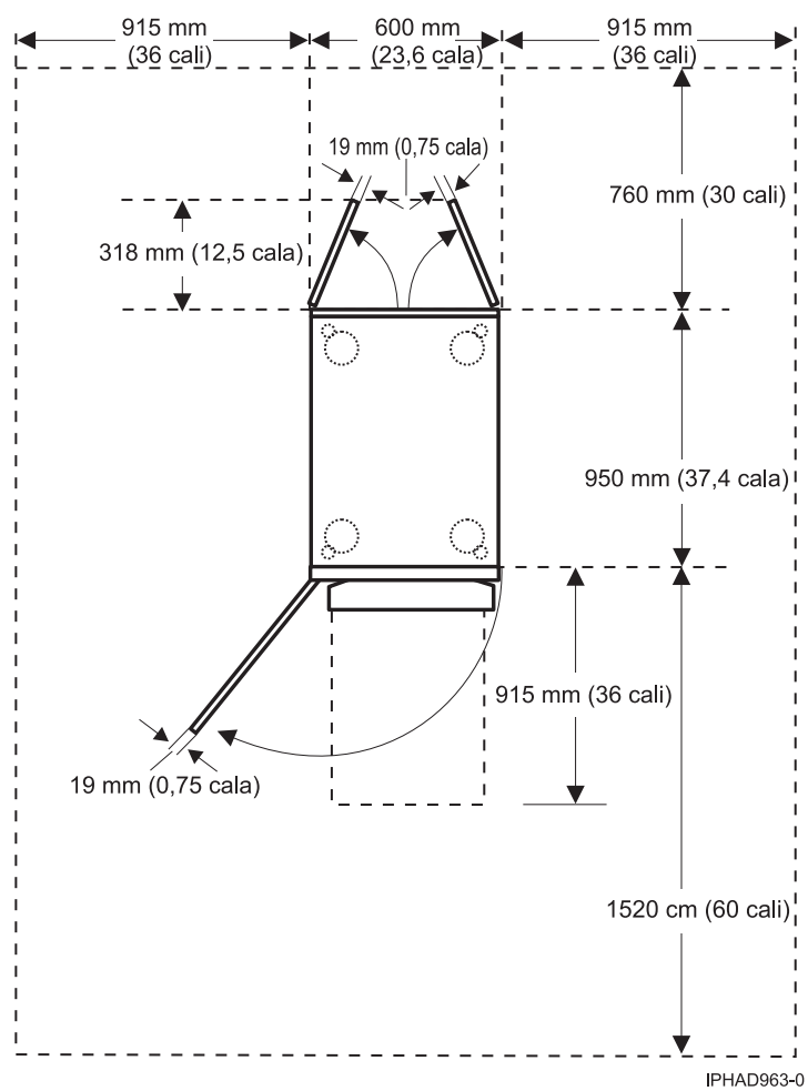
Rysunek 20. Widok planarny stelaży 0555 i 7014-S25
