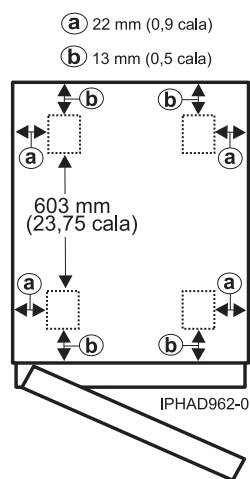
Rysunek 18. Rozmieszczenie kółek w stelażach 0554 i 7014-S11
