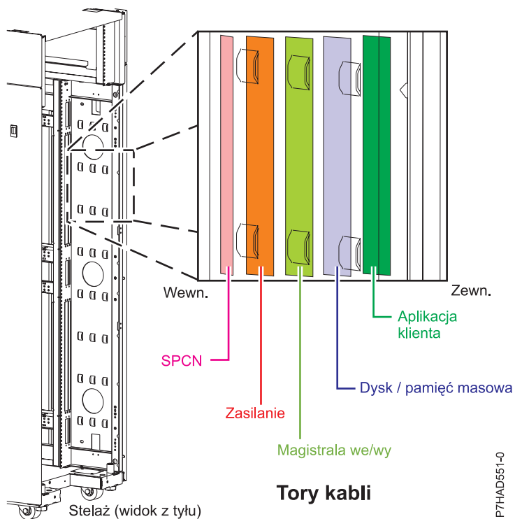
Rysunek 135. Nacięcia mostowe do zarządzania kablami
