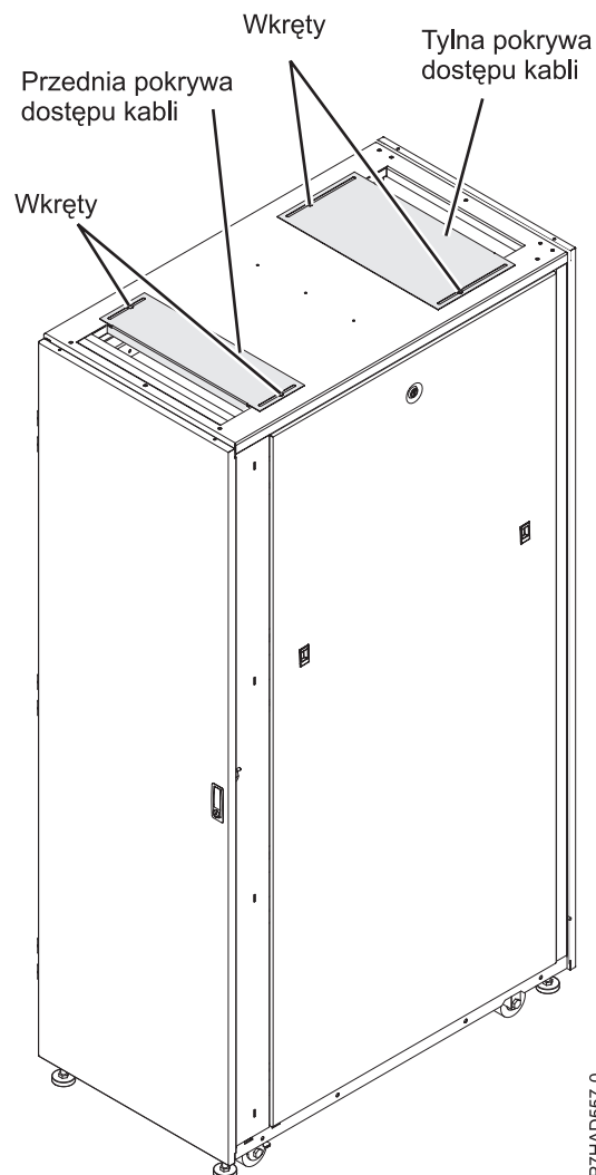
Rysunek 27. Pokrywy dostępu kabli
