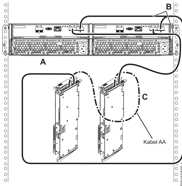
Rysunek 168. Połączenie trybu 1 szuflady 5887 z użyciem kabli YO do podwójnych adapterów SAS
