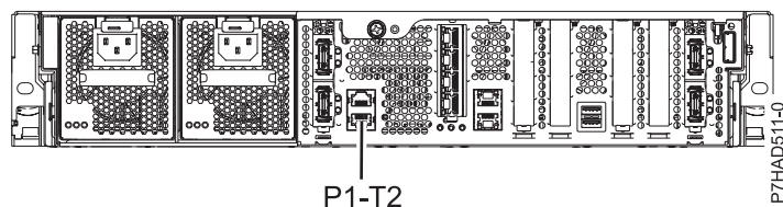
Rysunek 132. Widok z tyłu serwerów 8231-E2B, 8231-E1C, 8231-E1D, 8231-E2C, 8231-E2D i 8268-E1D - miejsce podłączenia kabli
