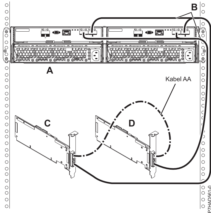
Rysunek 162. Połączenie trybu 2 szuflady 5887 z użyciem kabli YO do dwóch pojedynczych adapterów SAS
