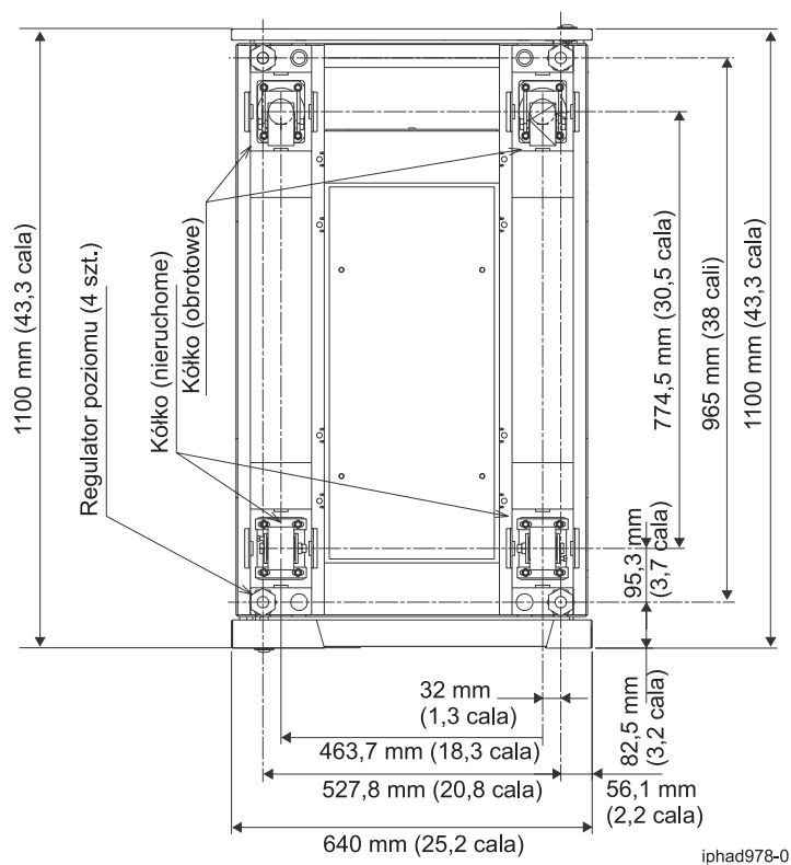
Rysunek 5. Miejsce kółek i regulatora poziomu
