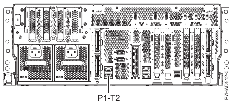
Rysunek 133. Widok z tyłu serwerów 8202-E4B, 8202-E4C, 8202-E4D, 8205-E6B, 8205-E6C i 8205-E6D — miejsce podłączenia kabli
