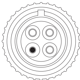
Rysunek 114. Wtyczka typu RS 7328DP
