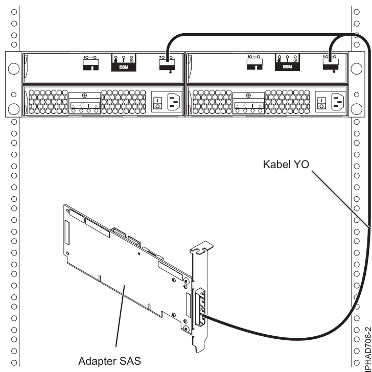
Rysunek 141. Podłączanie adaptera SAS do szuflady rozszerzeń dysków
