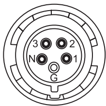
Rysunek 32. Rozmieszczenie wtyków
