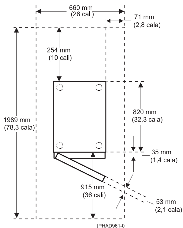
Rysunek 17. Widok planarny stelaży 0554 i 7014-S11
