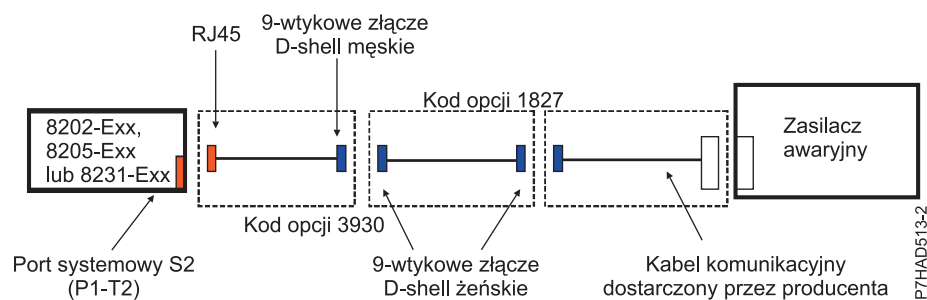
Rysunek 134. Okablowanie zasilaczy awaryjnych serwerów 8202-E4B, 8202-E4C, 8205-E6B, 8205-E6C, 8231-E2B, 8231-E1C, 8231-E1D, 8231-E2C, 8231-E2D i 8268-E1D
