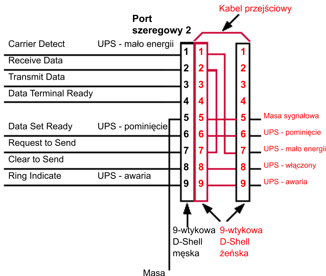
Rysunek 128. Podłączanie kabla 1827
