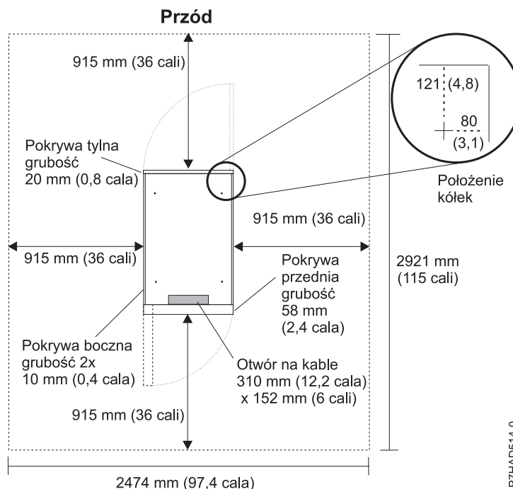
Rysunek 23. Wolne przestrzenie serwisowe i rozmieszczenie kótek w stelażach 7014-T00, 7014-T42 i 0553
