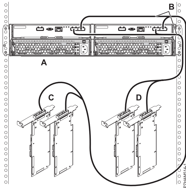
Rysunek 163. Połączenie trybu 2 szuflady 5887 z użyciem kabli X do dwóch par adapterów SAS
