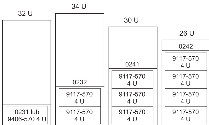
Rysunek 8. 570 w stelażu
