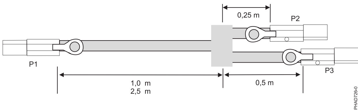
Rysunek 140. Długości kabli w zestawie zewnętrznych kabli YI do adapterów SAS
