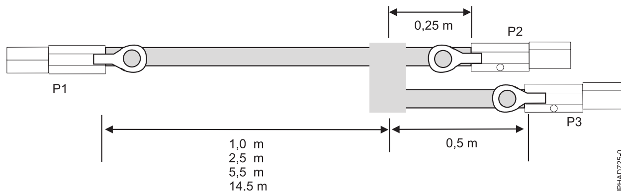
Rysunek 139. Długości kabli w zestawie zewnętrznych kabli YO do adapterów SAS
