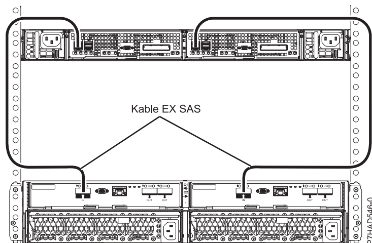
Rysunek 173. Połączenie jednej szuflady 5887 za pomocą kabli HD EX do jednej obudowy EDR1
