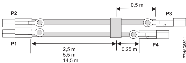
Rysunek 138. Długości kabli w zestawie zewnętrznych kabli X do adapterów SAS
