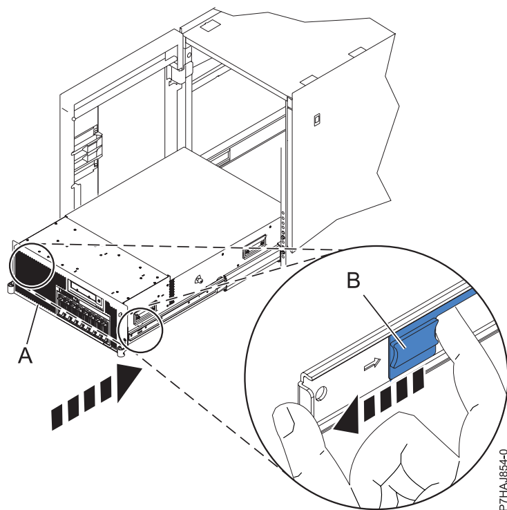
Rysunek 18. Zwalnianie zatrzasków blokady prowadnicy
