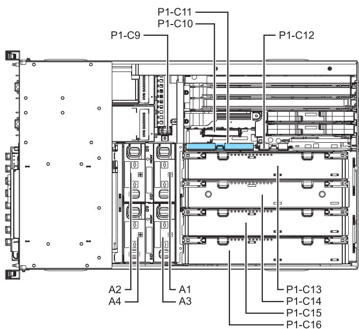
Rysunek 9. Położenie gniazda do instalacji karty udostępniania RAID
