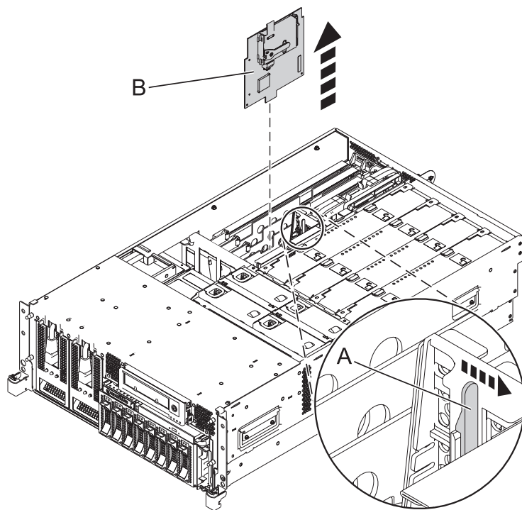
Rysunek 5. Demontaż karty pamięci podręcznej RAID ze stelażowej jednostki systemowej
