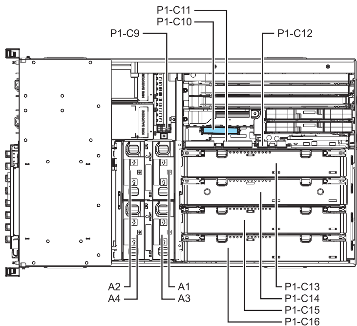
Rysunek 3. Położenie gniazda do instalowania pomocniczej karty pamięci podręcznej
