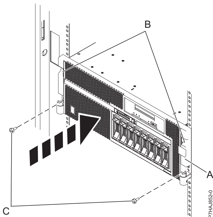
Rysunek 19. Instalowanie wkrętów płytkowych
