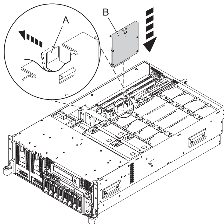
Rysunek 10. Wymiana karty udostępniania RAID w stelażowej jednostce systemowej
