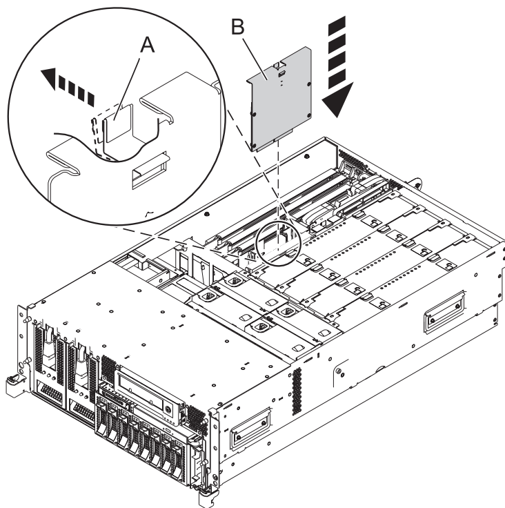
Rysunek 2. Wymiana karty udostępniania RAID w serwerach stelażowych
