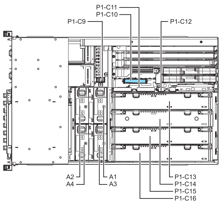
Rysunek 6. Położenie gniazda pomocniczej karty pamięci podręcznej RAID
