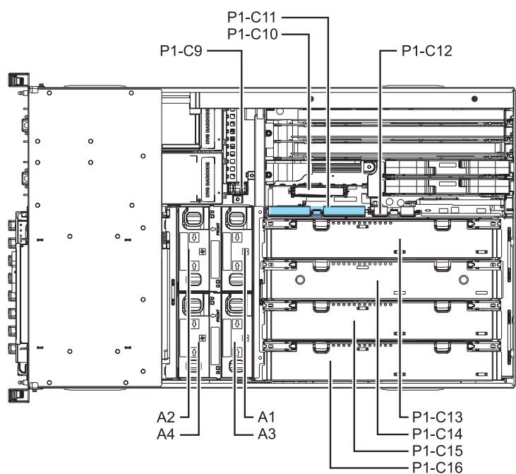
Rysunek 1. Położenie gniazda do instalacji karty udostępniania RAID
