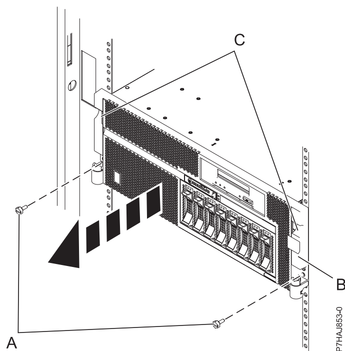
Rysunek 13. Demontaż przedniej pokrywy
