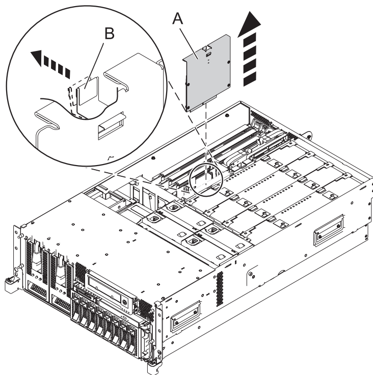
Rysunek 8. Demontaż karty udostępniania RAID ze stelażowej jednostki systemowej
