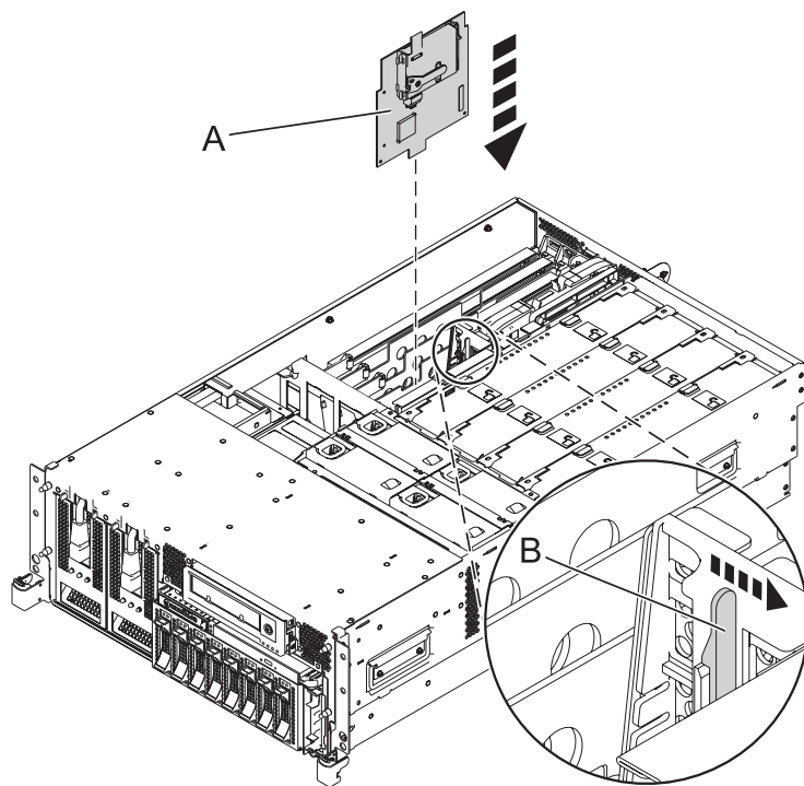
Rysunek 4. Model stelażowy - wymiana pomocniczej karty pamięci podręcznej RAID
