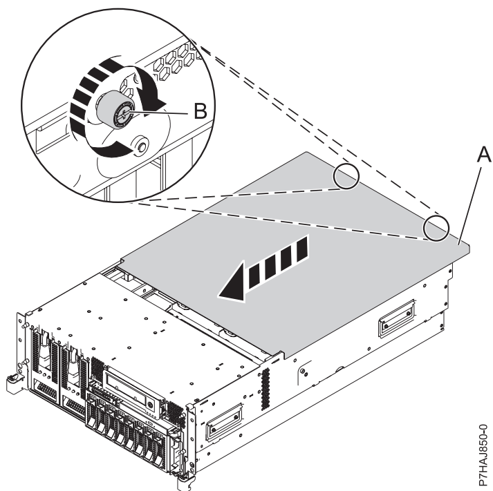
Rysunek 16. Instalowanie pokrywy dostępu serwisowego
