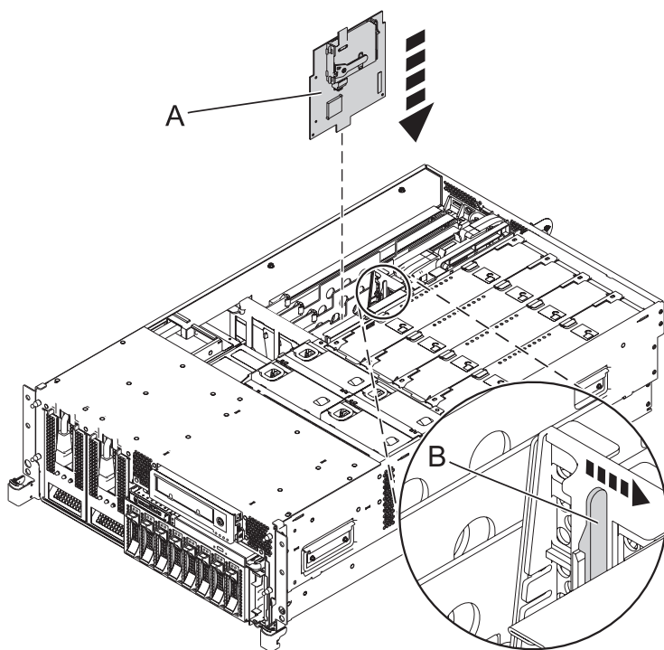
Rysunek 7. Wymiana pomocniczej karty pamięci podręcznej RAID w serwerach stelażowych
