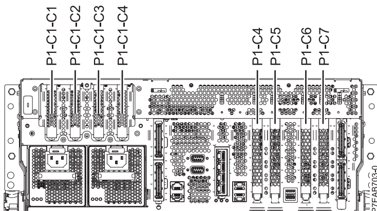
Rysunek 1. Widok serwerów 8202-E4B i 8205-E6B z tyłu wraz z kodami położenia gniazd PCI
