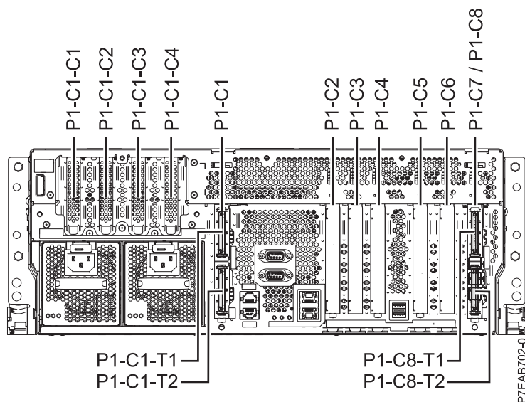
Rysunek 4. Widok serwerów z tyłu, z widocznymi gniazdami PCI i ich kodami położenia
