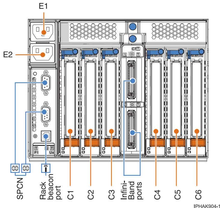
Rysunek 5. Widok z tyłu
