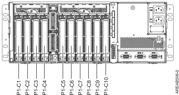
Rysunek 6. Widok z tyłu. Rysunek przedstawia widok jednostki rozszerzeń z tyłu.
