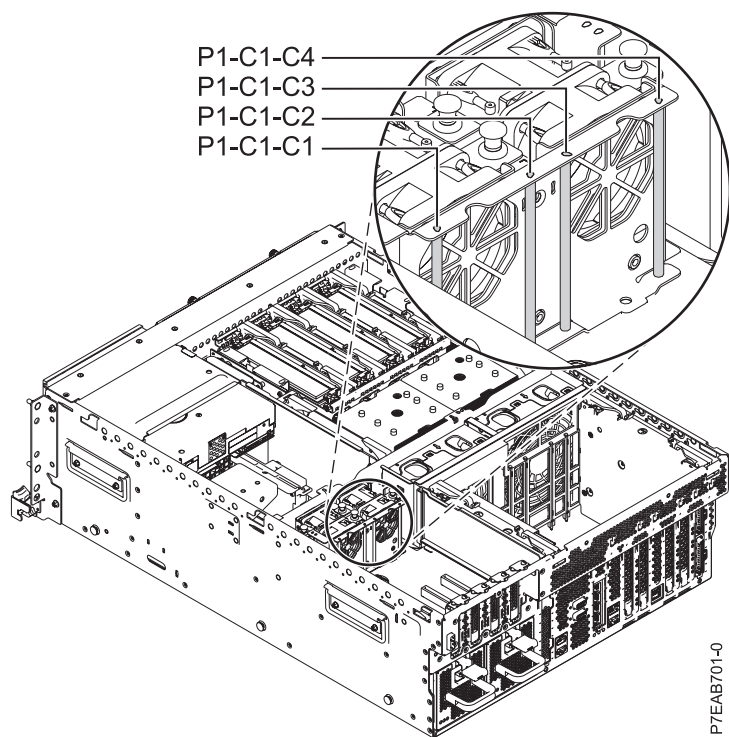
Rysunek 3. Karta nośna PCI z kodami położenia w serwerach 8202-E4B i 8205-E6B
