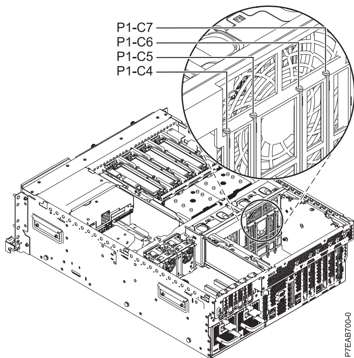
Rysunek 2. Kody położenia gniazd PCI w serwerach 8202-E4B i 8205-E6B
