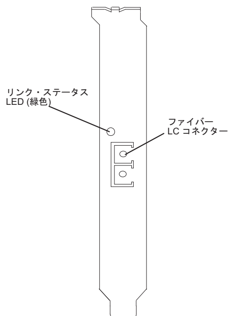
図 29. 1 ギガビット SX iSCSI TOE PCI-X アダプター上の LED
