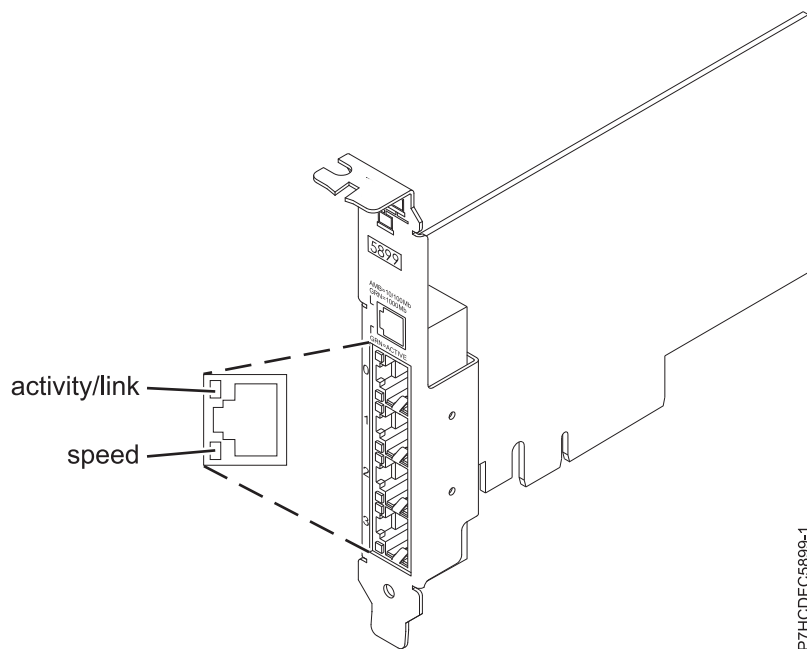
図 42. アダプター
