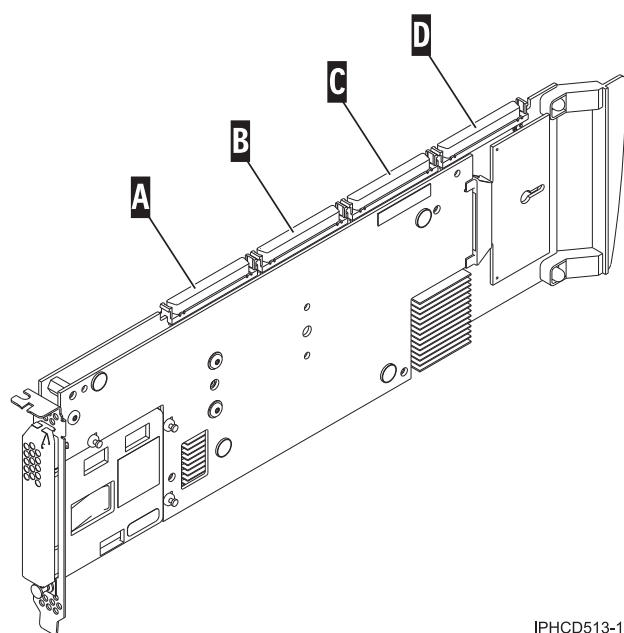
図 73. アダプター SCSI コネクター
