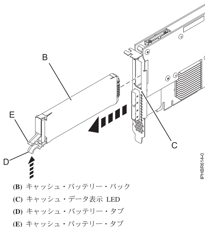
図 85. 574E キャッシュ・バッテリーの取り替え
