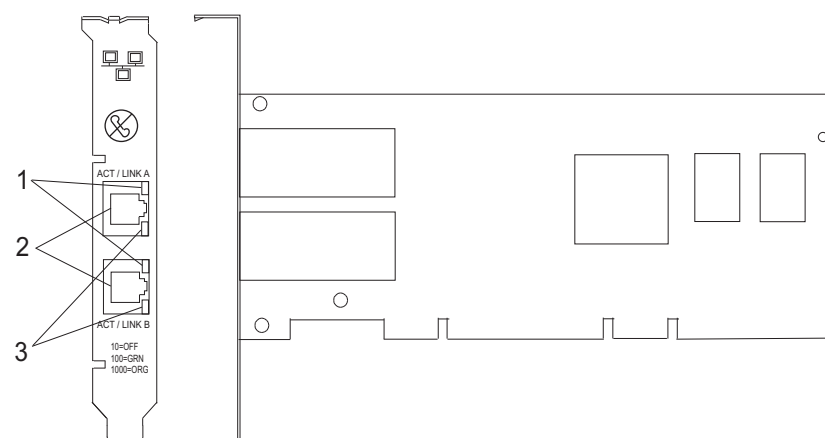
図 24. 2 ポート 10/100/1000 Base-TX イーサネット PCI-X アダプター
