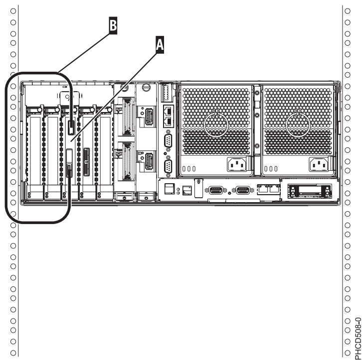
図 64. フィーチャー 5911 が取り付けられ、ケーブル接続された状態のシステムの背面図
