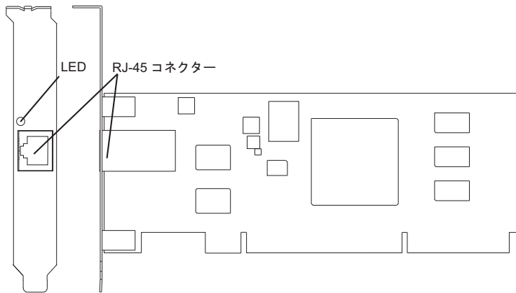
図 28. 1 ギガビット TX iSCSI TOE PCI-X アダプター
