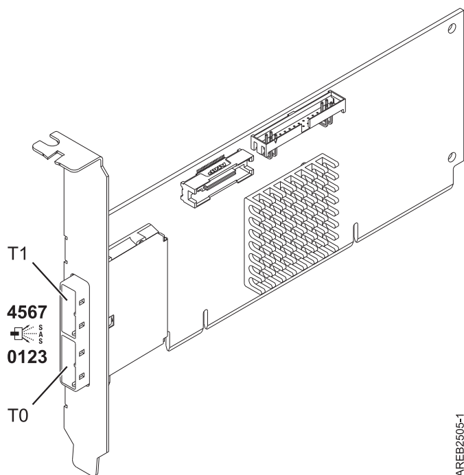
図 65. PCI-X DDR External Dual -x4 ポート SAS アダプター
