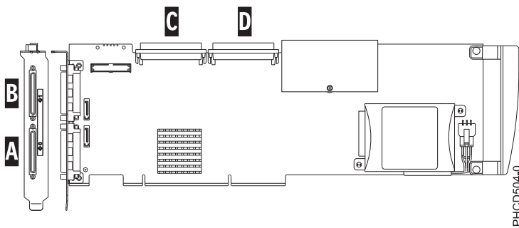
図 71. PCI-X DDR デュアル・チャネル Ultra320 SCSI RAID アダプター
