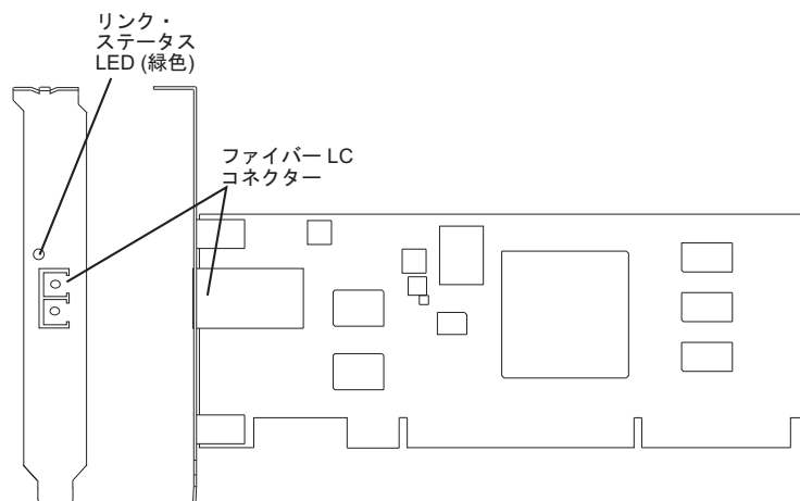
図 27. 1 ギガビット SX iSCSI TOE PCI-X アダプター
