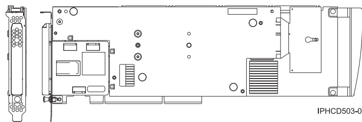
図 68. アダプター側面図と端面図
