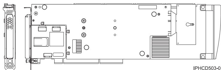
図 72. アダプター側面図と端面図
