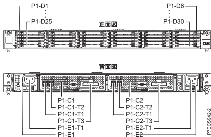
図 78. PCIe2 3.1GB キャッシュ統合 SAS RAID アダプターのロケーション・コード
