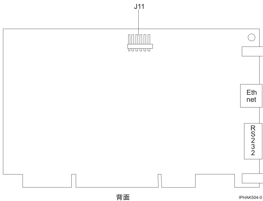
図 52. アダプター背面
