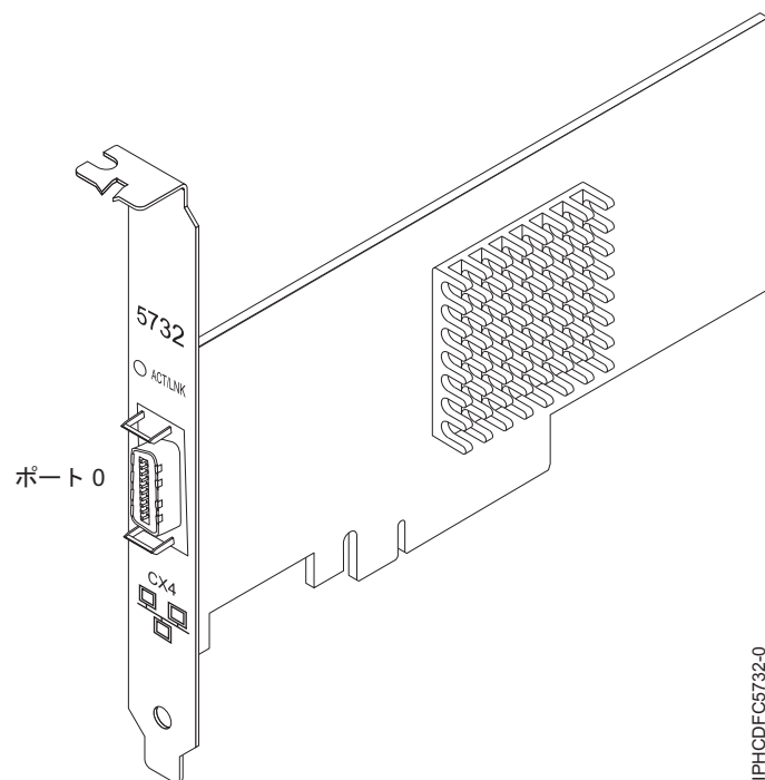
図 32. 10 ギガビット・イーサネット CX4 PCI Express (PCIe) アダプター
