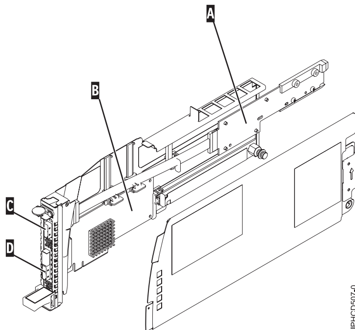
図 61. カセット内の PCI Express x8 Ext Dual -x4 3 Gb SAS アダプターおよびテーブル・カード
