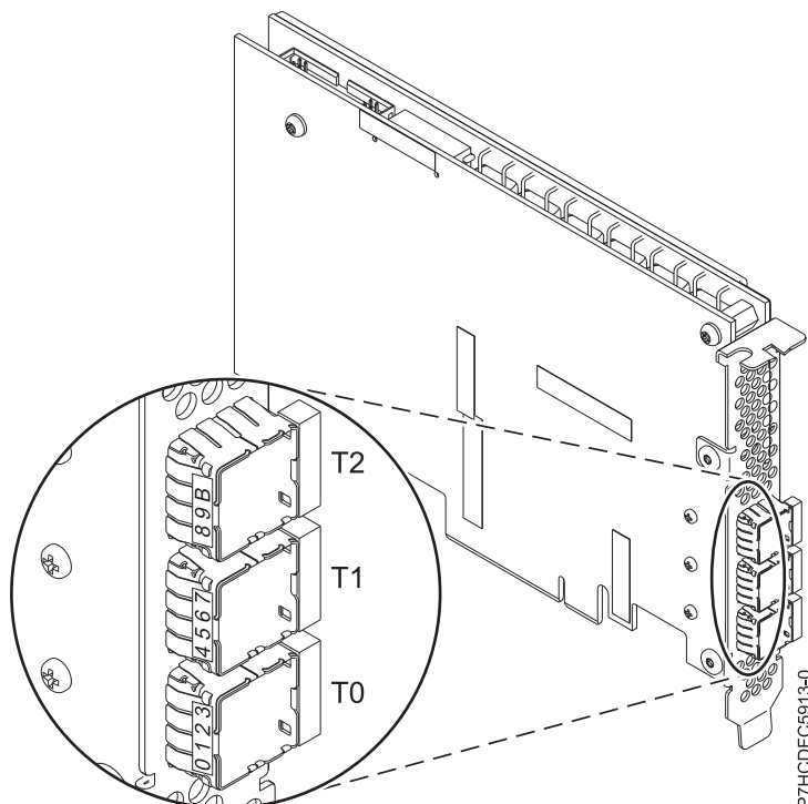
図 66. 5913 アダプター
