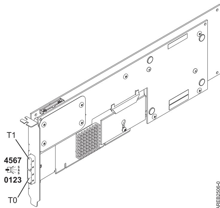
図 58. PCI-X DDR デュアル -x4 ポート SAS RAID アダプター
