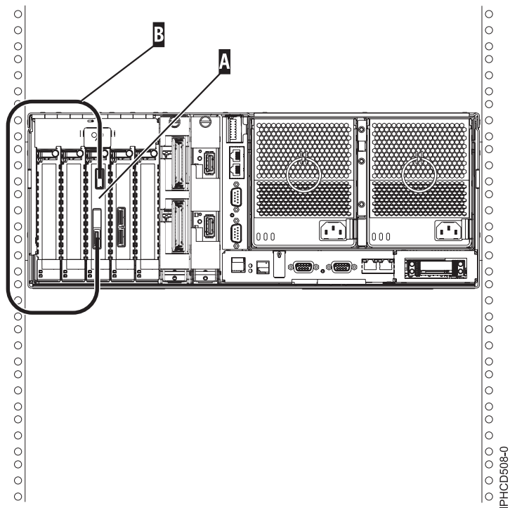
図 62. フィーチャー 5909 が取り付けられ、ケーブル接続された状態での、システム装置の背面図
