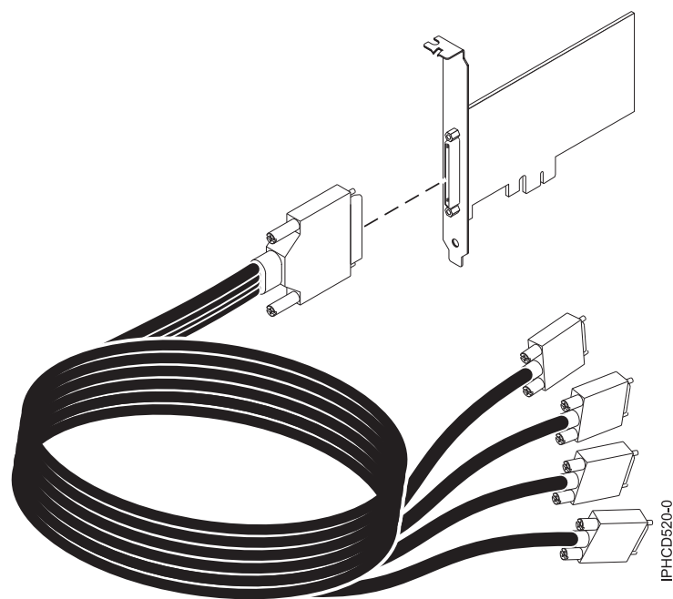
図 7. ケーブル
