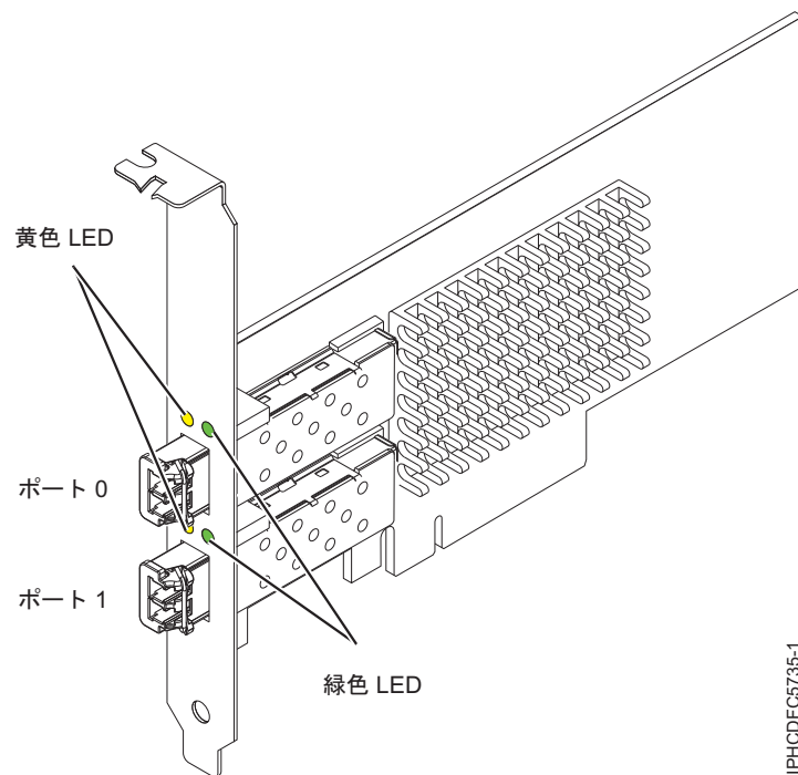
図 14. EN0A アダプター
