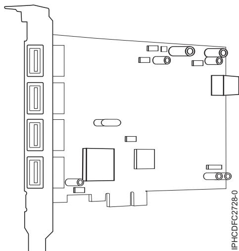
図 50. 4 ポート USB PCIe アダプター
