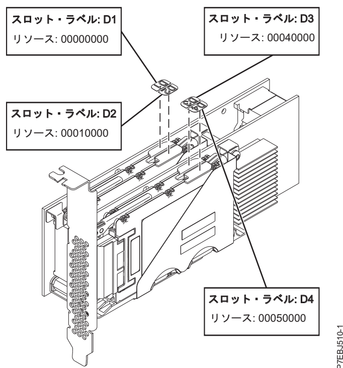
図 54. PCIe デュアル x4 3 Gb SAS RAID アダプター
