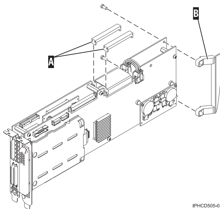
図 75. アダプターをカセットに配置する準備
