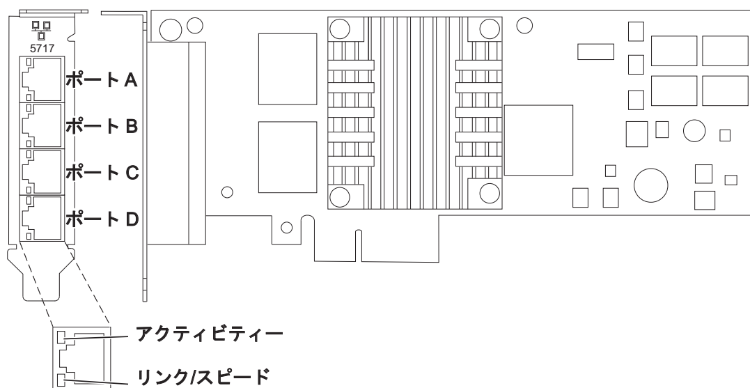
図 31. 4 ポート 10/100/1000 Base-TX PCIe アダプター
