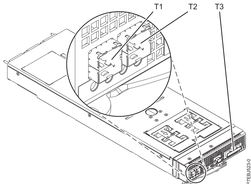
図 79. CCIN 57C3 PCIe2 3.1GB キャッシュ RAID SAS エンクロージャー 6Gb x8
