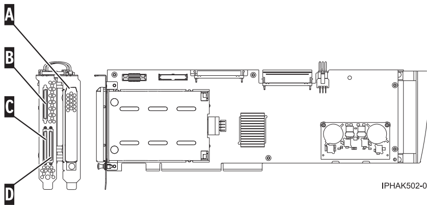
図 74. アダプター
