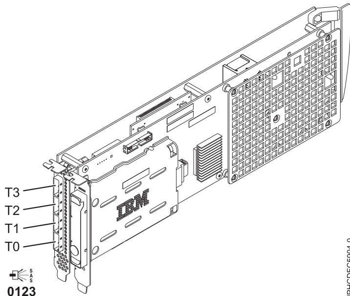
図 60. PCI-X DDR 1.5GB キャッシュ SAS RAID アダプター
