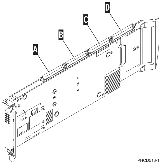
図 69. アダプター SCSI コネクター
