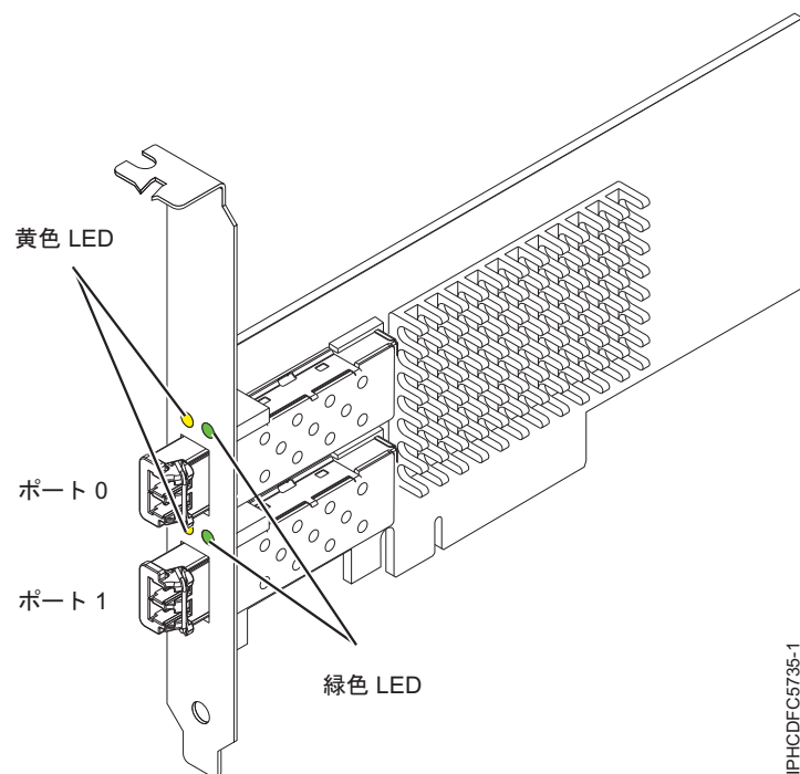
図 9. 5735 アダプター
