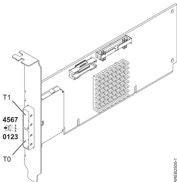
図 56. PCI-X DDR External Dual -x4 ポート SAS アダプター
