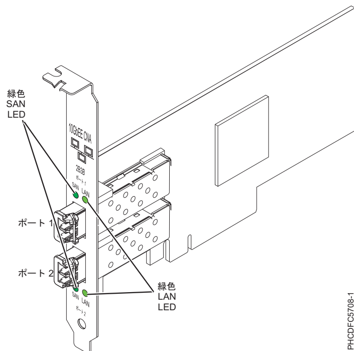
図 26. 10 Gb FCoE PCIe デュアル・ポート・アダプター
