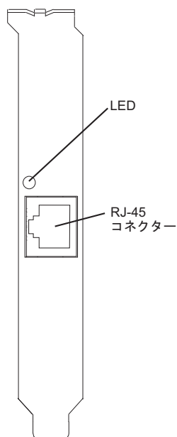
図 30. 1 ギガビット TX iSCSI TOE PCI-X アダプター上の LED
