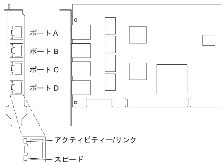
図 33. 4 ポート 10/100/1000 Base-TX PCI-X アダプター
