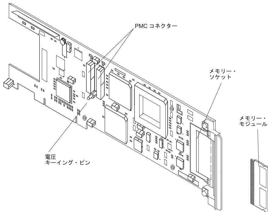
図 76. IBM ARTIC960Hx ベース PCI アダプター
