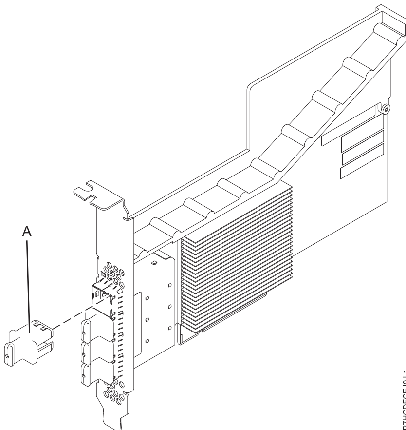
図 17. PCIe3 RAID SAS アダプター
