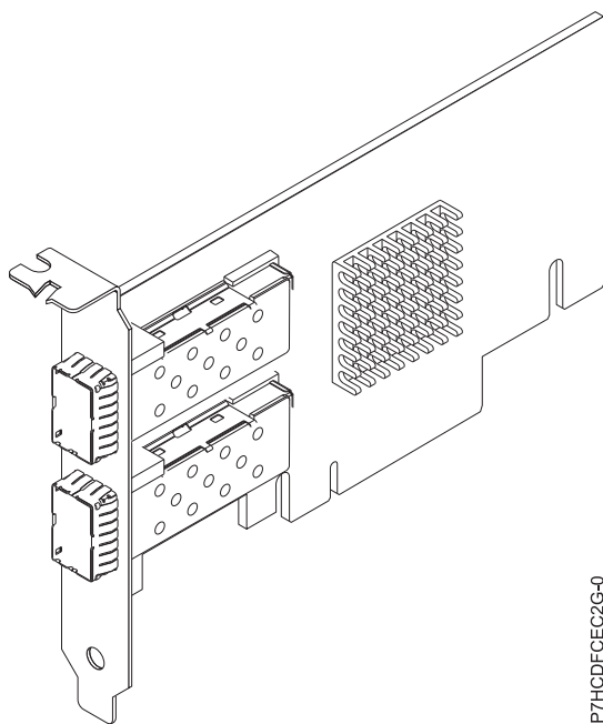
図 44. FC EC2J アダプター
