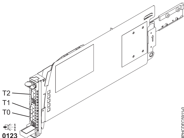
図 63. 内部分割 DASD オプション用 SAS アダプター
