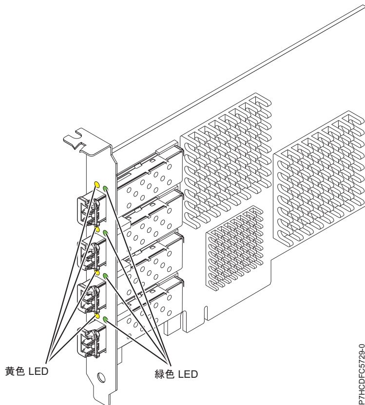
図 8. FC 5729 アダプター
