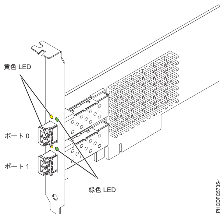
図 21. 5735 アダプター
