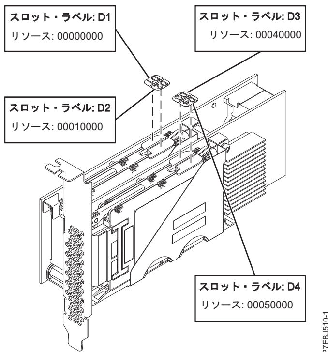
図 49. PCIe デュアル x4 3 Gb SAS RAID アダプター
