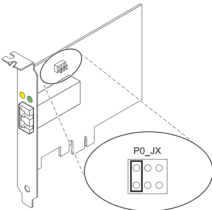
図 23. デバイス ID ジャンパー
