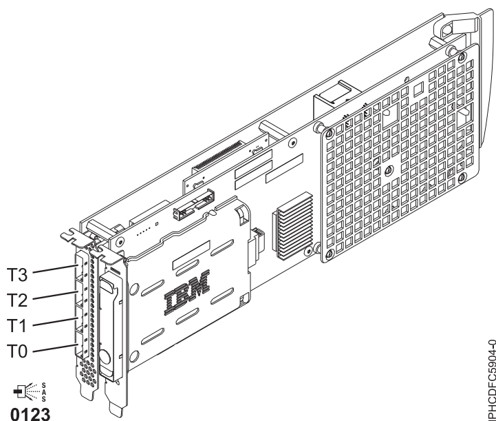
図 16. PCI-X DDR 1.5GB キャッシュ SAS RAID アダプター
