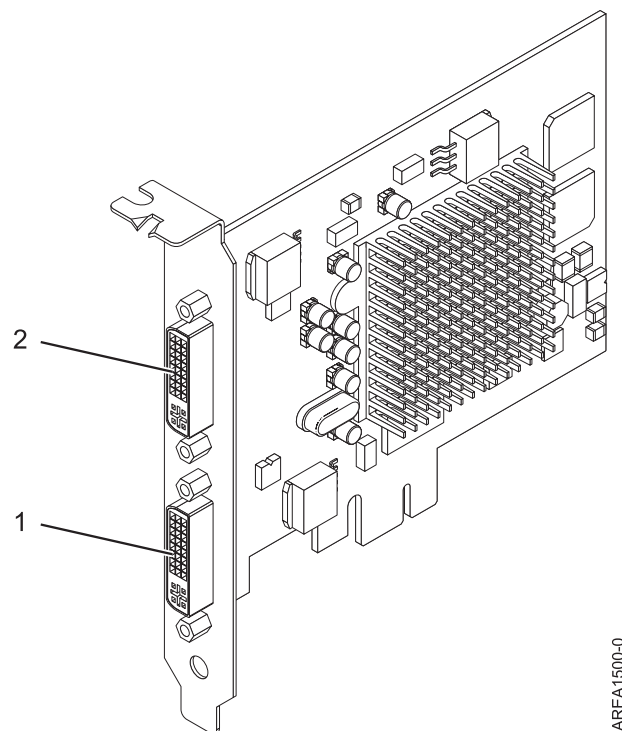
図 27. POWER GXT145 PCI Express グラフィックス・アクセラレーター・アダプター
