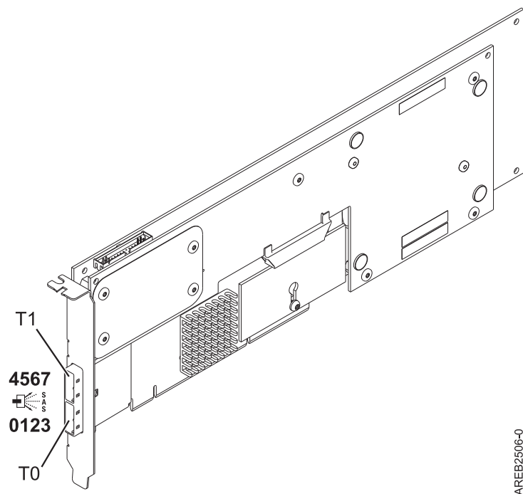
図 14. PCI-X DDR デュアル -x4 ポート SAS RAID アダプター
