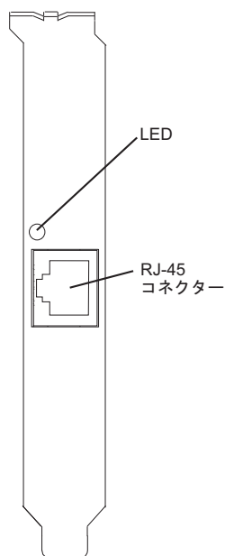
図 34. 1 ギガビット TX iSCSI TOE PCI-X アダプター上の LED
