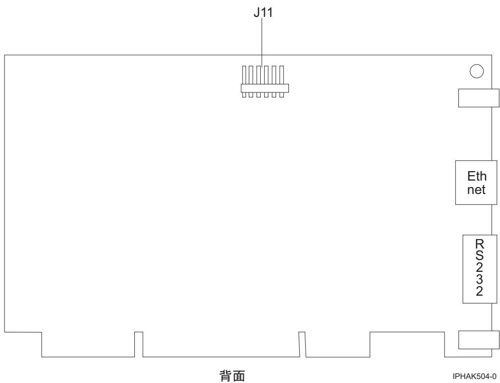
図 48. アダプター背面
