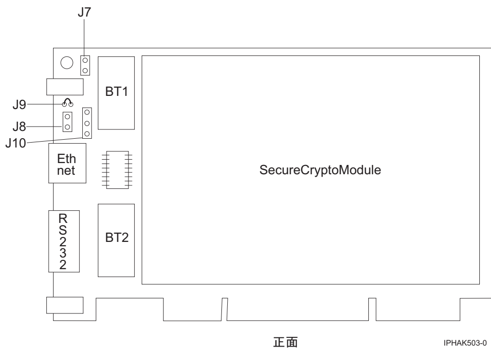
図 47. アダプター正面
