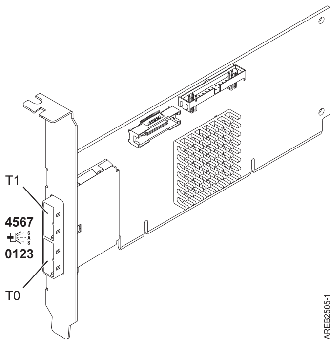
図 18. PCI-X DDR External Dual -x4 ポート SAS アダプター
