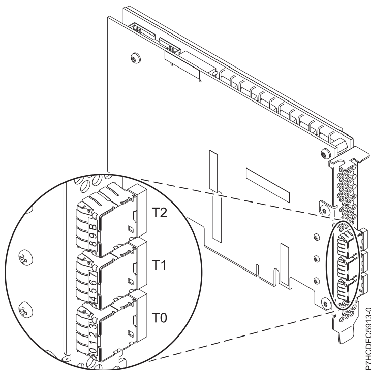
図 19. 5913 アダプター
