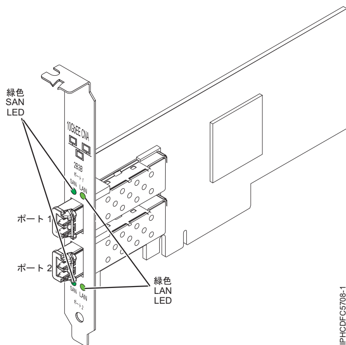
図 30. 10 Gb FCoE PCIe デュアル・ポート・アダプター
