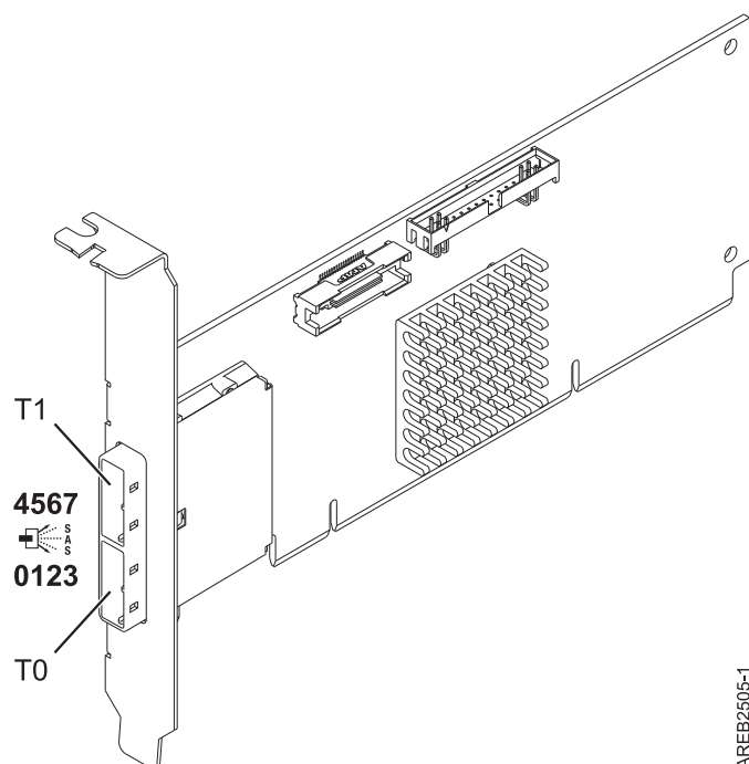
図 12. PCI-X DDR External Dual -x4 ポート SAS アダプター
