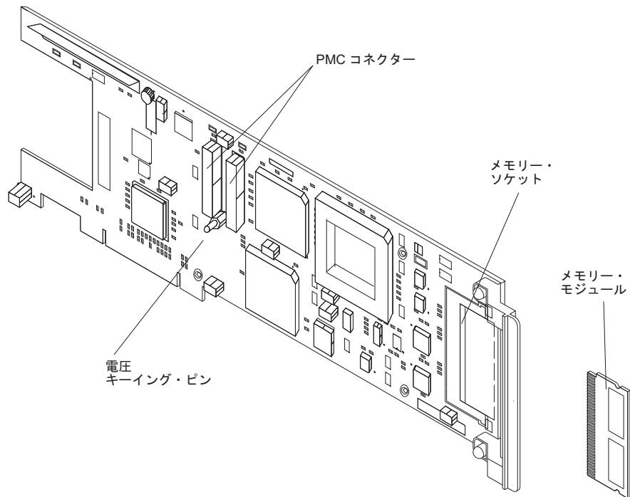
図 44. IBM ARTIC960Hx ベース PCI アダプター
