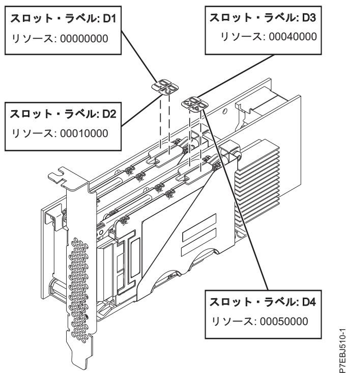
図 50. PCIe デュアル x4 3 Gb SAS RAID アダプター
