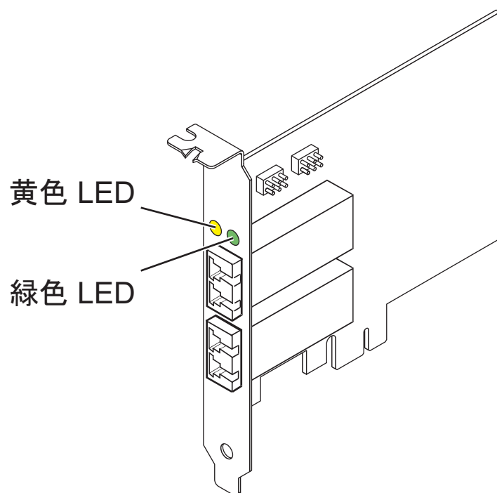
図 24. 5774 アダプター
