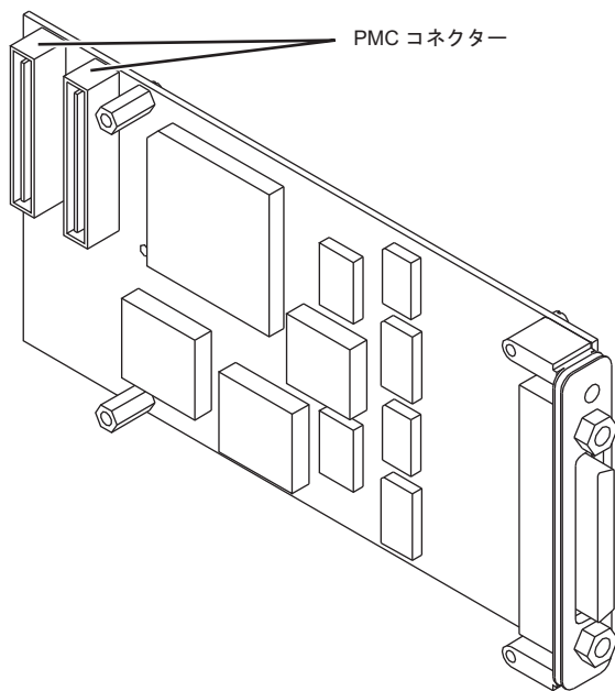
図 45. 4 ポート選択可能 PMC
