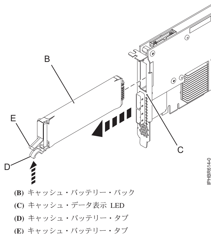
図 55. 574E キャッシュ・バッテリーの取り替え
