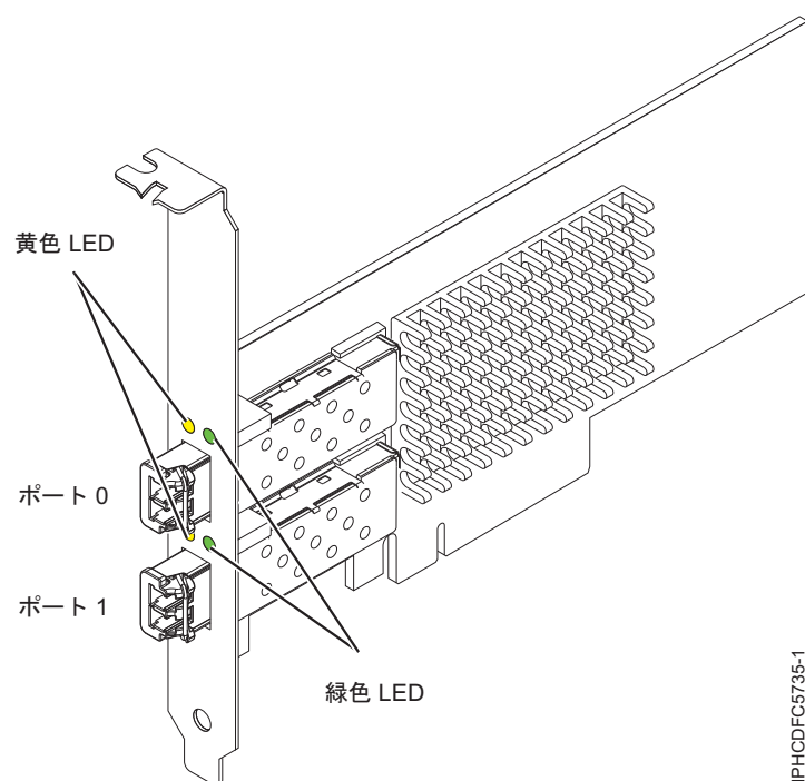
図 20. 5735 アダプター
