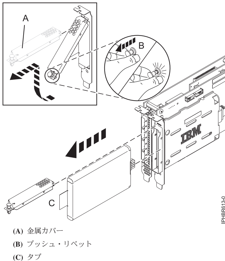
図 52. 572F/575C キャッシュ・バッテリーの取り替え
