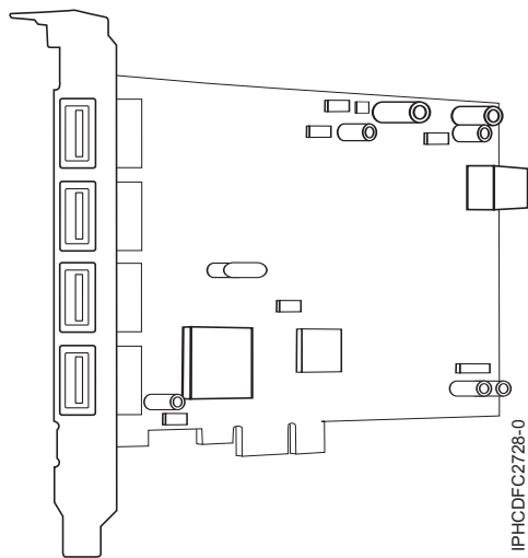
図 46. 4 ポート USB PCIe アダプター
