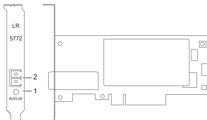
図 42. 10 ギガビット・イーサネット LR PCI Express アダプター
