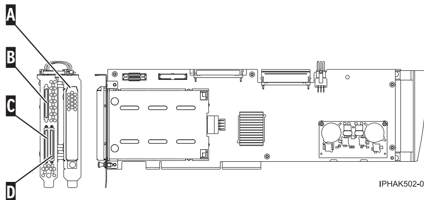
図 8. アダプター
