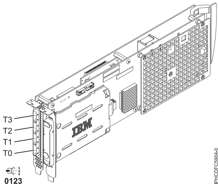
図 17. PCI-X DDR 1.5GB キャッシュ SAS RAID アダプター
