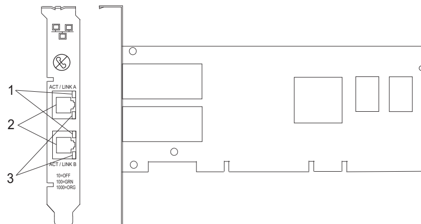
図 29. 2 ポート 10/100/1000 Base-TX イーサネット PCI-X アダプター
