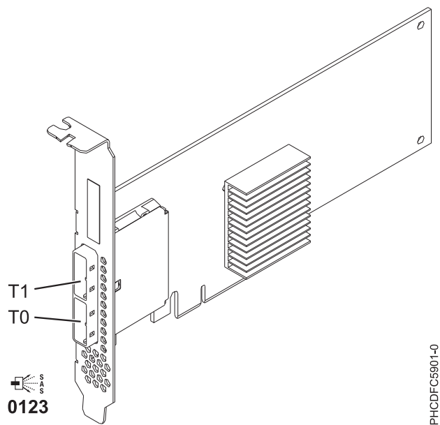
図 13. PCIe デュアル x4 SAS アダプター
