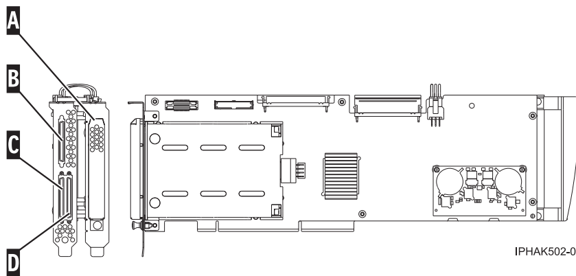
図 10. 5782 アダプター
