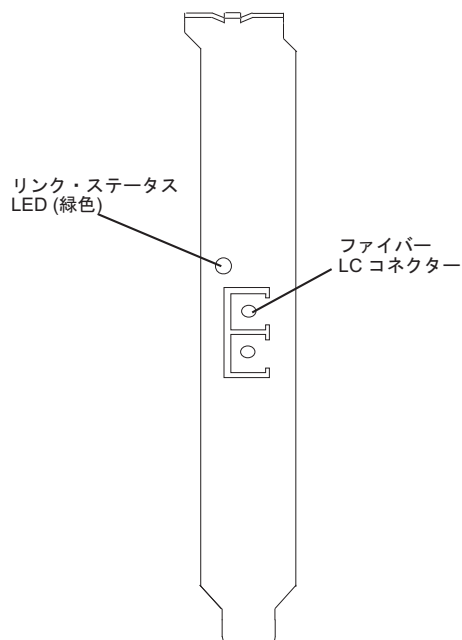
図 33. 1 ギガビット SX iSCSI TOE PCI-X アダプター上の LED
