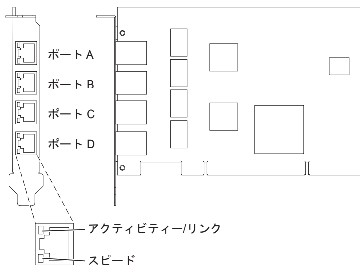
図 38. 4 ポート 10/100/1000 Base-TX PCI-X アダプター
