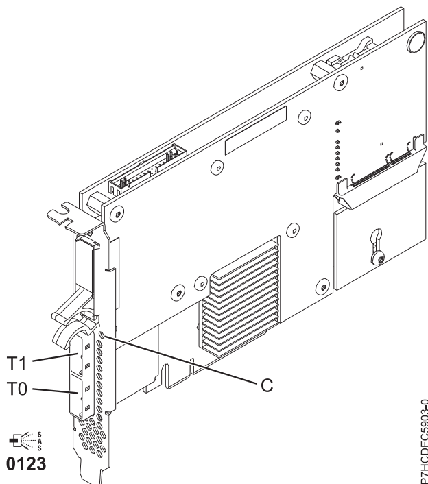
図 15. PCIe デュアル x4 3 Gb SAS RAID アダプター
