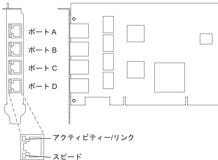
図 37. 4 ポート 10/100/1000 Base-TX PCI-X アダプター
