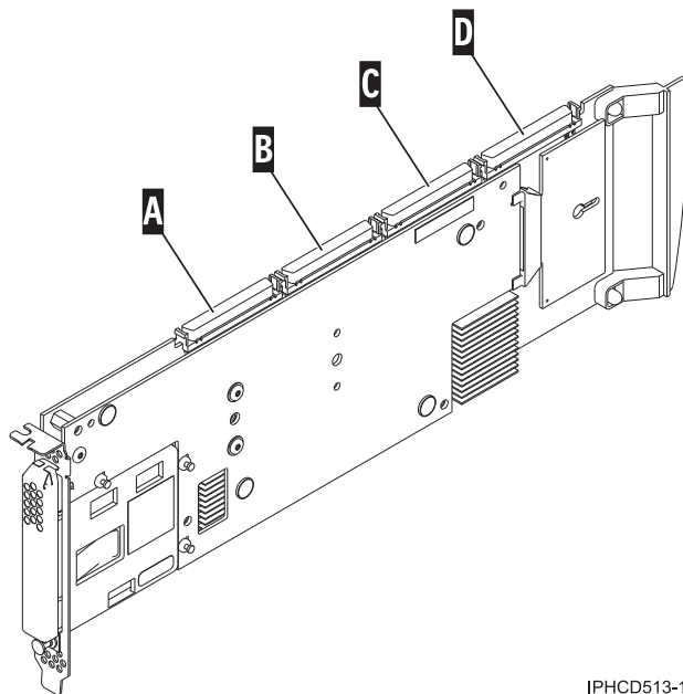
図 98. アダプター SCSI コネクター
