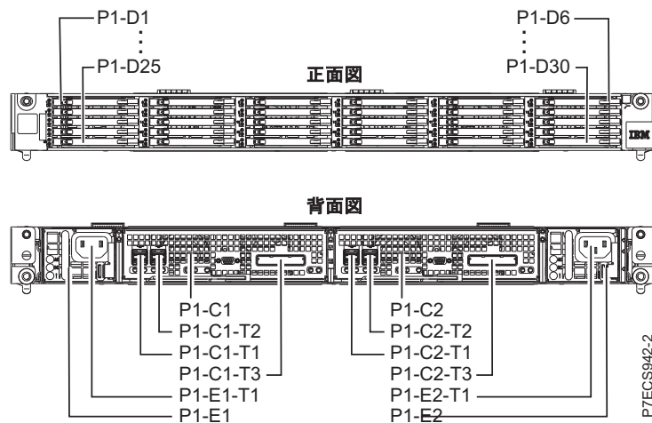
図 105. PCIe2 3.1GB キャッシュ統合 SAS RAID アダプターのロケーション・コード
