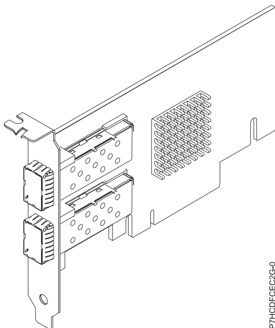
図 65. FC EC2G アダプター
