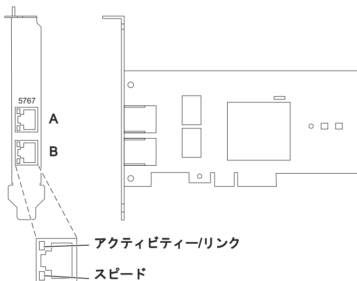
図 39. 2 ポート 10/100/1000 Base-TX イーサネット PCI Express アダプター
