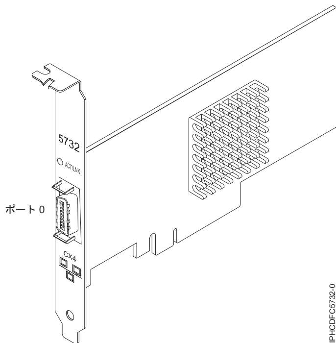
図 52. 10 ギガビット・イーサネット CX4 PCI Express (PCIe) アダプター
