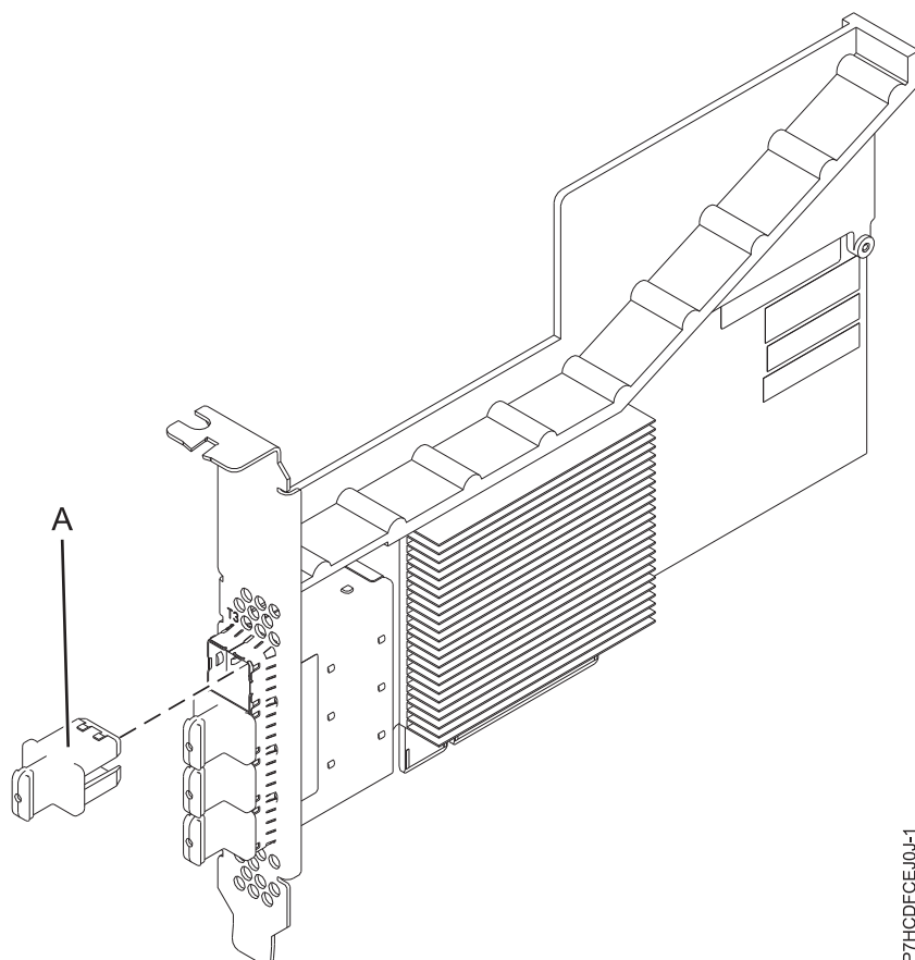
図 25. PCIe3 RAID SAS アダプター
