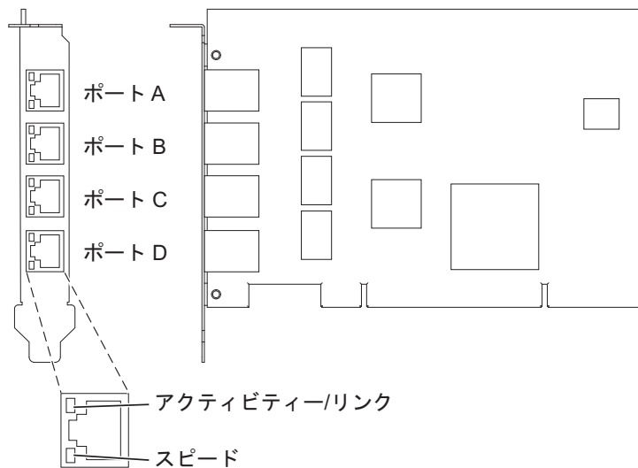
図 54. 4 ポート 10/100/1000 Base-TX PCI-X アダプター
