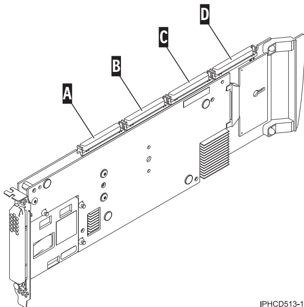
図 95. アダプター SCSI コネクター
