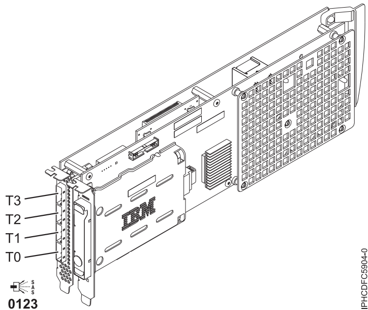
図 89. PCI-X DDR 1.5GB キャッシュ SAS RAID アダプター
