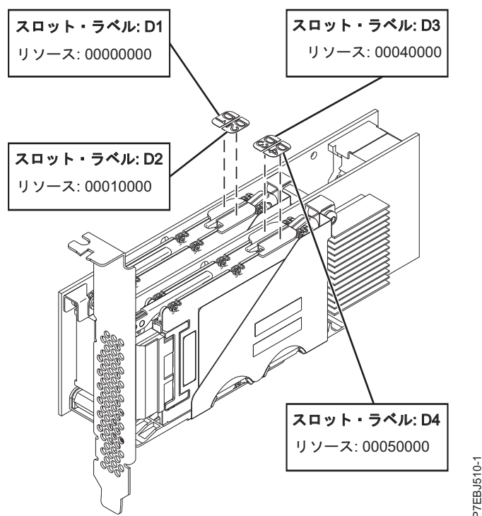
図 82. PCIe デュアル x4 3 Gb SAS RAID アダプター
