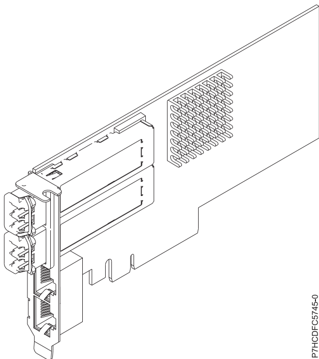
図 56. PCIe2 2x10GbE SFP+ 銅線 2x1GbE UTP アダプター
