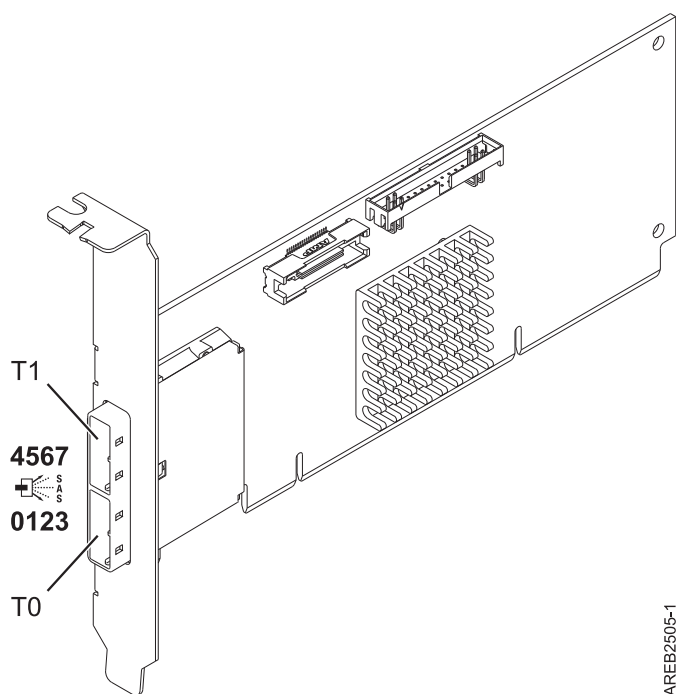
図 90. PCI-X DDR External Dual -x4 ポート SAS アダプター
