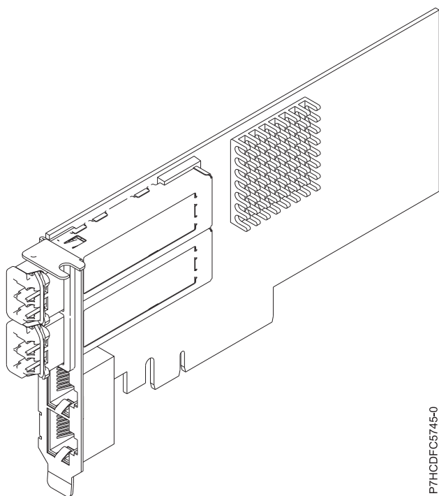
図 36. PCIe2 LP 2x10GbE SFP+ 銅線 2x1GbE UTP アダプター
