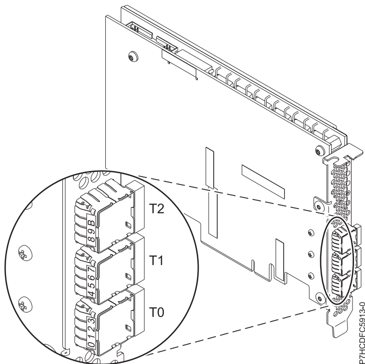
図 92. ESA3 アダプター
