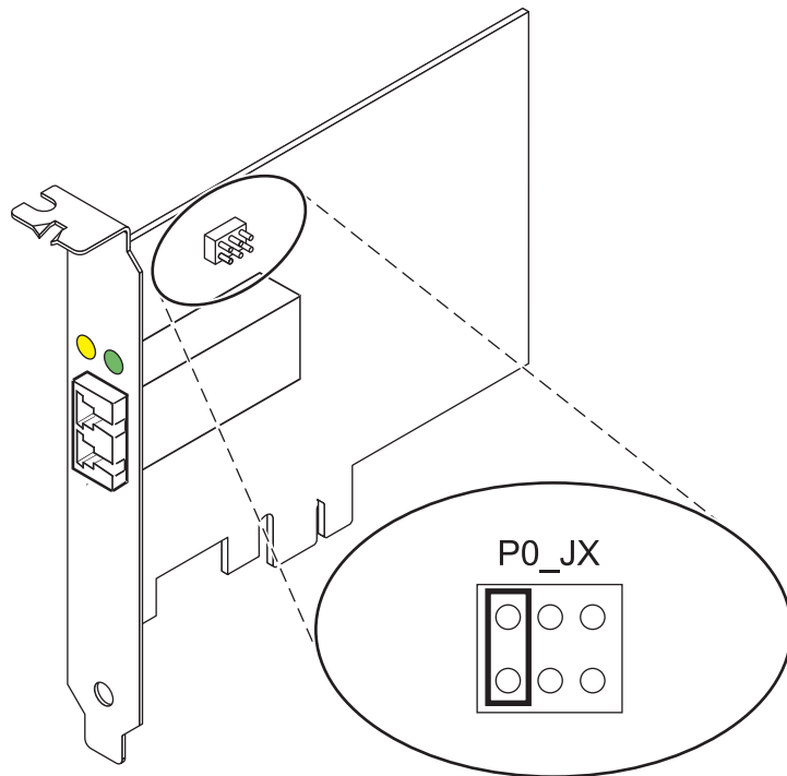
図 16. デバイス ID ジャンパー
