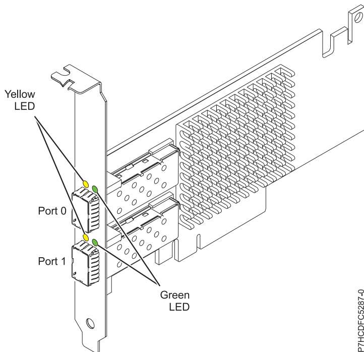
図 42. PCIe 2 ポート 10GbE SR アダプター
