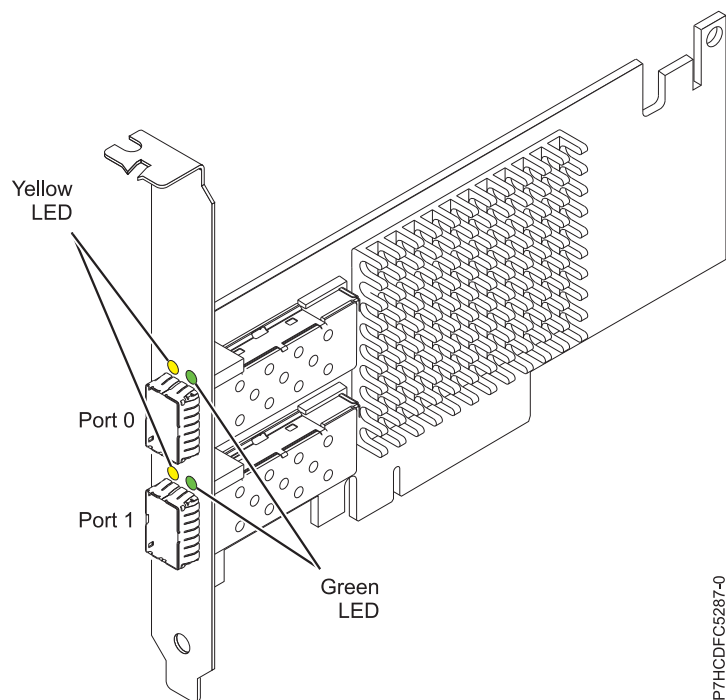
図 40. PCIe2 LP 2 ポート 10GbE SR アダプター
