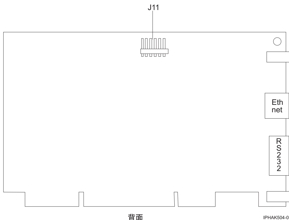
図 79. アダプター背面
