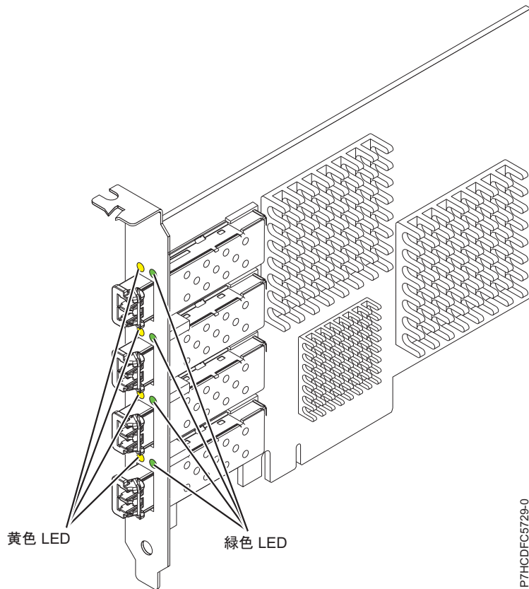
図 13. FC 5729 アダプター
