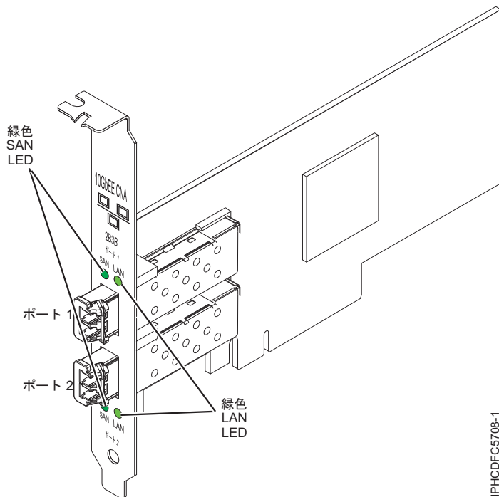
図 31. PCIe LP 10-Gb FCoE 2 ポート・アダプター
