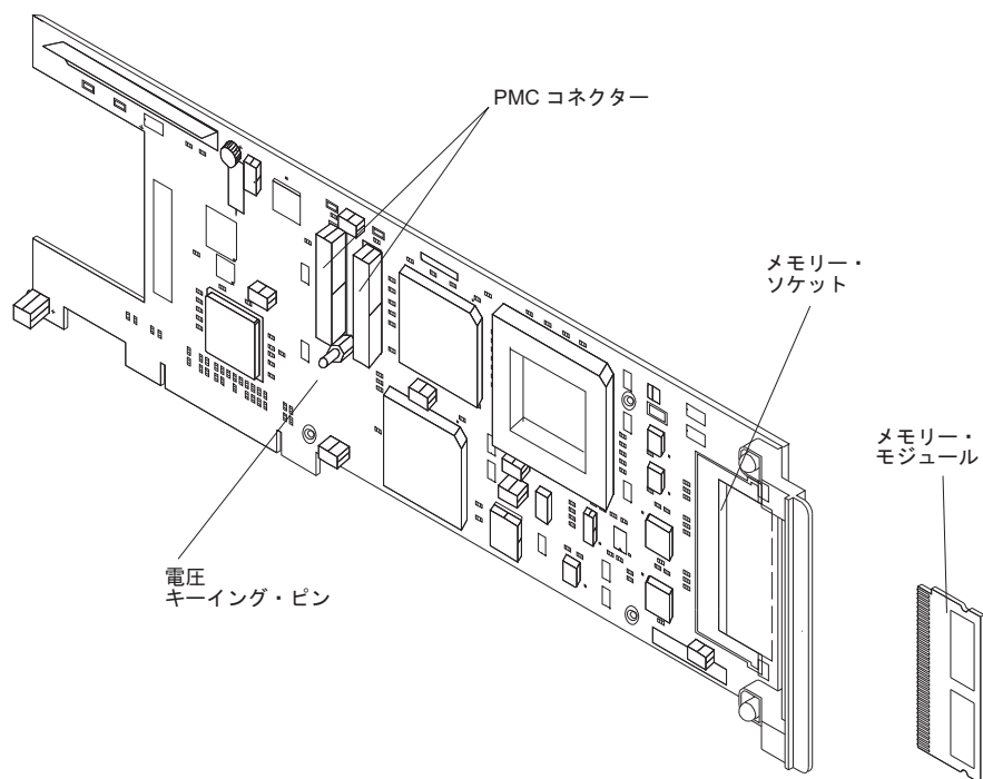
図 103. IBM ARTIC960Hx ベース PCI アダプター
