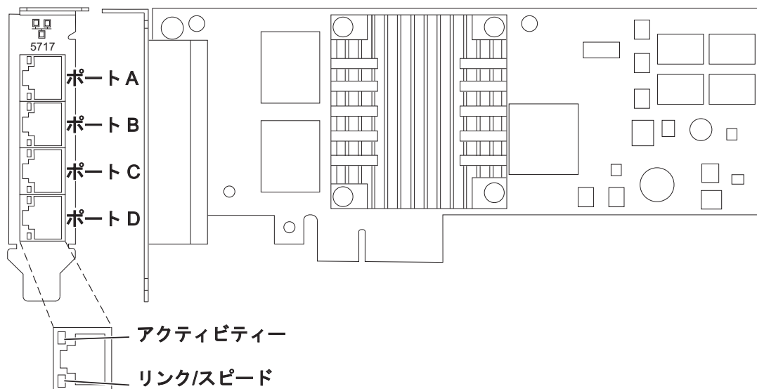
図 32. FC 5271 アダプター
