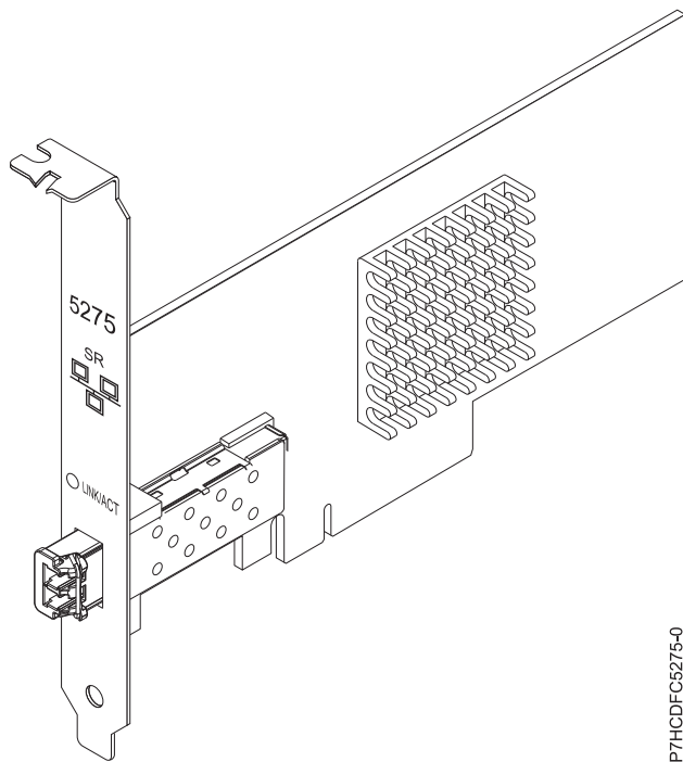
図 35. PCIe LP 10GbE SR 1 ポート・アダプター
