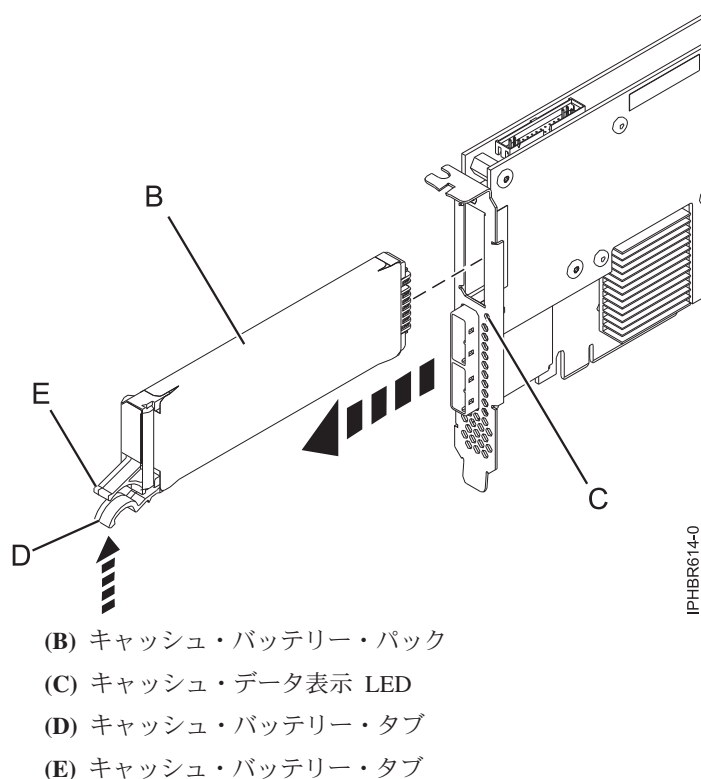
図 112. 574E キャッシュ・バッテリーの取り替え
