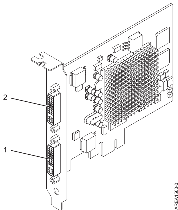
図 24. POWER GXT145 PCI Express グラフィックス・アクセラレーター・アダプター
