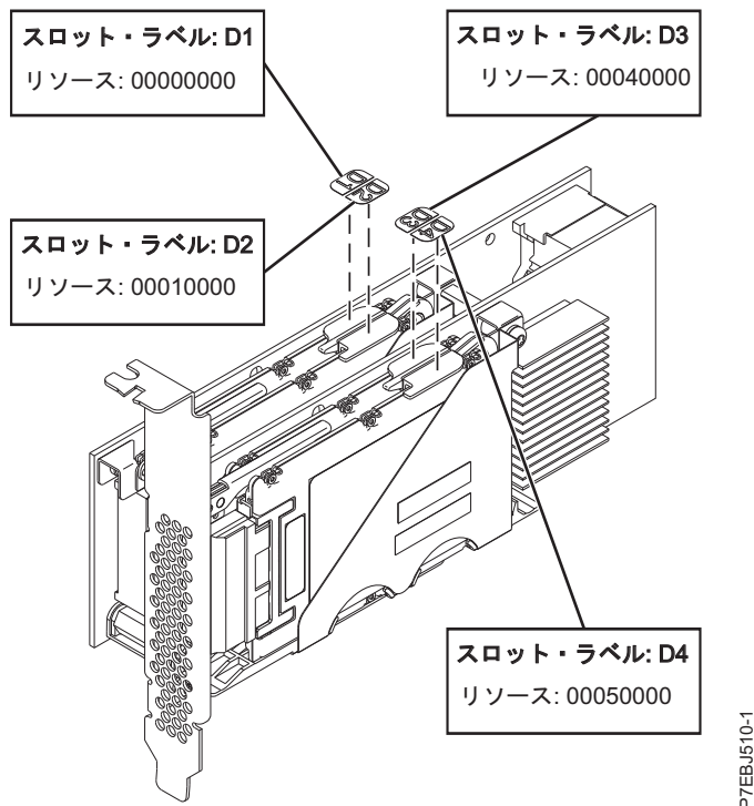
図 81. PCIe デュアル x4 3 Gb SAS RAID アダプター
