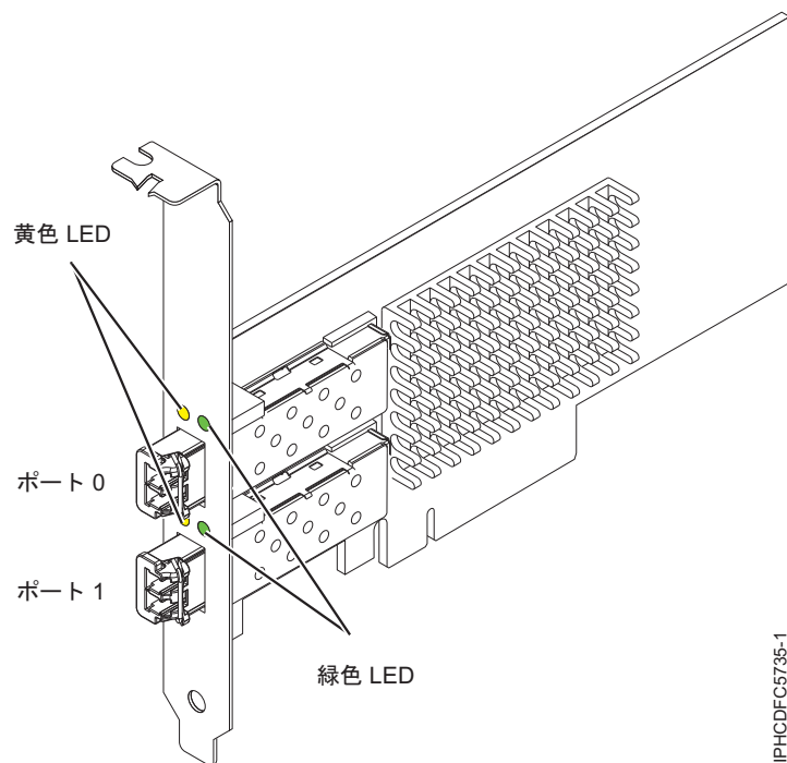
図 20. EN0B アダプター
