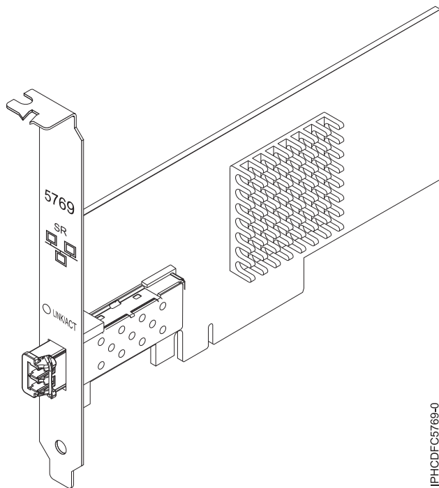
図 60. 10 ギガビット・イーサネット SR PCIe アダプター
