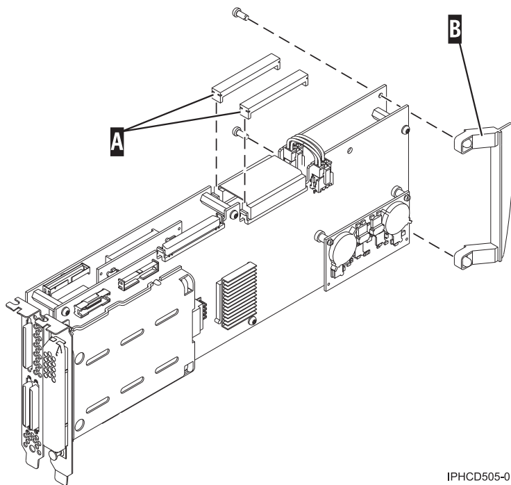
図 100. アダプターをカセットに配置する準備
