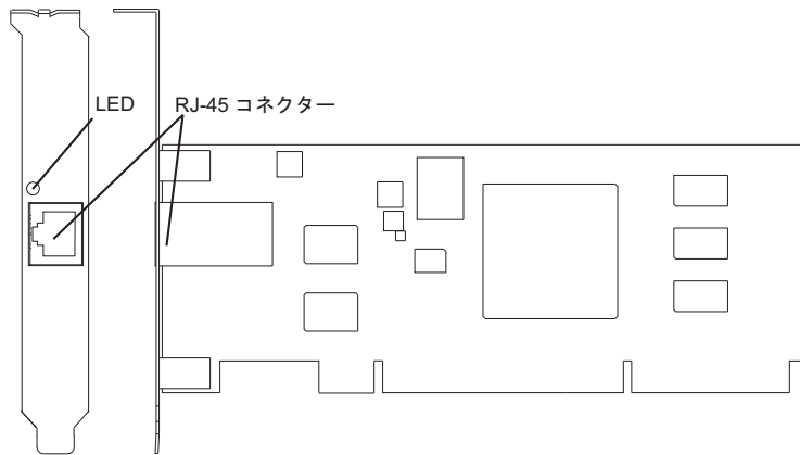
図 48. 1 ギガビット TX iSCSI TOE PCI-X アダプター
