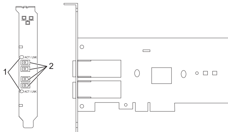
図 34. PCIe LP 2 ポート 1GbE SX アダプター
