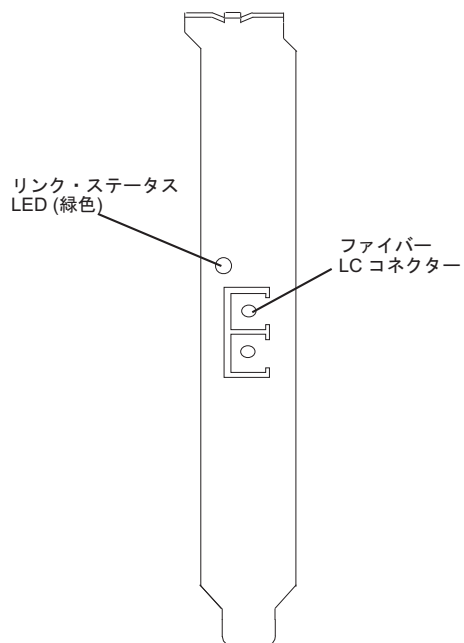
図 49. 1 ギガビット SX iSCSI TOE PCI-X アダプター上の LED
