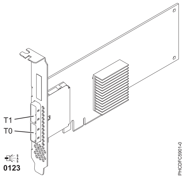
図 83. PCIe デュアル x4 SAS アダプター
