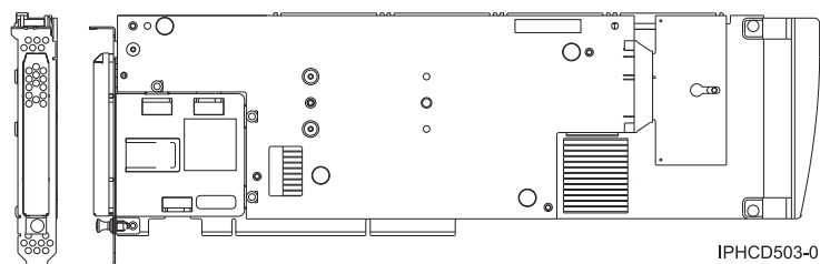
図 97. アダプター側面図と端面図
