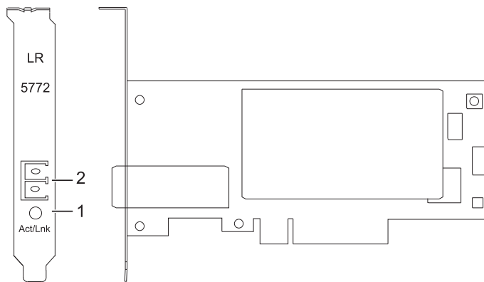
図 61. 10 ギガビット・イーサネット LR PCI Express アダプター
