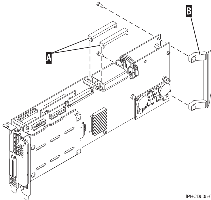
図 102. アダプターをカセットに配置する準備
