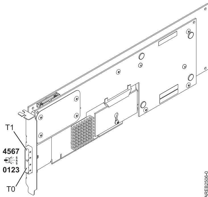
図 86. PCI-X DDR デュアル -x4 ポート SAS RAID アダプター
