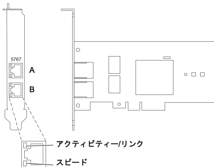
図 58. 2 ポート 10/100/1000 Base-TX イーサネット PCI Express アダプター
