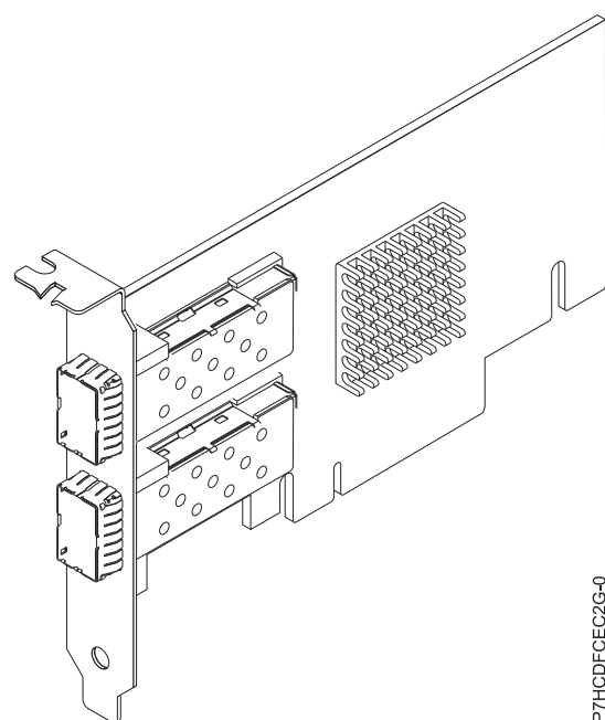
図 69. FC EC2J アダプター
