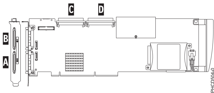
図 96. PCI-X DDR デュアル・チャネル Ultra320 SCSI RAID アダプター
