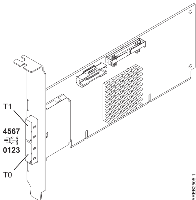
図 84. PCI-X DDR External Dual -x4 ポート SAS アダプター
