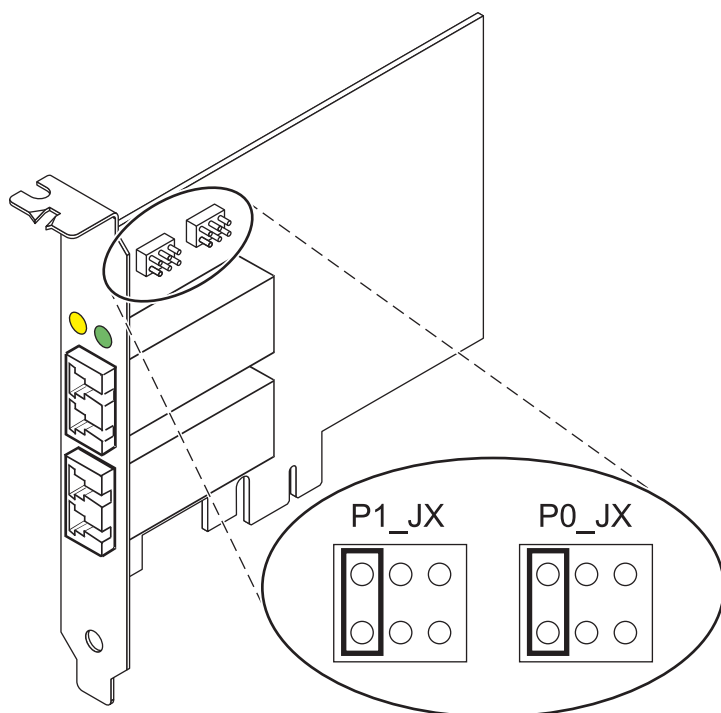
図 18. デバイス ID ジャンパー
