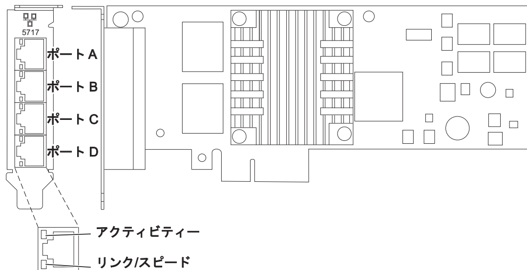
図 51. 4 ポート 10/100/1000 Base-TX PCIe アダプター
