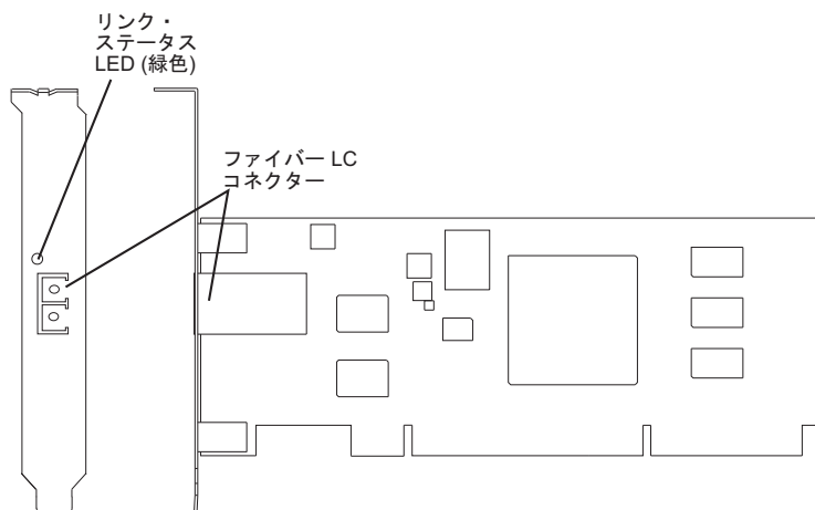
図 47. 1 ギガビット SX iSCSI TOE PCI-X アダプター
