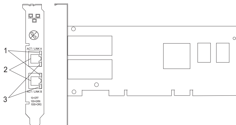
図 45. 2 ポート 10/100/1000 Base-TX イーサネット PCI-X アダプター
