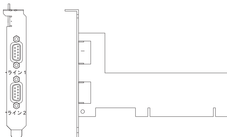
図 7. 2 ポート非同期 EIA-232 PCI アダプター
