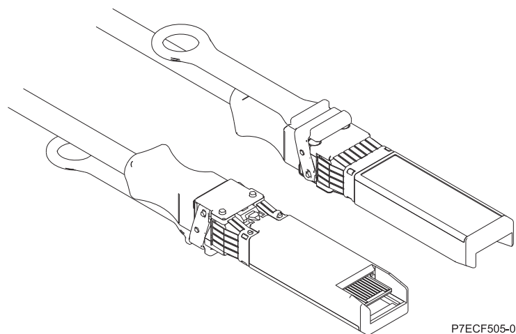
図 64. ケーブルの上面および下面の図
