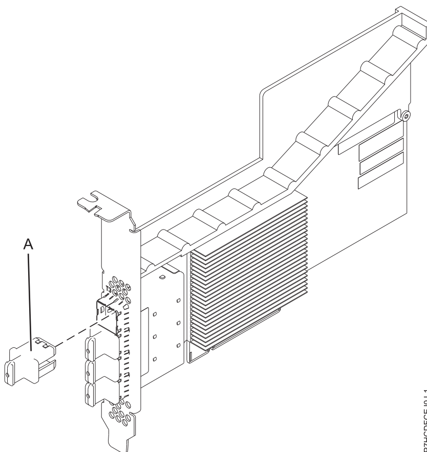
図 28. PCIe3 4 x8 SAS ポート・アダプター
