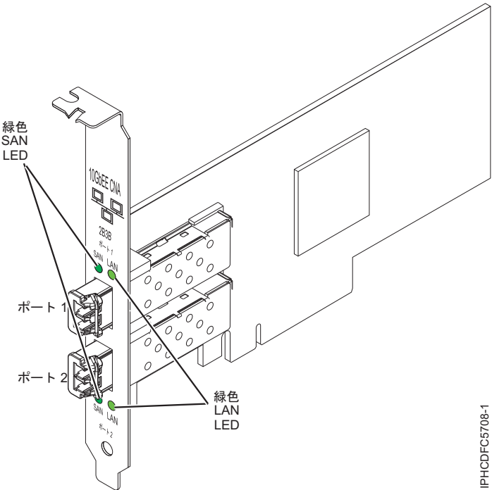
図 46. 10 Gb FCoE PCIe デュアル・ポート・アダプター
