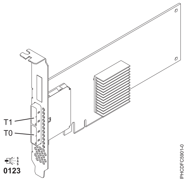
図 85. PCIe デュアル x4 SAS アダプター
