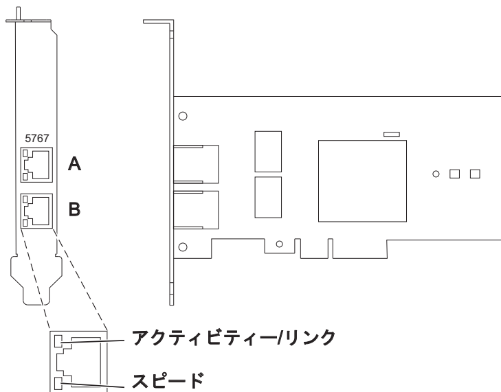
図 63. PCIe 2 ポート 1GbE TX アダプター
