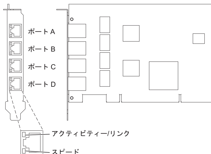
図 53. 4 ポート 10/100/1000 Base-TX PCI-X アダプター
