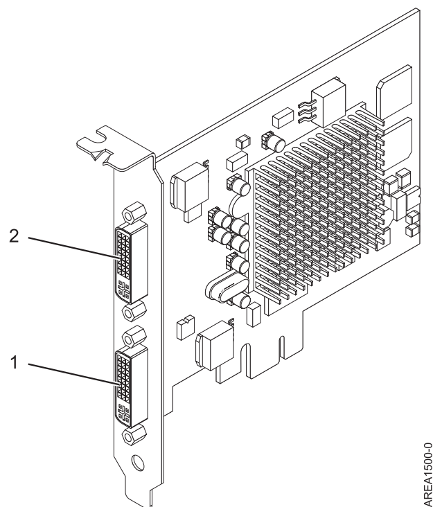
図 23. PCIe LP POWER GXT145 グラフィックス・アクセラレーター・アダプター
