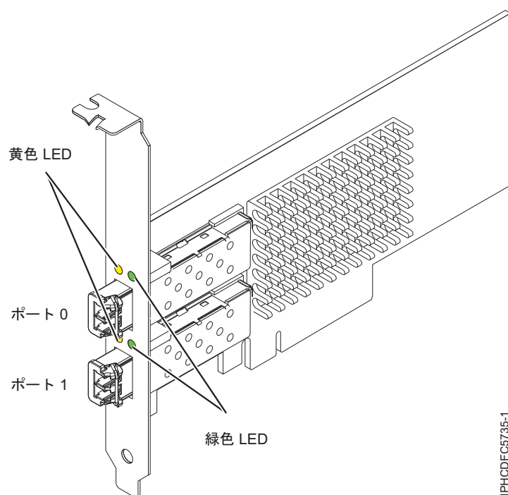
図 19. EN0A アダプター
