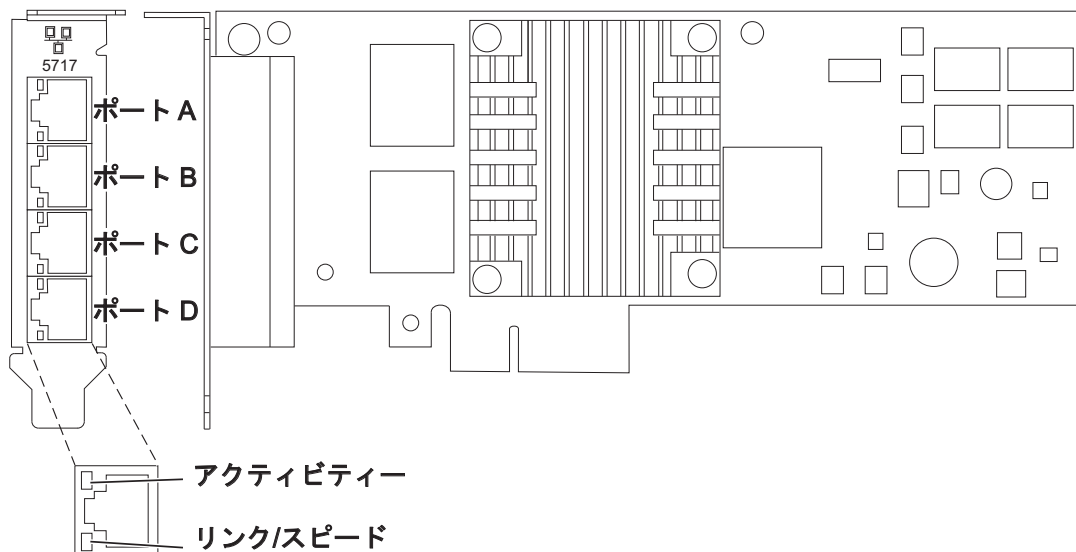
図 25. FC 5271 アダプター
