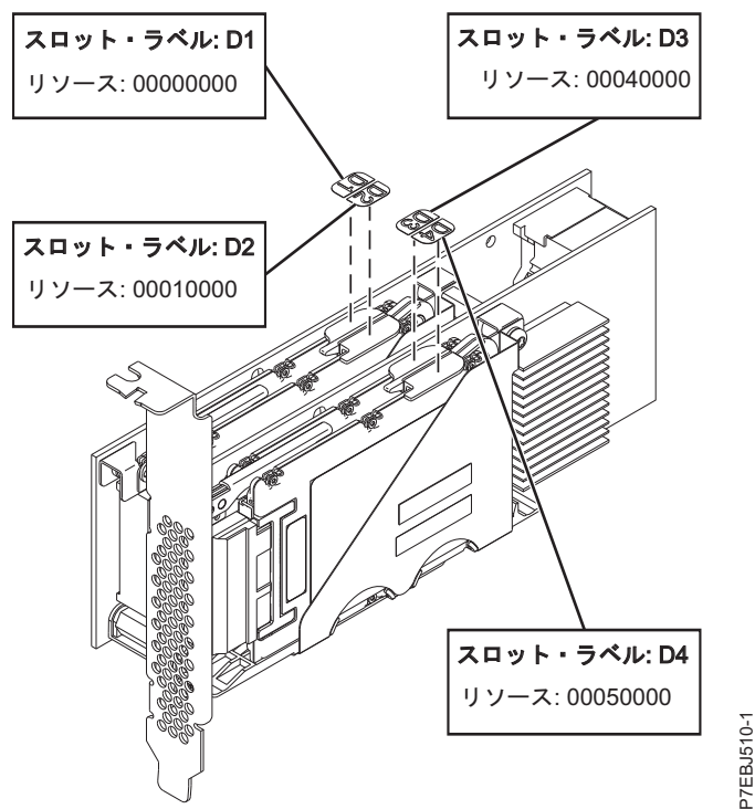
図 52. PCIe デュアル x4 3 Gb SAS RAID アダプター
