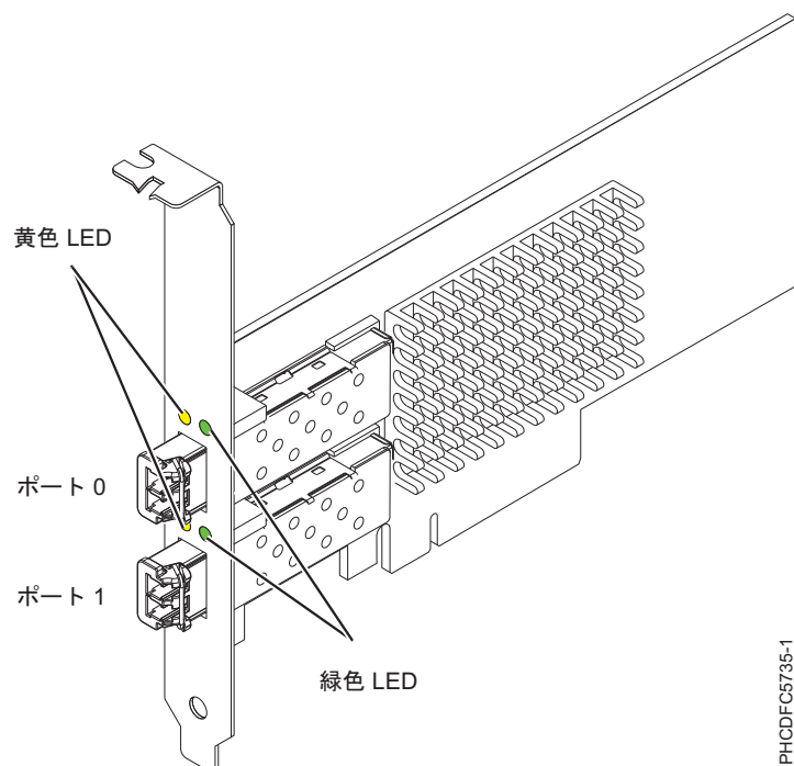
図 6. 5273 アダプター
