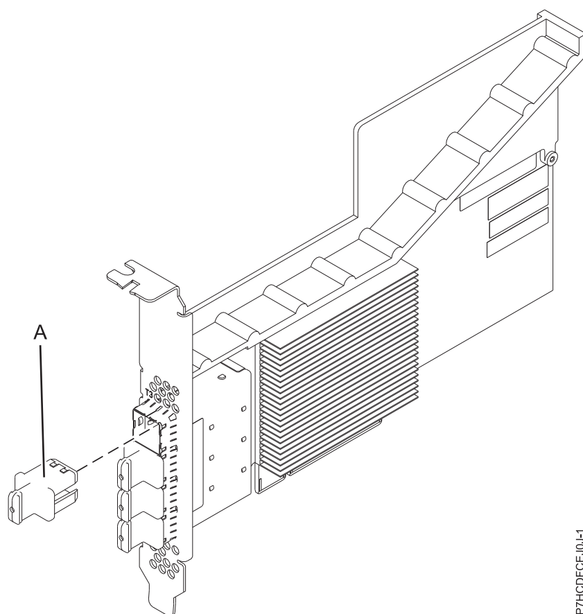
図 21. PCIe 4 x8 SAS ポート・アダプター
