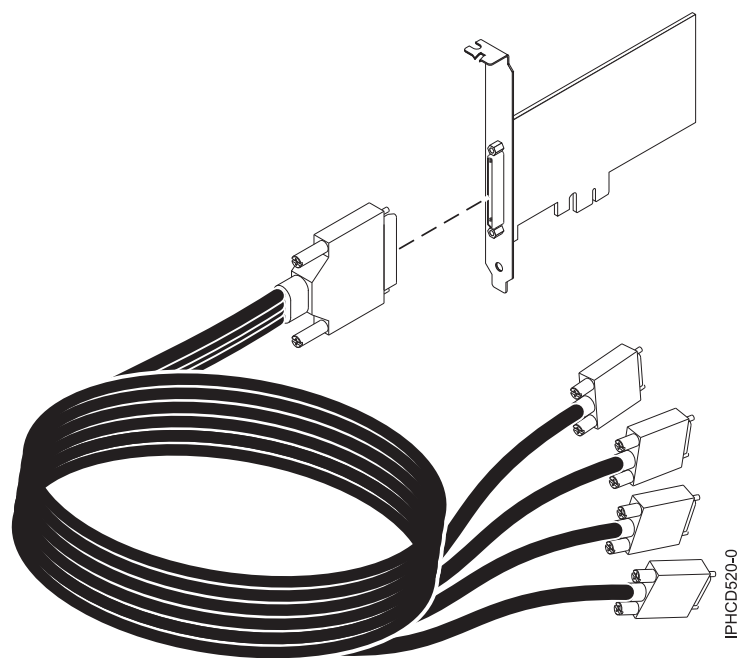
図 5. ケーブル
