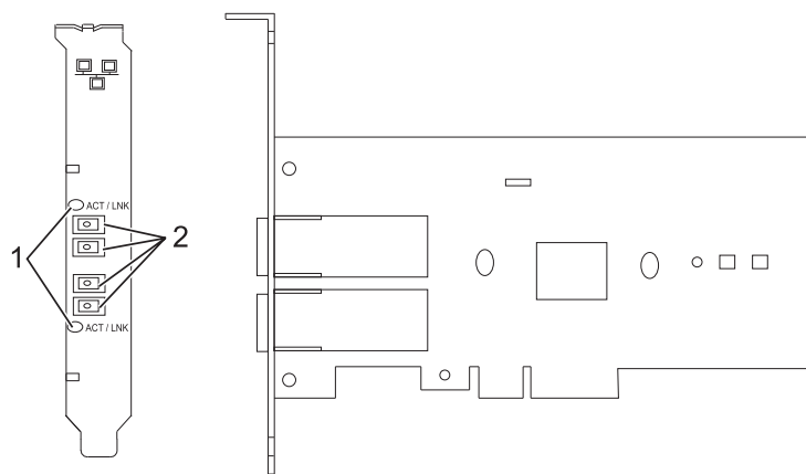
図 39. 2 ポート・ギガビット・イーサネット SX PCI Express アダプター
