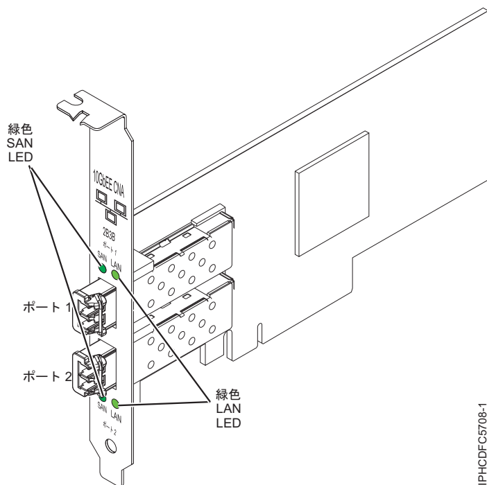
図 35. 10 Gb FCoE PCIe デュアル・ポート・アダプター
