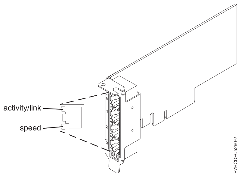
図 23. アダプター
