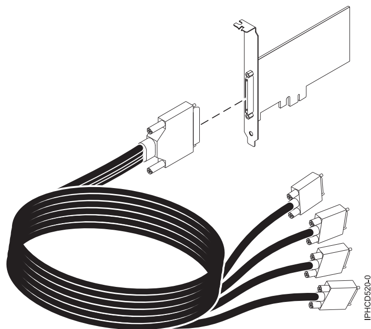
図 3. ケーブル
