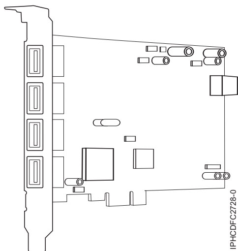
図 51. 4 ポート USB PCIe アダプター
