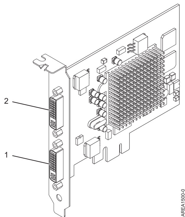
図 17. POWER GXT145 PCI Express グラフィックス・アクセラレーター・アダプター
