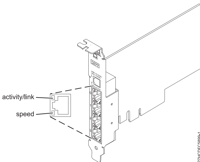
図 42. アダプター
