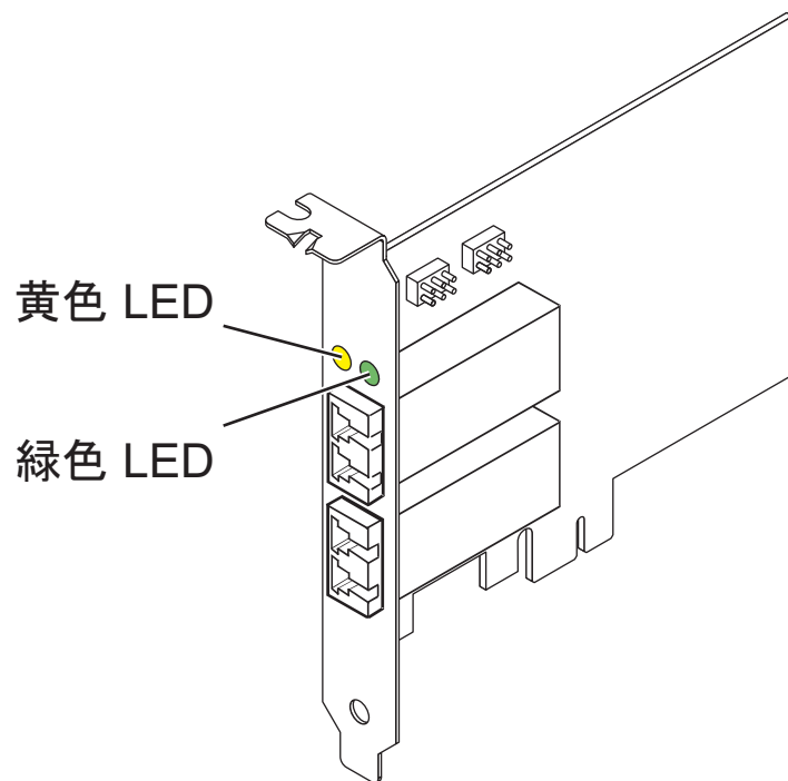
図 13. 5774 アダプター
