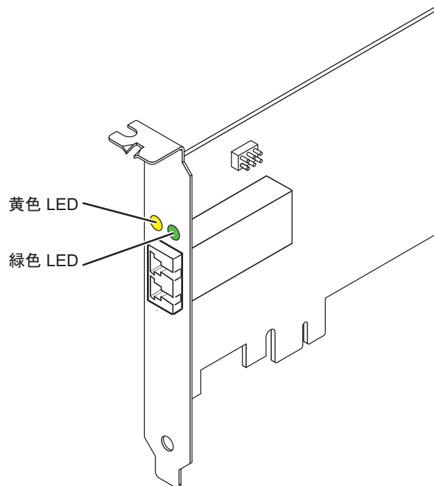
図 11. 5773 アダプター
