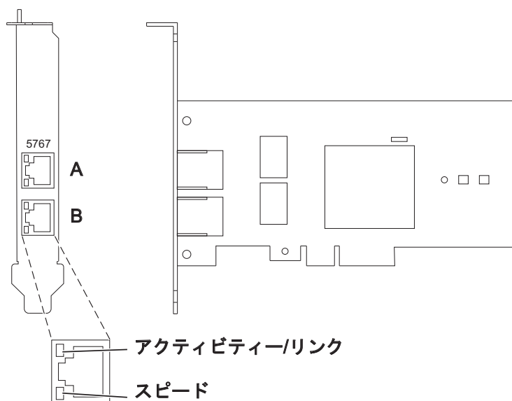
図 38. 2 ポート 10/100/1000 Base-TX イーサネット PCI Express アダプター
