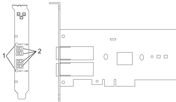
図 27. PCIe LP 2 ポート 1GbE SX アダプター
