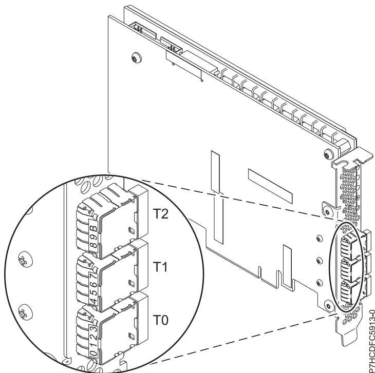
図 56. 5913 アダプター
