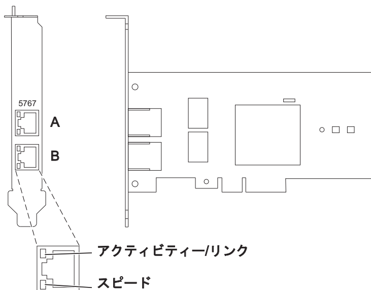
図 32. 2 ポート 10/100/1000 Base-TX イーサネット PCI Express アダプター
