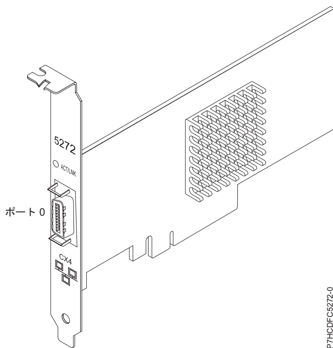
図 26. PCIe LP 10GbE CX4 1 ポート・アダプター
