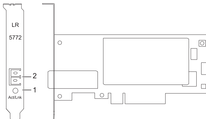
図 41. 10 ギガビット・イーサネット LR PCI Express アダプター
