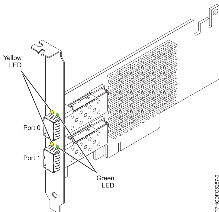
図 33. PCIe2 LP 2 ポート 10GbE SR アダプター
