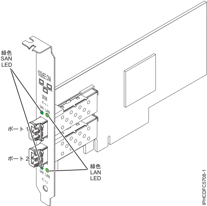
図 24. PCIe LP 10-Gb FCoE 2 ポート・アダプター
