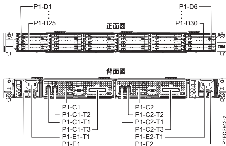
図 57. PCIe2 3.1GB キャッシュ統合 SAS RAID アダプターのロケーション・コード
