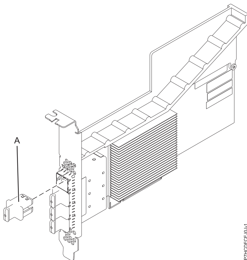
図 18. PCIe3 RAID SAS アダプター
