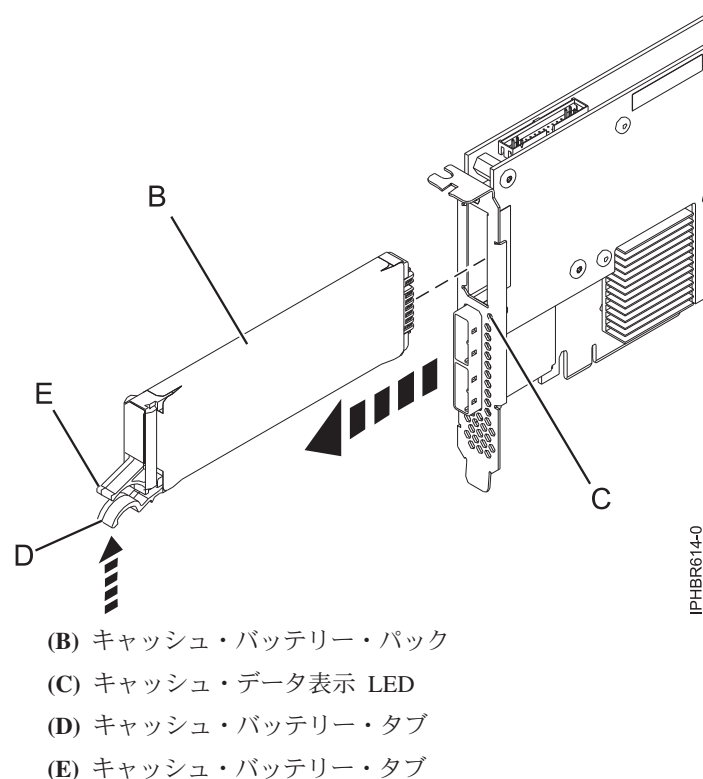
図 64. 574E キャッシュ・バッテリーの取り替え
