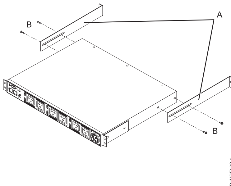
図 43. 長いマウント・ブラケットの取り付け
