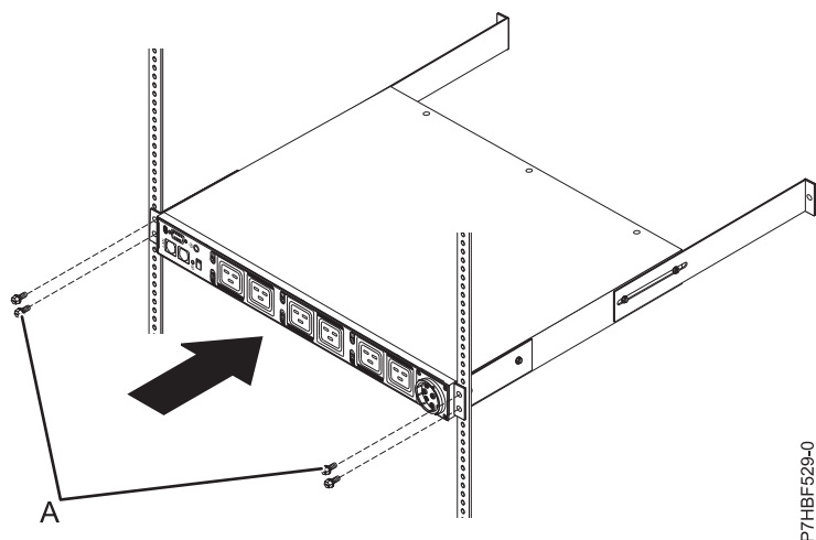
図 44. PDU+ の前部のラックへの取り付け
