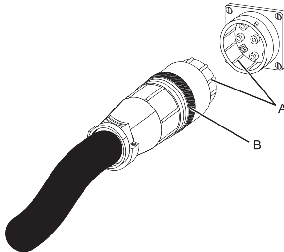
図 46. 電源コードのコネクタと PDU モデルとの位置合わせ
