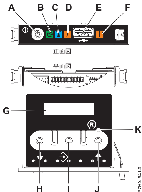
図 19. コントロール・パネル
