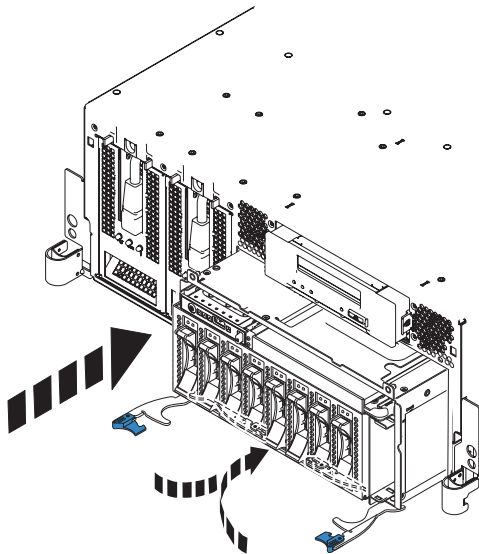
図 12. 装着されたディスク・ドライブ・バックプレーンのラック・マウント型モデルへの取り付け
