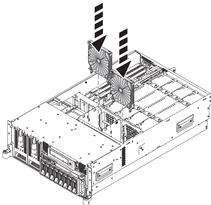
図 16. ファン・ケージへのエア・バッフルの取り付け
