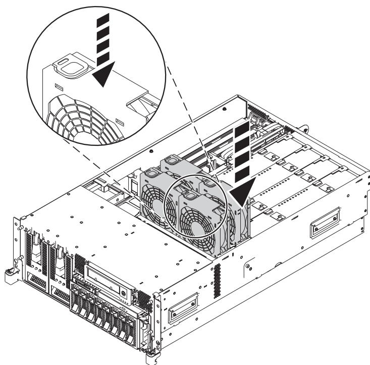
図 17. ファン・ケージへのファンの取り付け
