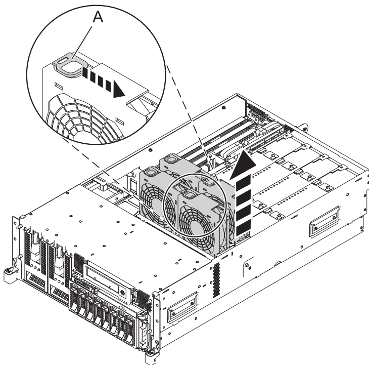
図 2. ファン・ケージからのファンの取り外し
