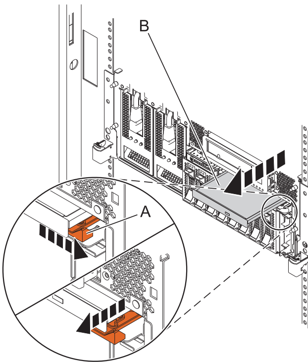
図7. ディスク・ドライブ・バックプレーンからのメディア・デバイスの取り外し
