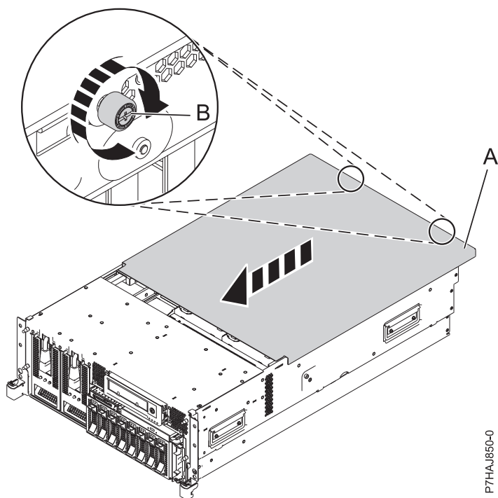
図 23. 保守アクセス・カバーの取り付け
