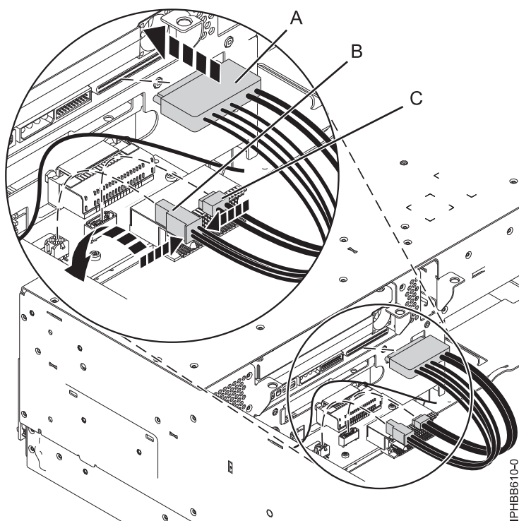
図 13. ディスク・ドライブ・バックプレーンへのケーブルの接続
