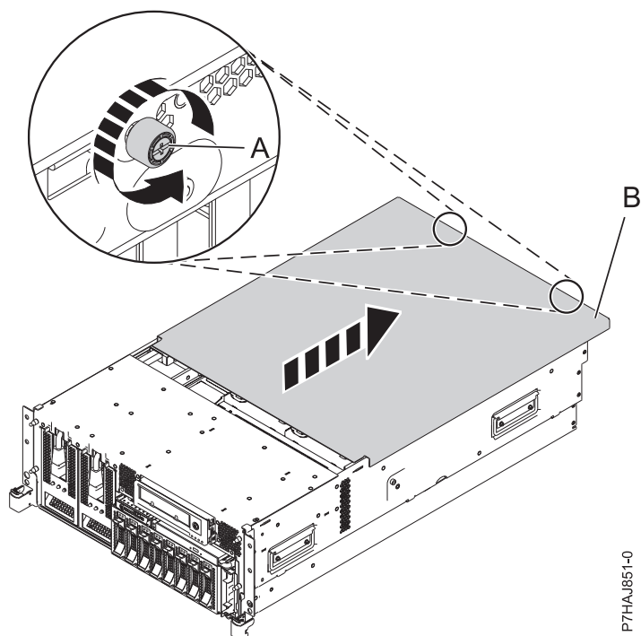
図 22. 保守アクセス・カバーの取り外し
