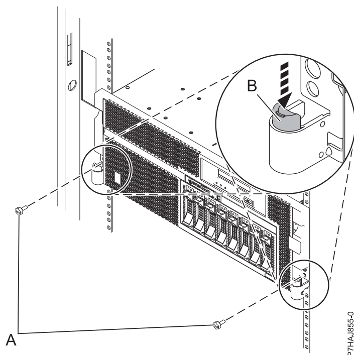
図 24. ラック・ラッチの解除
