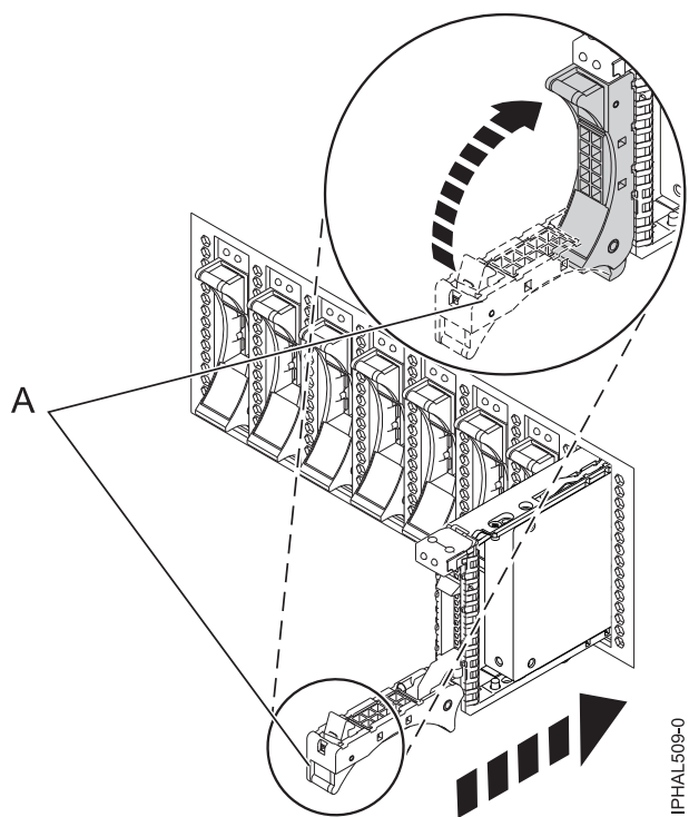
図 14. バックプレーン・ディスク・ドライブの取り付け
