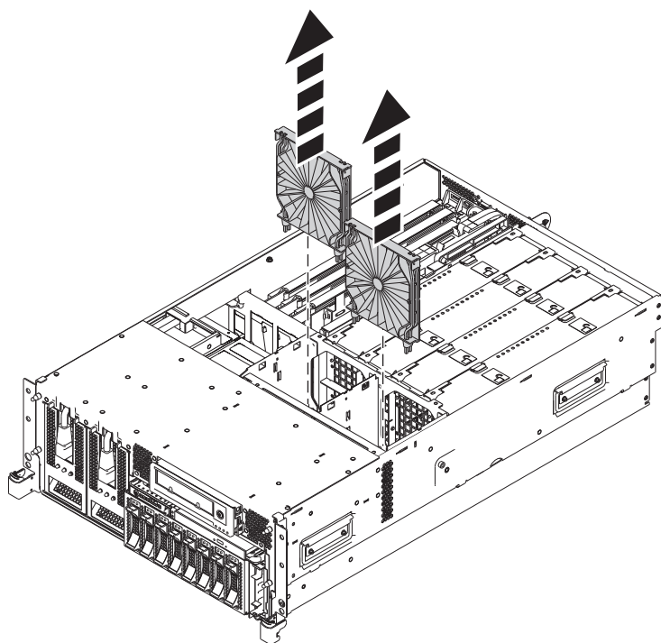
図3. ファン・ケージからのエア・バッフルの取り外し
