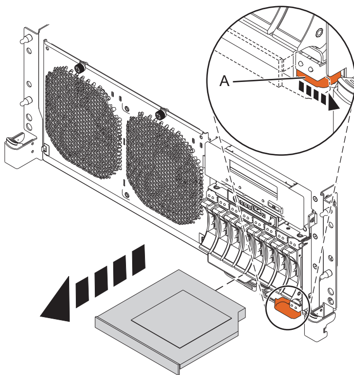
図4. ディスク・ドライブ・バックプレーンからのメディア・デバイスの取り外し
