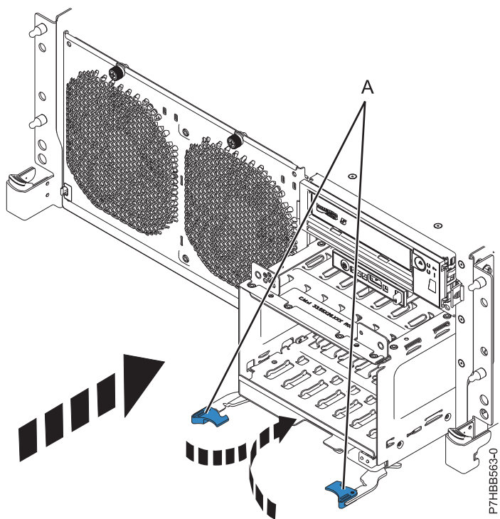
図7. ラック・マウント型モデルへのディスク・ドライブが装着されていないバックプレーンの取り付け
