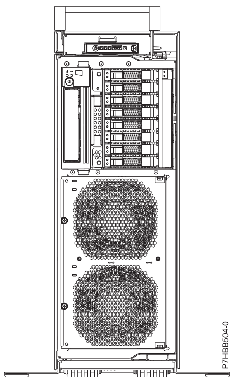
図2. スタンドアロン型システムのディスク・ドライブ・バックプレーン
