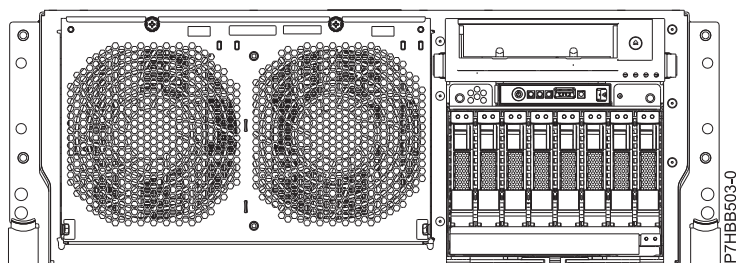
図1. ラック・マウント型システムのディスク・ドライブ・バックプレーン
