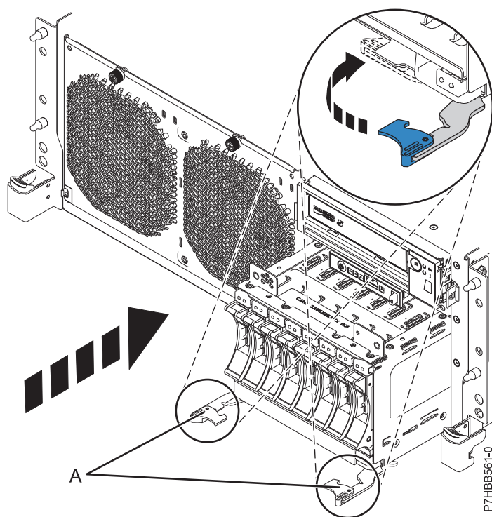
図8. ラック・マウント型モデルへのディスク・ドライブが装着されているバックプレーンの取り付け
