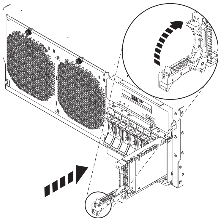
図9. バックプレーン・ディスク・ドライブの取り付け
