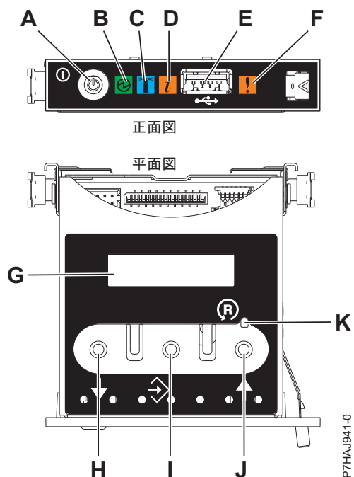
図 12. コントロール・パネル
