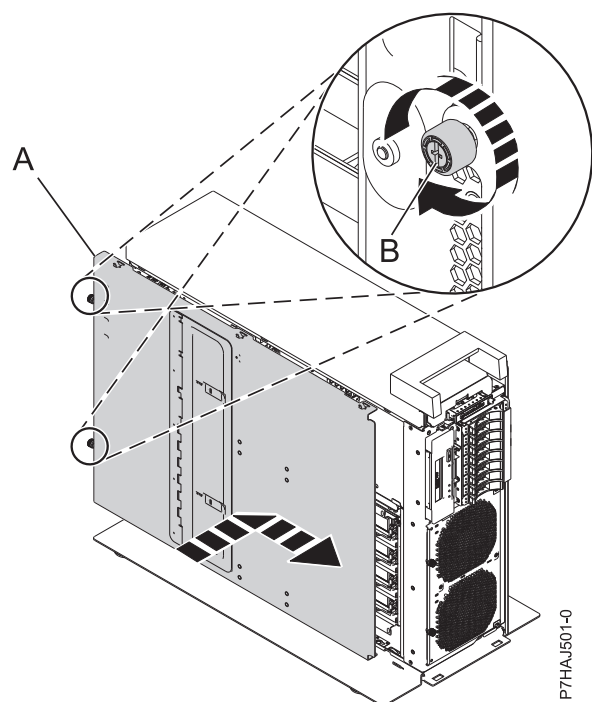
図 22. 内側の保守アクセス・カバーの取り付け
