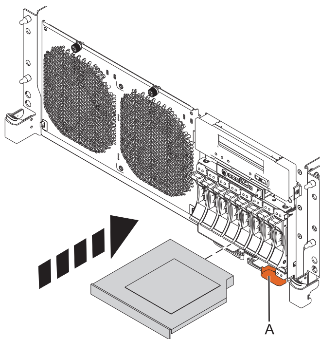
図 10. メディア・デバイスの取り付け
