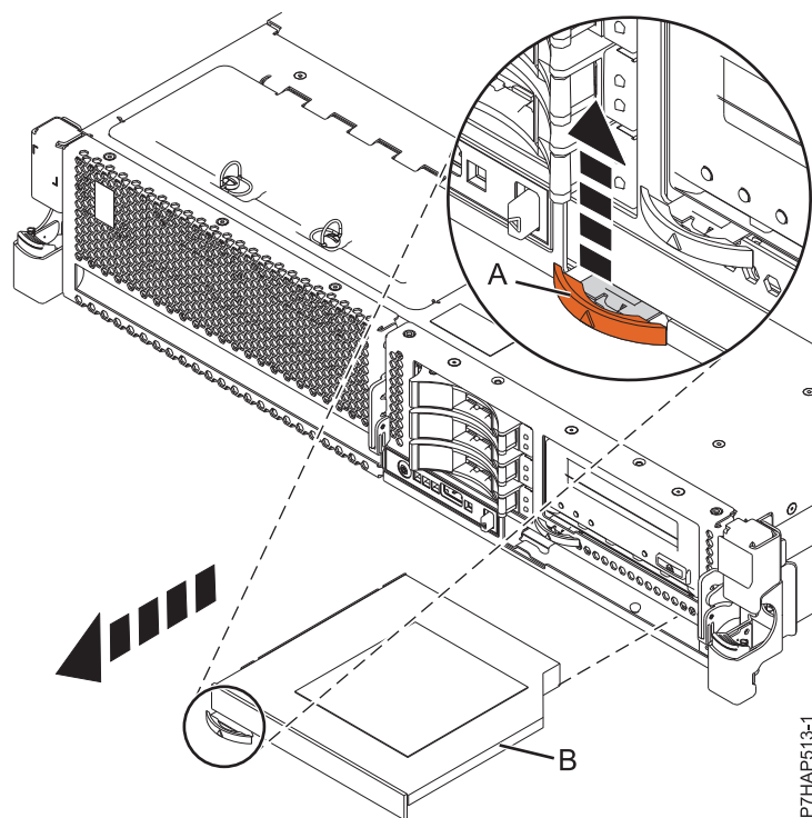
図5. ディスク・ドライブ・バックプレーンからの SAS メディア・デバイスの取り外し
