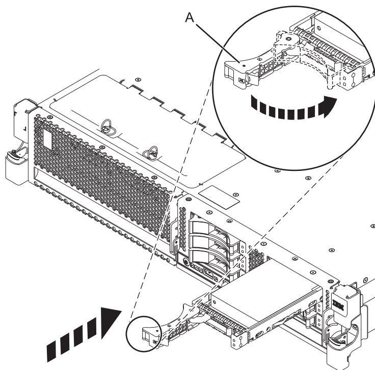
図 10. バックプレーン・ディスク・ドライブの取り付け
