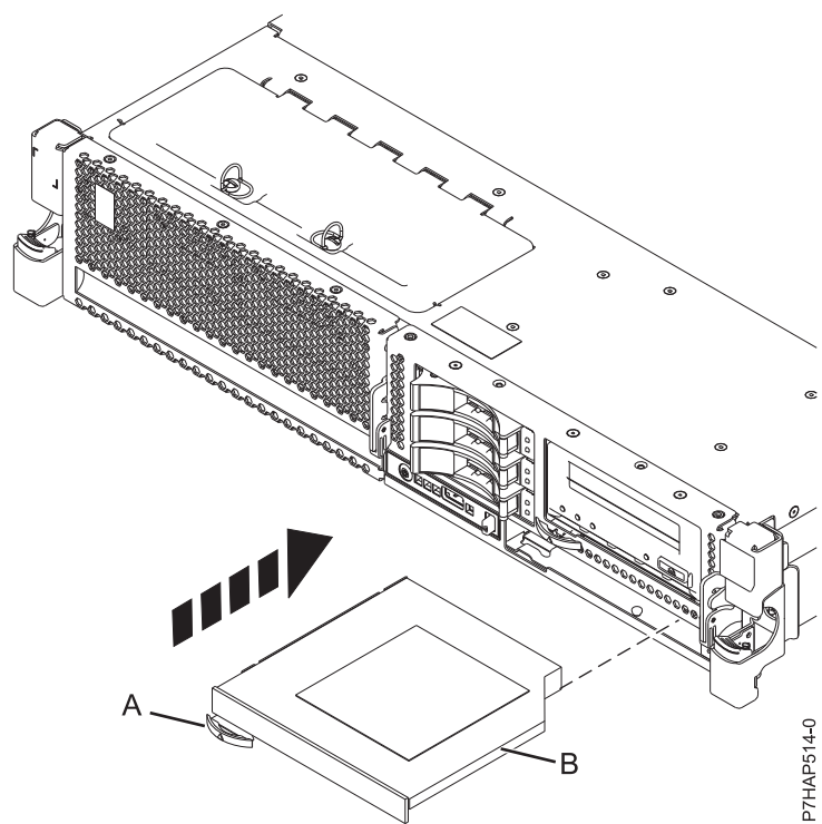
図 11. SAS メディア・デバイスの取り付け
