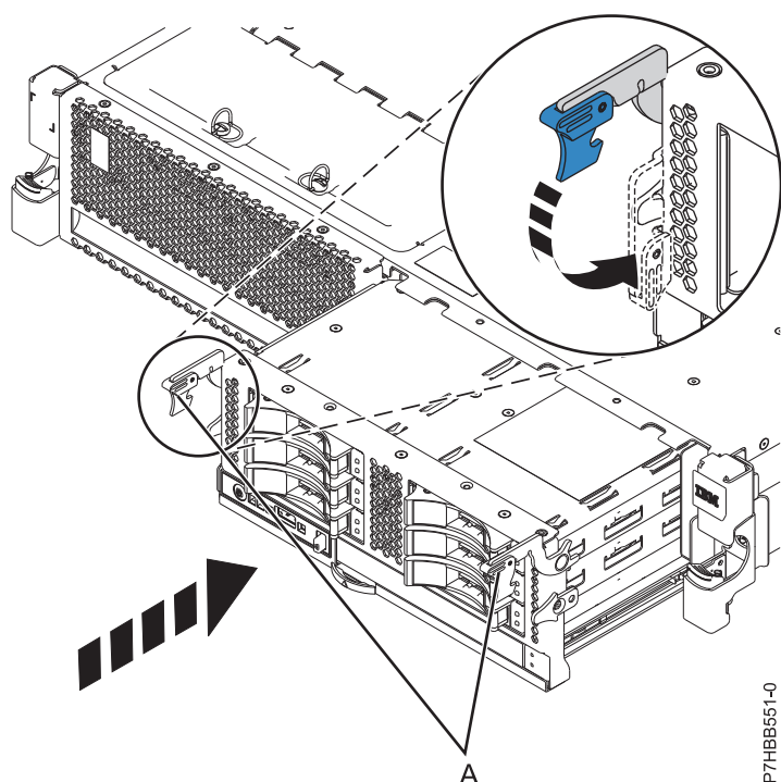
図9. ラック・マウント型モデルへのディスク・ドライブが装着されているバックプレーンの取り付け
