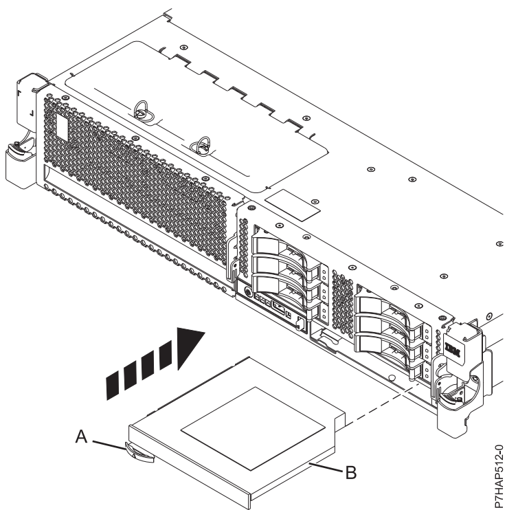
図 12. スリムライン・メディア・デバイスの取り付け
