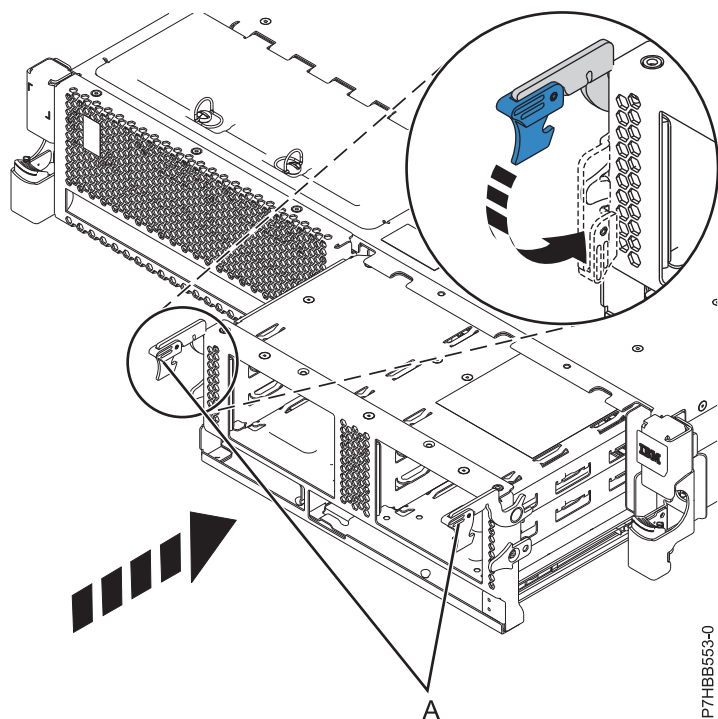
図8. ラック・マウント型モデルへのディスク・ドライブが装着されていないバックプレーンの取り付け
