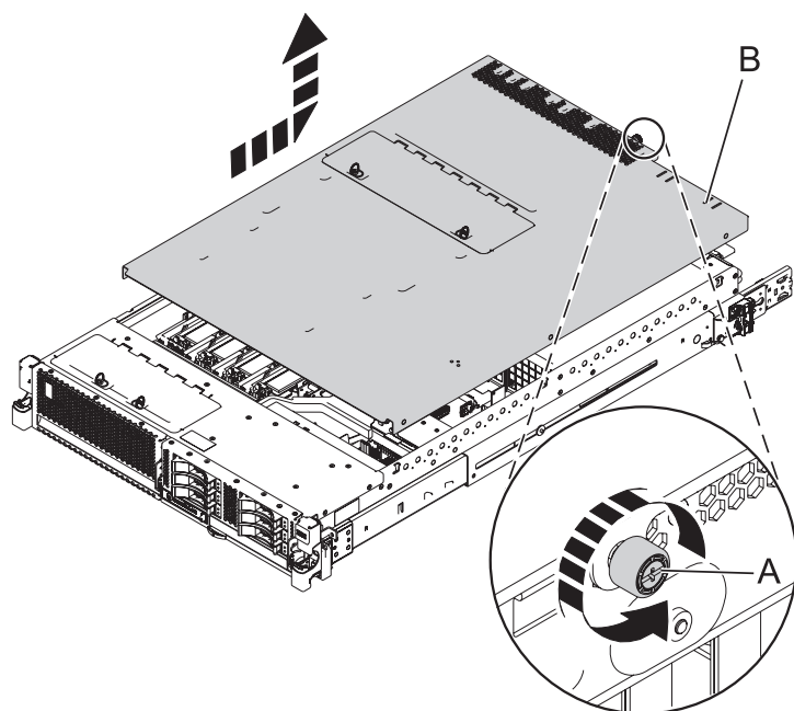
図 16. 保守アクセス・カバーの取り外し
