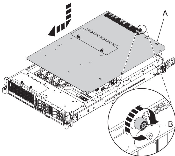
図 17. 保守アクセス・カバーの取り付け
