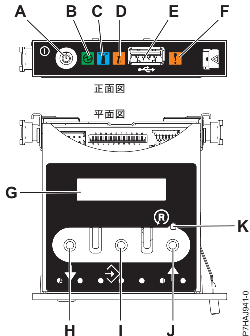
図 14. コントロール・パネル
