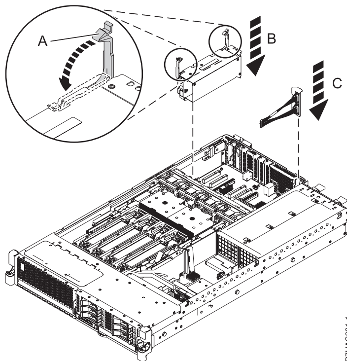
図 10. システムでの FC EJ0G GX アダプターの取り替え
