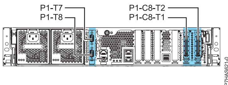
図 1. GX アダプターのスロットおよびロケーション・コード
