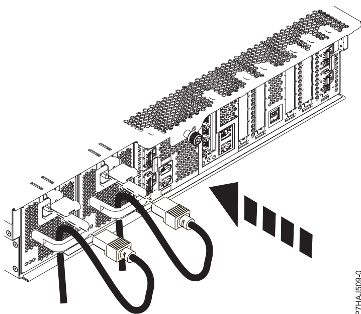
図 22. 電源コードの接続
