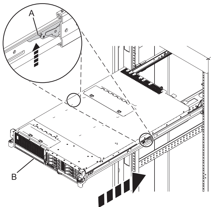
図 19. 安全レール・ラッチのアンロック
