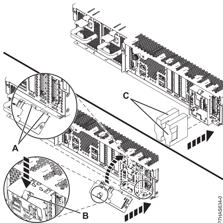
図 5. ケーブル保持ブラケットの取り付け
