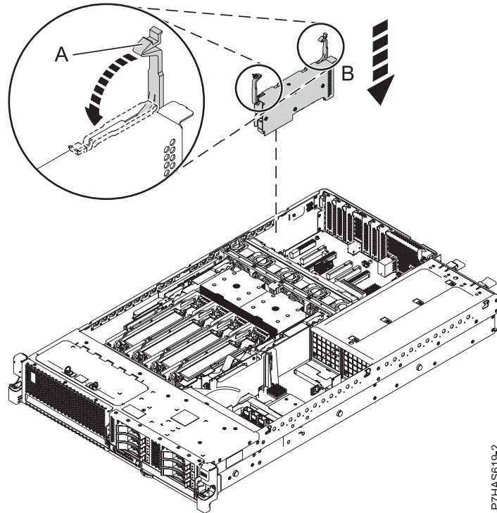
図 11. システムでの FC EJ0H GX アダプターの取り替え
