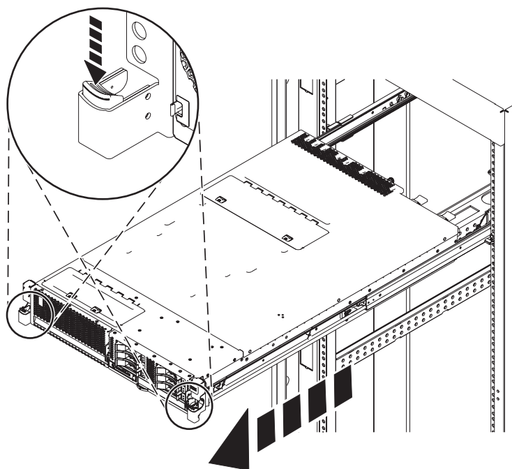
図 18. システムの保守位置への設置
