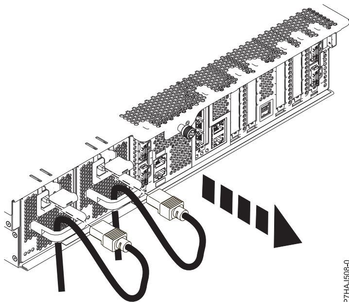
図 15. 電源コードの取り外し
