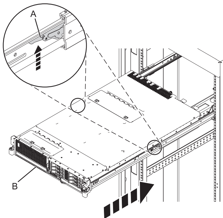
図 13. 安全レール・ラッチのアンロック
