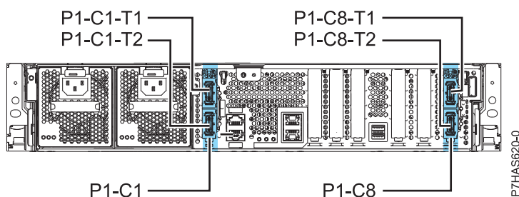
図 1. GX アダプターのスロットおよびロケーション・コード
