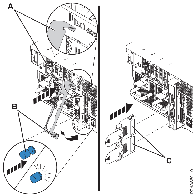
図 7. ケーブル保持ブラケットの取り付け
