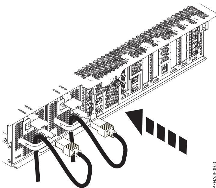
図 16. 電源コードの接続
