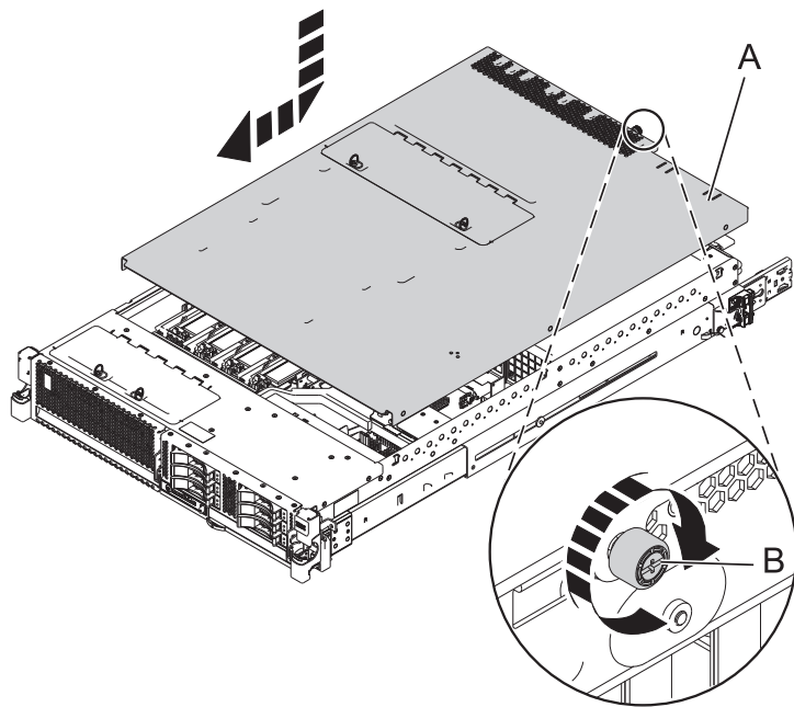
図 11. 保守アクセス・カバーの取り付け
