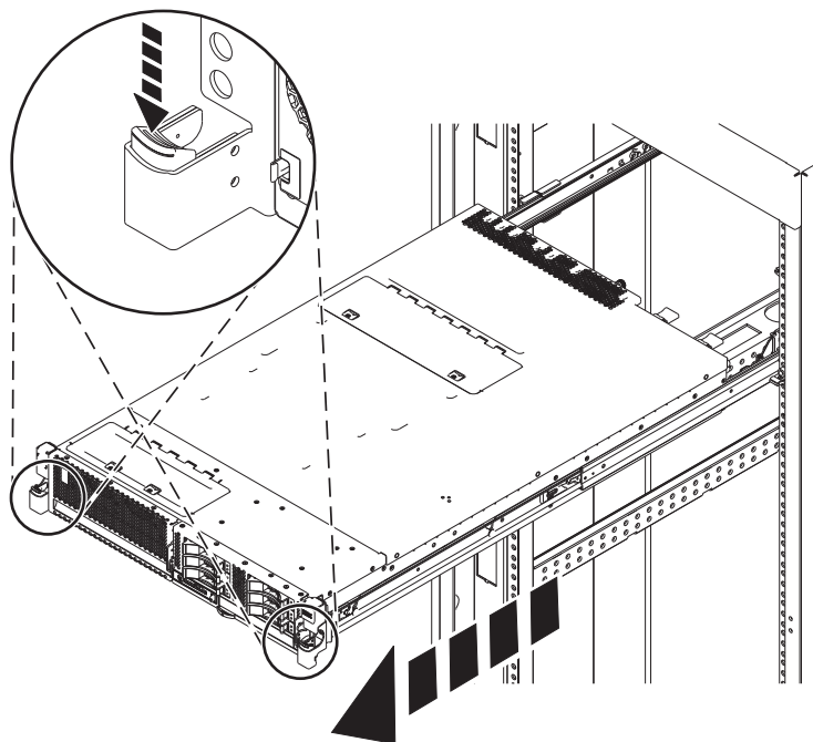
図 12. システムの保守位置への設置
