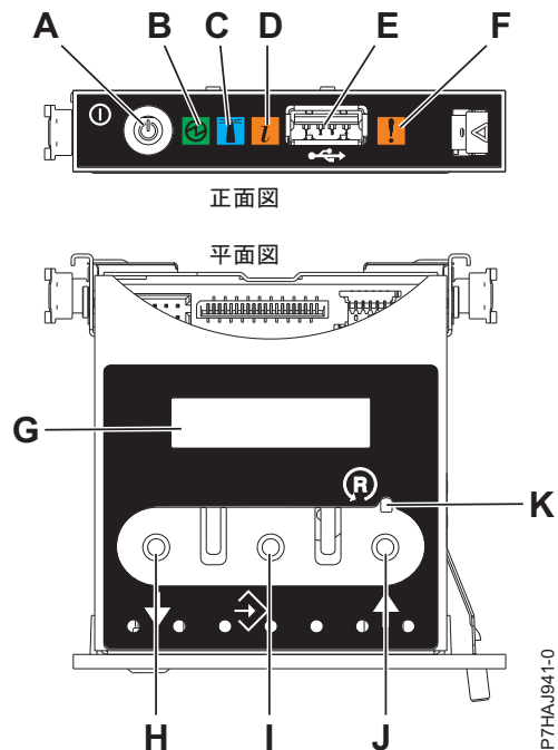
図 8. コントロール・パネル
