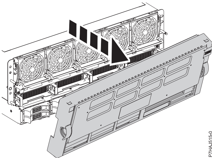
図 14. カバーの取り外し
