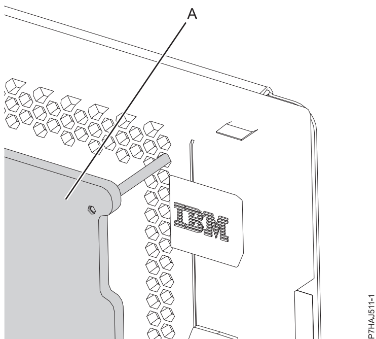
図 10. カバー取り外しツールの位置合わせ
