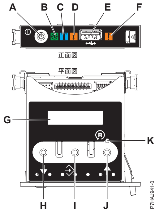
図 5. コントロール・パネル
