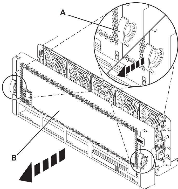
図 8. 前面カバーの取り外し
