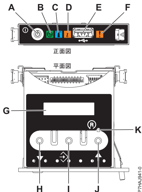
図6. コントロール・パネル
