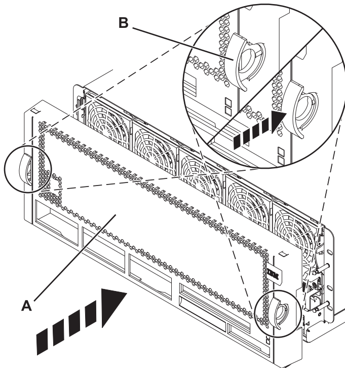
図 15. 前面カバーの取り付け
