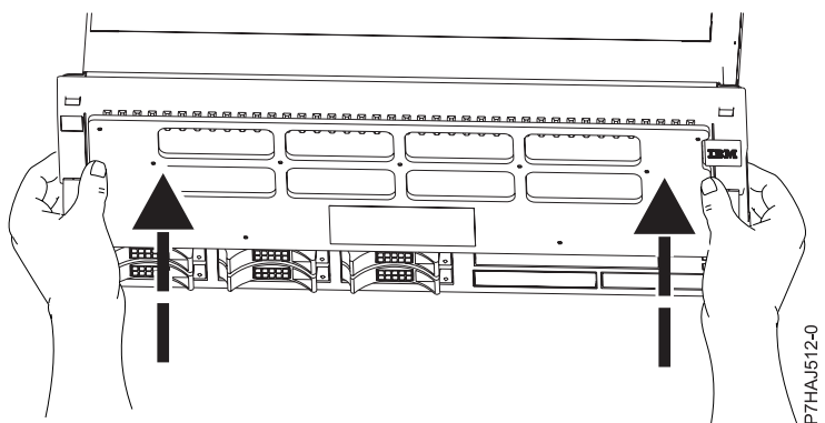
図 11. カバー取り外しツールの使用
