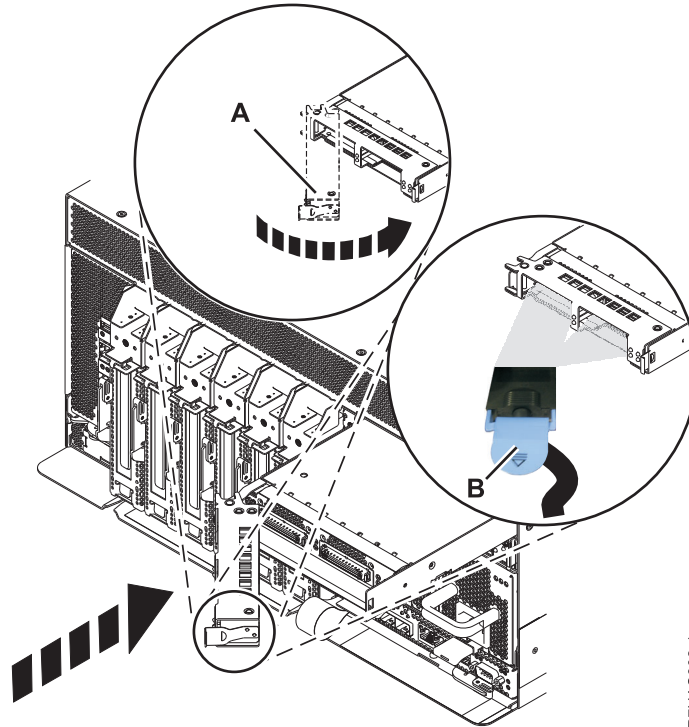
図2. システムへの GX アダプターの取り付け
