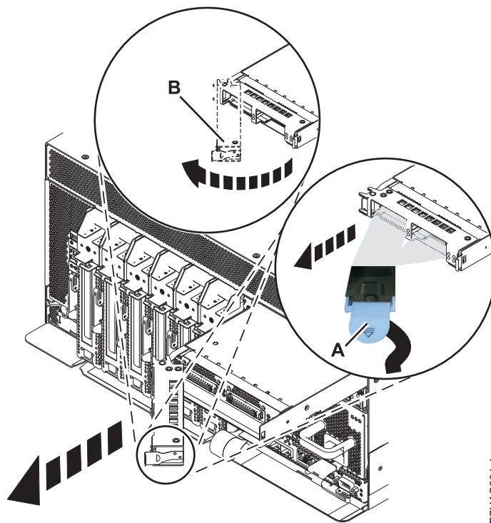
図3. システムからの GX アダプターの取り外し
