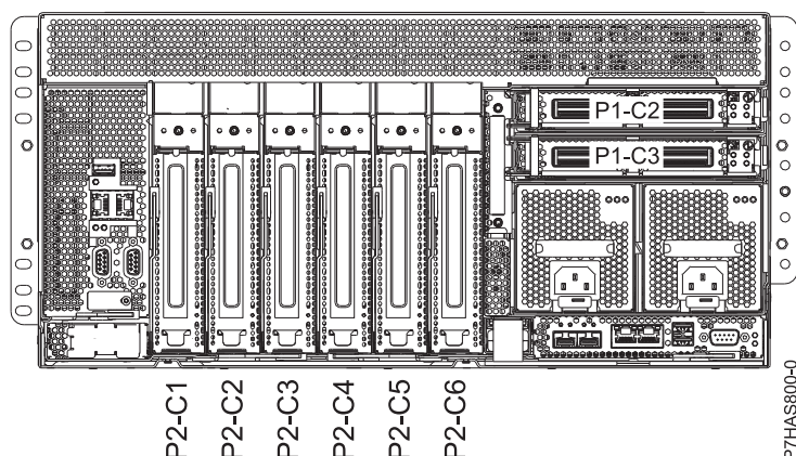
図1. ロケーション・コード付きシステム背面図
