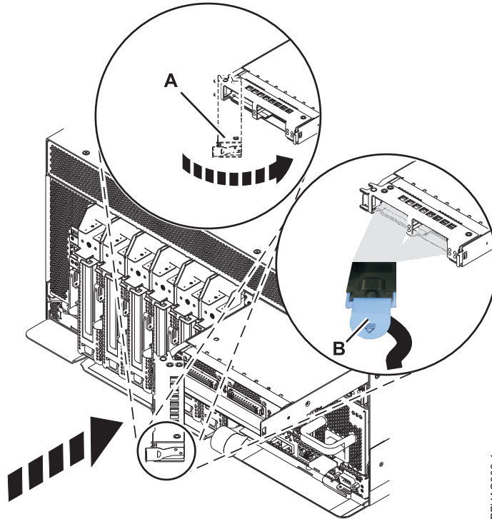
図4. システム内の GX アダプターの取り替え
