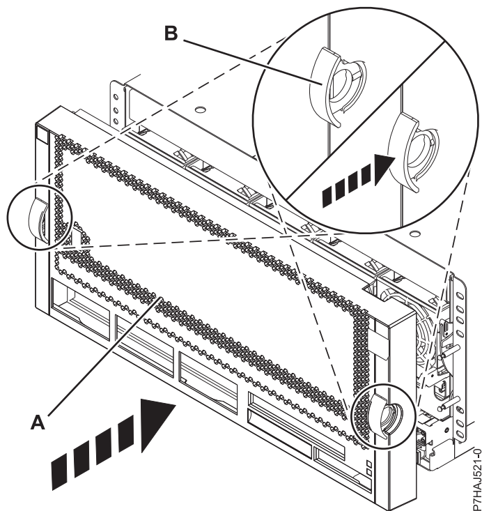
図 8. 前面カバーの取り付け
