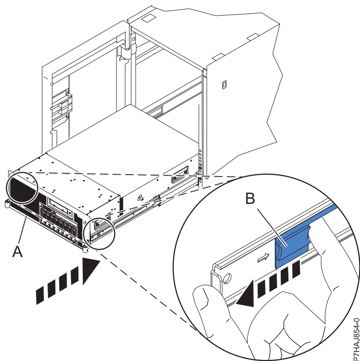
図 14. レール安全ラッチの解除
