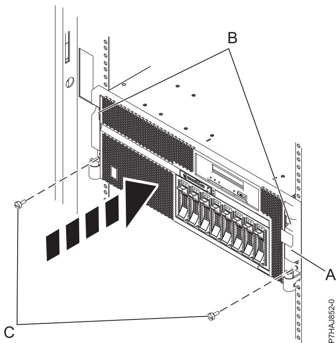
図 15. つまみねじの取り替え
