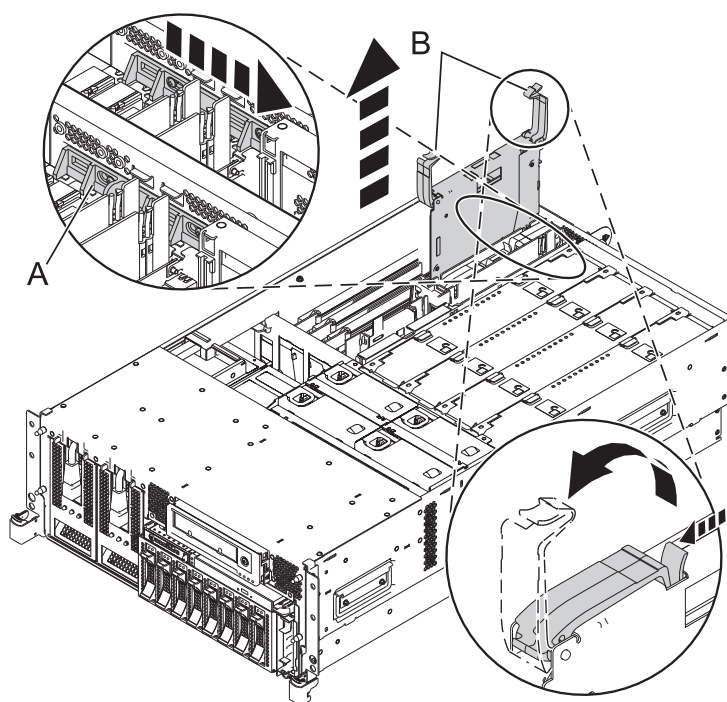
図2. ラック・マウント型システムからのアダプターの取り外し
