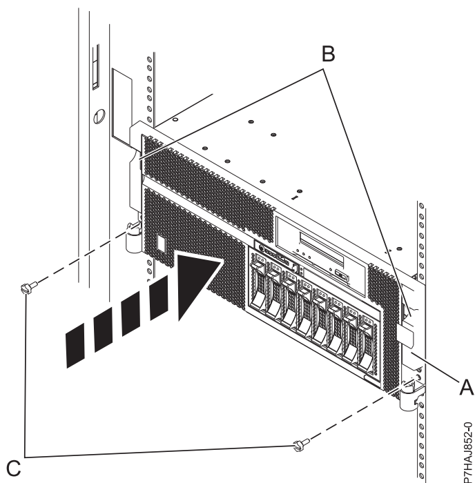
図 10. 前面カバーの取り付け
