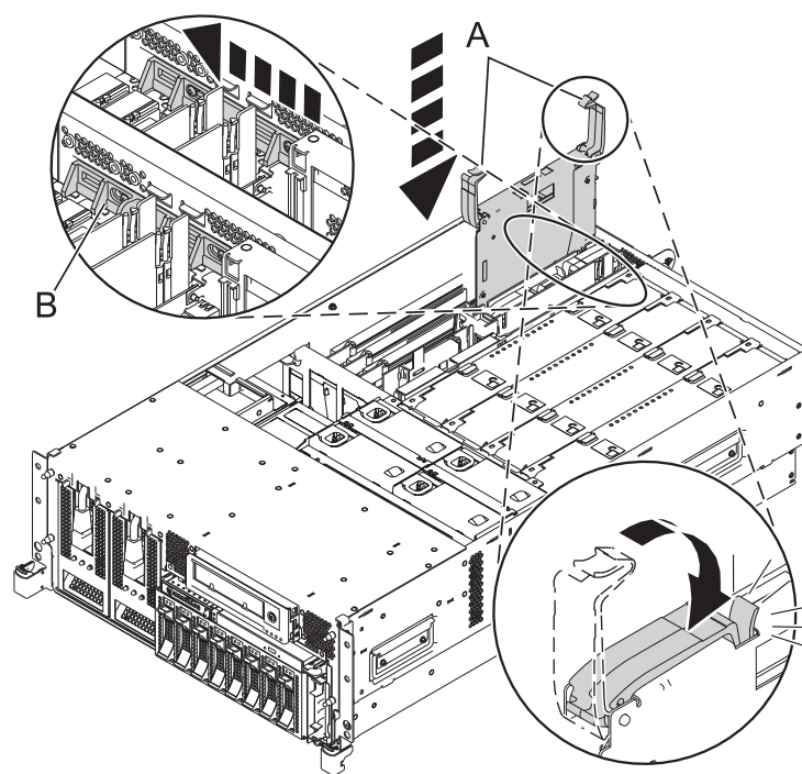
図3. ラック・マウント型システムへのアダプターの取り付け
