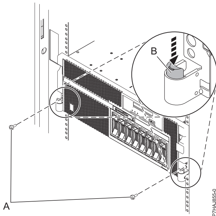
図 13. ラック・ラッチの解除
