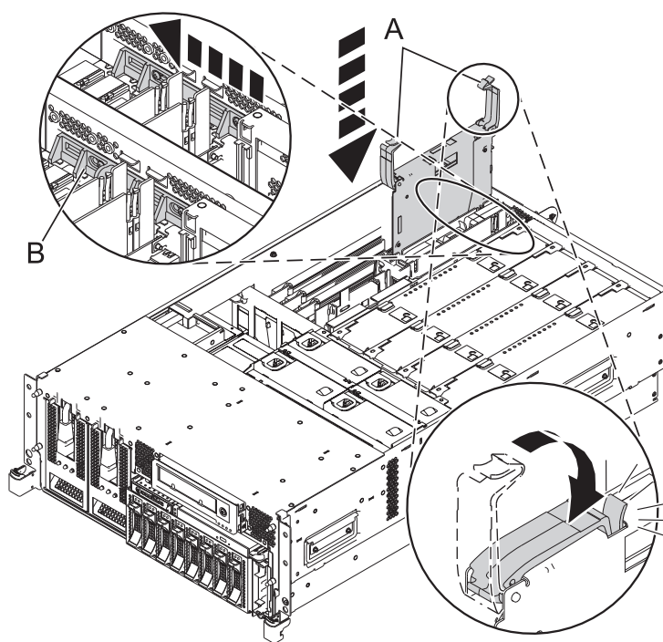
図6. ラック・マウント型システムへのアダプターの取り付け
