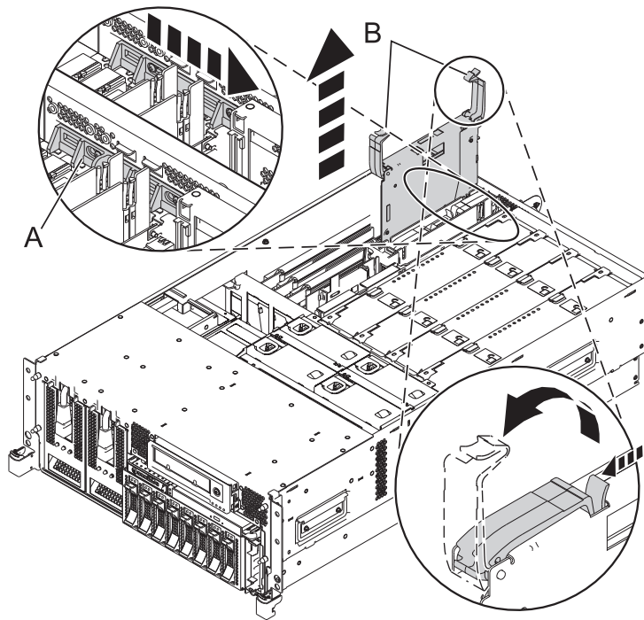
図5. ラック・マウント型システムからのアダプターの取り外し
