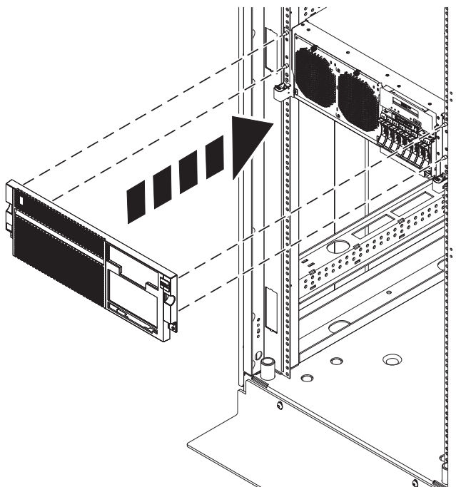
図 15. 前面カバーの取り外し
