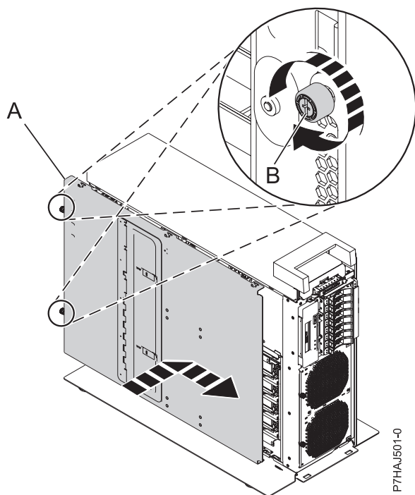
図 22. 内側の保守アクセス・カバーの取り付け
