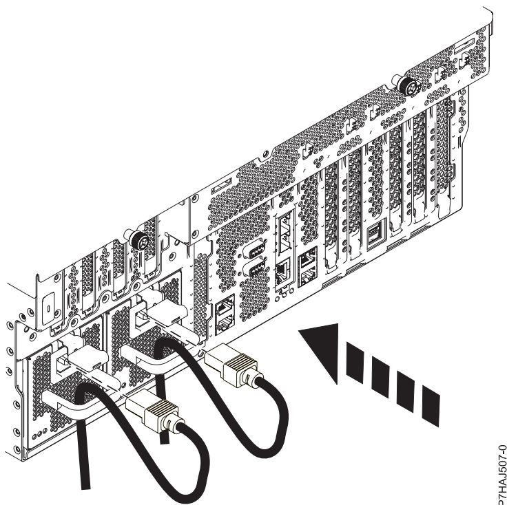
図 28. 電源コードの接続
