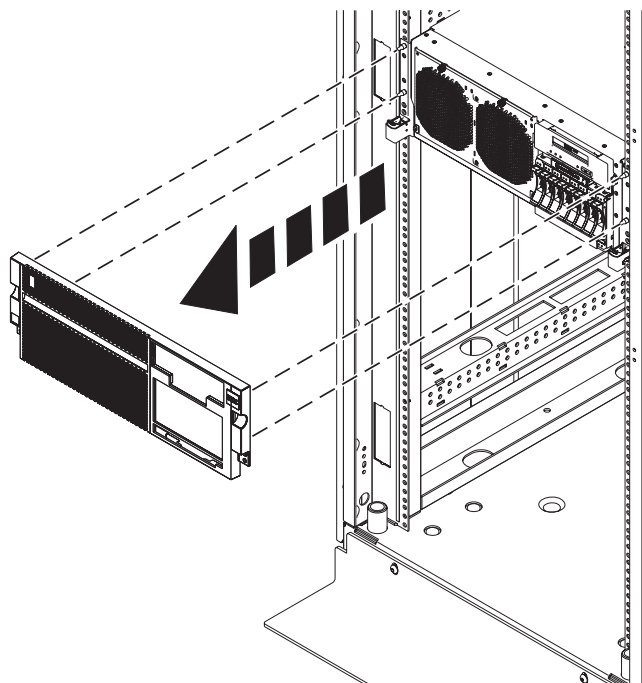
図 13. 前面カバーの取り外し
