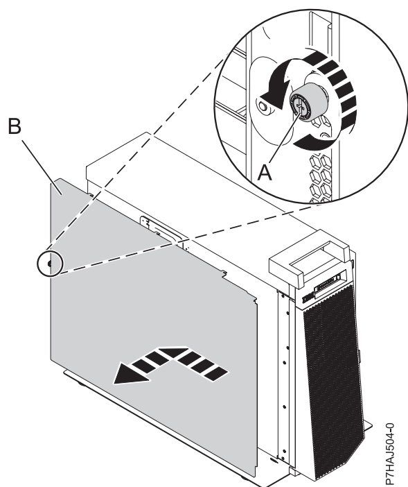
図 19. 外側の保守アクセス・カバーの取り付け
