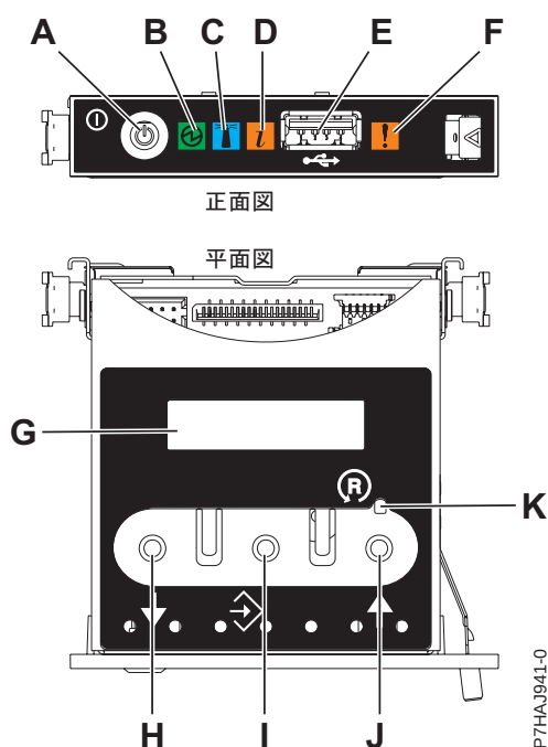
図 12. コントロール・パネル
