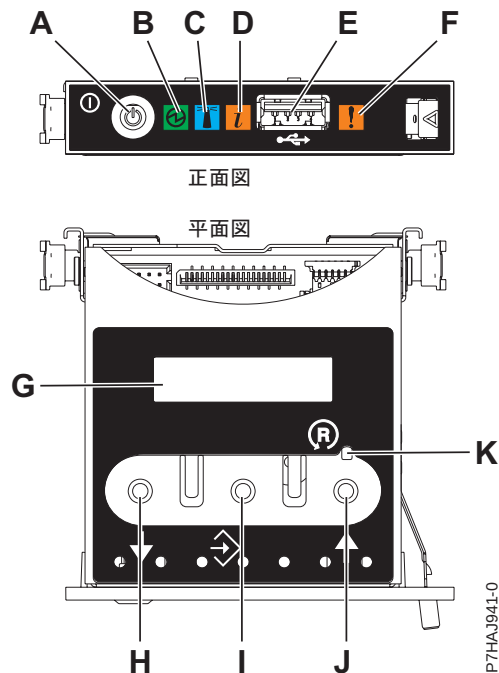
図 11. コントロール・パネル
