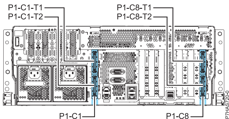
図 2. GX++ アダプター・スロット P1-C1 および P1-C8 を示す 8202-E4C、8202-E4D、8205-E6C、または 8205-E6D の背面図
