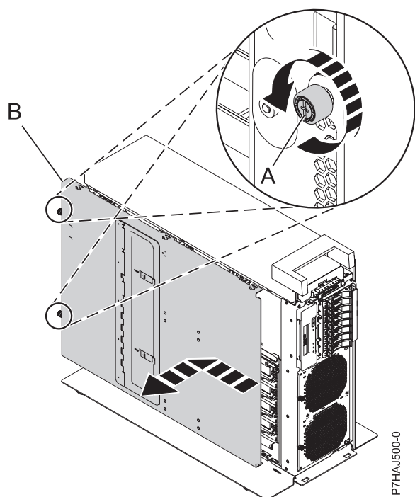
図 20. 内側の保守アクセス・カバーの取り外し
