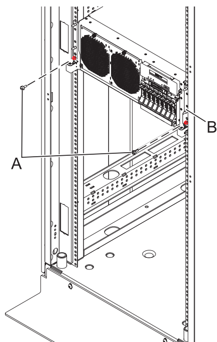
図 24. システム装置の保守位置への設置
