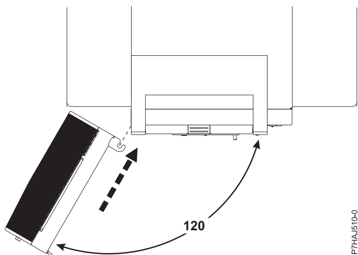
図 17. 前面ドアの取り付け
