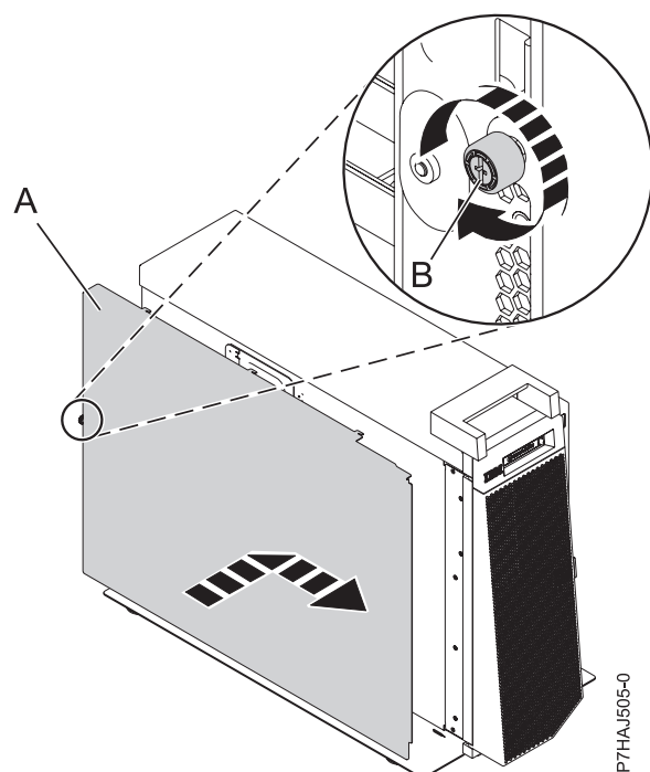
図 23. 外側の保守アクセス・カバーの取り付け
