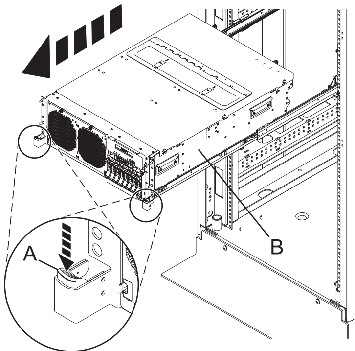
図 25. システム装置の保守位置へのロック
