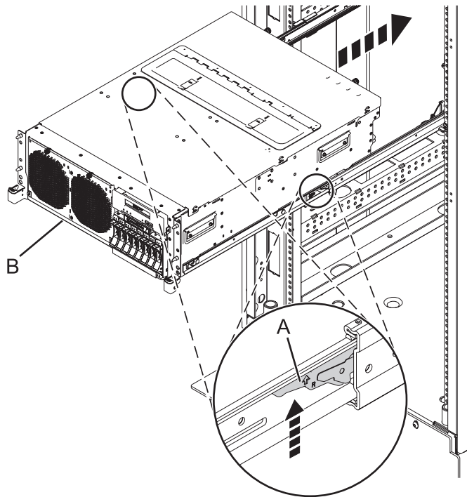
図 26. システム装置の操作位置への設置
