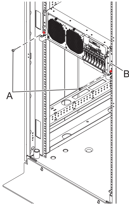
図 27. システム装置の操作位置への設置
