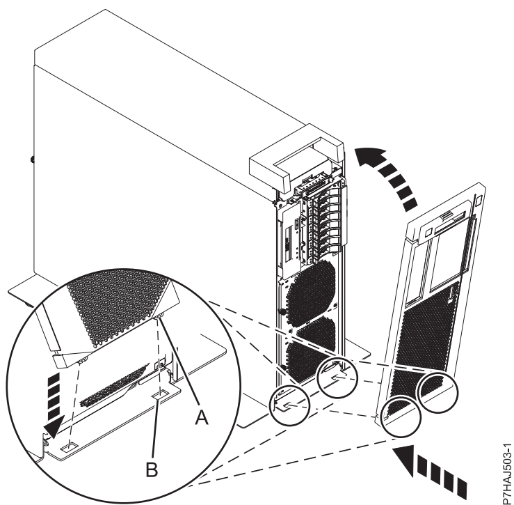
図 16. 前面カバーの取り付け
