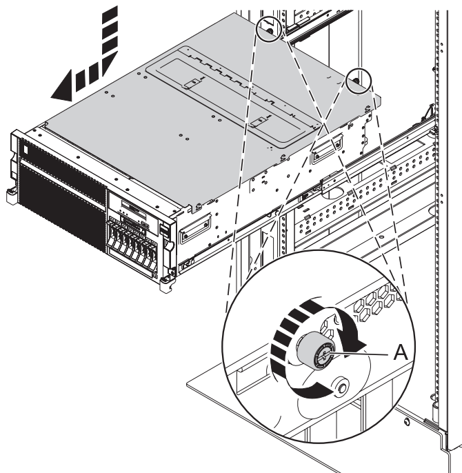
図 21. 保守アクセス・カバーの取り付け
