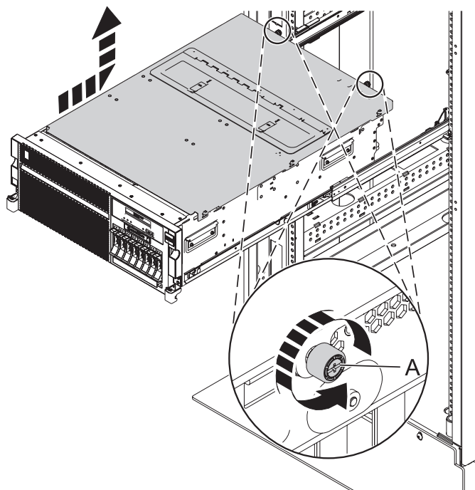
図 18. 保守アクセス・カバーの取り外し
