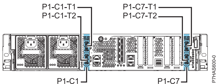
図 1. GX アダプター・スロットおよびロケーション・コードを示す、8231-E2B システムの背面図
