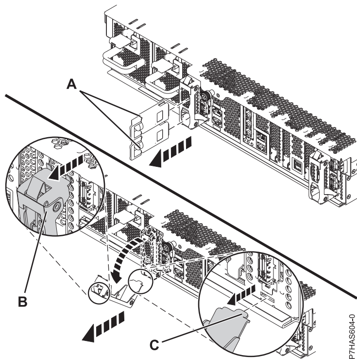
図 5. ケーブル保持ブラケットの取り外し
