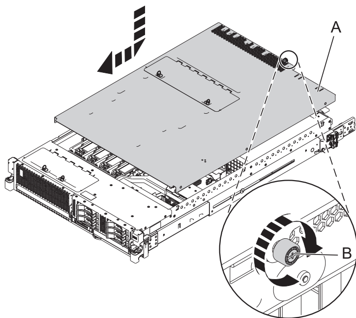
図 12. 保守アクセス・カバーの取り付け
