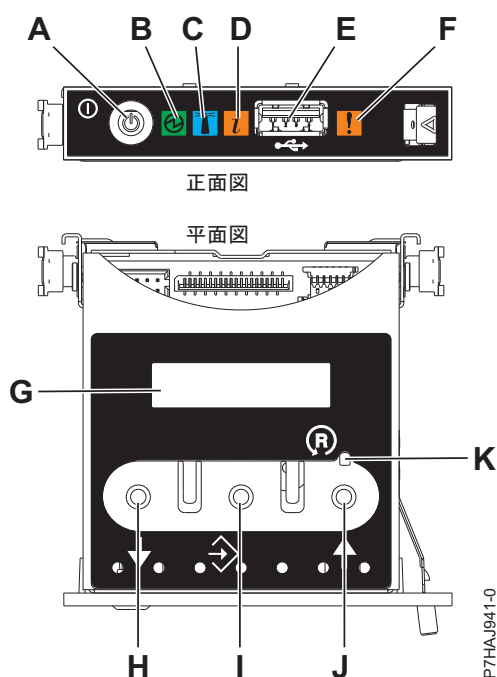
図 10. コントロール・パネル
