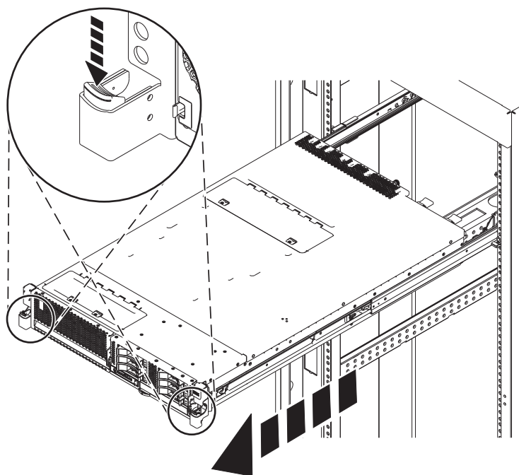
図 13. システムの保守位置への設置
