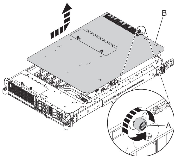
図 11. 保守アクセス・カバーの取り外し
