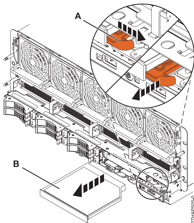
図 12. スリムライン・メディア装置の取り外し
