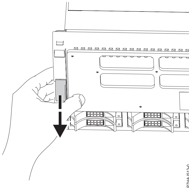
図 26. カバー・ラッチの解放
