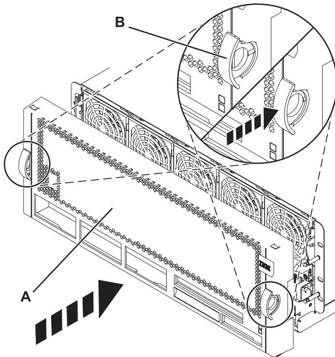
図 29. 前面カバーの取り付け
