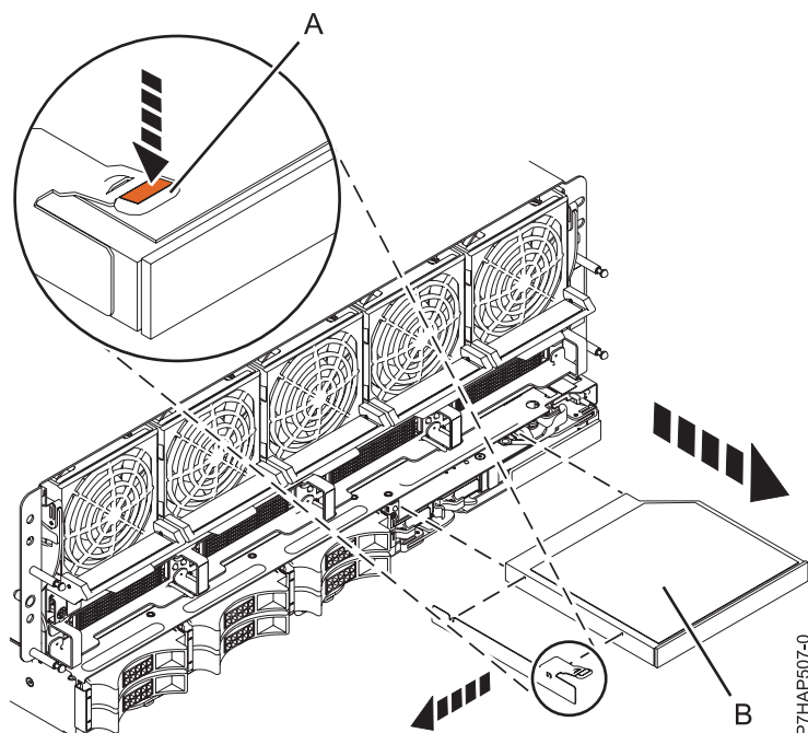
図 9. デバイス並行保守の画面の例
