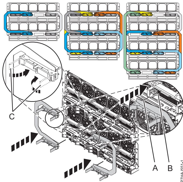
図 20. SMP ケーブルの取り付け
