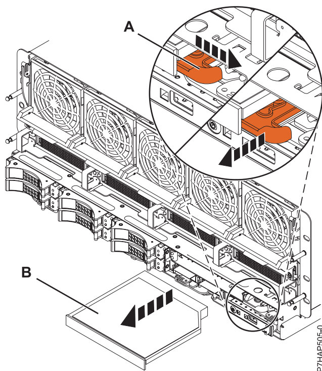
図 3. スリムライン・メディア装置の取り外し
