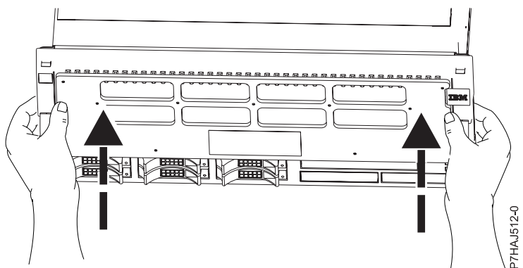
図 25. カバー取り外しツールの使用
