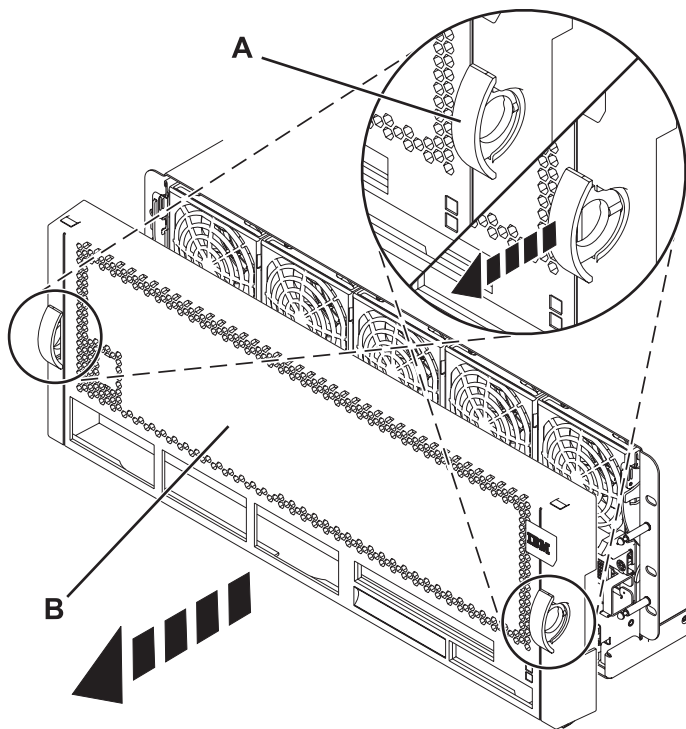
図 22. 前面カバーの取り外し
