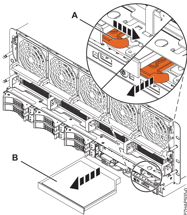
図 7. スリムライン・メディア装置の取り外し
