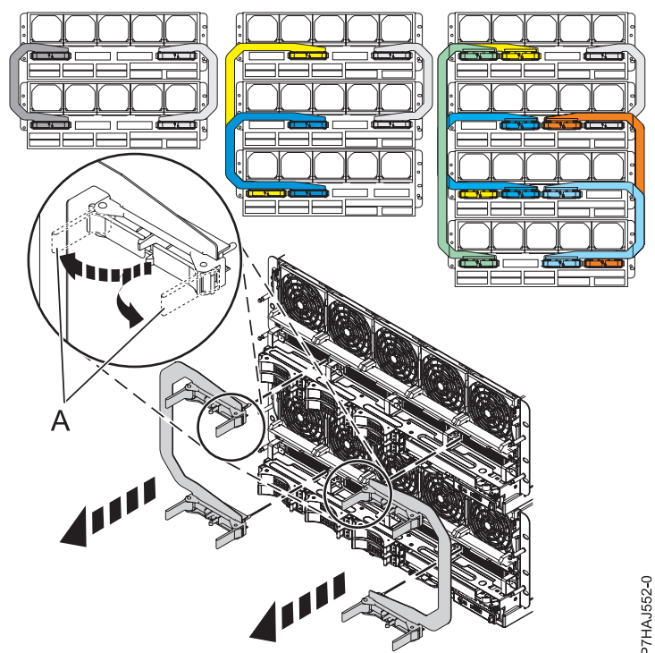
図 17. SMP ケーブルの切り離し
