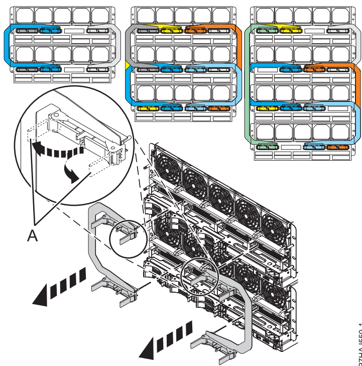
図 18. SMP ケーブルの切り離し
