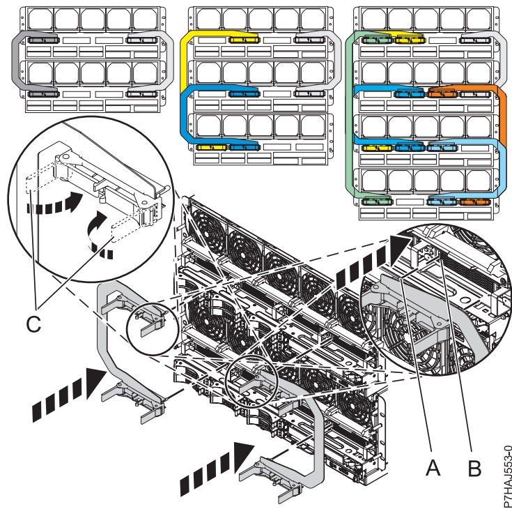
図 19. SMP ケーブルの再接続
