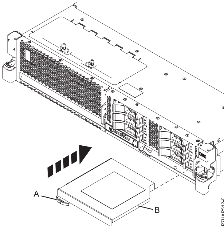
図 18. スリムライン・メディア装置の取り付け
