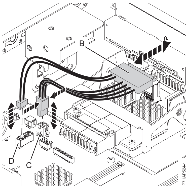
図 3. メディア・ケーブル接続
