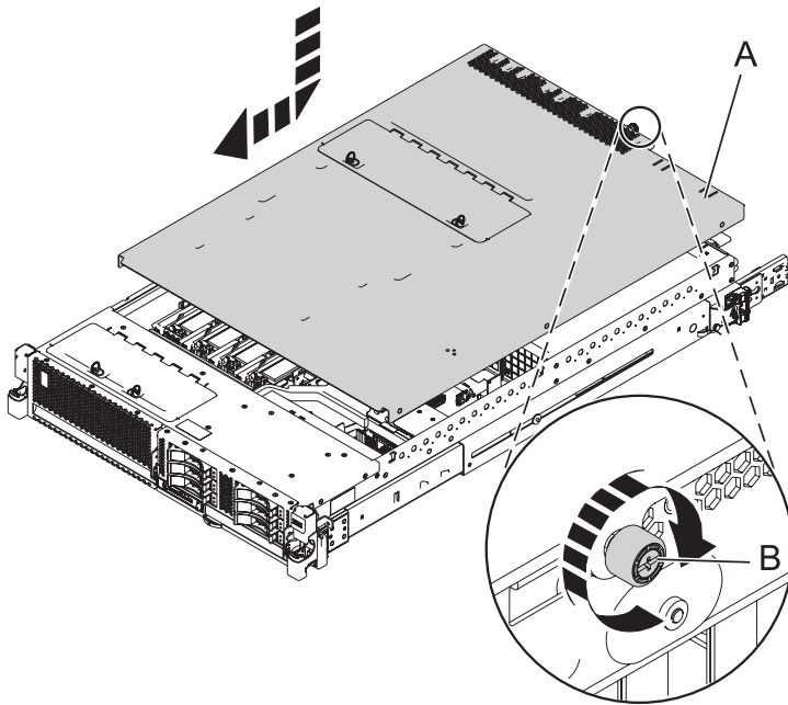
図 27. 保守アクセス・カバーの取り付け
