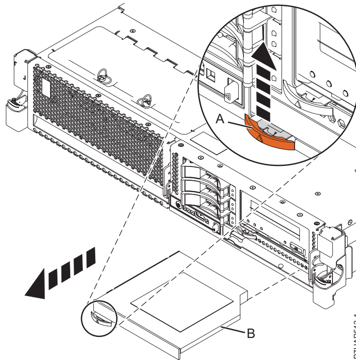
図4. スリムライン・メディア装置の取り外し
