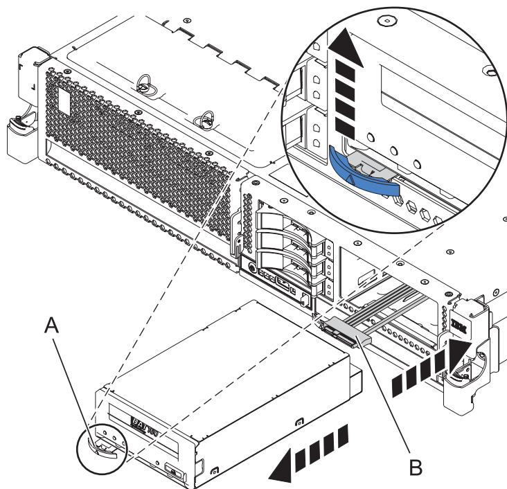
図 1. SAS メディア装置の取り外し
