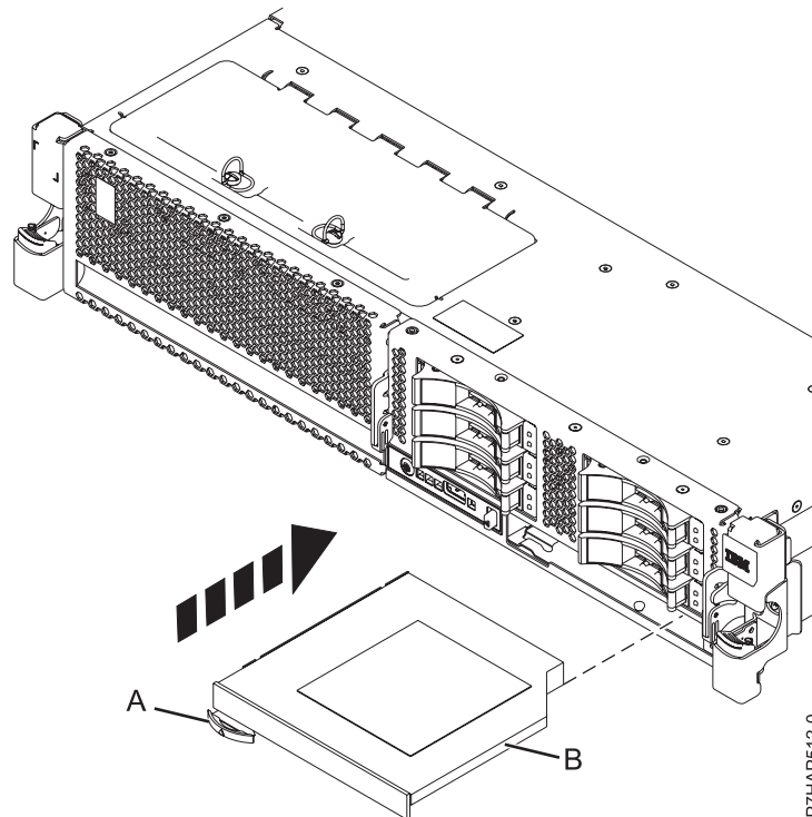
図 12. スリムライン・メディア装置の取り付け
