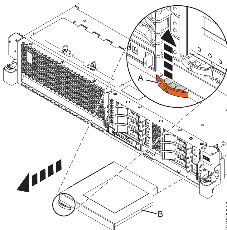
図6. スリムライン・メディア装置の取り外し
