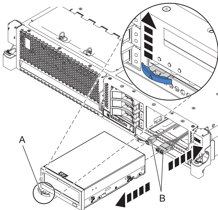
図 19. メディア装置の取り外し
