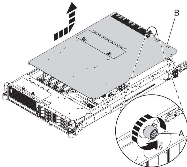
図 26. 保守アクセス・カバーの取り外し
