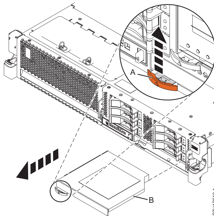
図 11. スリムライン・メディア装置の取り外し
