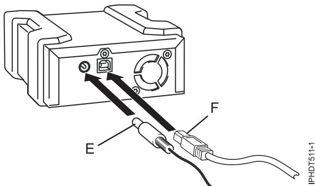
図 23. USB と電源機構ケーブルの接続
