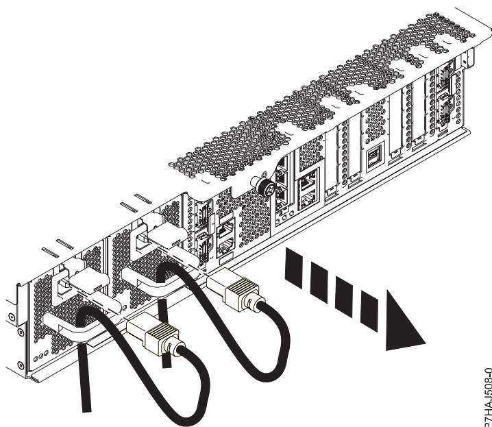
図 31. 電源コードの取り外し
