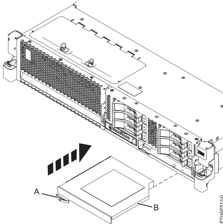
図 17. スリムライン・メディア装置の取り付け
