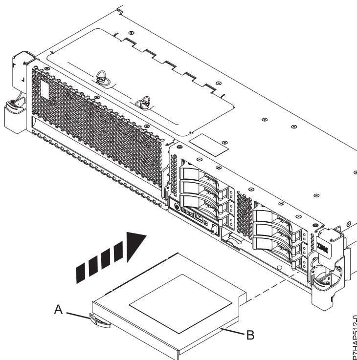
図 15. スリムライン・メディア装置の取り付け
