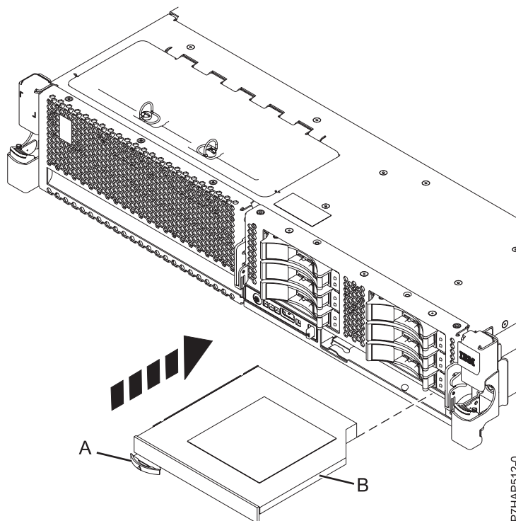
図 8. スリムライン・メディア装置の取り付け
