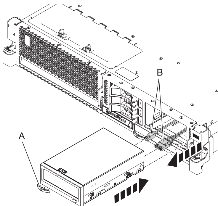
図 21. USB ディスク・ドライブの取り付け
