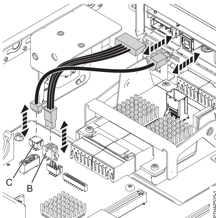
図 22. メディア・ケーブル接続
