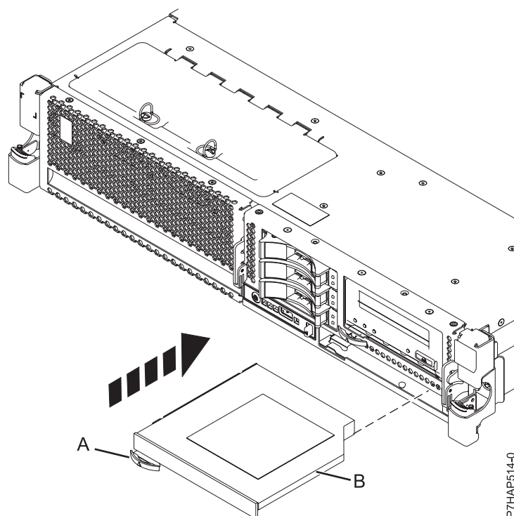
図 5. スリムライン・メディア装置の取り付け
