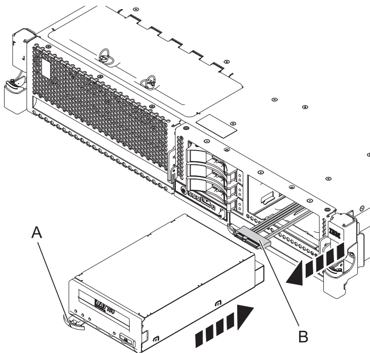
図 2. SAS メディア装置の取り付け
