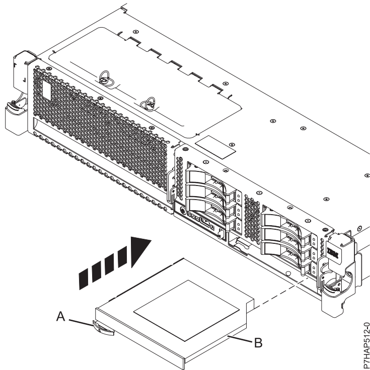
図7. スリムライン・メディア装置の取り付け
