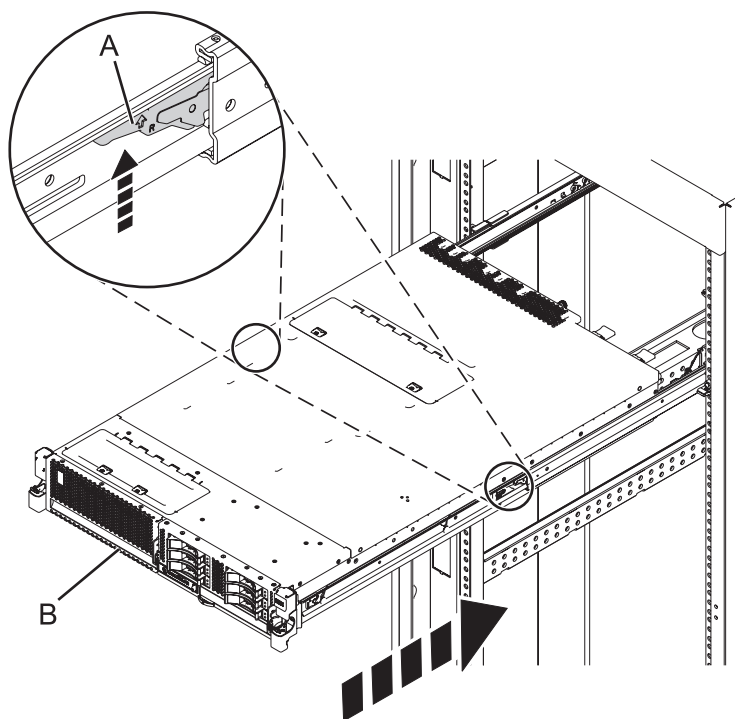
図 29. レール安全ラッチのアンロック
