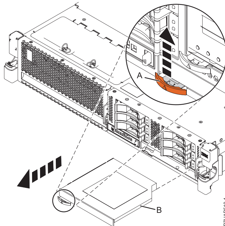
図 16. スリムライン・メディア装置の取り外し
