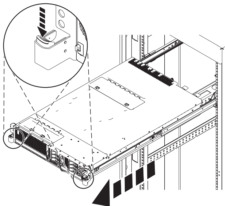
図 28. システムの保守位置への設置
