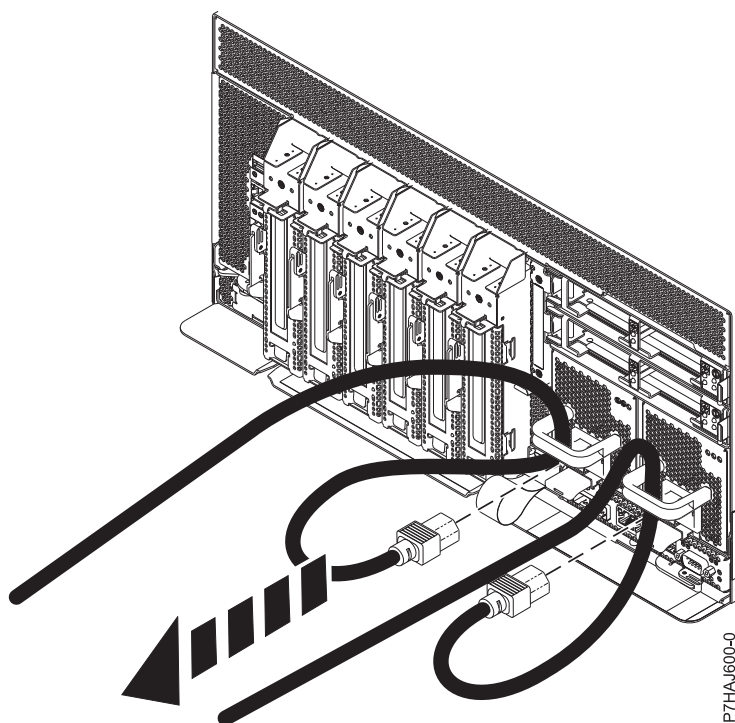
図 10. 電源コードの切り離し
