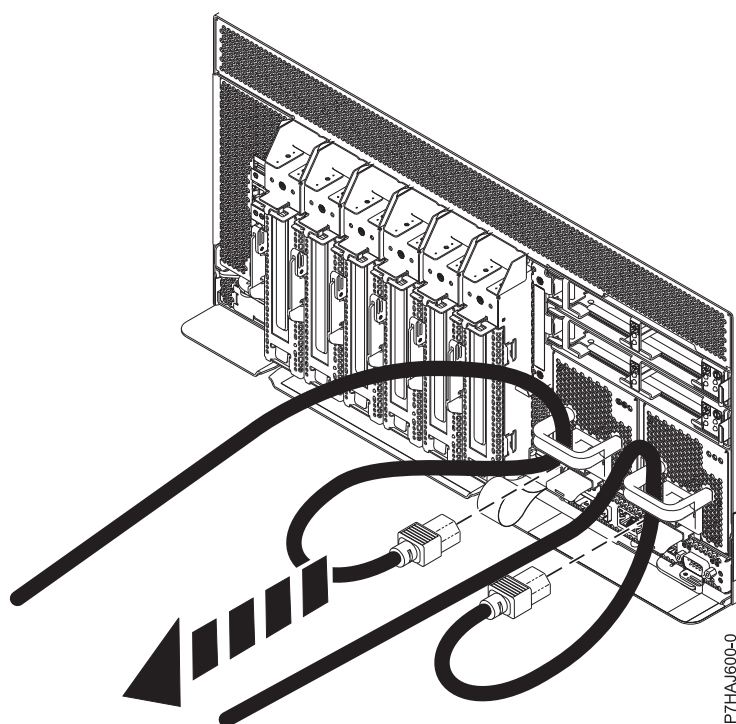
図 4. 電源コードの切り離し
