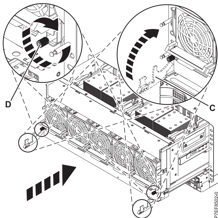
図 32. システム装置解放ラッチのロック
