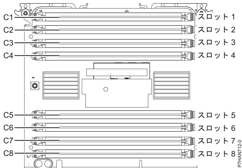
図 15. 8248-L4T、8408-E8D、または9109-RMD のメモリー・モジュール・スロットの位置
