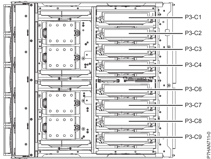
図 14. メモリー・ライザーの差し込み順序
