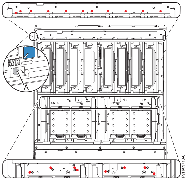
図 8. プレーナー上のプッシュボタン
