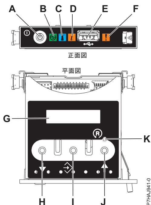
図 26. コントロール・パネル
