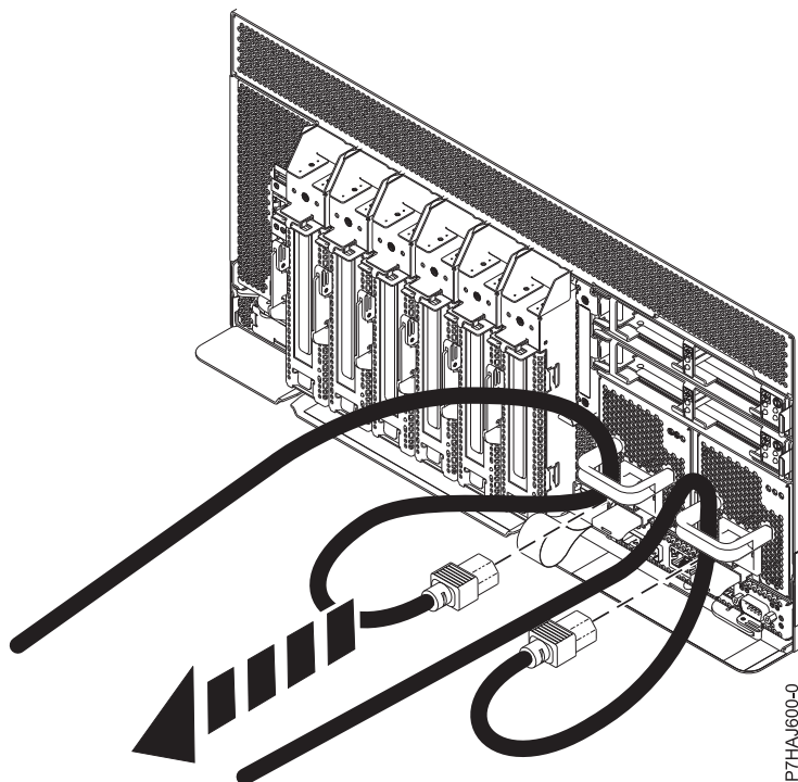
図 16. 電源コードの切り離し
