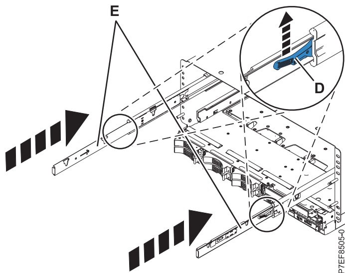
図 31. レール安全ラッチのアンロック
