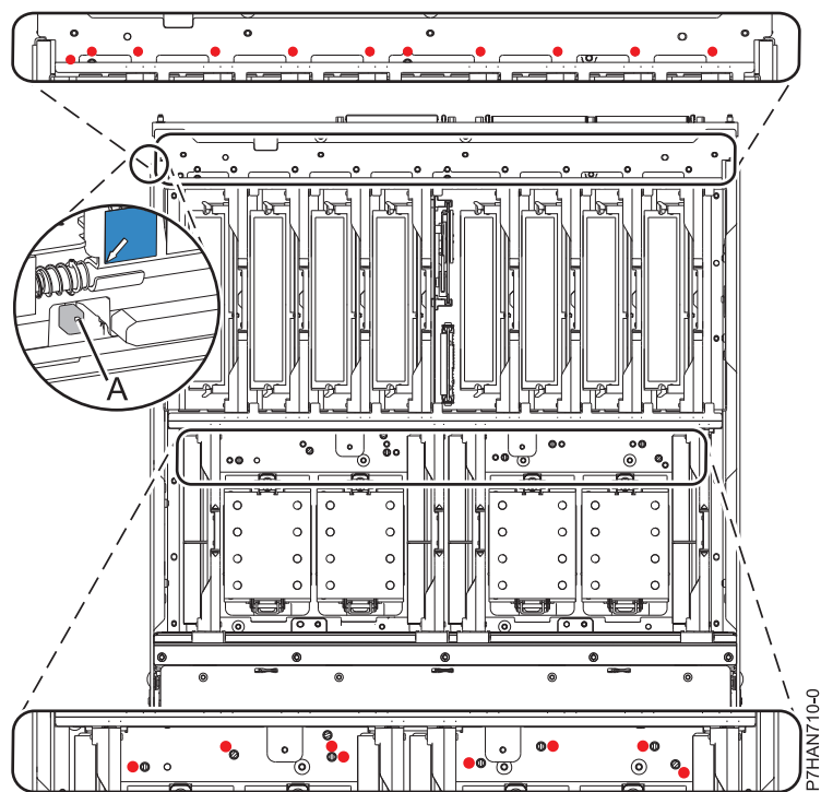
図 11. プレーナー上のプッシュボタン
