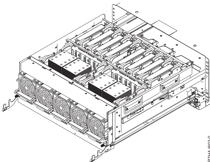
図 30. 保守位置のシステム
