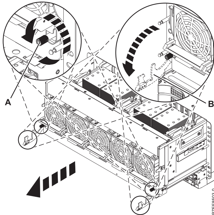
図 29. サイド・ラッチの解放
