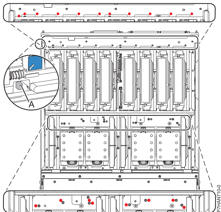
図 17. プレーナー上のプッシュボタン
