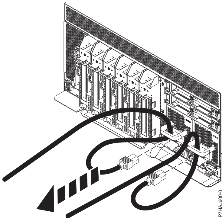
図7. 電源コードの切り離し
