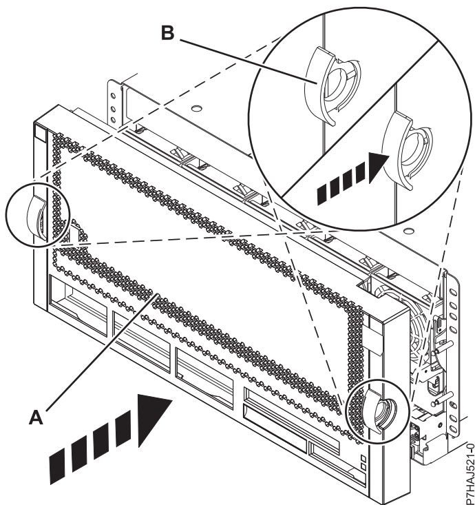
図 28. 前面カバーの取り付け
