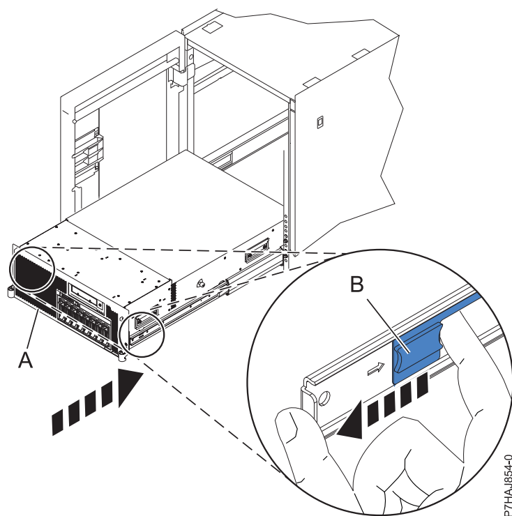
図 15. レール安全ラッチの解放
