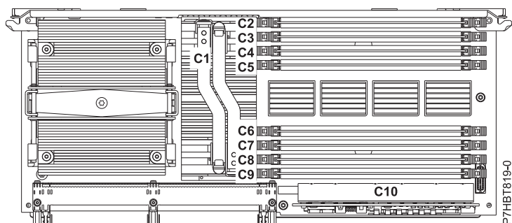
図1. プロセッサ・アセンブリ内のメモリー・モジュール・スロットの位置
