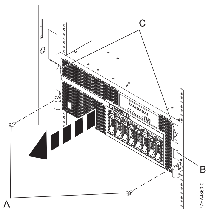
図 10. 前面カバーの取り外し
