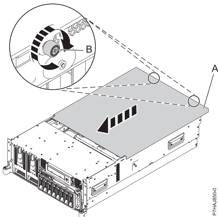
図 13. 保守アクセス・カバーの取り付け
