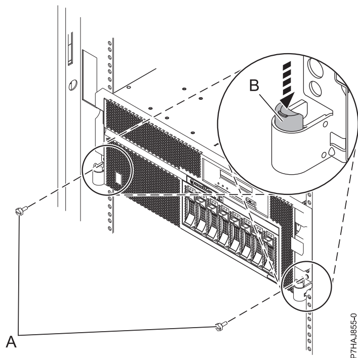
図 14. ラック・ラッチの解除
