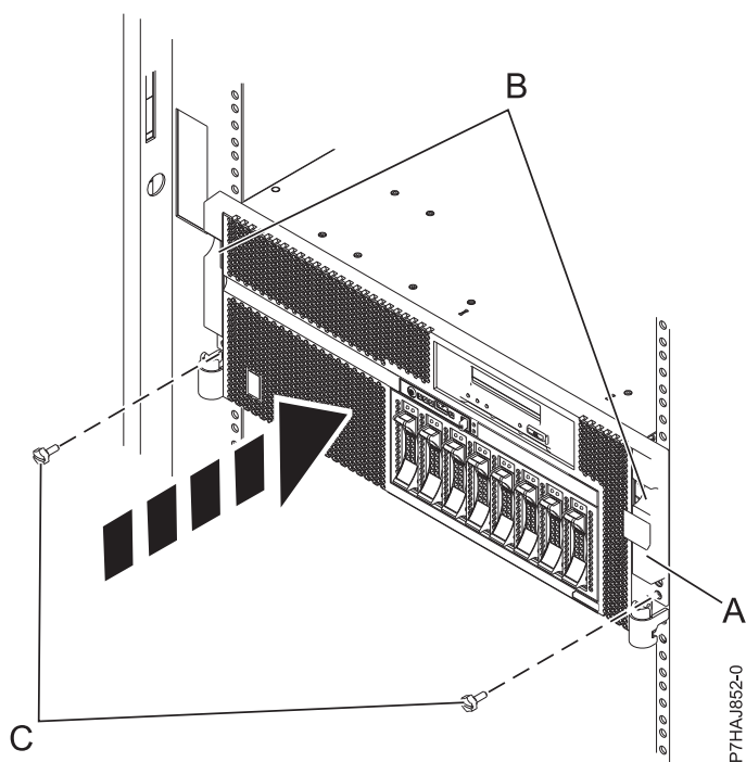
図 16. つまみねじの再取り付け
