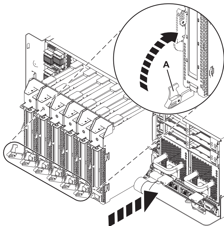
図3. システム装置に取り付けられる PCI アダプター・カセット
