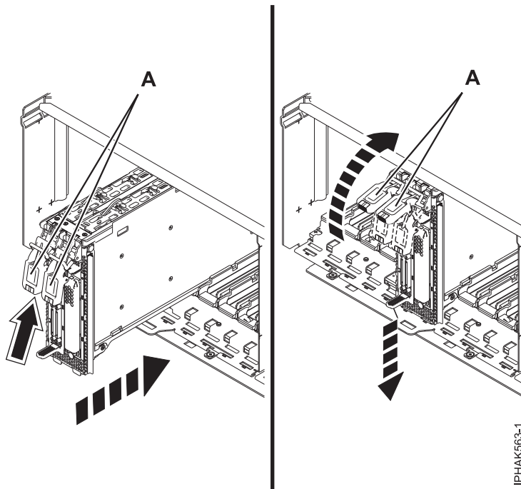
図 64. 入出力拡張装置へのカセット・アセンブリーの取り付け
