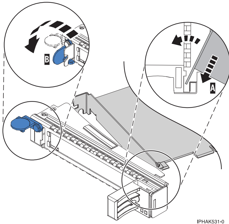
図 144. シングル幅 PCI アダプター・カセットから取り外されたアダプター
