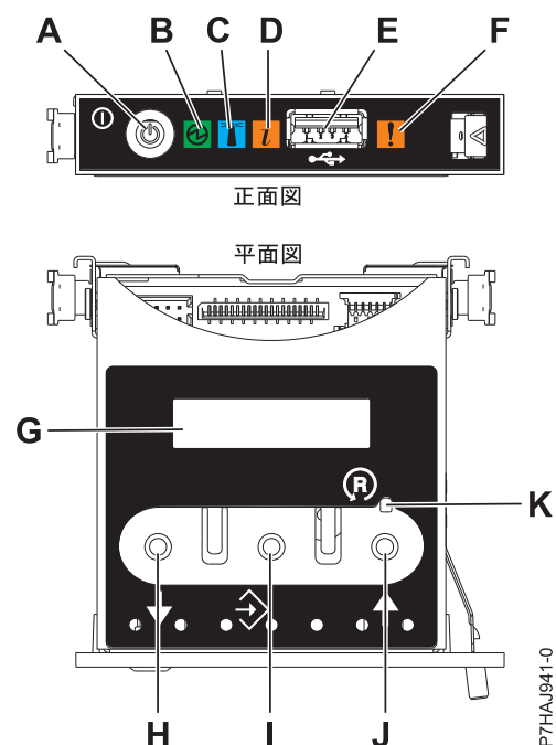
図 164. コントロール・パネル
