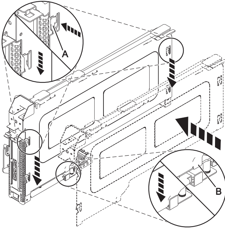
図 21. 元に戻された PCI アダプター・カセット・カバー
