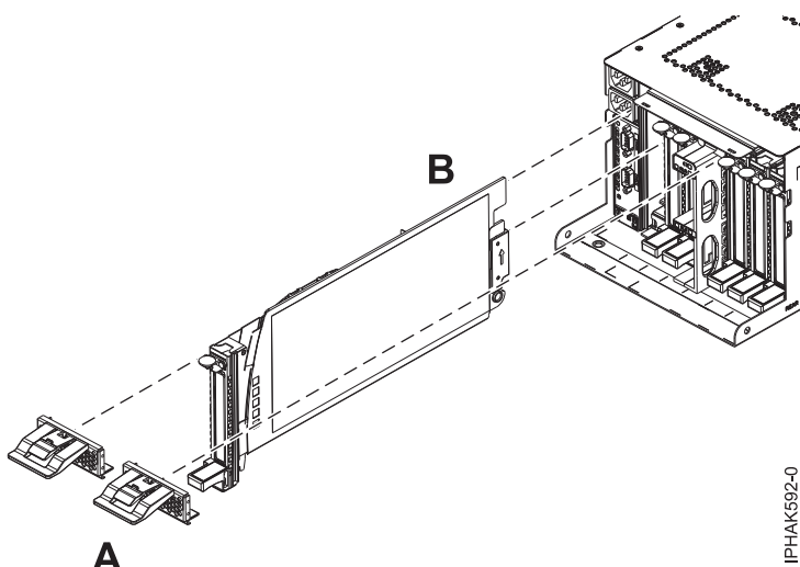
図 123. カセットの再取り付けおよび EMC グリルの取り付け
