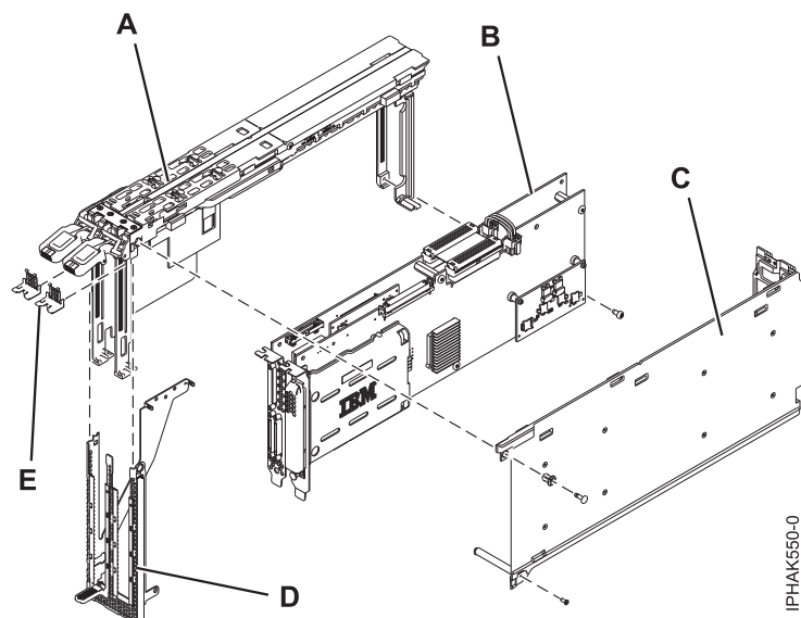
図 65. PCI-X ダブル幅 4 チャンネル Ultra320 SCSI RAID コントローラー、およびカセット・アセンブリーを構成する主要部品
