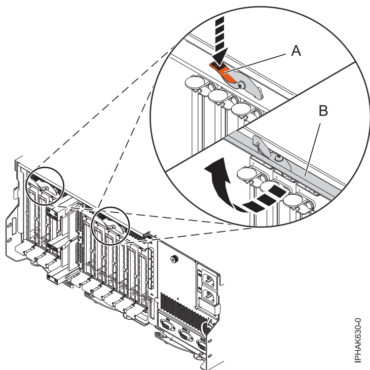
図 136. アクセス・ドアを開く
