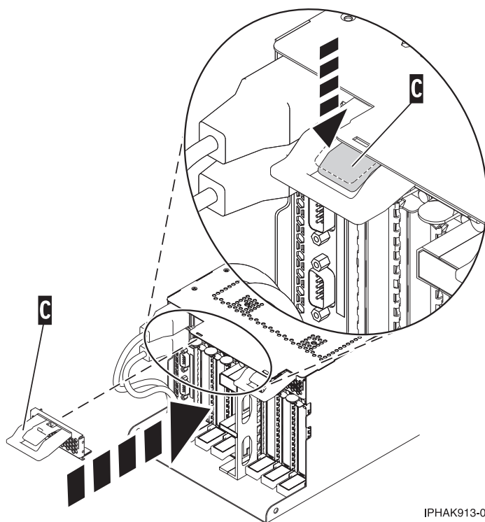
図 84. クローズ位置にある PCI アダプター EMC シールド
