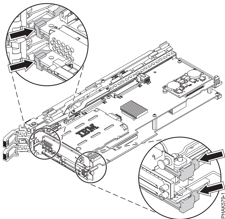
図 74. カセット・アセンブリーの隅の切り離し
