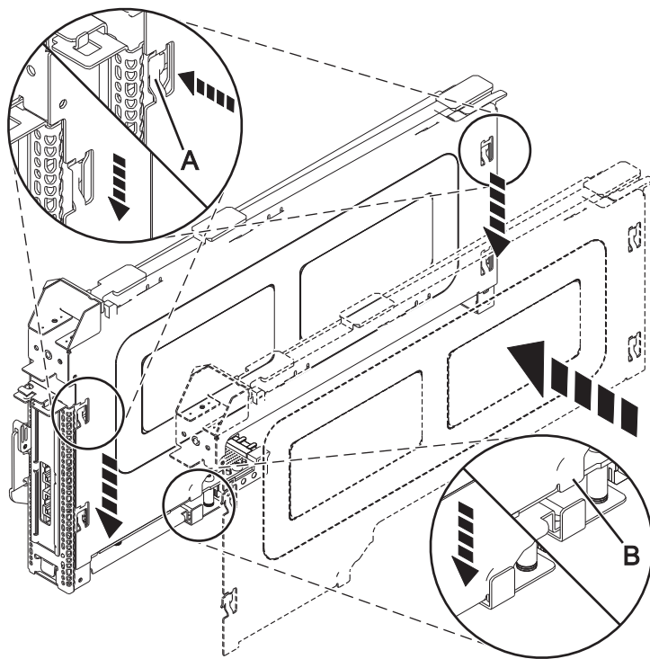
図 26. 元に戻された PCI アダプター・カセット・カバー
