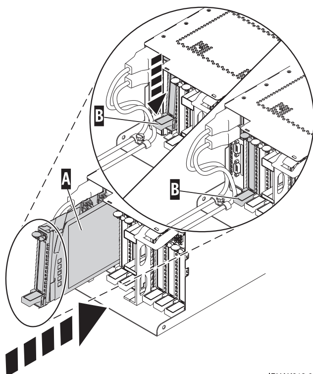
図 91. システム装置に取り付けられている PCI アダプター・カセット
