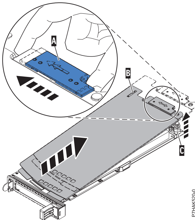
図 138. 取り外された PCI アダプター・カセット・カバー
