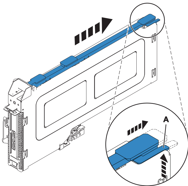
図 23. 取り外された PCI アダプター・カセット・ガイド・レール
