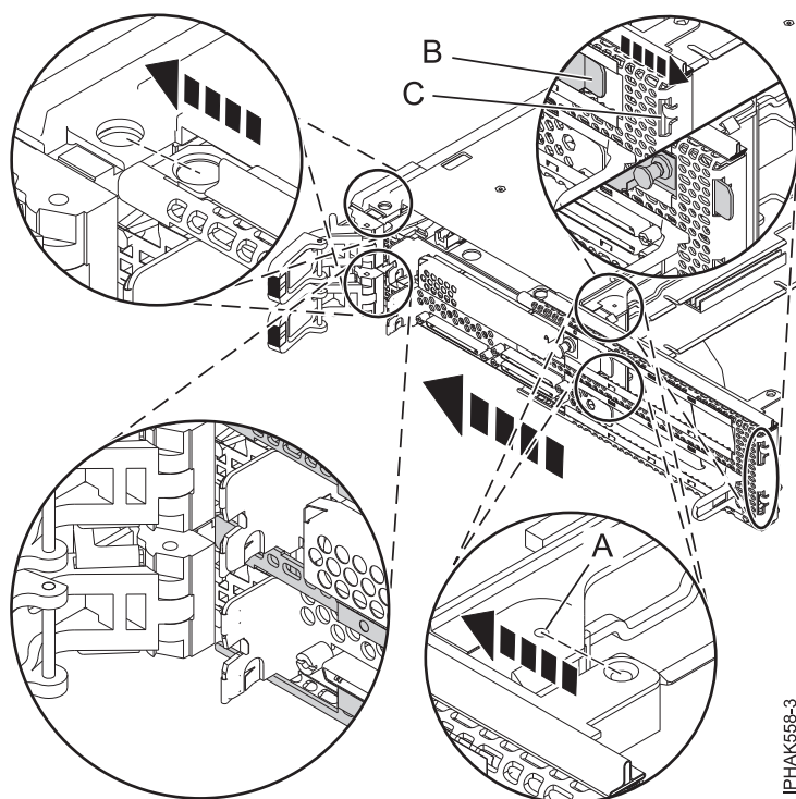
図 59. フェース・プレートの取り付け
