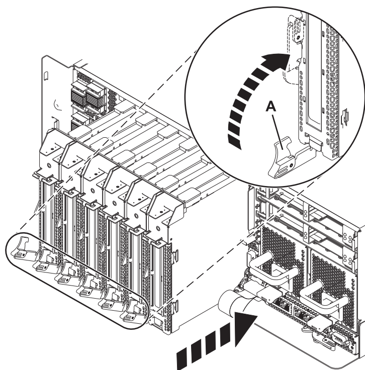
図 12. システム装置に取り付けられる PCI アダプター・カセット
