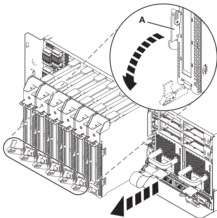
図9. システム装置から取り外された PCI アダプター・カセット
