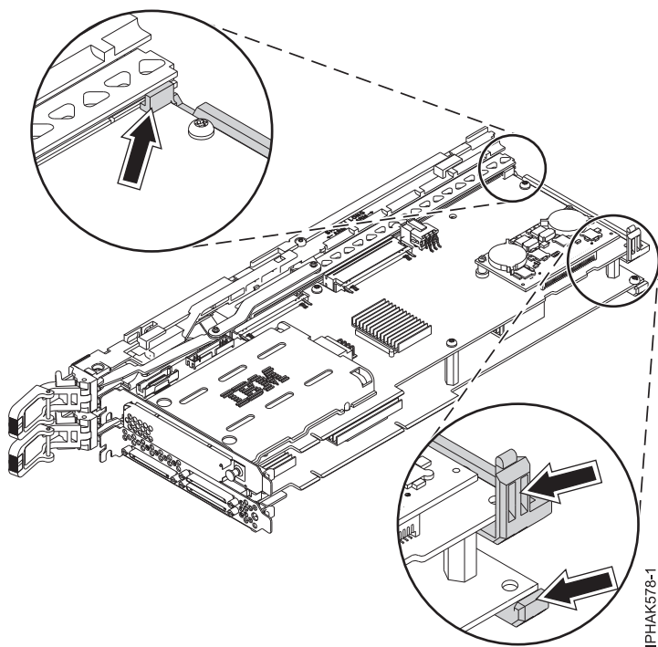
図 75. カセット・アセンブリーの後部アームの切り離し
