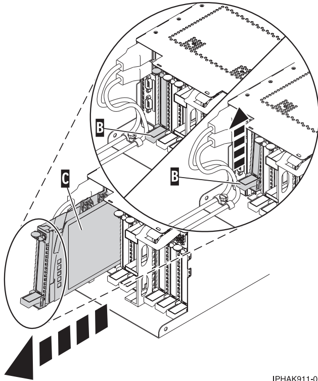
図 100. システム装置から取り外された PCI アダプター・カセット
