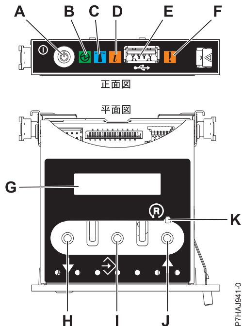
図 163. コントロール・パネル
