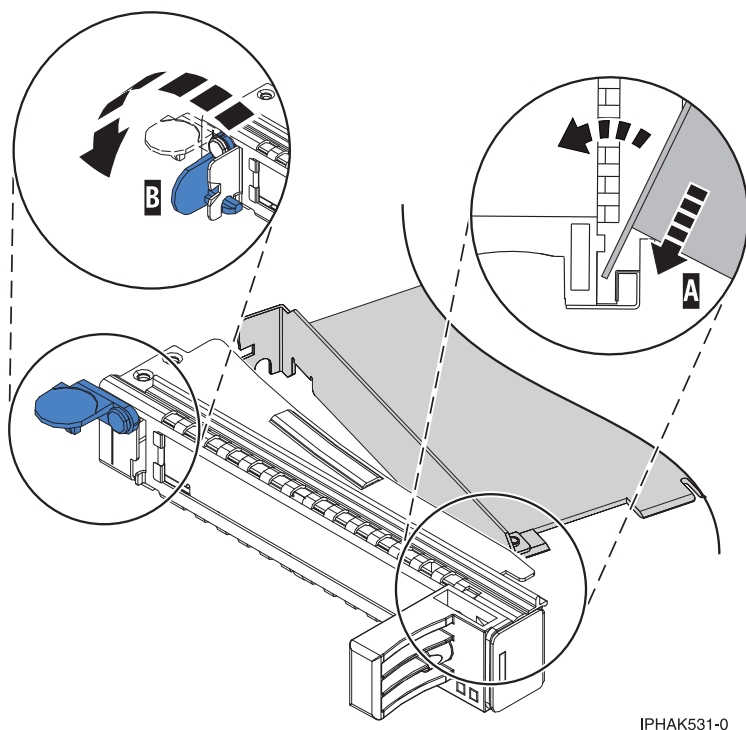
図 114. シングル幅 PCI アダプター・カセットから取り外されたアダプター
