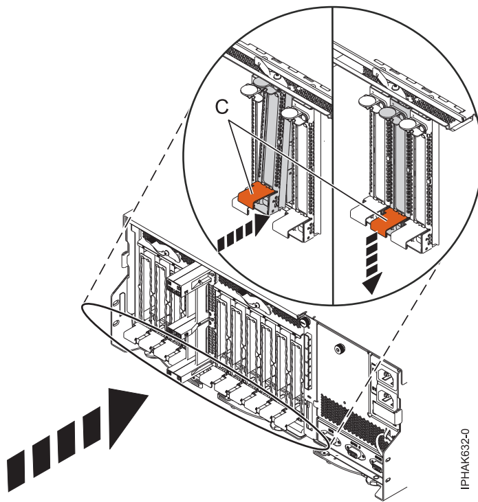
図 134. PCI アダプター・カセットの取り付け
