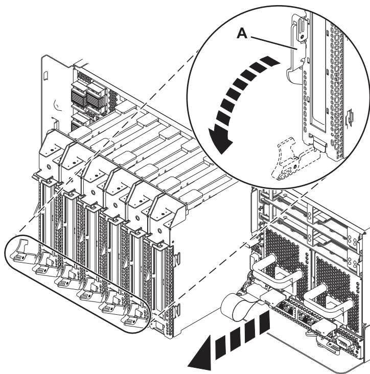
図6. システム装置から取り外された PCI アダプター・カセット
