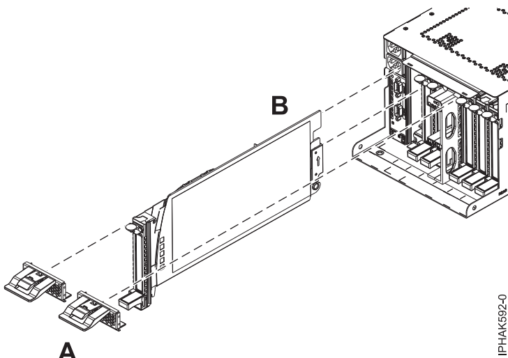
図 40. カセットの再取り付けおよび EMC グリルの取り付け
