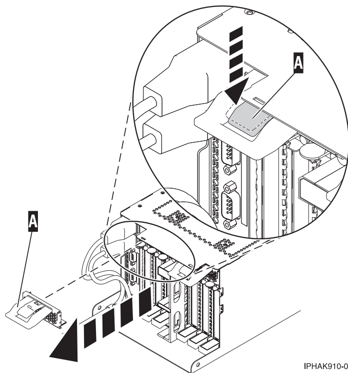
図 89. EMC シールドの取り外し
