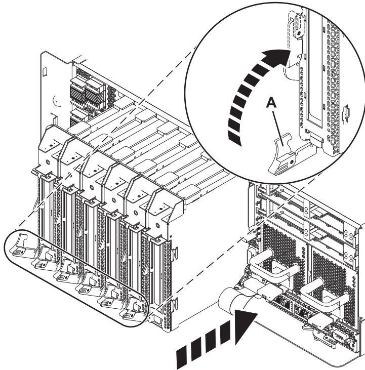
図 16. システム装置に取り付けられる PCI アダプター・カセット
