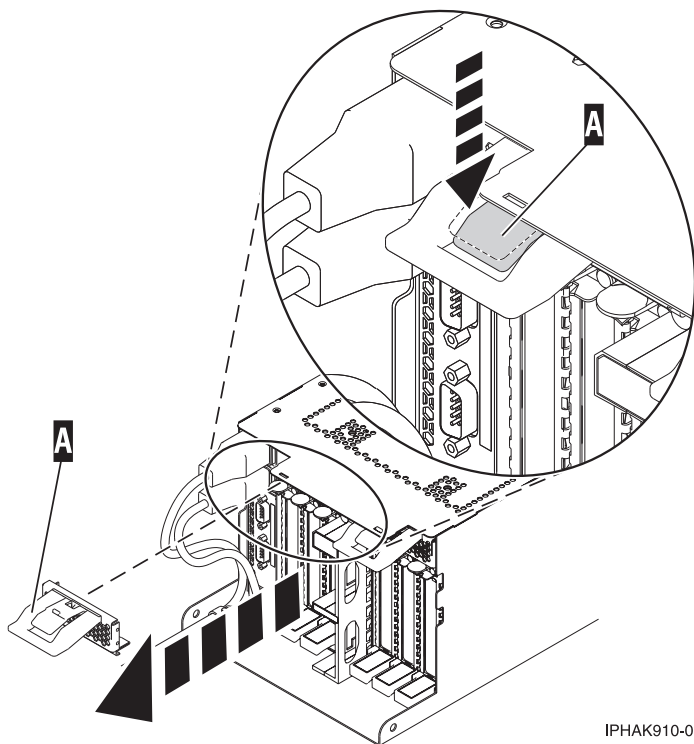
図 97. EMC シールドの取り外し
