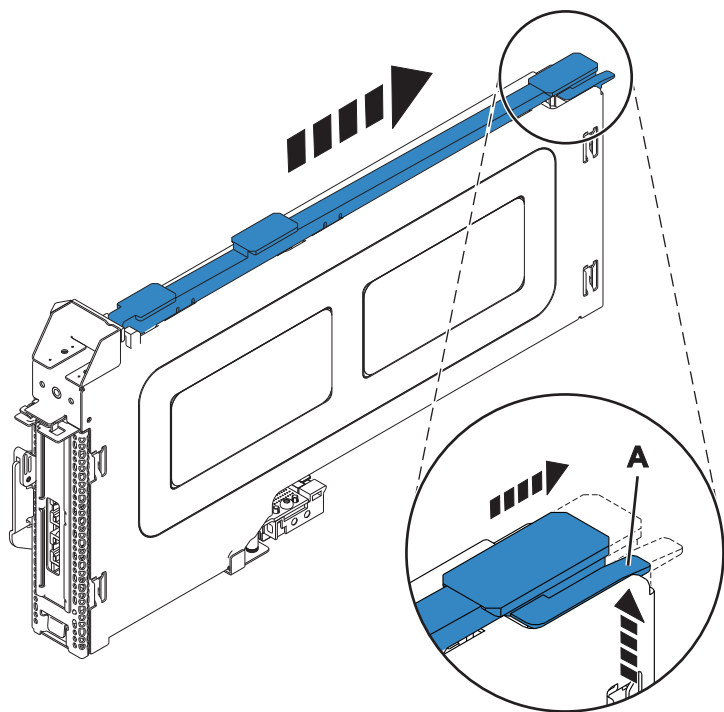
図 18. 取り外された PCI アダプター・カセット・ガイド・レール
