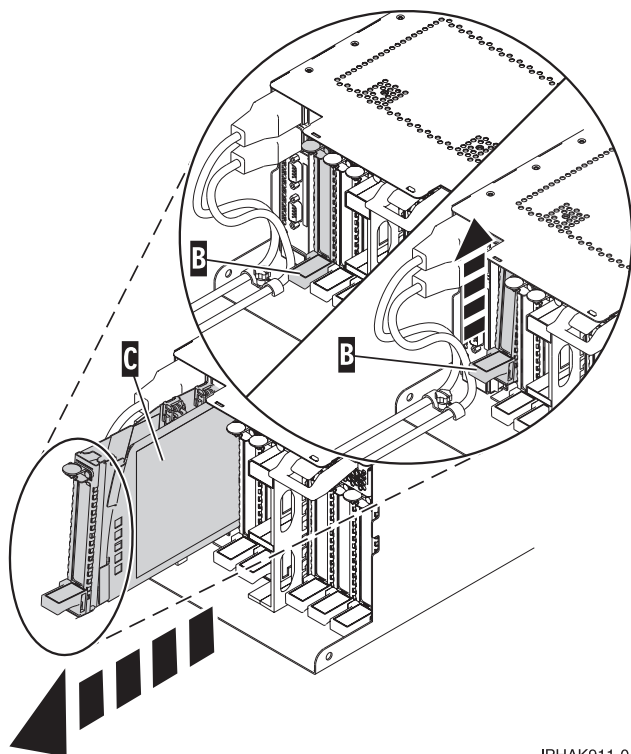
図 86. システム装置から取り外された PCI アダプター・カセット
