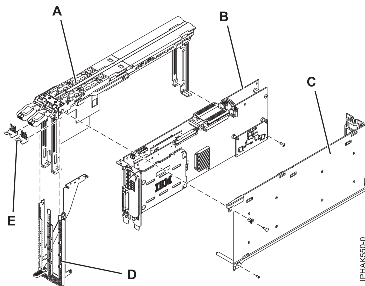
図 51. PCI-X ダブル幅 4 チャンネル Ultra320 SCSI RAID コントローラー、およびカセット・アセンブリーを構成する主要部品
