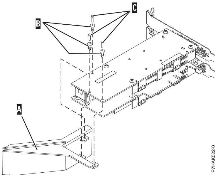
図 154. 新しい PCIe RAID および SSD SAS アダプターへの通気遮断壁の取り付け
