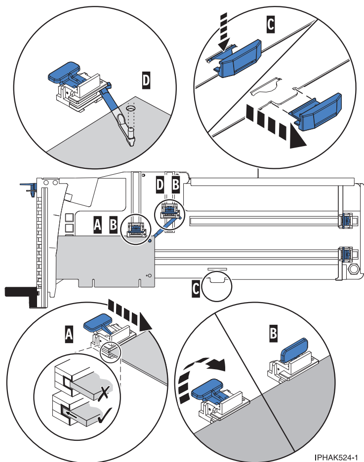
図 147. 所定位置に保持具およびフック・アームが付いた PCI アダプター・カセット内の小型 PCI アダプター
