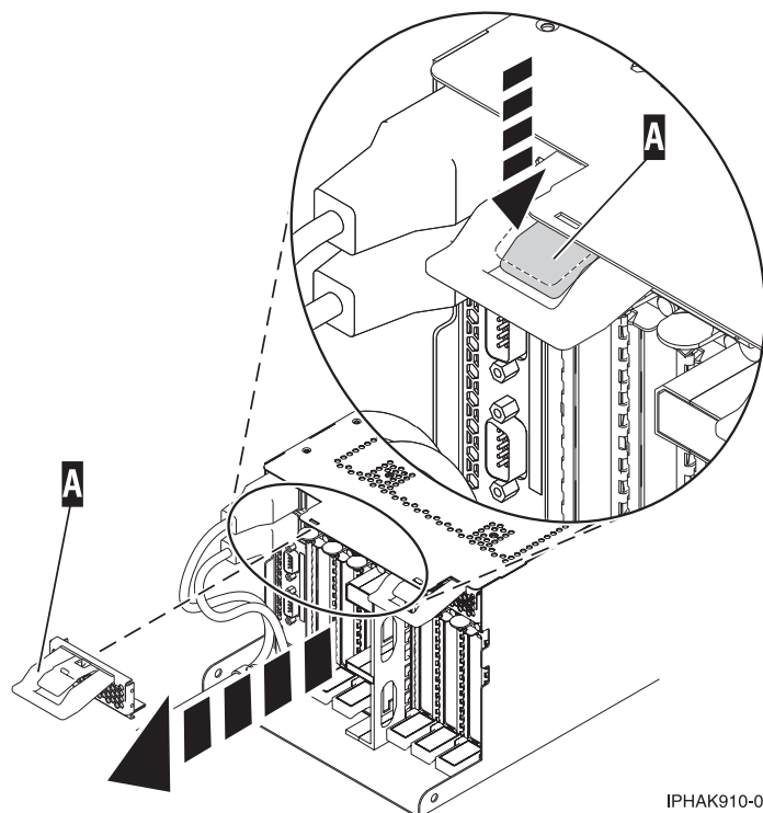
図 93. EMC シールドの取り外し
