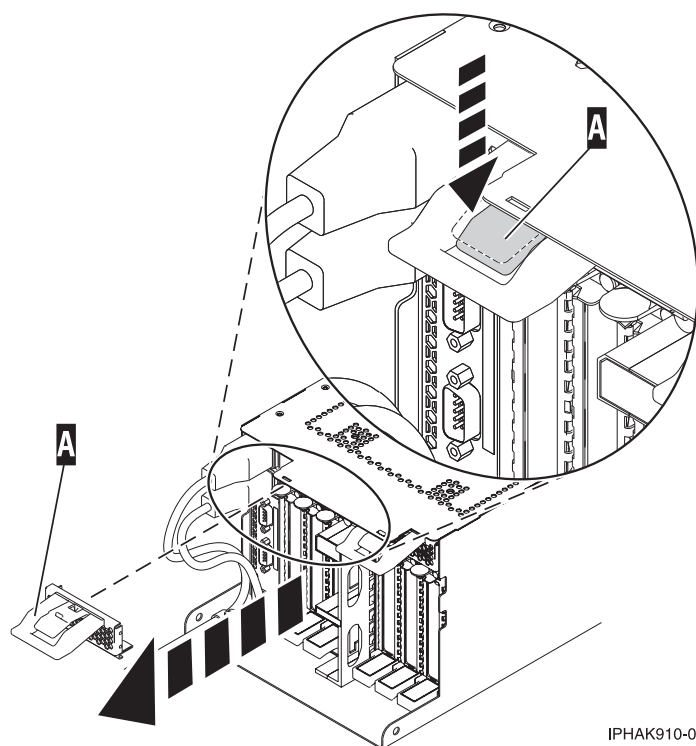
図 101. EMC シールドの取り外し
