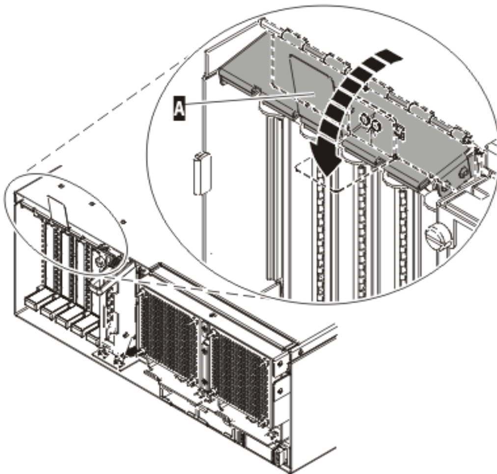
図 15. クローズ位置にある PCI アダプター EMC シールド
