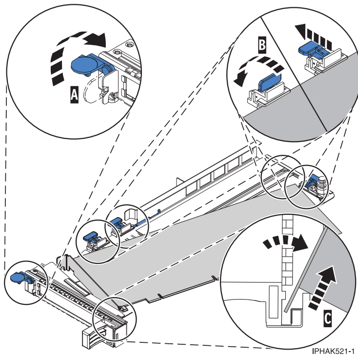
図 139. PCI アダプター・カセットから取り外されたアダプター
