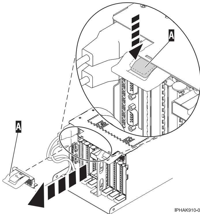
図 85. EMC シールドの取り外し
