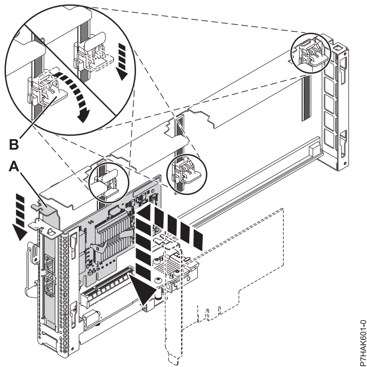
図 20. PCI アダプターのシングル幅のカセットに取り付けられたアダプター
