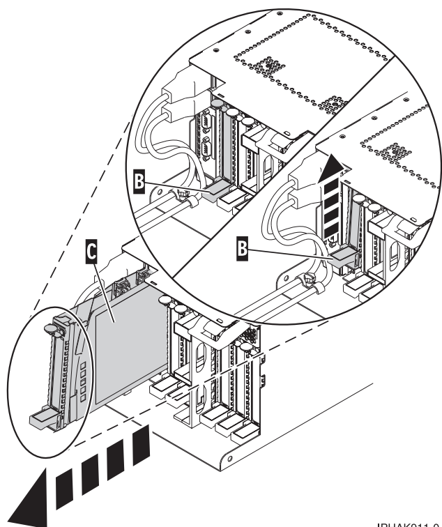
図 98. システム装置から取り外された PCI アダプター・カセット
