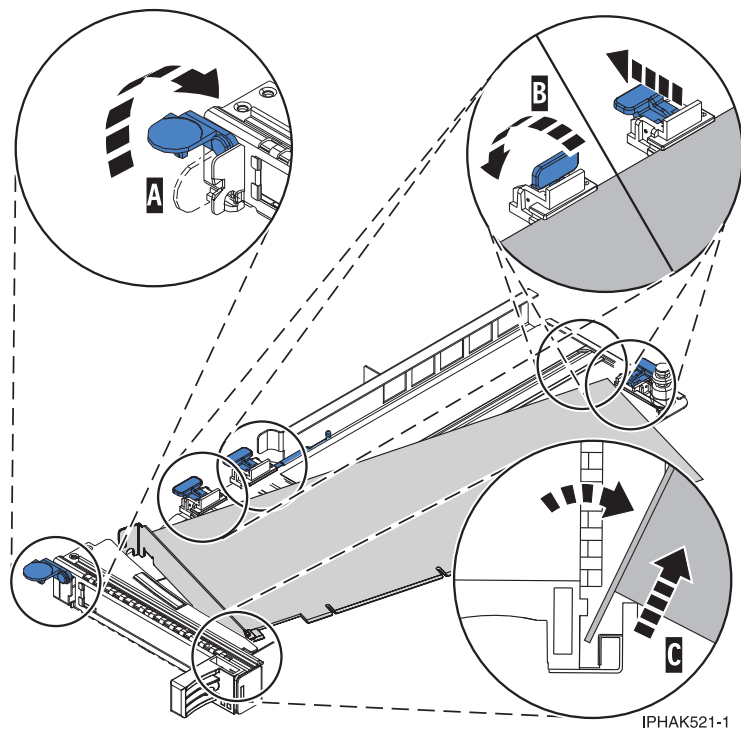
図 125. PCI アダプター・カセットから取り外されたアダプター
