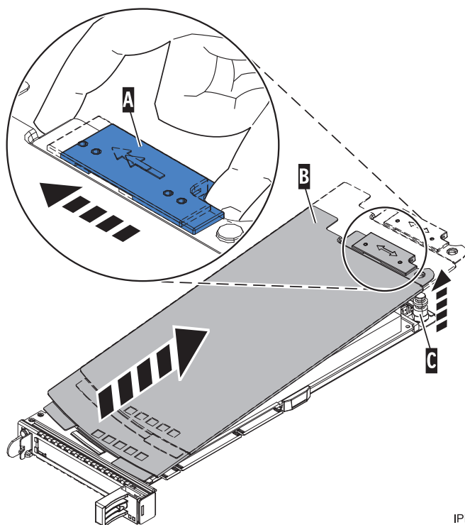
図 111. 取り外されたシングル幅 PCI アダプター・カセット・カバー
