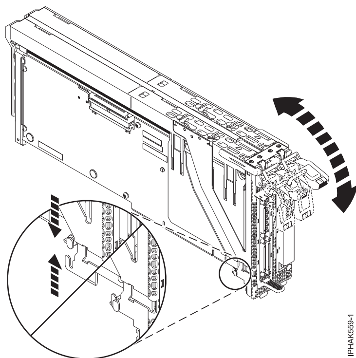
図 60. フェース・プレートの取り付け
