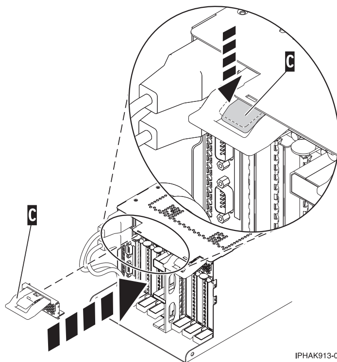
図 88. クローズ位置にある PCI アダプター EMC シールド
