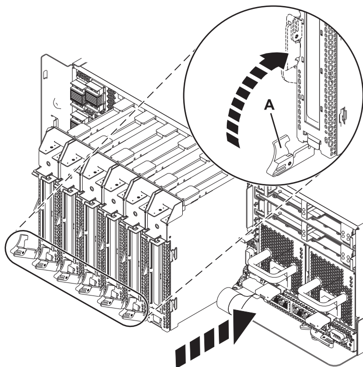
図7. システム装置に取り付けられる PCI アダプター・カセット
