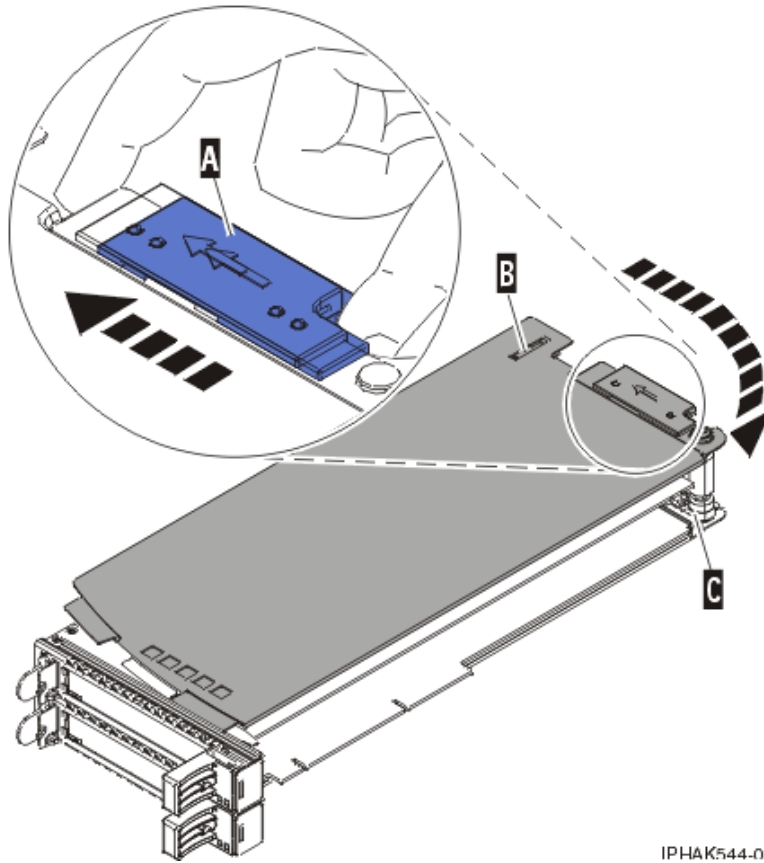
図 153. 取り外された PCI アダプター・カセット・カバー
