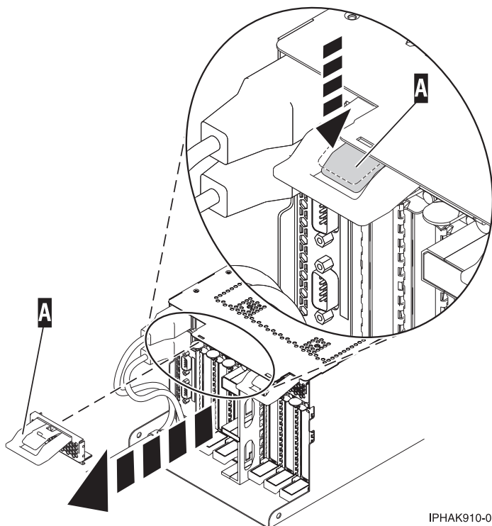
図 108. EMC シールドの取り外し
