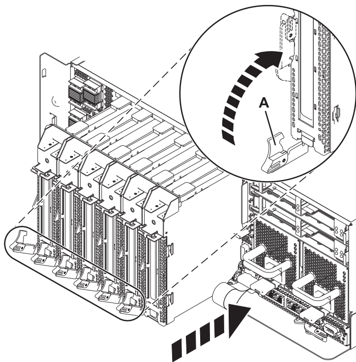
図 14. システム装置に取り付けられる PCI アダプター・カセット
