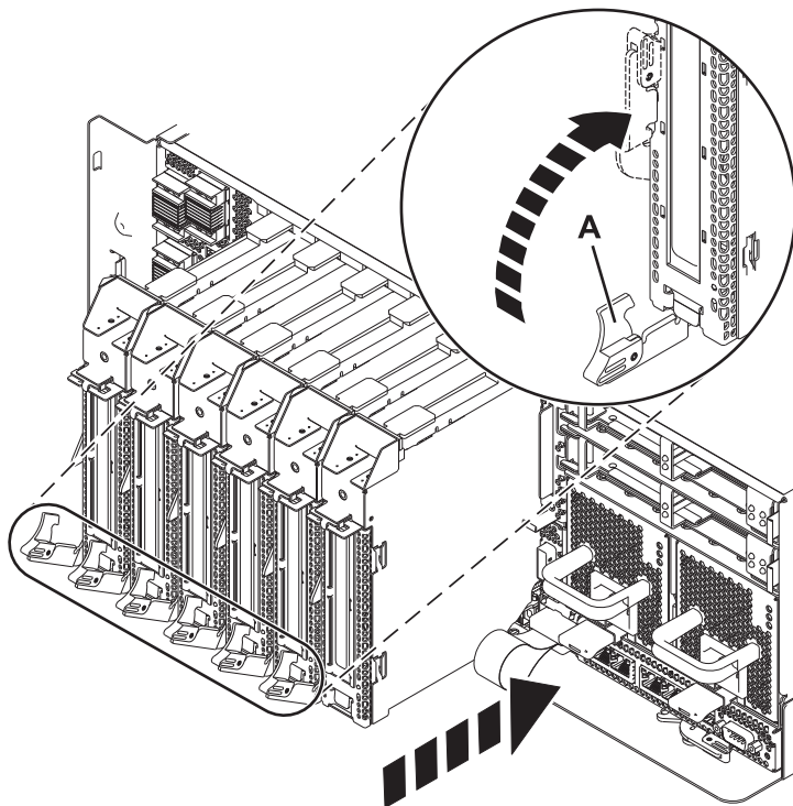
図 1. システム装置に取り付けられる PCI アダプター・カセット
