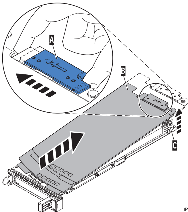
図 36. 取り外されたシングル幅 PCI アダプター・カセット・カバー
