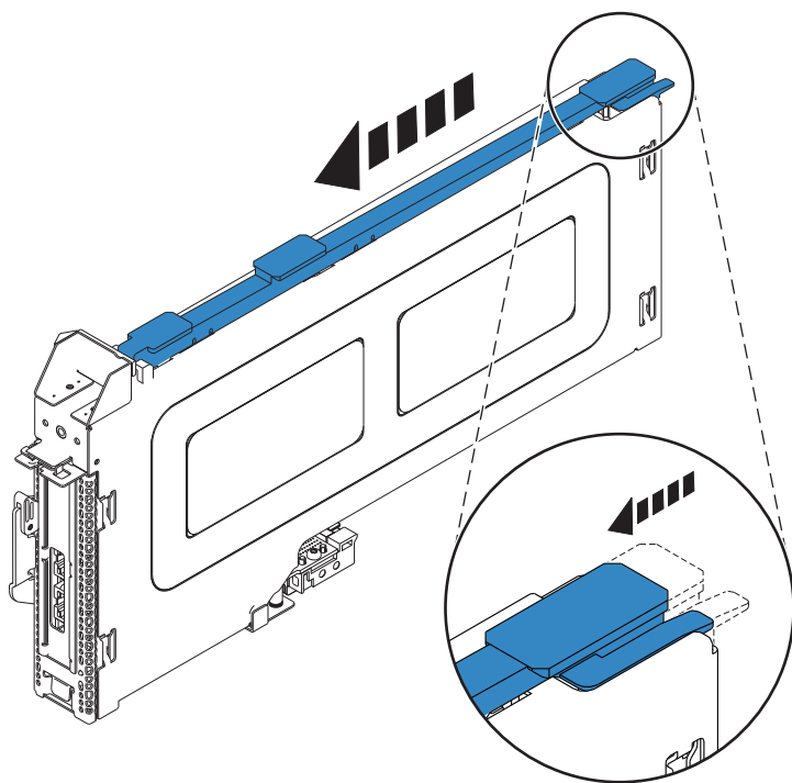
図 27. ロックされた PCI アダプター・カセット・ガイド・レール
