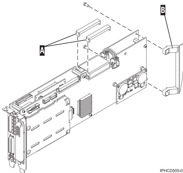
図 160. カセットに取り付けるためのアダプターの準備
