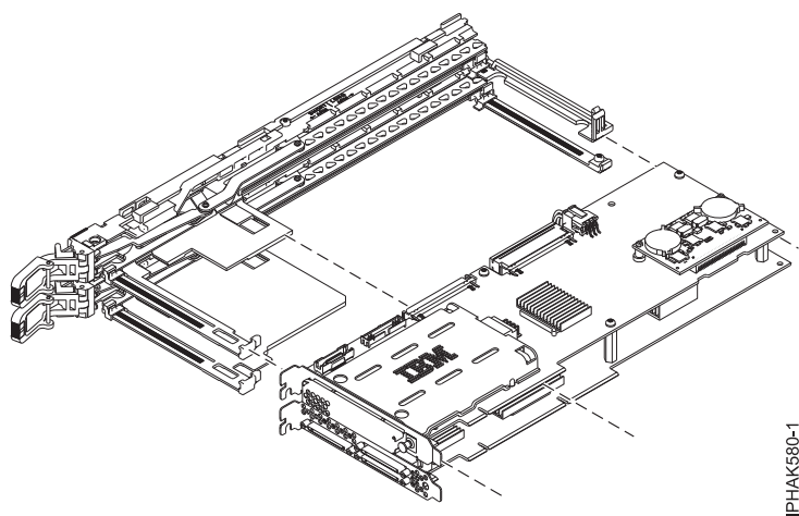
図 76. ダブル幅アダプターのカセット・アセンブリーからの引き出し
