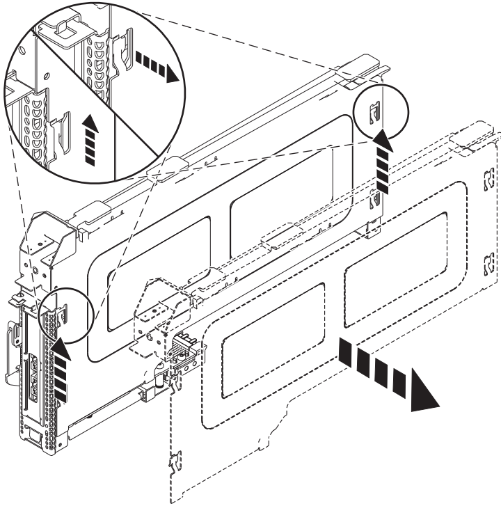
図 19. 取り外された PCI アダプター・カセット・カバー
