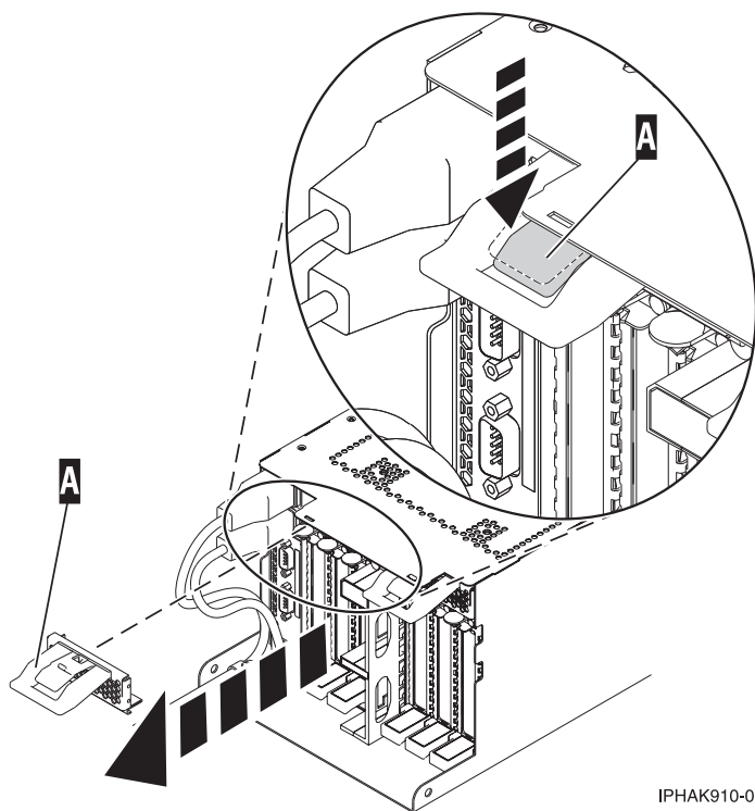
図 81. EMC シールドの取り外し
