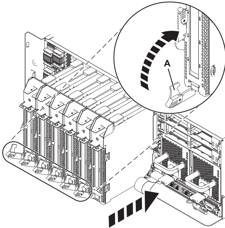
図 13. システム装置に取り付けられる PCI アダプター・カセット
