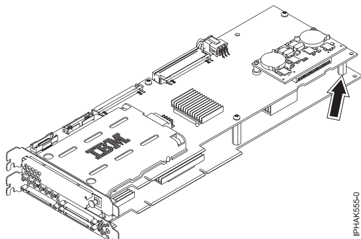
図 161. 支柱の取り外し
