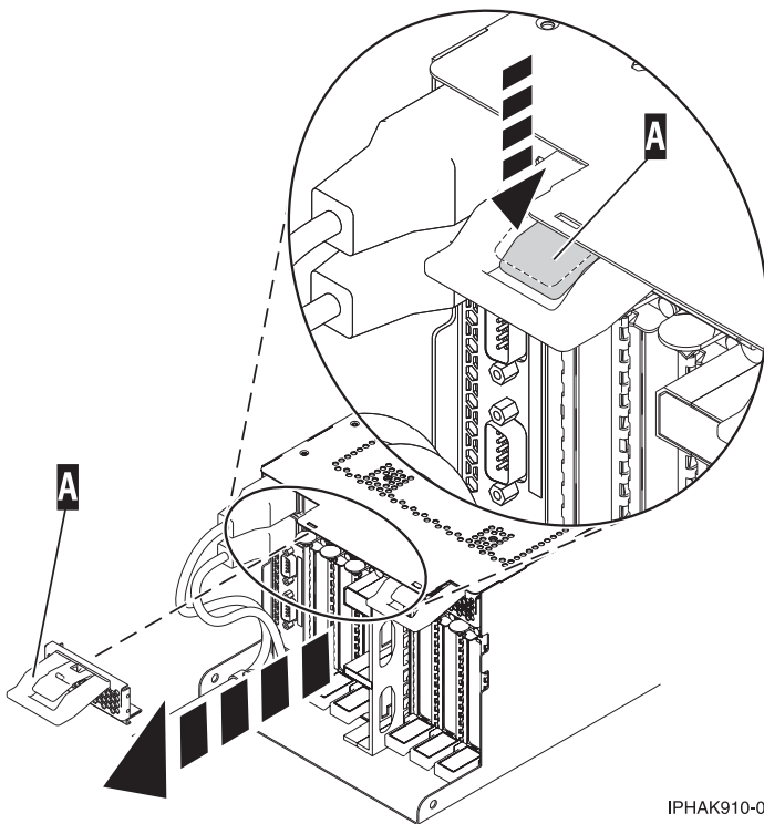
図 99. EMC シールドの取り外し
