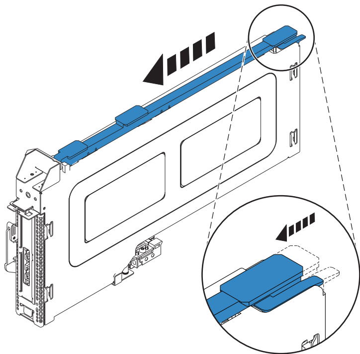
図 22. ロックされた PCI アダプター・カセット・ガイド・レール
