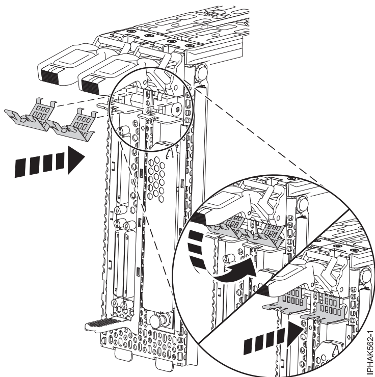
図 63. アセンブリー前面への 2 つのメタル・クリップの挿入
