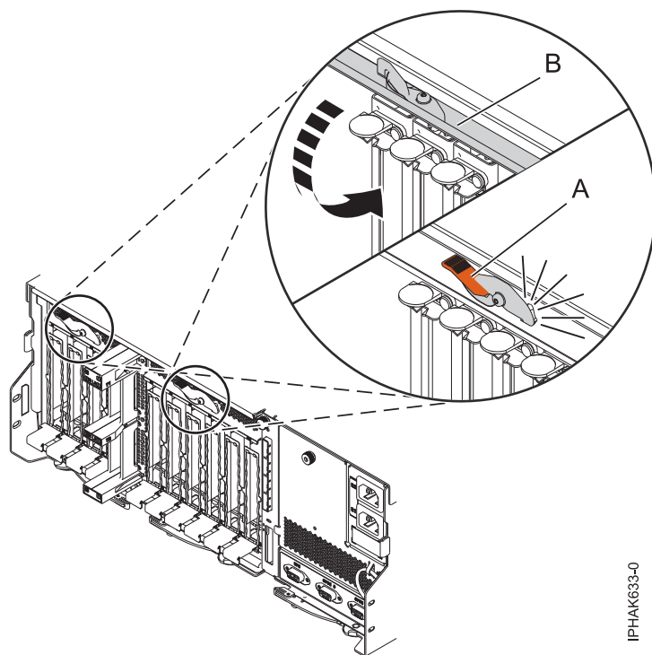
図 135. アクセス・ドアを閉じる
