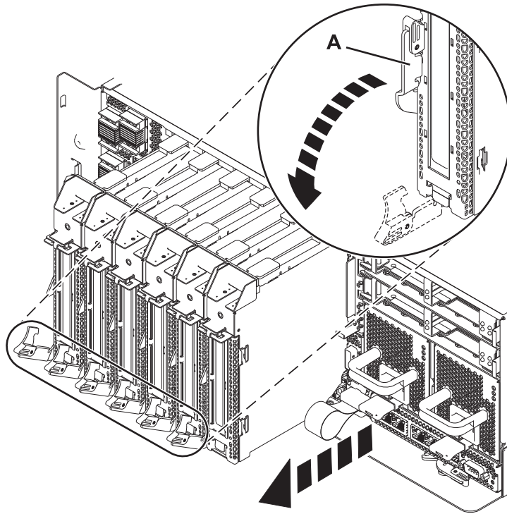
図 11. システム装置から取り外された PCI アダプター・カセット
