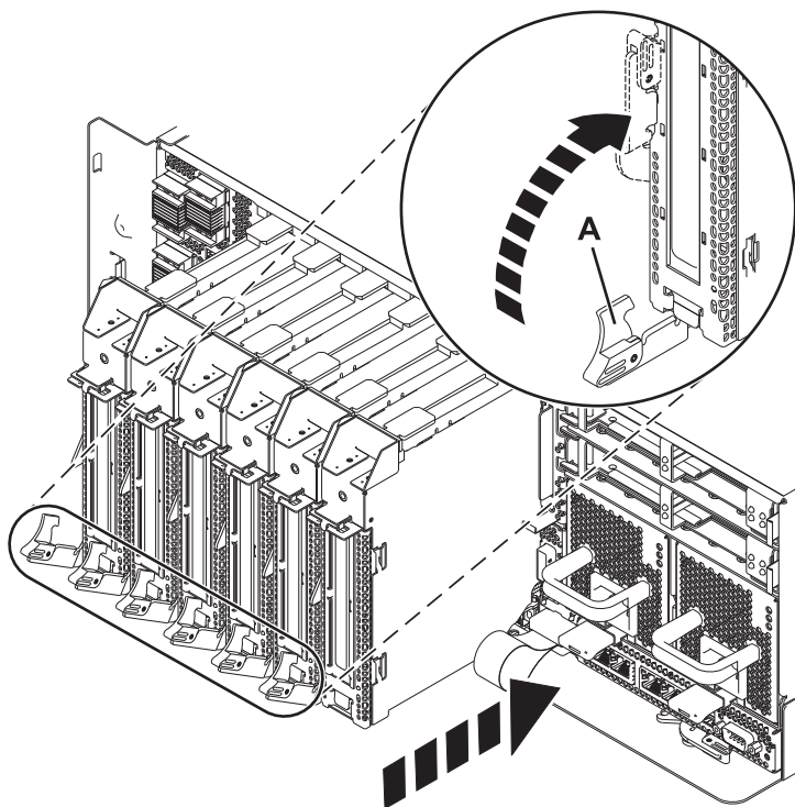
図2. システム装置に取り付けられる PCI アダプター・カセット
