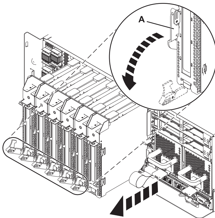
図8. システム装置から取り外された PCI アダプター・カセット
