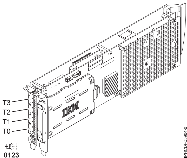
図 162. PCI-X DDR 1.5GB キャッシュ SAS RAID アダプター
