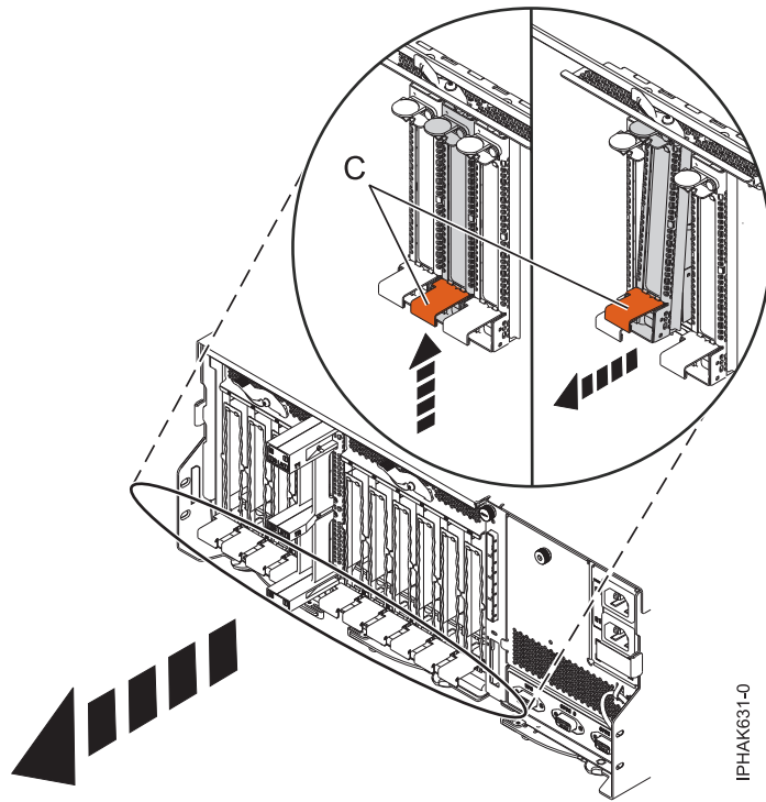
図 137. PCI アダプター・カセットの取り外し
