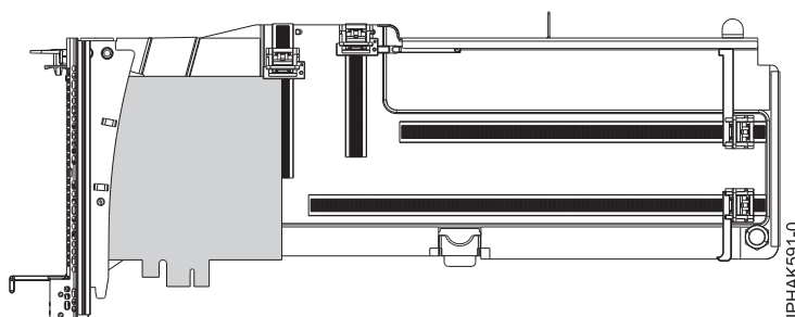
図 38. カセット内のアダプターの側面図
