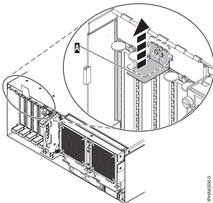
図4. EMC シールドを持ち上げる
