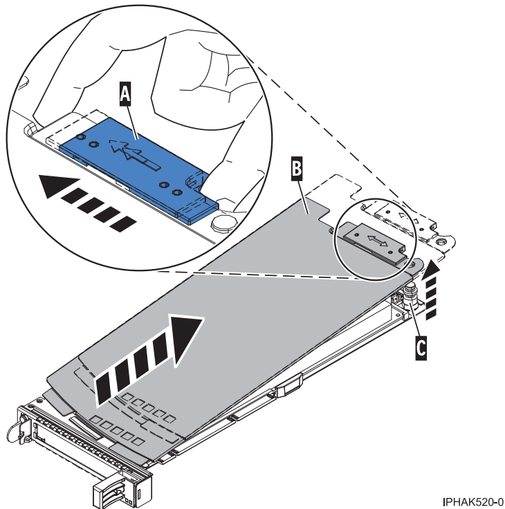
図 124. 取り外された PCI アダプター・カセット・カバー
