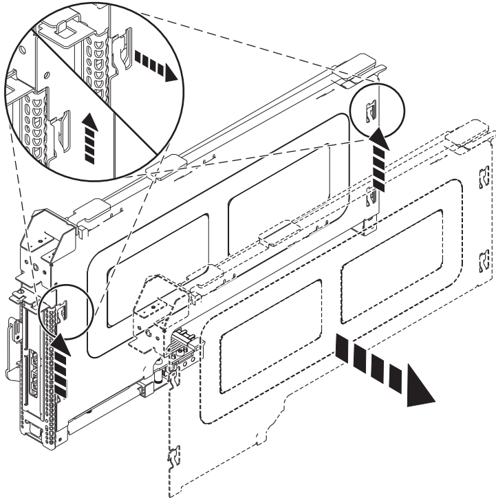
図 24. 取り外された PCI アダプター・カセット・カバー
