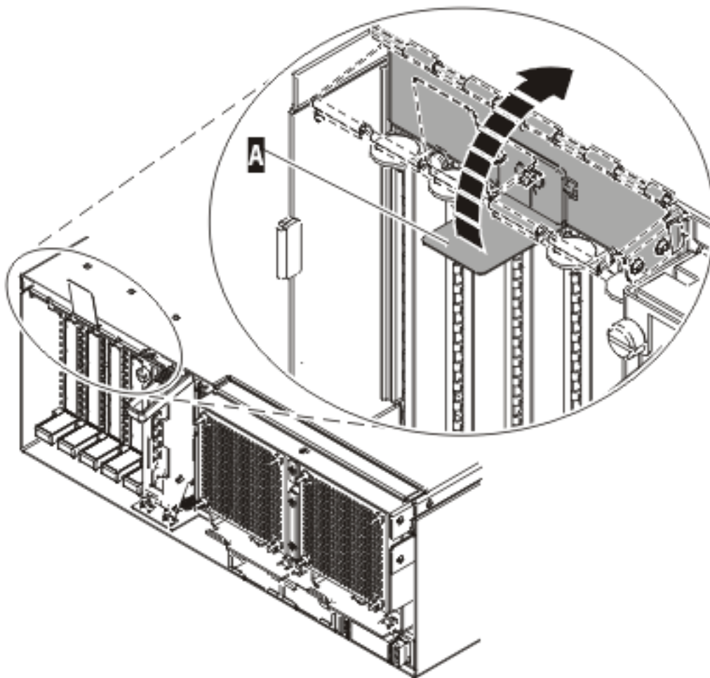
図5. EMC シールドを回転してオープン位置にする
