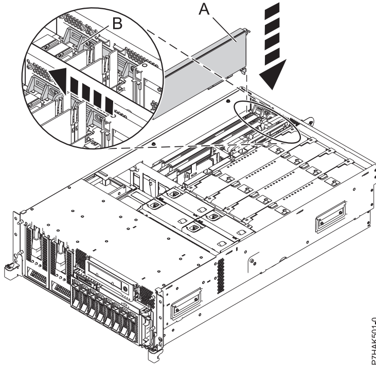
図 8. ラック・マウント型システム装置で取り替えられた PCI アダプター
