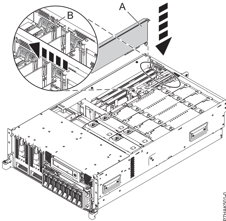
図 15. ラック・マウント型システム装置で取り替えられた PCI アダプター
