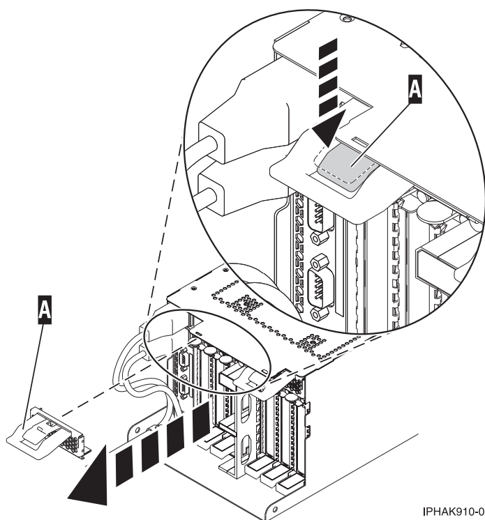
図 65. EMC シールドの取り外し
