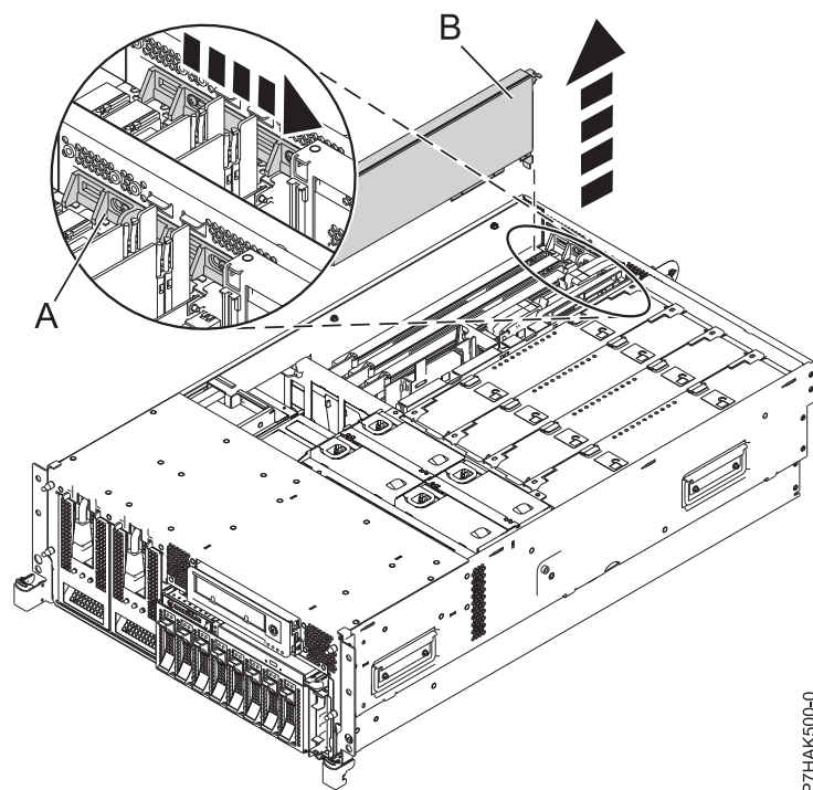
図 20. ラック・マウント型システム装置から取り外された PCI アダプターまたはフィラー・プレート
