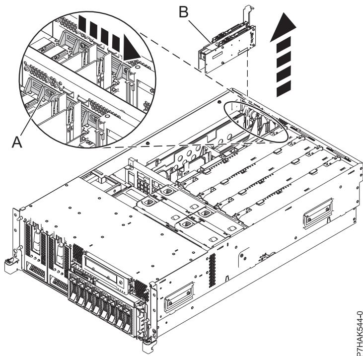
図 28. ラック・マウント型システム装置から取り外された PCI RAID および SSD SAS アダプター
