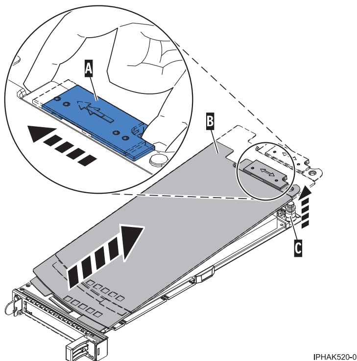
図 88. 取り外された PCI アダプター・カセット・カバー
