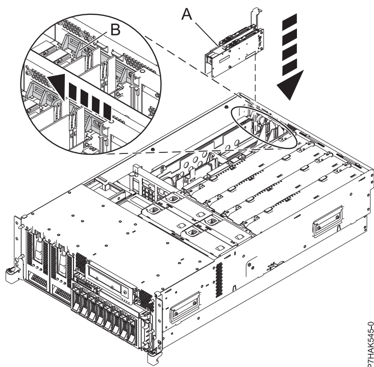
図 30. ラック・マウント型システム装置で取り替えられた PCI RAID および SSD SAS アダプター
