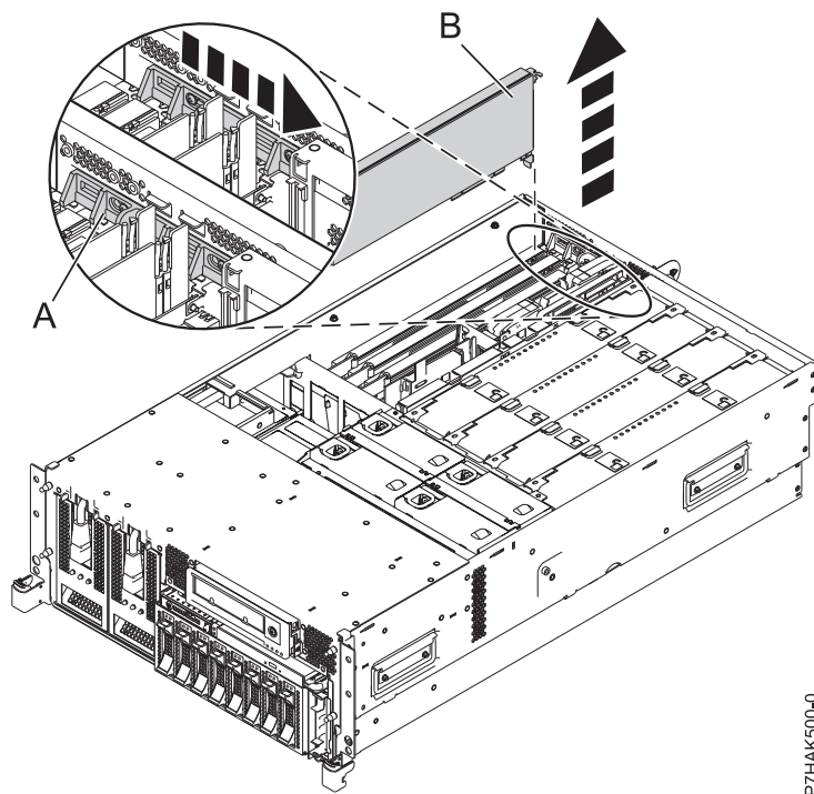
図 38. ラック・マウント型システム装置から取り外された PCI アダプターまたはフィラー・プレート
