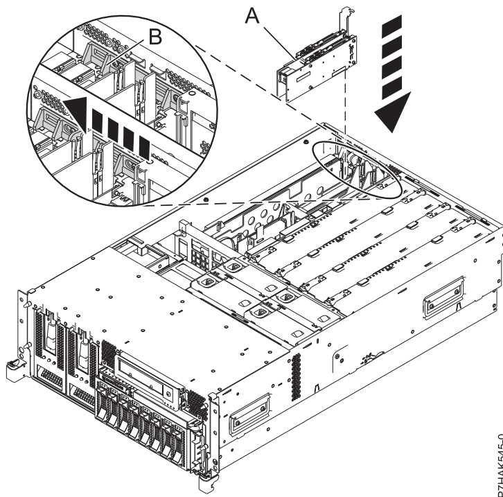
図 34. ラック・マウント型システム装置で取り替えられた PCI RAID および SSD SAS アダプター
