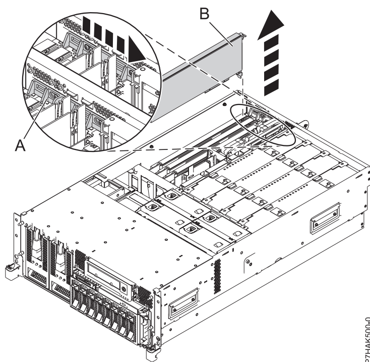
図 10. ラック・マウント型システム装置から取り外された PCI アダプターまたはフィラー・プレート
