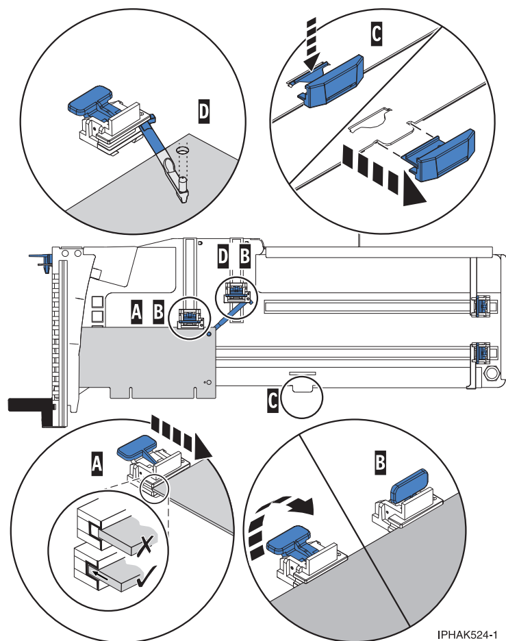
図 111. 所定位置に保持具およびフック・アームが付いた PCI アダプター・カセット内の小型 PCI アダプター
