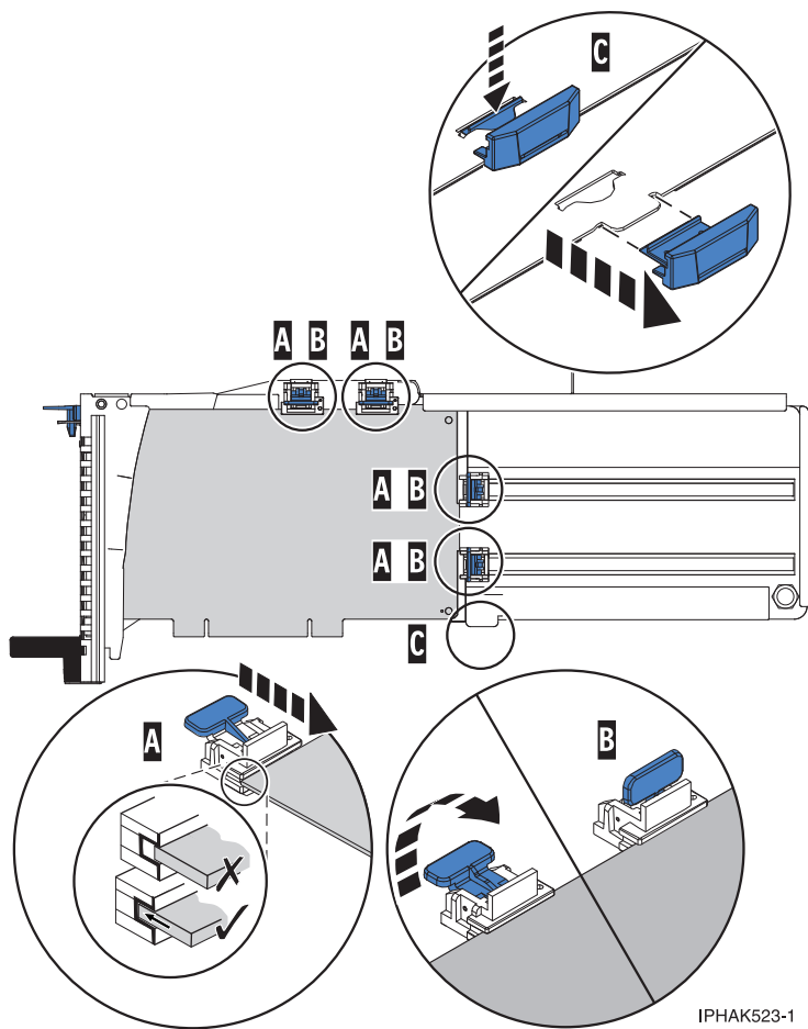
図 80. 所定位置に保持具が付いた PCI アダプター・カセット内の中型 PCI アダプター
