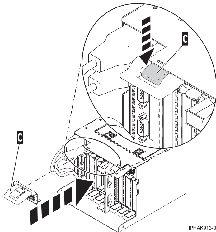
図 44. クローズ位置にある PCI アダプター EMC シールド
