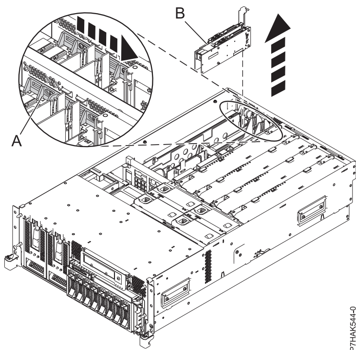
図 26. ラック・マウント型システム装置から取り外された PCI RAID および SSD SAS アダプター
