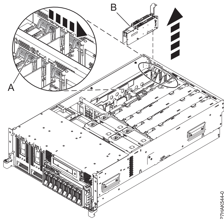
図 29. ラック・マウント型システム装置から取り外された PCI RAID および SSD SAS アダプター
