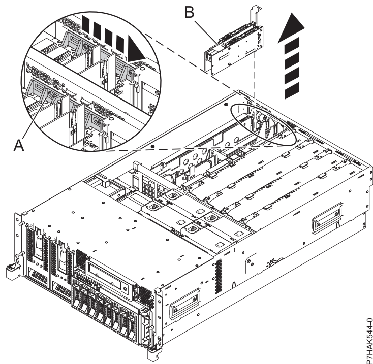
図 27. ラック・マウント型システム装置から取り外された PCI RAID および SSD SAS アダプター
