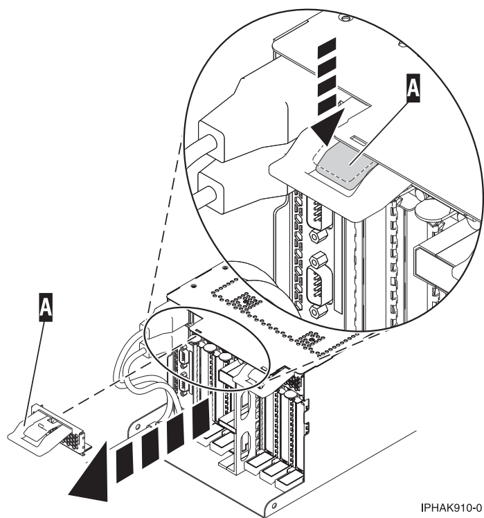
図 63. EMC シールドの取り外し
