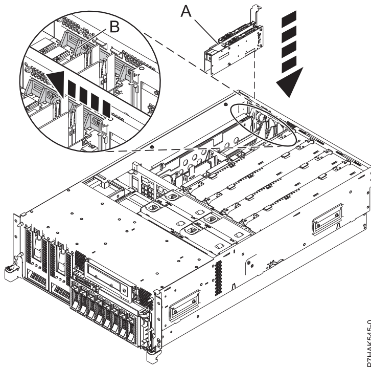
図 25. ラック・マウント型システム装置で取り替えられた PCI RAID および SSD SAS アダプター
