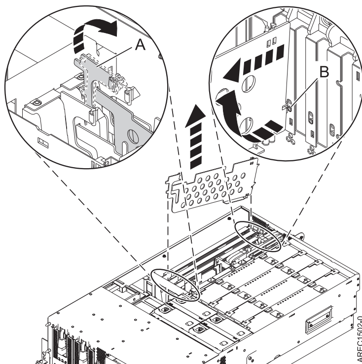
図 36. システム装置から取り外された PCI アダプター・セパレーター
