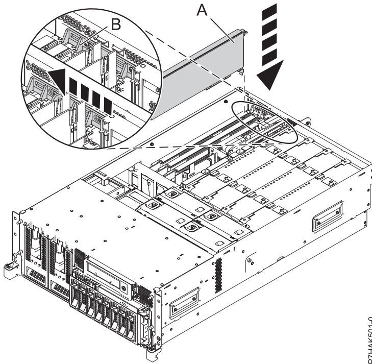
図4. ラック・マウント型システム装置で取り替えられた PCI アダプター
