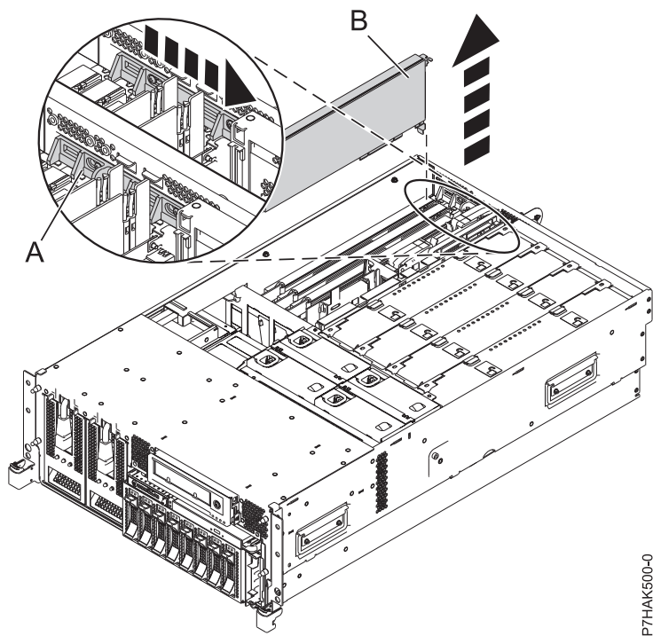
図 35. ラック・マウント型システム装置から取り外された PCI アダプターまたはフィラー・プレート
