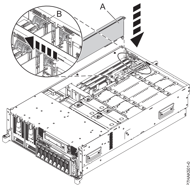
図 13. ラック・マウント型システム装置で取り替えられた PCI アダプター
