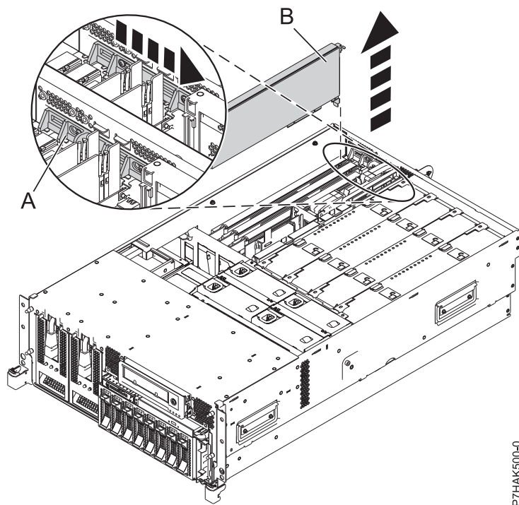
図9. ラック・マウント型システム装置から取り外された PCI アダプターまたはフィラー・プレート
