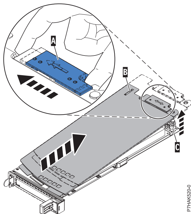
図 102. 取り外された PCI アダプター・カセット・カバー
