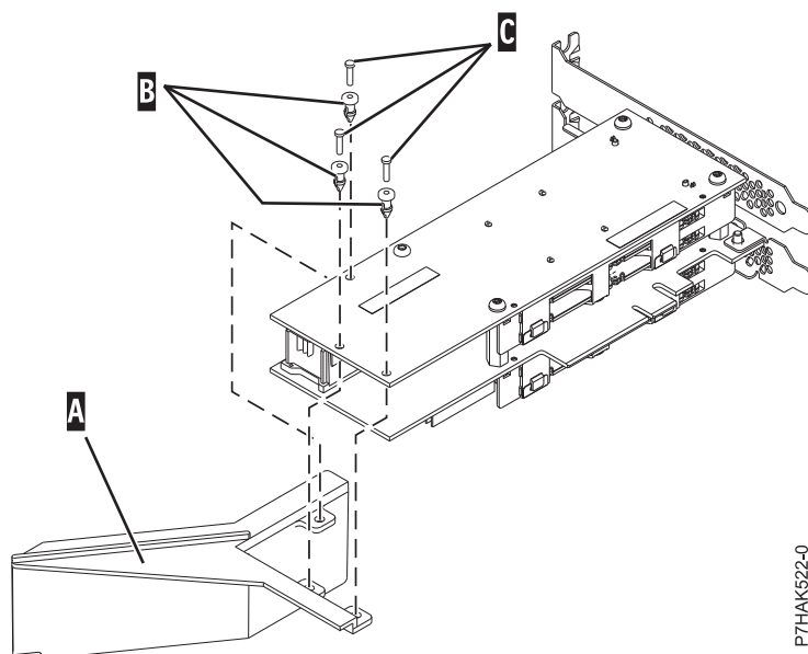
図 118. 新しい PCIe RAID および SSD SAS アダプターへの通気遮断壁の取り付け
