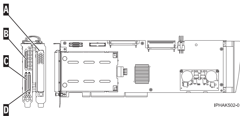
図 123. アダプター
