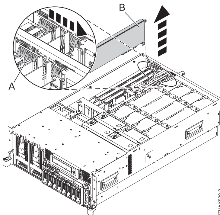
図1. ラック・マウント型システム装置から取り外された PCI アダプターまたはフィラー・プレート
