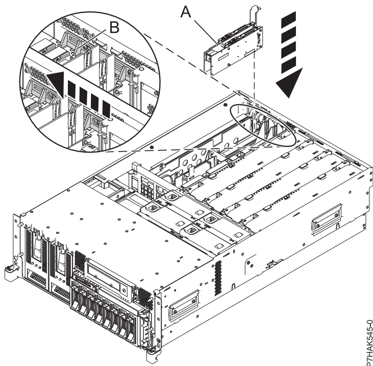
図 21. ラック・マウント型システム装置で取り替えられた PCI RAID および SSD SAS アダプター
