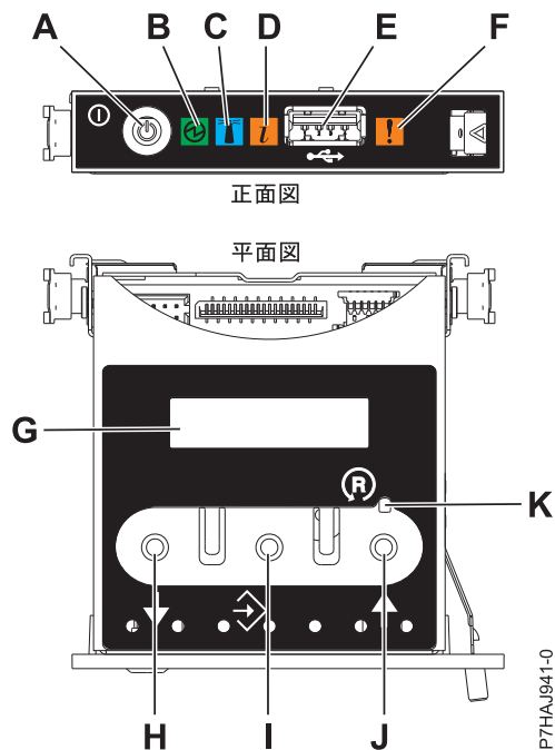
図 128. コントロール・パネル
