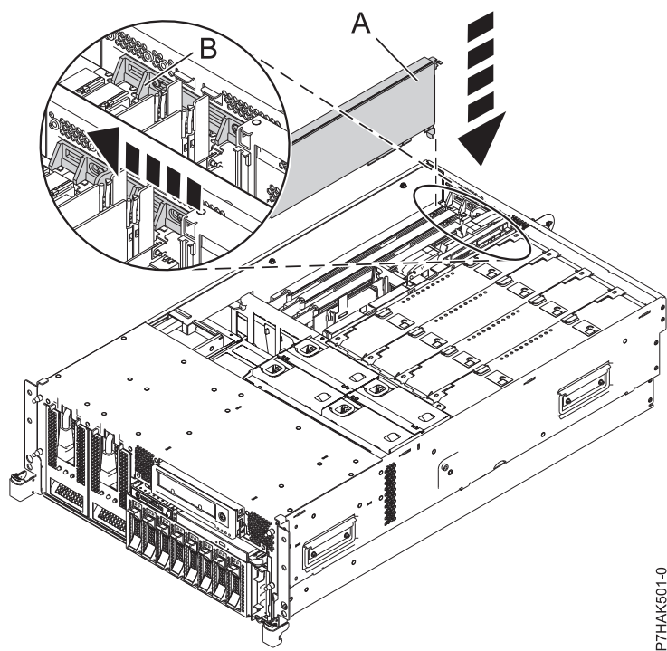
図 40. ラック・マウント型システム装置で取り替えられた PCI アダプター
