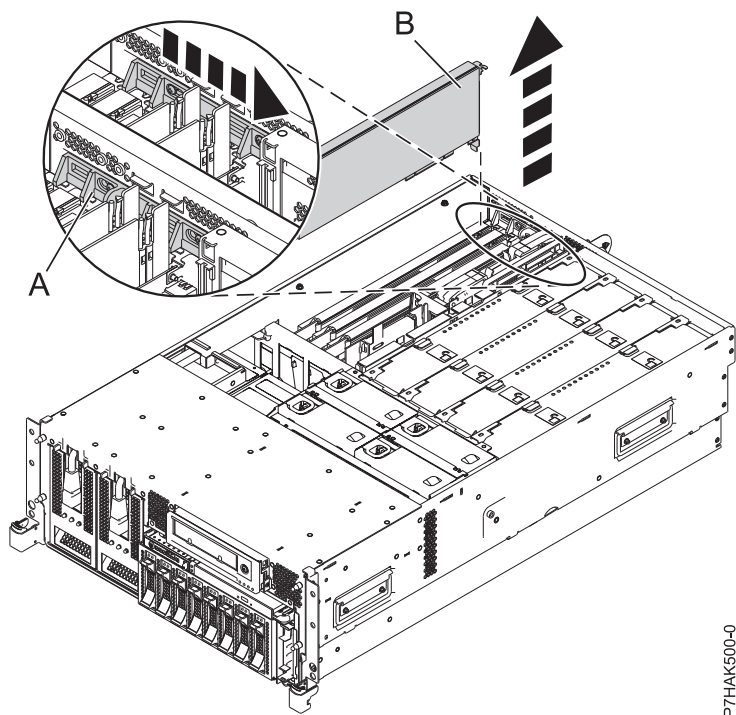
図 22. ラック・マウント型システム装置から取り外された PCI アダプターまたはフィラー・プレート
