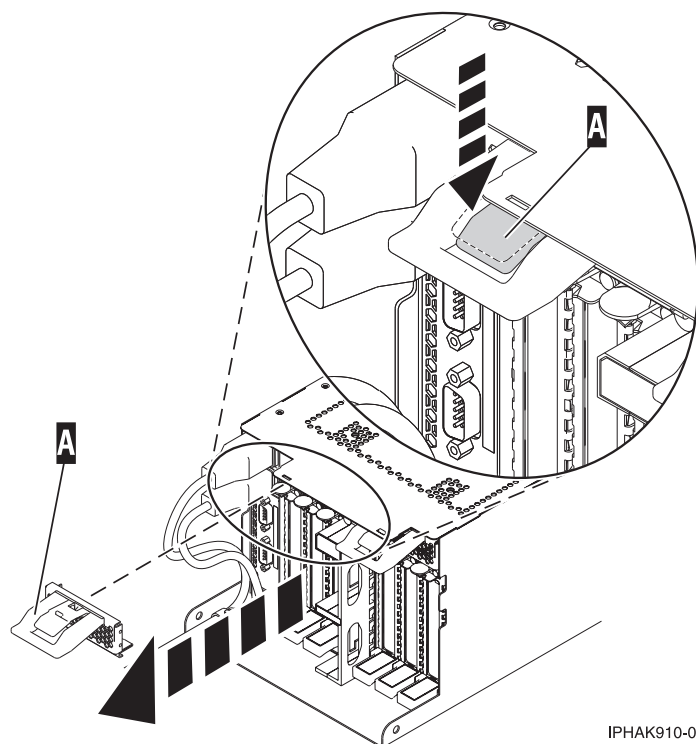
図 59. EMC シールドの取り外し
