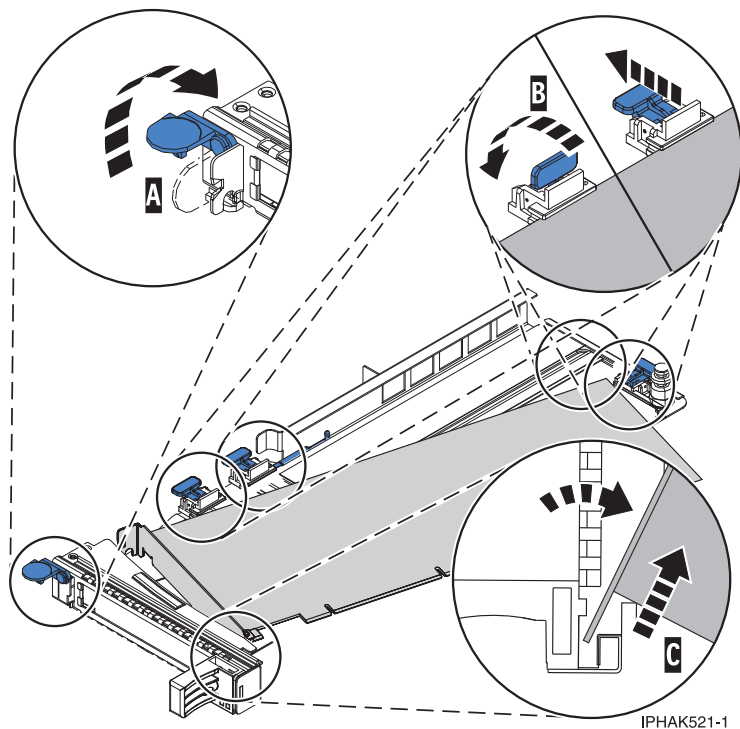
図 89. PCI アダプター・カセットから取り外されたアダプター
