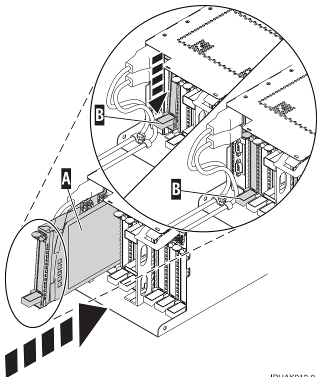
図 43. システム装置に取り付けられている PCI アダプター・カセット
