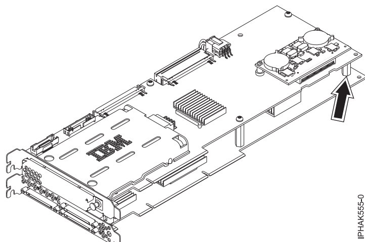
図 125. 支柱の取り外し
