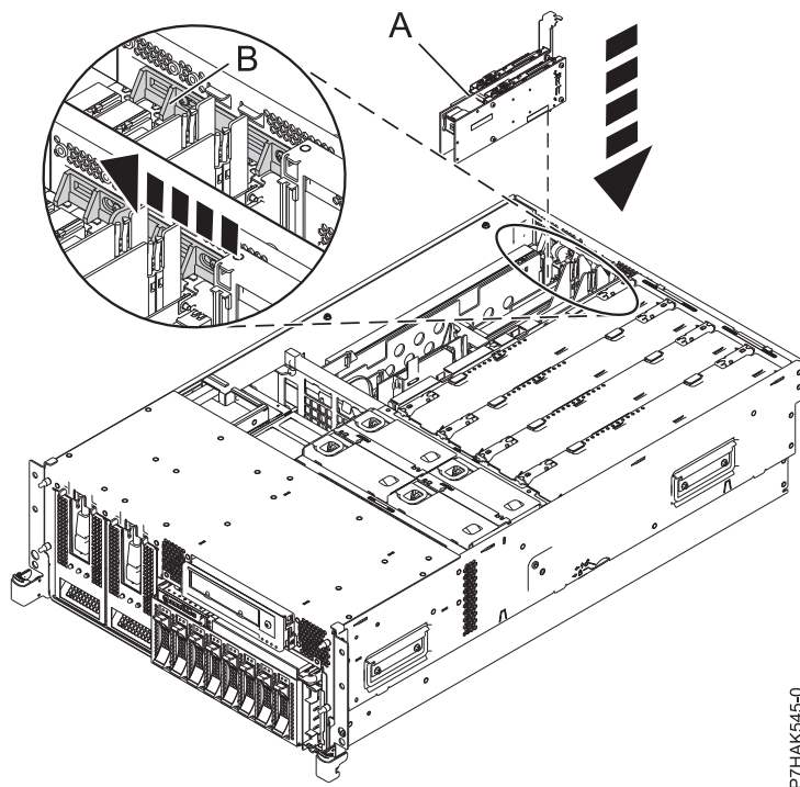
図 19. ラック・マウント型システム装置で取り替えられた PCIe RAID および SSD SAS アダプター
