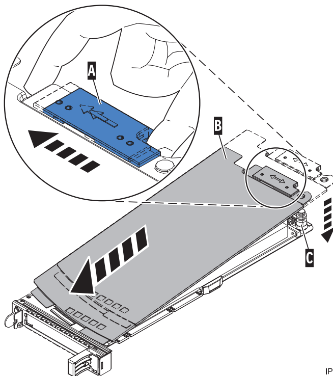
図 90. 元に戻された PCI アダプター・カセット・カバー
