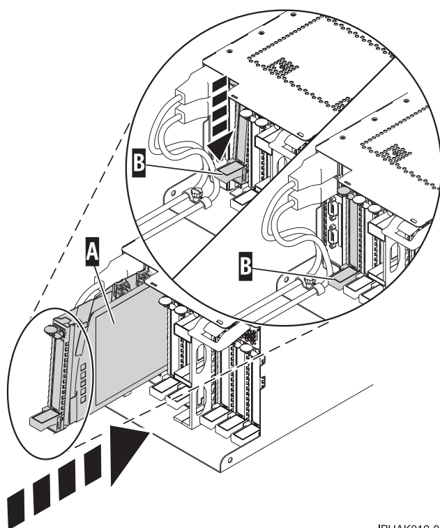
図 55. システム装置に取り付けられている PCI アダプター・カセット
