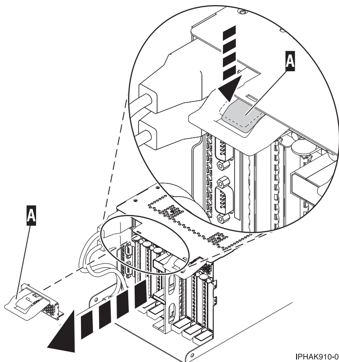
図 57. EMC シールドの取り外し
