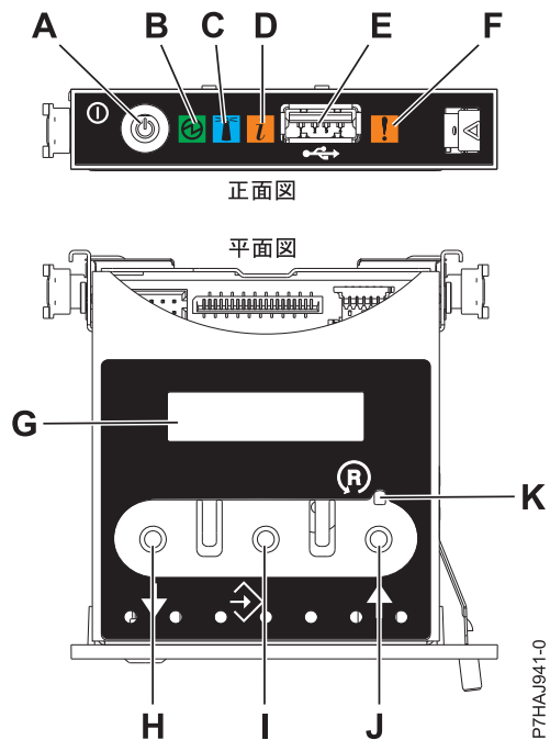
図 127. コントロール・パネル
