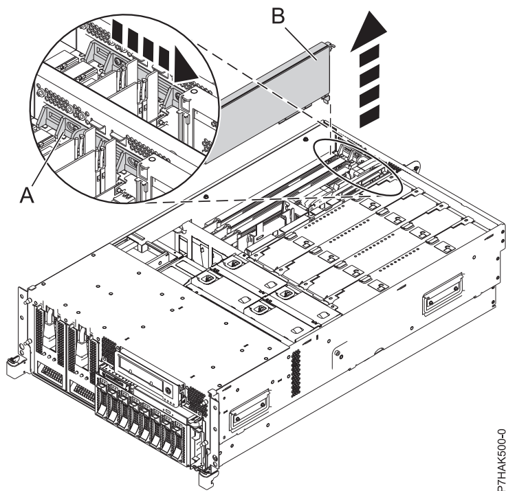
図 18. ラック・マウント型システム装置から取り外された PCI アダプターまたはフィラー・プレート
