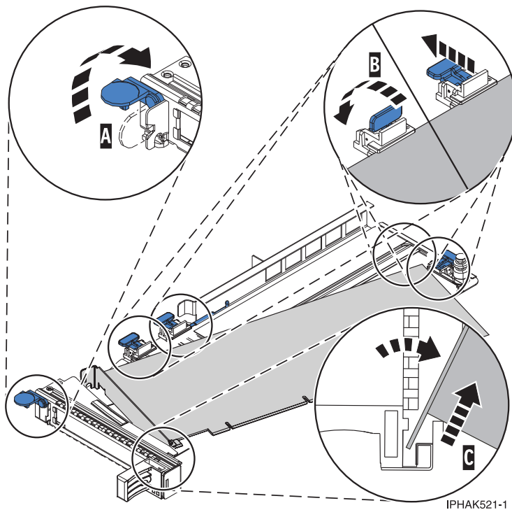
図 103. PCI アダプター・カセットから取り外されたアダプター
