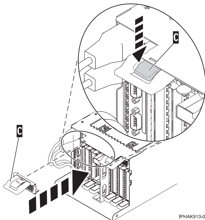
図 56. クローズ位置にある PCI アダプター EMC シールド
