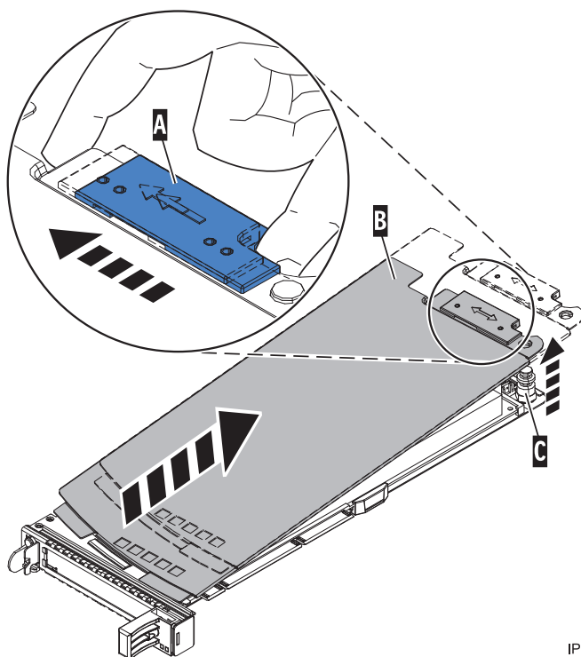
図 105. 取り外されたシングル幅 PCI アダプター・カセット・カバー
