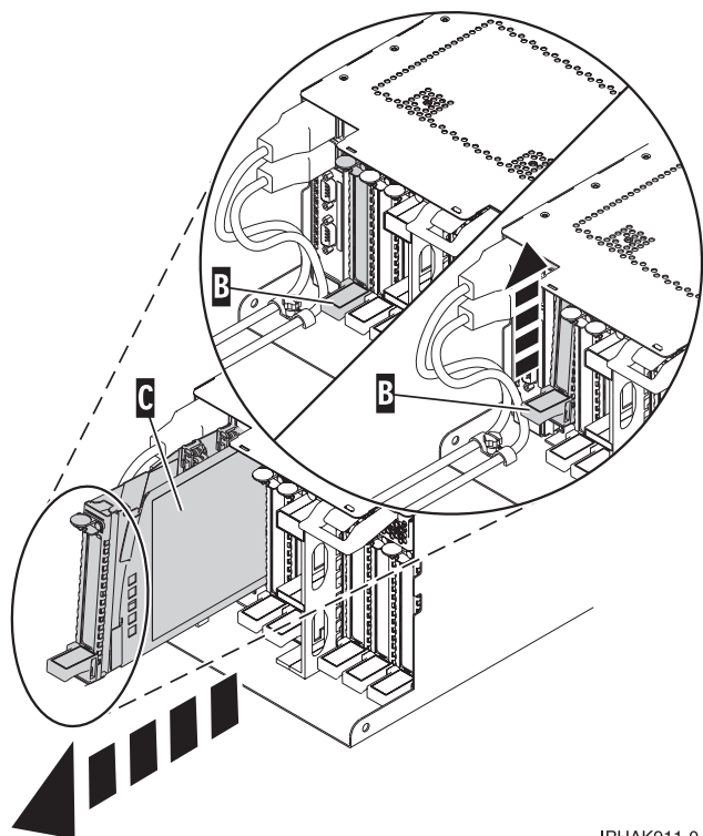
図 50. システム装置から取り外された PCI アダプター・カセット
