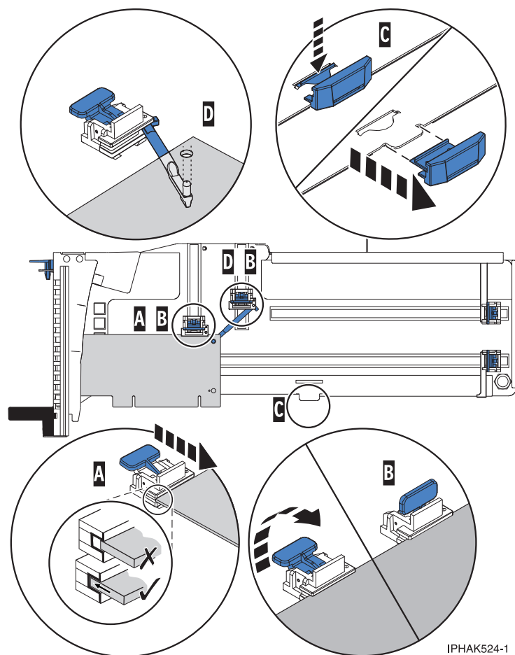
図 81. 所定位置に保持具およびフック・アームが付いた PCI アダプター・カセット内の小型 PCI アダプター
