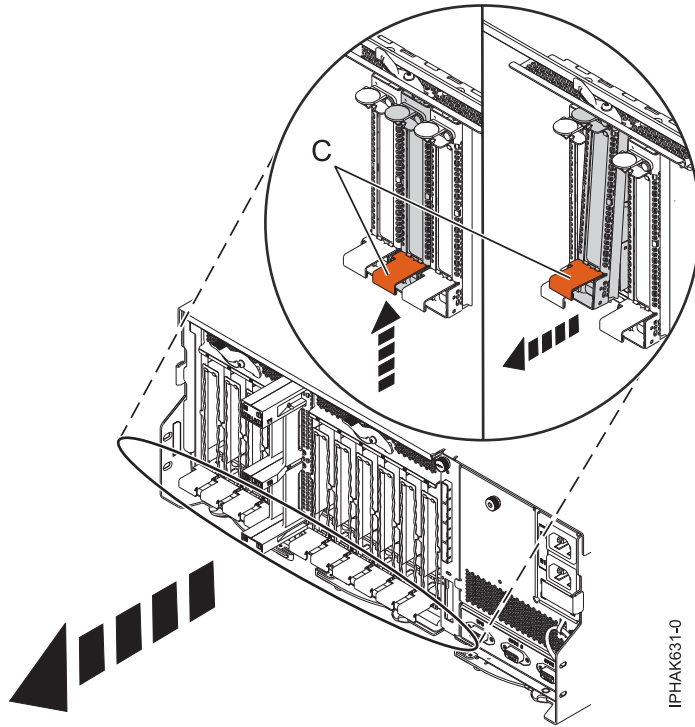
図 101. PCI アダプター・カセットの取り外し
