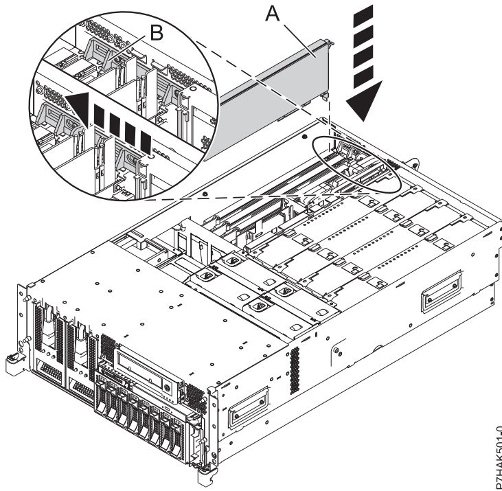
図 17. ラック・マウント型システム装置で取り替えられた PCI アダプター
