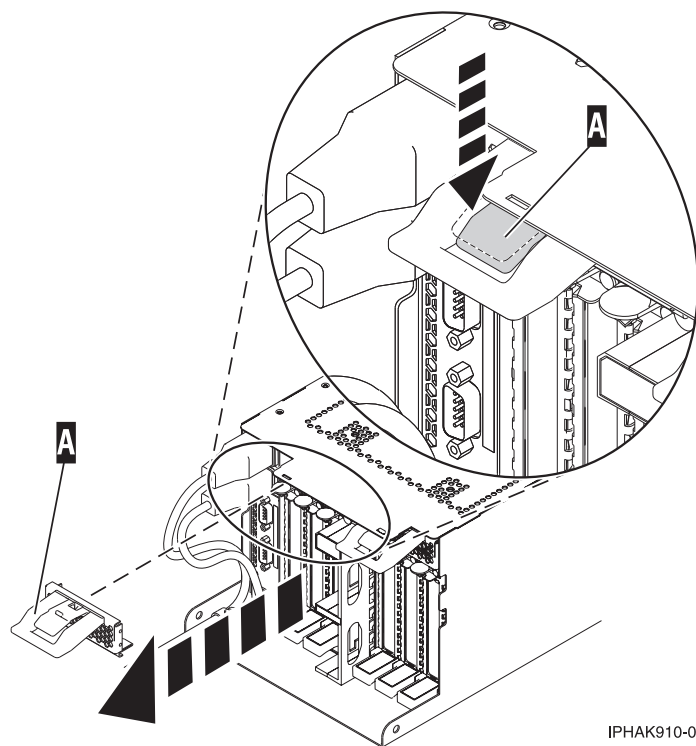
図 45. EMC シールドの取り外し
