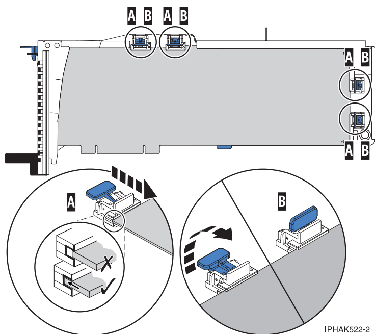
図 109. 所定位置に保持具およびスタビライザーが付いた PCI アダプター・カセット内の大型 PCI アダプター
