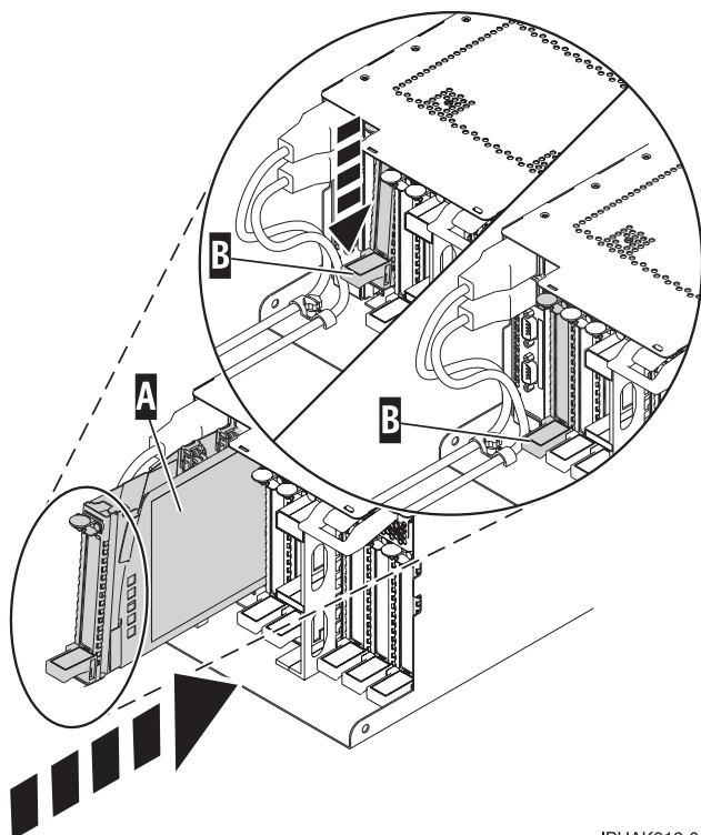
図 51. システム装置に取り付けられている PCI アダプター・カセット
