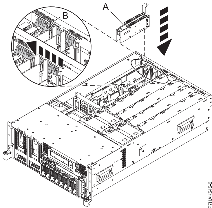
図 23. ラック・マウント型システム装置で取り替えられた PCI RAID および SSD SAS アダプター
