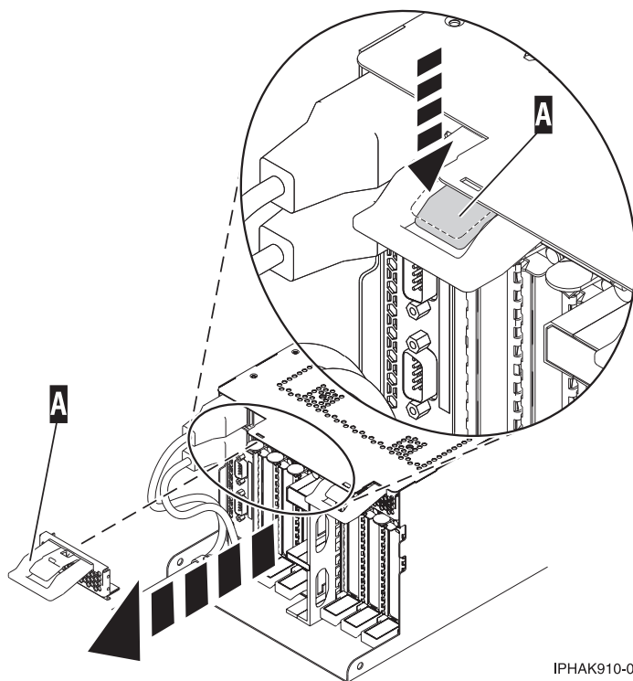
図 53. EMC シールドの取り外し
