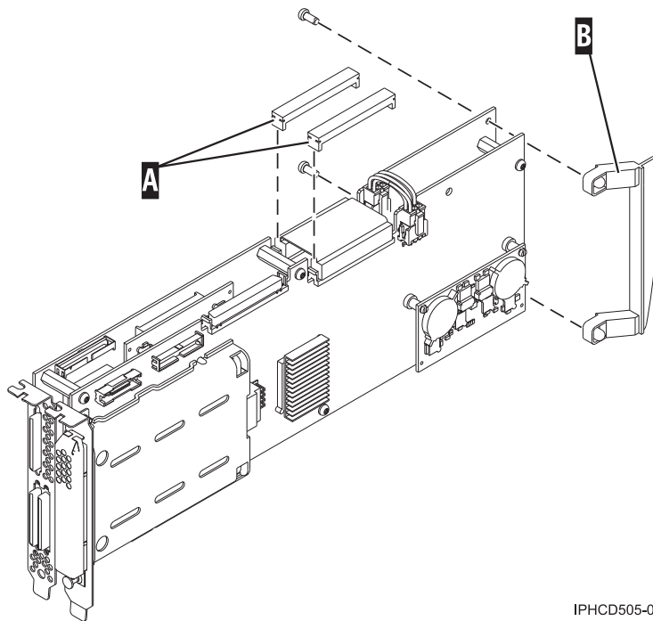
図 124. カセットに取り付けるためのアダプターの準備
