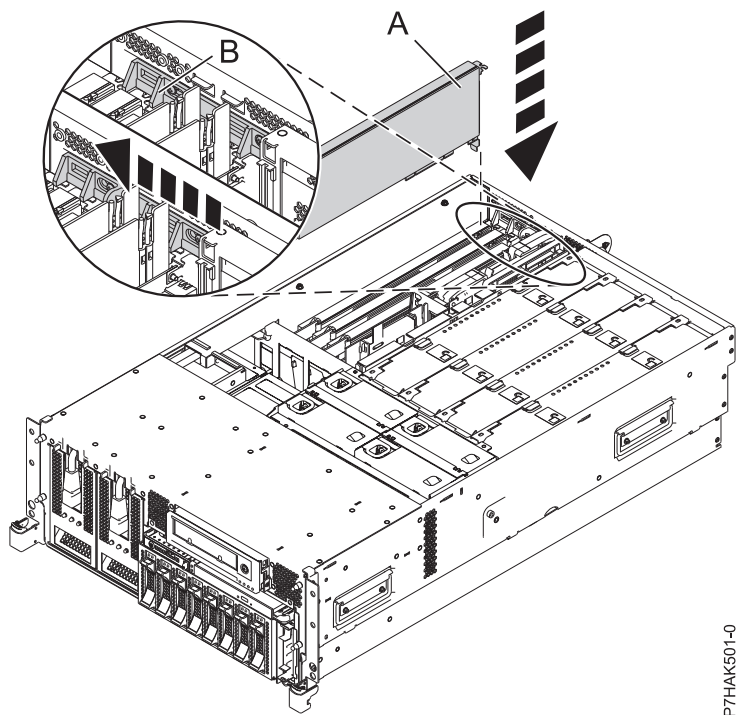
図 37. ラック・マウント型システム装置で取り替えられた PCI アダプター
