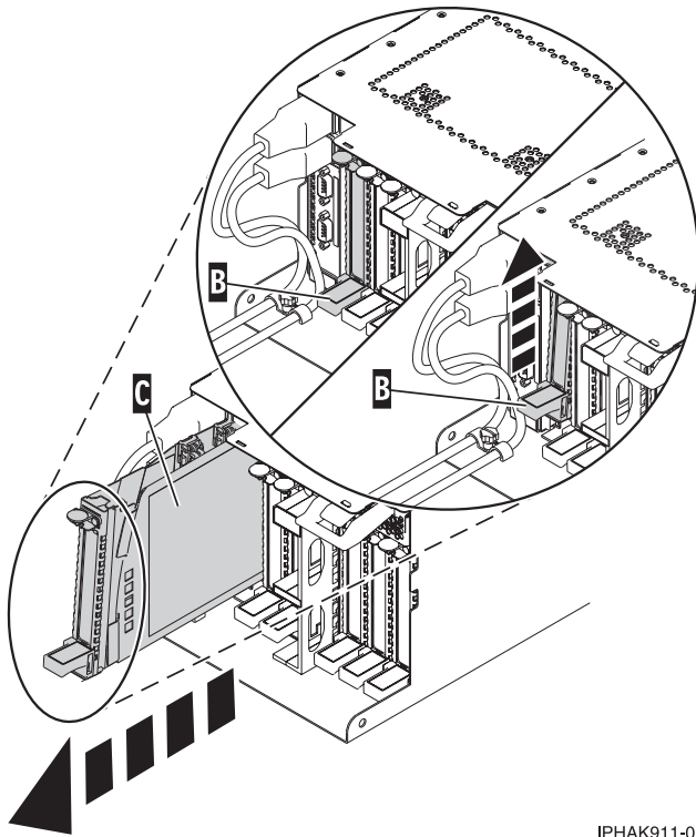
図 60. システム装置から取り外された PCI アダプター・カセット
