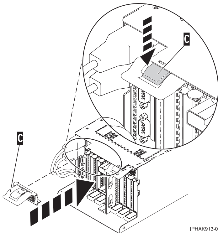
図 52. クローズ位置にある PCI アダプター EMC シールド
