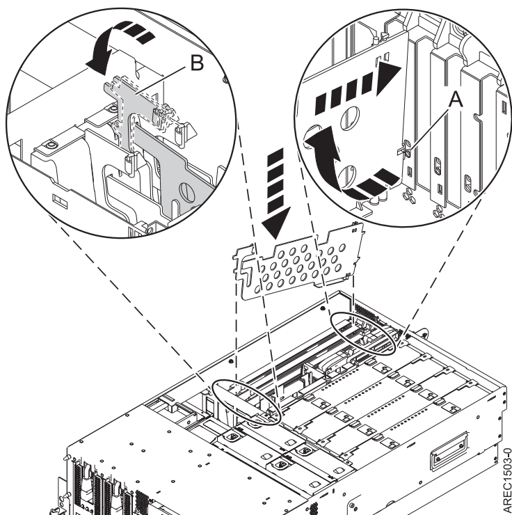
図 39. システム装置で取り替えられた PCI アダプター・セパレーター
