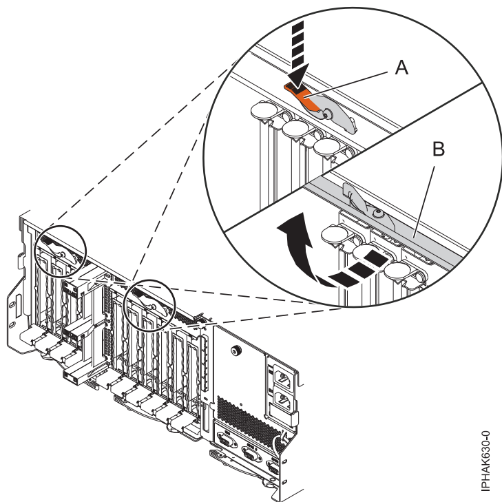
図 100. アクセス・ドアを開く
