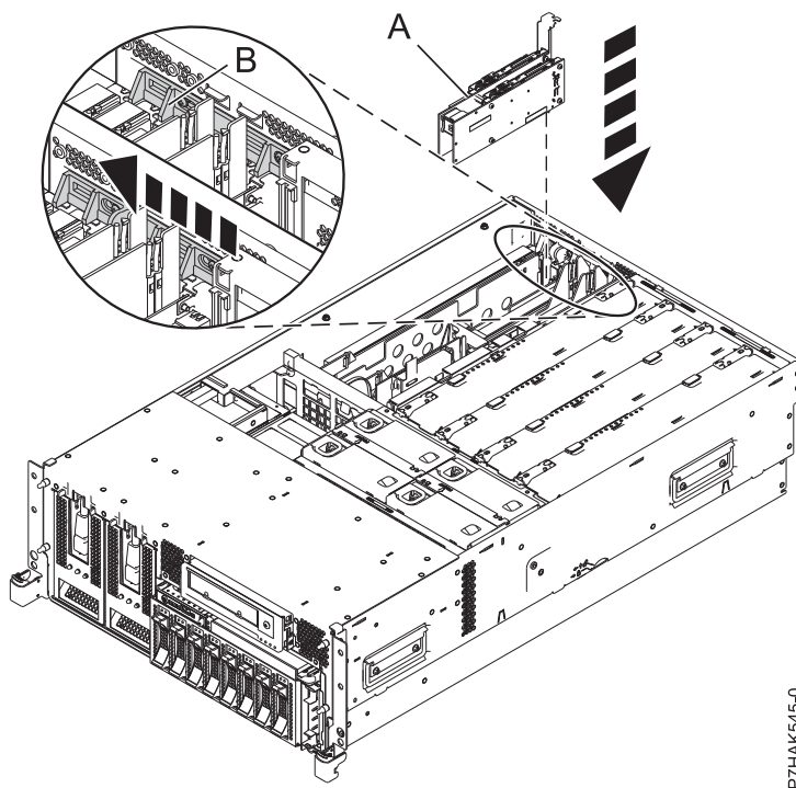
図 33. ラック・マウント型システム装置で取り替えられた PCI RAID および SSD SAS アダプター
