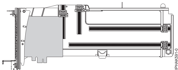
図 85. カセット内のアダプターの側面図
