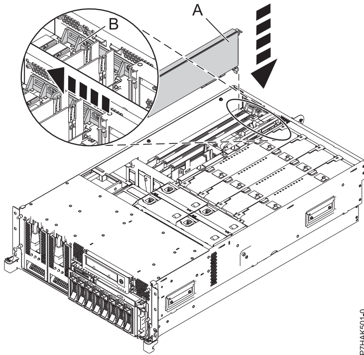
図 16. ラック・マウント型システム装置で取り替えられた PCI アダプター
