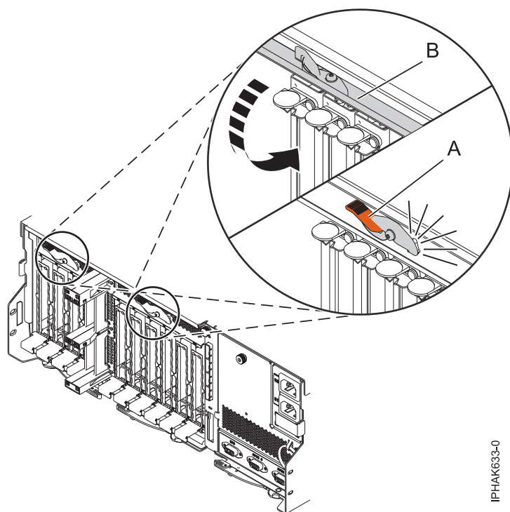
図 99. アクセス・ドアを閉じる
