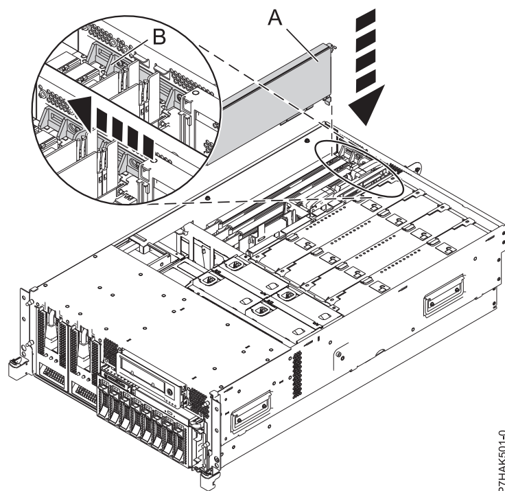
図2. ラック・マウント型システム装置で取り替えられた PCI アダプター
