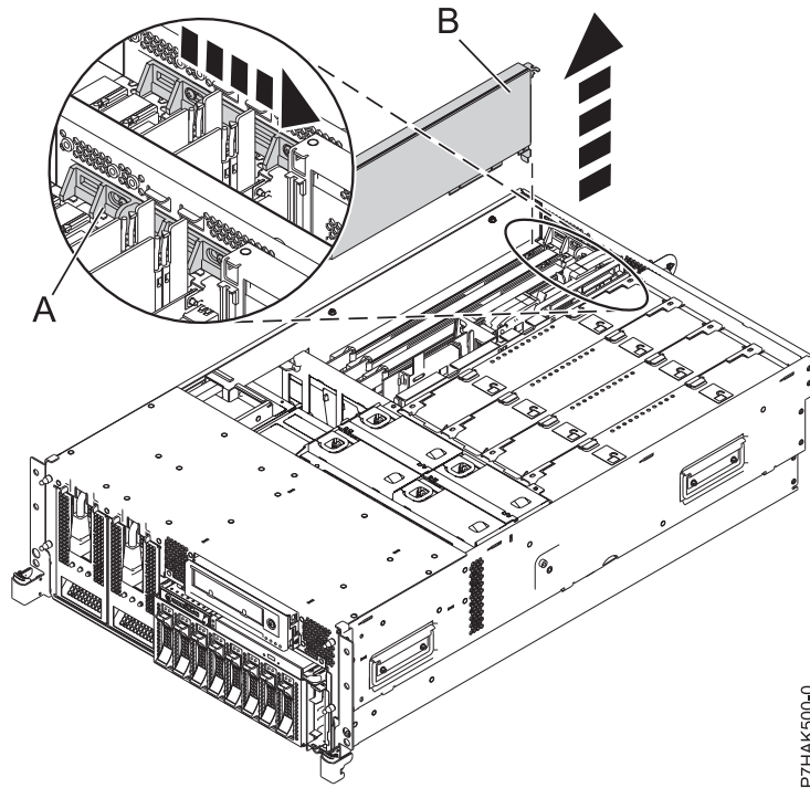
図 24. ラック・マウント型システム装置から取り外された PCI アダプターまたはフィラー・プレート
