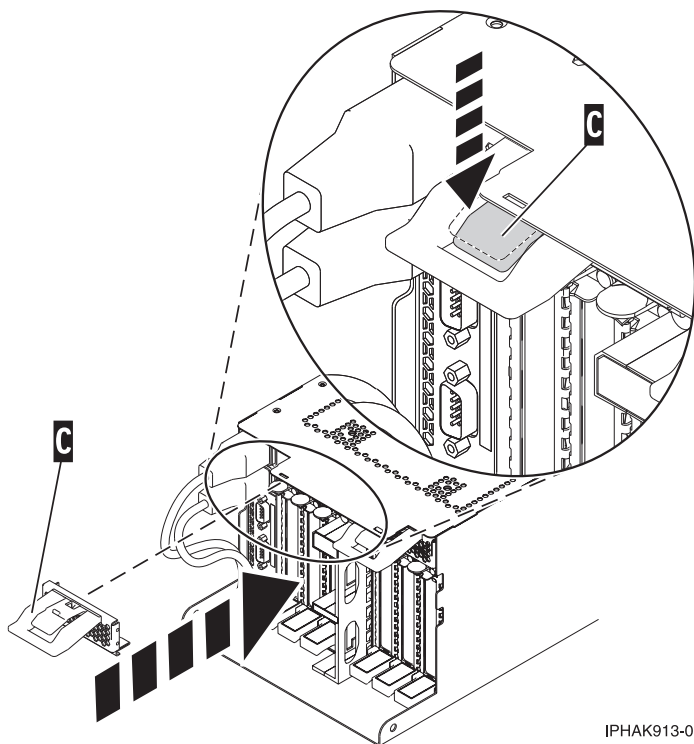
図 74. クローズ位置にある PCI アダプター EMC シールド
