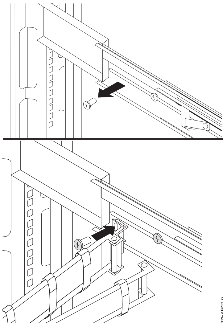
図 33. ケーブル・マネジメント・アームの取り付け
