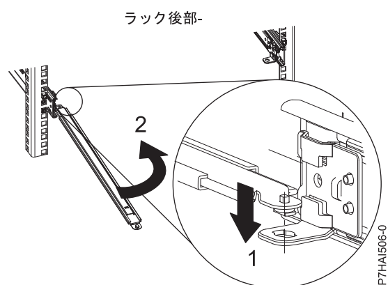
図 20. サポート・アームの接続
