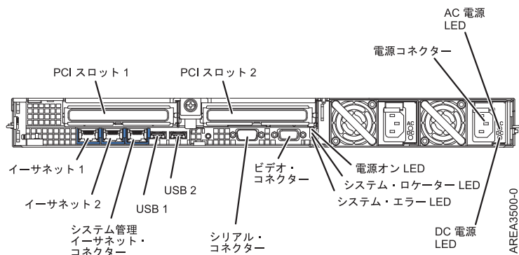
図 1. 7310-CR4 の背面図
