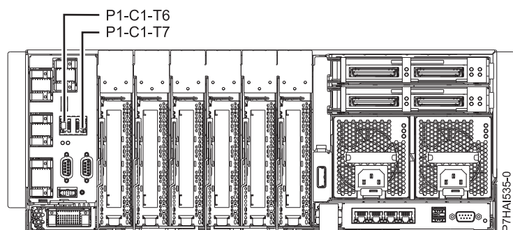
図 43. 9117-MMC、9117-MMD、9179-MHC、9179-MHD、または 8412-EAD の HMC ポートの位置
