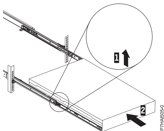
図 19. リリース・ラッチとサーバー
