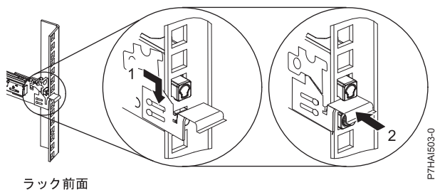
図 17. ラック前部のレールとピン
