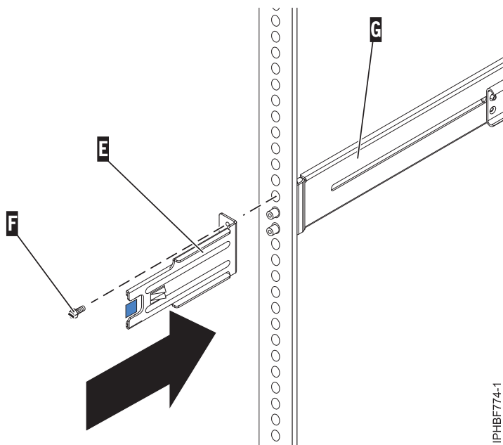
図7. ケーブル・マネージメント・ブラケットの左背面レールへの接続
