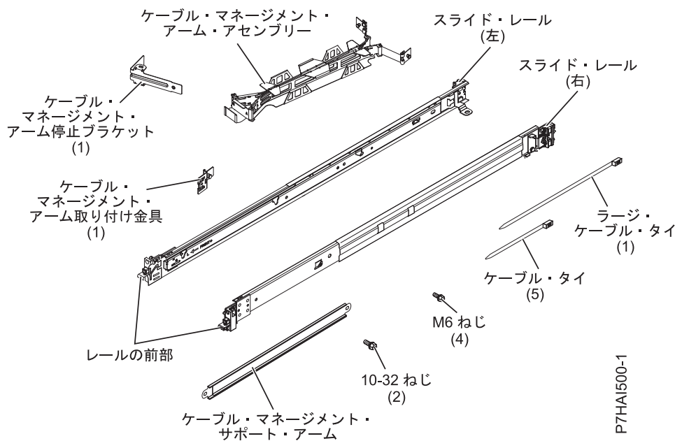
図 14. 部品目録
