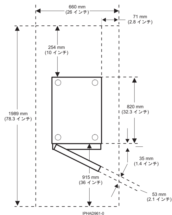
図 16. モデル 0554 および 7014-S11 平面図
