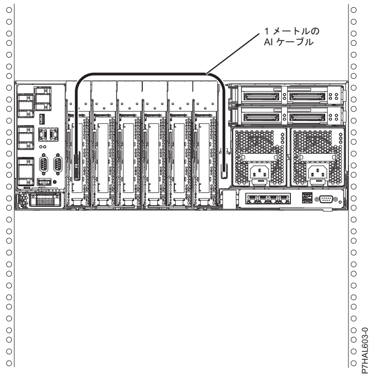
図 147. SAS アダプターと内部 SAS ディスク・スロット間 (システム外部 SAS ポートを使用)
