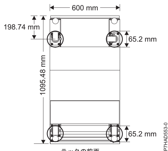
図 23. キャスターの位置
