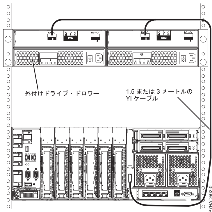
図 146. システム外部 SAS アダプター・ポートとディスク拡張ドロワー (モデル 9117-MMB および 9179-MHB) 間
