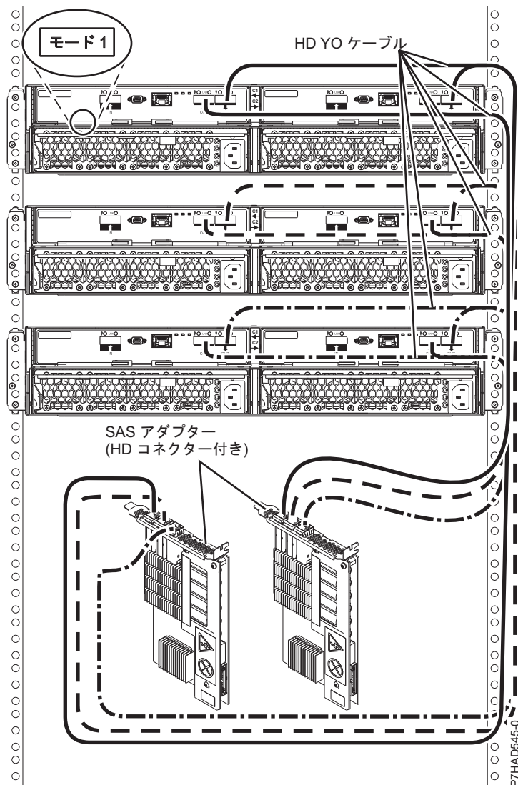
図 175. 2 つの SAS アダプターへの HD コネクターを使用した 3 つの 5887 ドロワーのモード 1 接続
