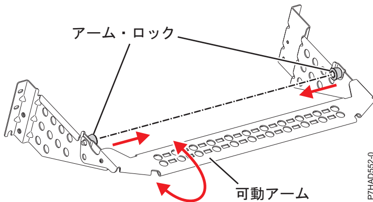
図 141. ケーブル管理ブラケット
