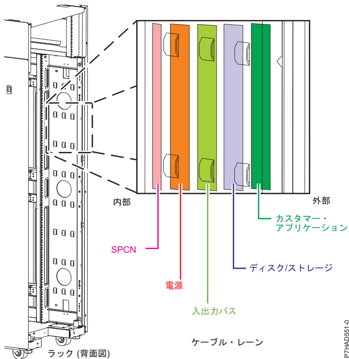
図 139. ケーブル管理ブリッジ LANCE
