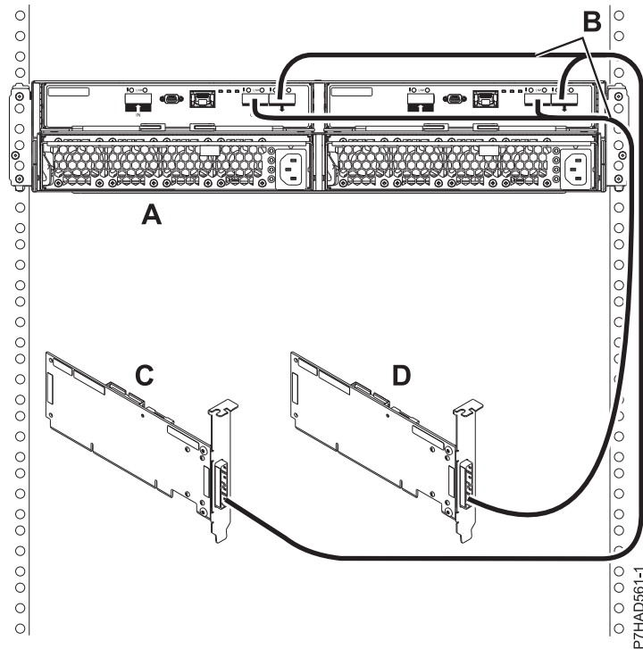
図 166. 2 つの単一 SAS アダプターへの YO ケーブルを使用した 5887 ドロワーのモード 2 接続
