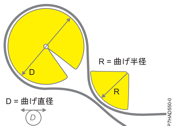
図 140. ケーブルの曲げ半径
