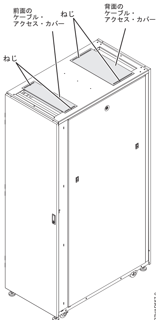
図 31. ケーブル・アクセス・カバー
