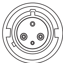
図 40. 電源コンセントのタイプ IEC 60309 3P+N+E
