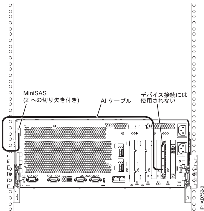
図 153. ディスク拡張ドロワーに接続された FC5904 または FC5908 アダプター
