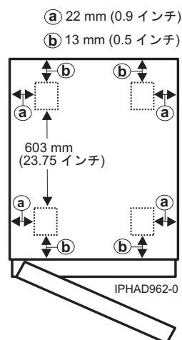
図 22. モデル 0554 および 7014-S11 のキャスター位置
