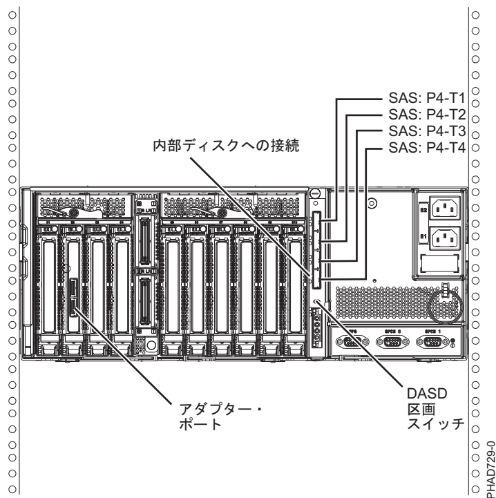
図 163. 2 つの RAID SAS アダプターと 1 つのディスク拡張ドロワー間 (マルチ・イニシエーター HA JBOD 構成)
