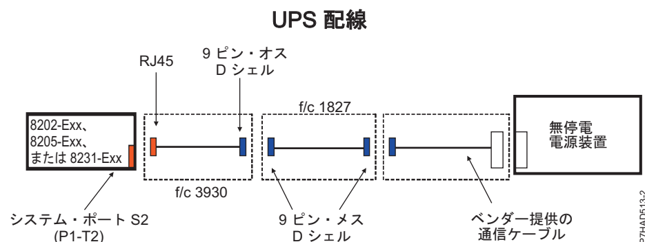
図 138. 8202-E4B、8202-E4C、8205-E6B、8205-E6C、8231-E2B、8231-E1C、8231-E1D、8231-E2C、8231-E2D、および 8268-E1D の無停電電源装置配線
