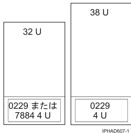
図 10. フィーチャー・コード 7884: 9406-520 および 9111-520 のラック搭載
