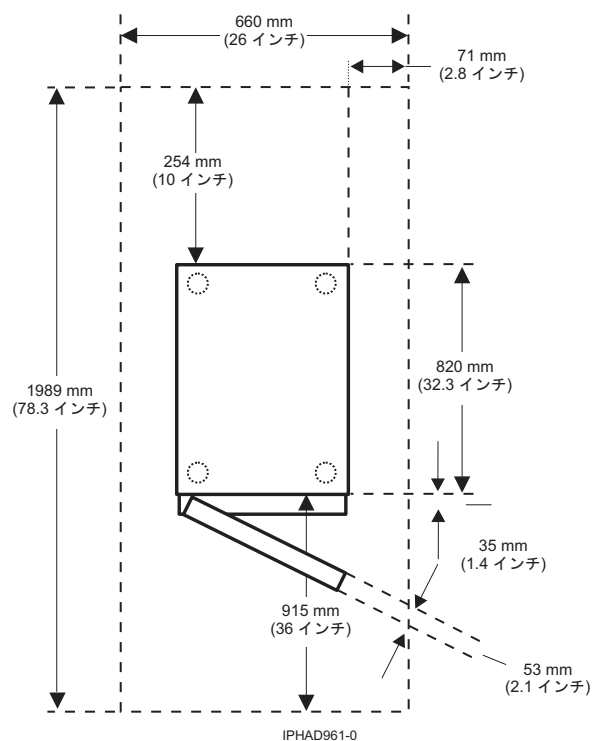
図 21. モデル 0554 および 7014-S11 平面図
