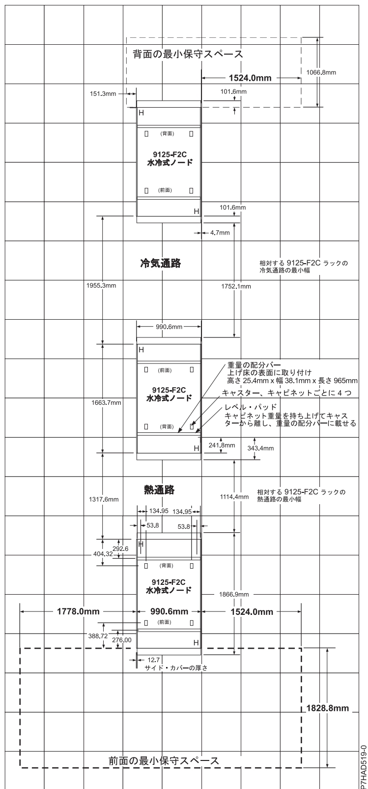
図 1. 単一ラックの場合の保守スペース - 熱通路と冷氣通路
