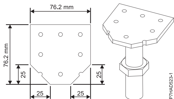
図4. 切り取る台座の寸法
