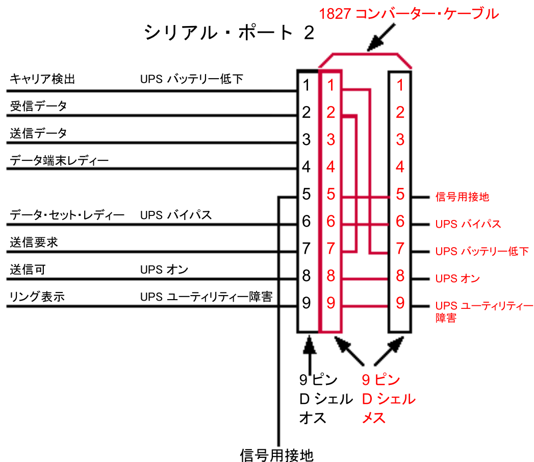
図 132. 1827 ケーブルの配線
