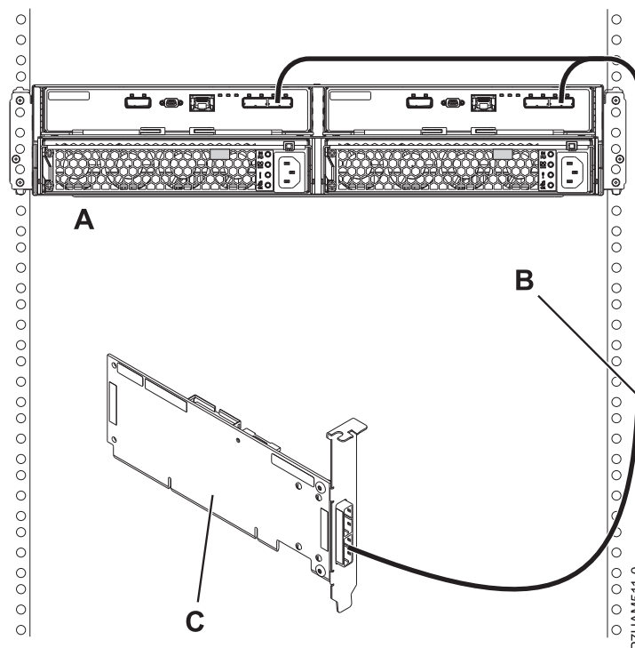
図 164. 単一の SAS アダプターへの YO ケーブルを使用した 5887 ドロワーのモード 1 接続
