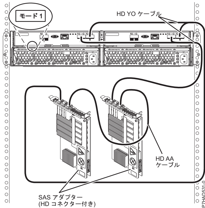
図 173. 2 つの SAS アダプターへの HD コネクターを使用した 5887 ドロワーのモード 1 接続
