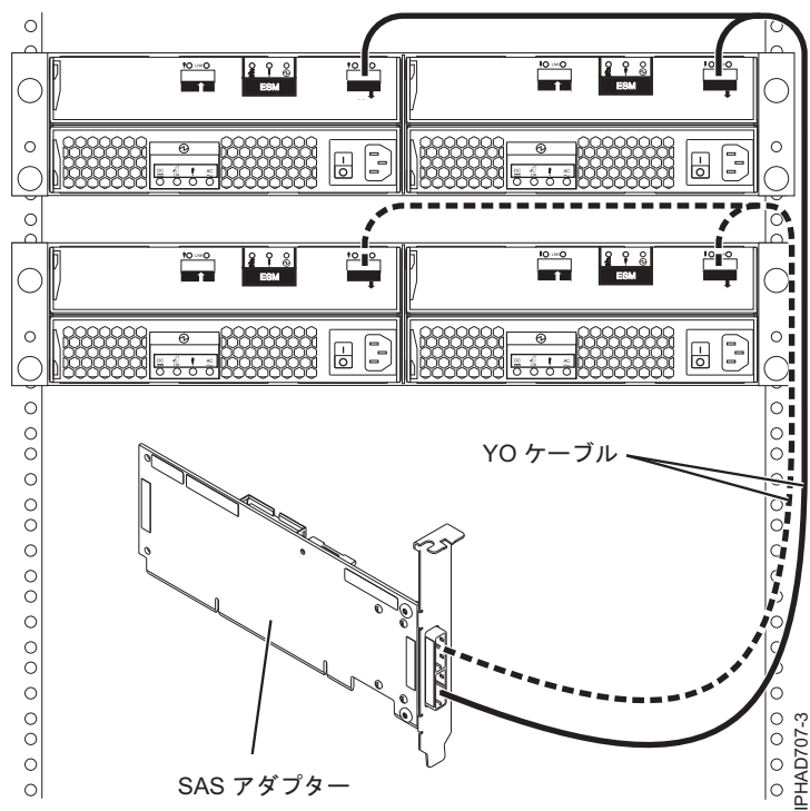
図 146. SAS アダプターと 2 つのディスク拡張ドロワー間
