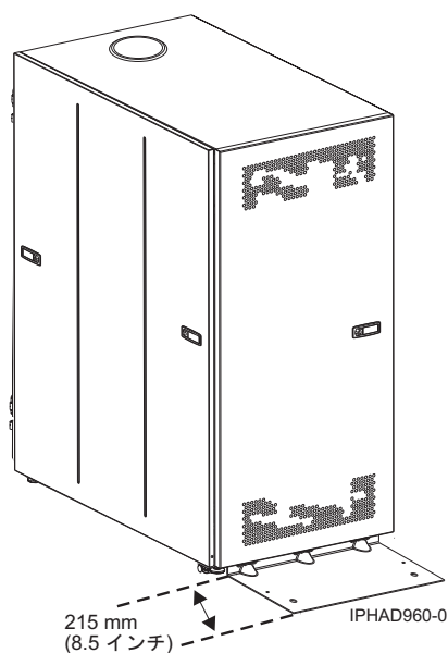
図 23. モデル 0555 および 7014-S25 (スタビライザー脚付属)
