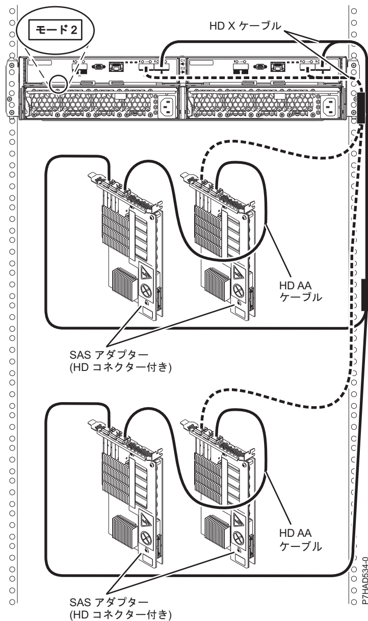
図 176. 2 ペアの SAS アダプターへの HD コネクターを使用した 5887 ドロワーのモード 2 接続
