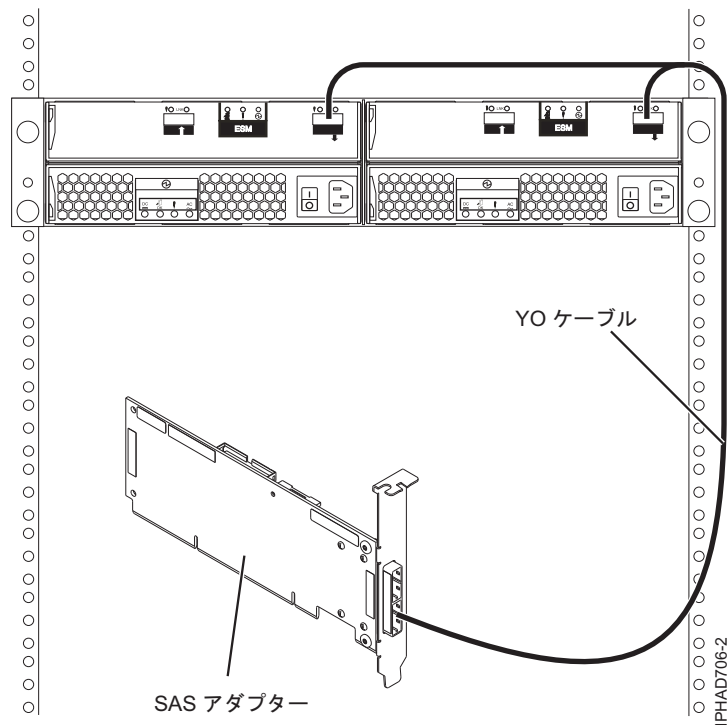
図 145. SAS アダプターとディスク拡張ドロワー間
