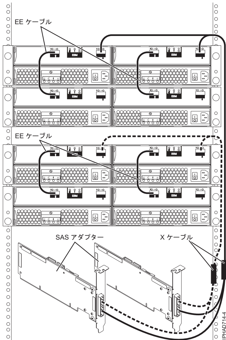
図 156. 2 つの SAS RAID アダプターと 4 つのディスク拡張ドロー間 (マルチ・イニシエーター HA RAID 構成)
