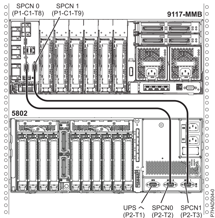
図 135. 8412-EAD、9117-MMB、9117-MMC、9117-MMD、9179-MHB、9179-MHC、9179-MHD、および 5208 または 5877 背面図のケーブル取り付け位置
