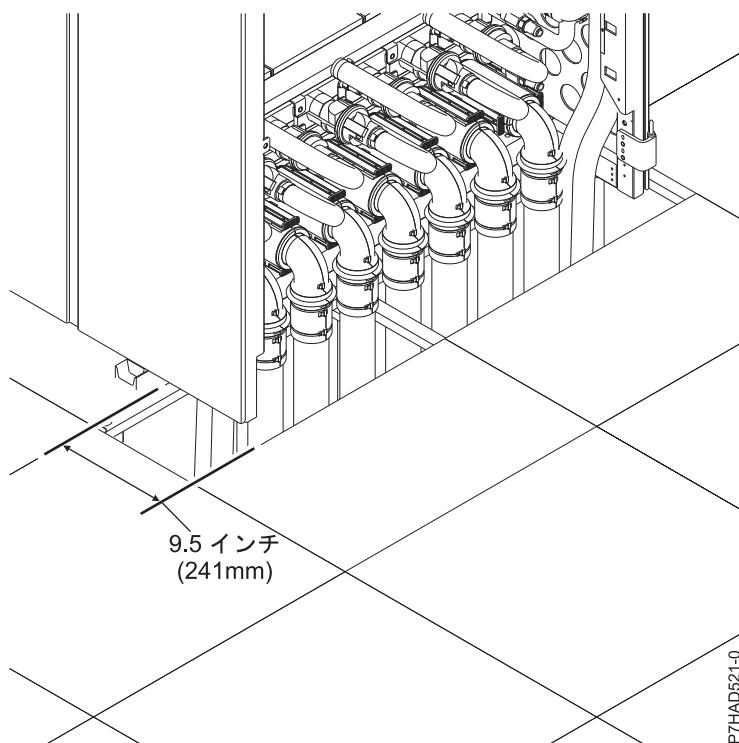
図 3. フロア・カットアウト
