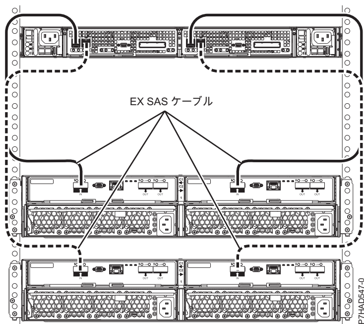
図 178. HD EX ケーブルを使用した、2 つの 5887 ドロワーから 1 つの EDR1 への接続
