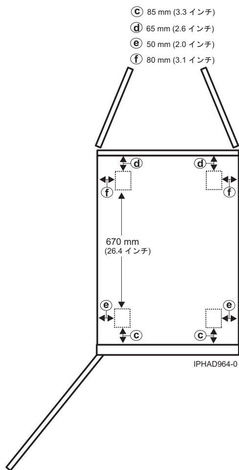
図 25. モデル 0555 および 7014-S25 のキャスター位置
