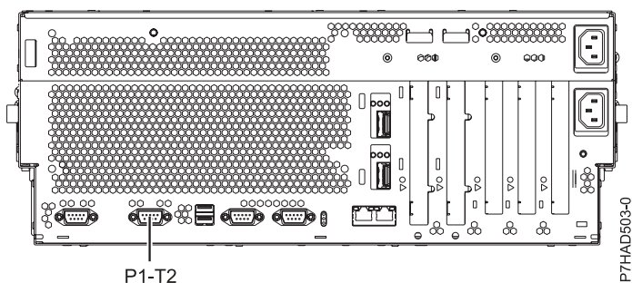
図 134. 8233-E8B および 8236-E8C の背面図とケーブル取り付け位置
