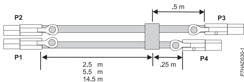
図 142. SAS 外付け X ケーブル・アセンブリのケーブルの長さ
