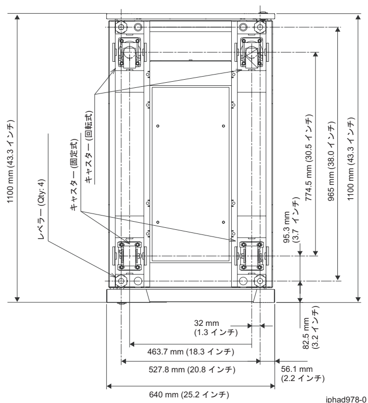
図 26. キャスターおよびレベラーの位置
