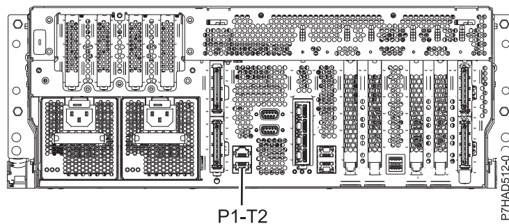
図 137. 8202-E4B、8202-E4C、8202-E4D、8205-E6B、8205-E6C、および 8205-E6D の背面図とケーブル取り付け位置
