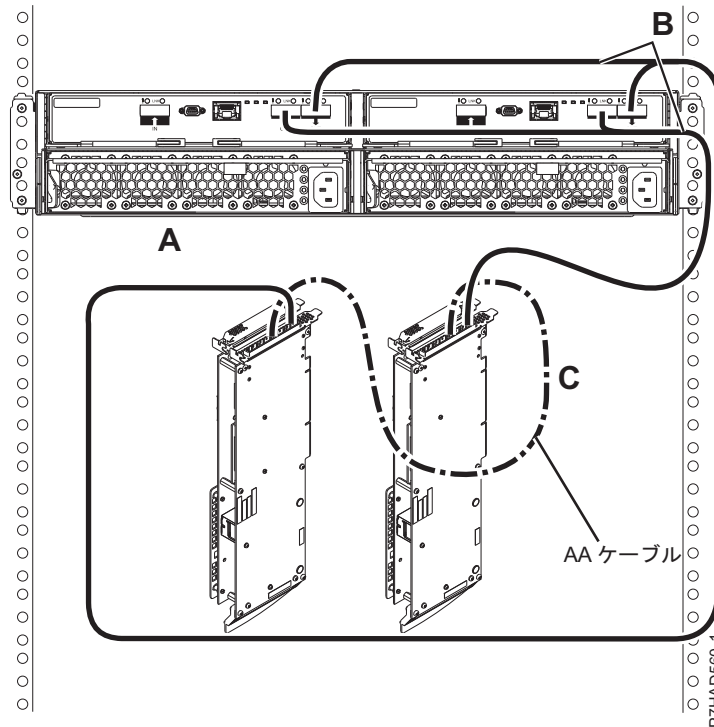
図 172. 2 つの SAS アダプターへの YO ケーブルを使用した 5887 ドロワーのモード 1 接続
