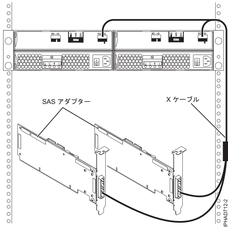
図 154. 2 つの SAS RAID アダプターと 1 つのディスク拡張ドロワー間 (マルチ・イニシエーター HA RAID 構成)
