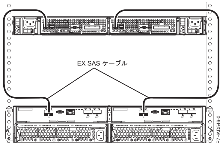
図 177. HD EX ケーブルを使用した、1 つの 5887 ドロワーから 1 つの EDR1 への接続
