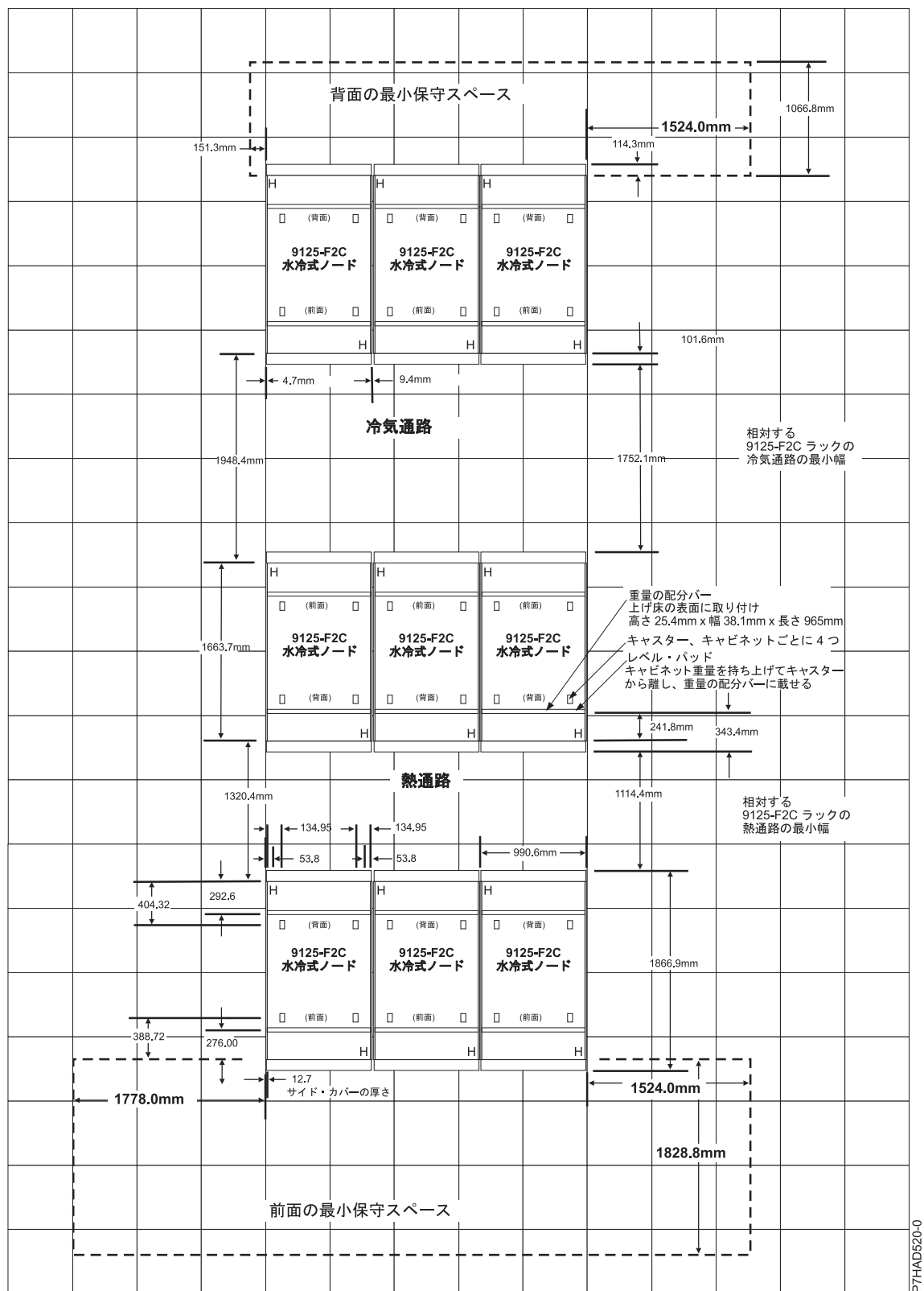
図 2. 複数ラックの場合の保守スペース - 熱通路と冷氣通路
