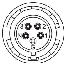
図 36. プラグ・ピン配列
