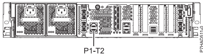
図 136. 8231-E2B、8231-E1C、8231-E1D、8231-E2C、8231-E2D、および 8268-E1D の背面図とケーブル取り付け位置
