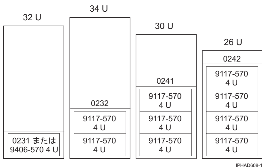
図 12. 570 のラック搭載
