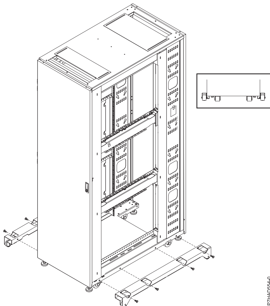
図 32. アウトリガーの位置
