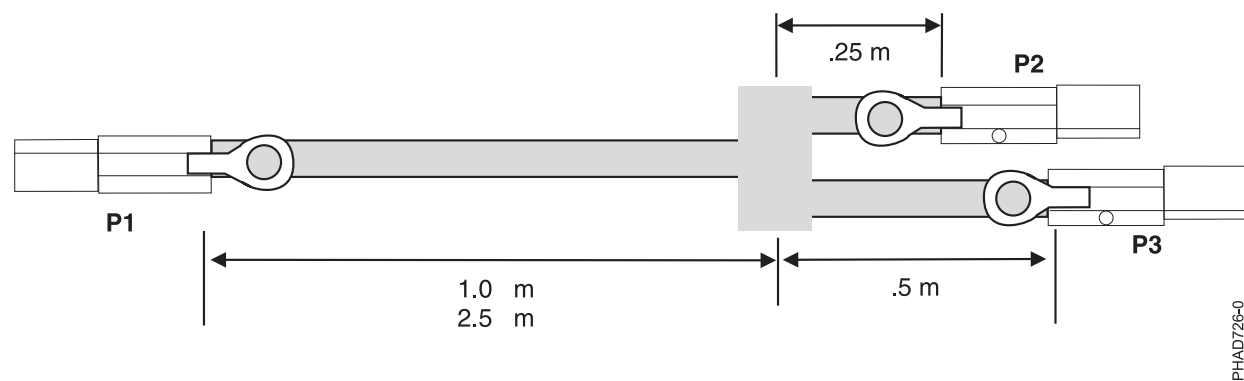
図 144. SAS 外付け Y1 ケーブル・アセンブリのケーブルの長さ
