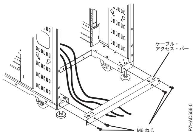
図 30. ケーブル・アクセス・バー
