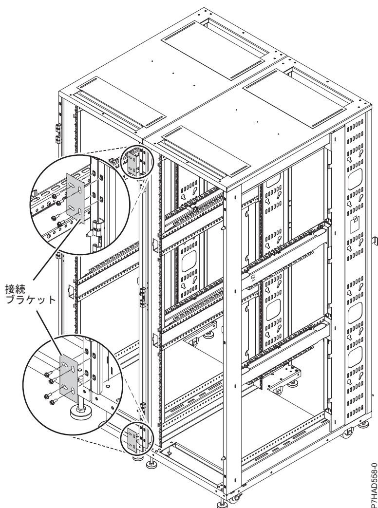
図 33. 接続ブラケット
