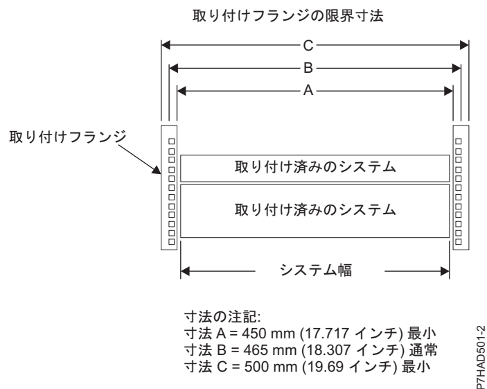
図 34. 取り付けフランジの限界寸法
