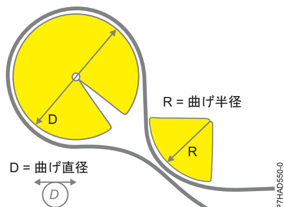
図 135. ケーブルの曲げ半径
