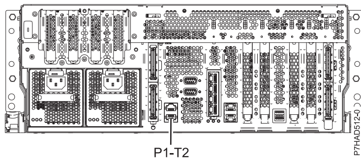
図 132. 8202-E4B、8202-E4C、8202-E4D、8205-E6B、8205-E6C、および 8205-E6D の背面図とケーブル取り付け位置
