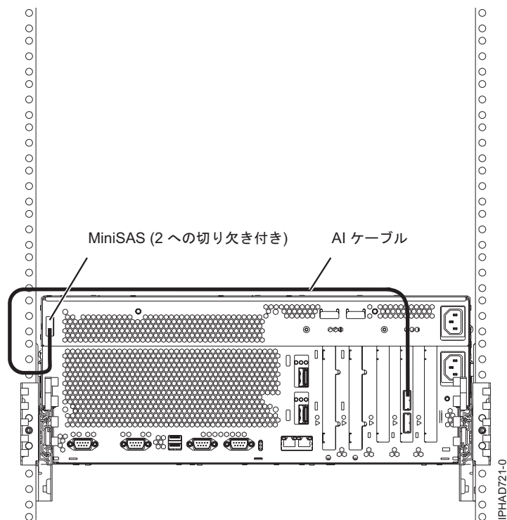
図 147. SAS アダプターと内部 SAS ディスク・スロット間 (システム外部 SAS ポートを使用)
