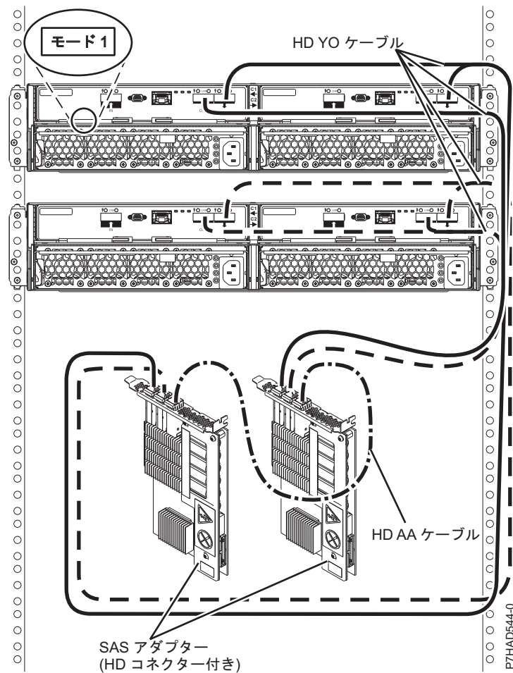
図 169. 2 つの SAS アダプターへの HD コネクターを使用した 2 つの 5887 ドロワーのモード 1 接続
