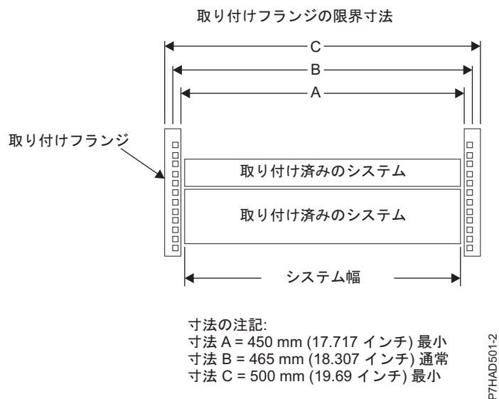
図 29. 取り付けフランジの限界寸法
