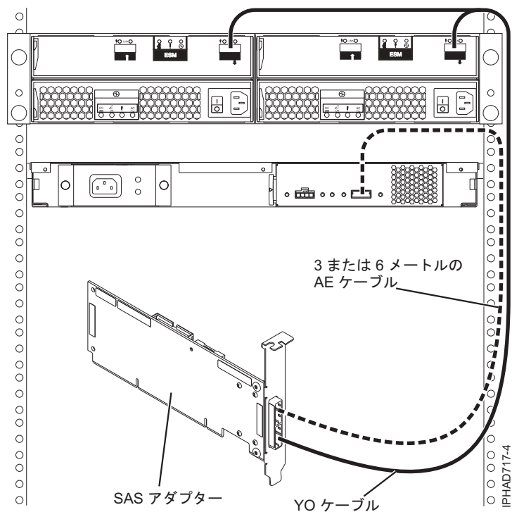
図 145. ディスク拡張ドロワーとメディア拡張ドロワーの両方と SAS アダプター間
