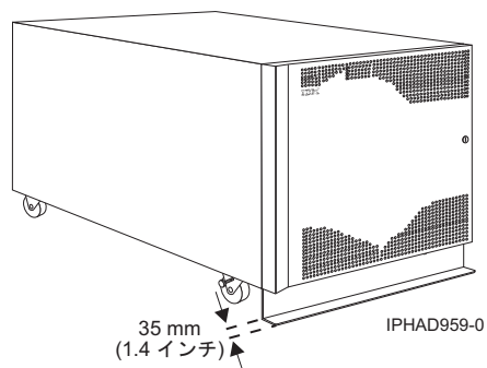
図 15. モデル 0554 および 7014-S11 (スタビライザー・バー付属)
