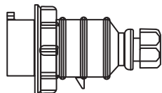
図 30. 電源プラグのタイプ IEC 60309 3P+N+E
