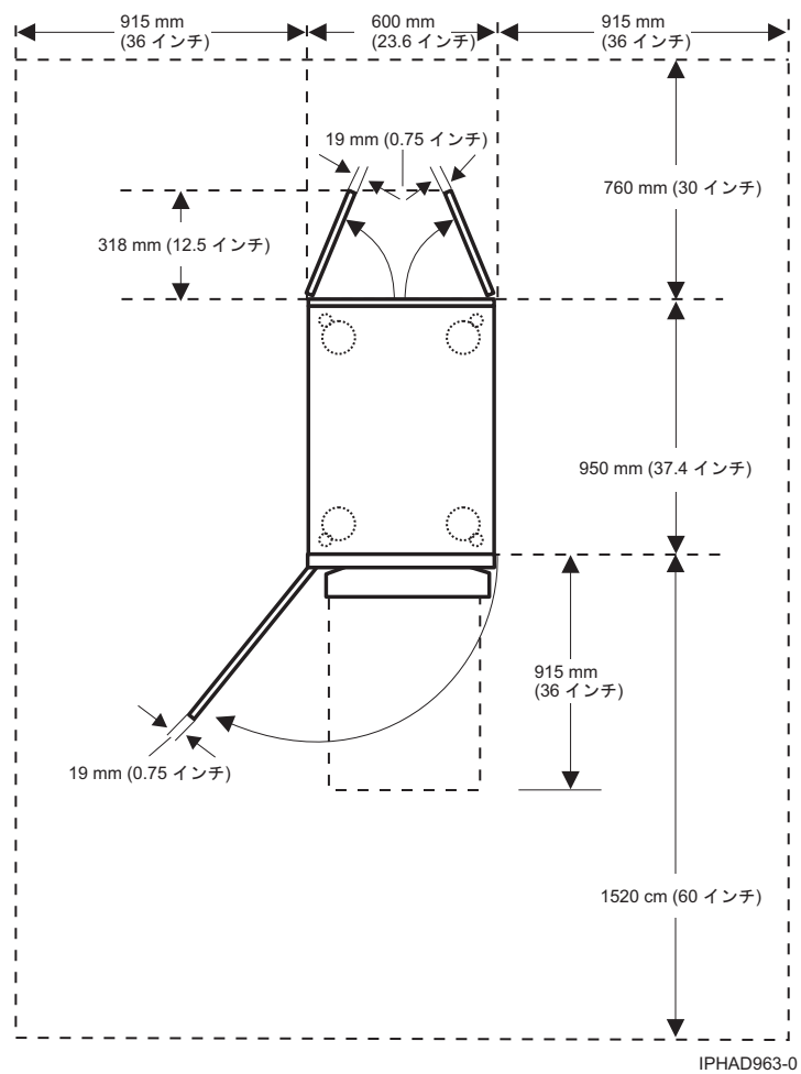
図 19. モデル 0555 および 7014-S25 平面図
