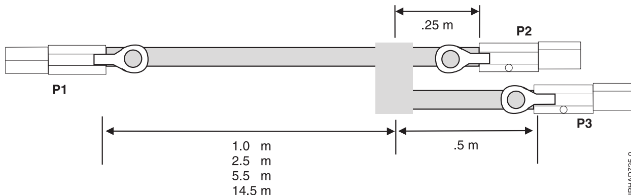
図 138. SAS 外付け Y0 ケーブル・アセンブリのケーブルの長さ
