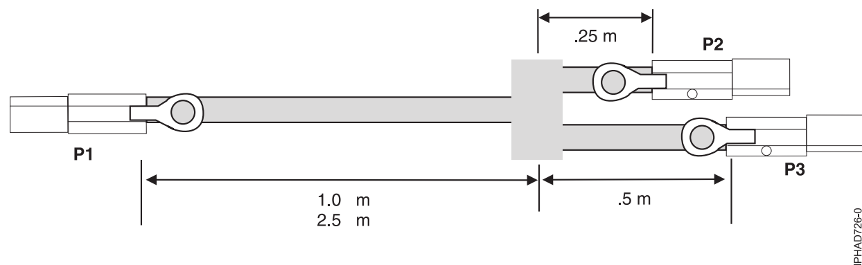
図 139. SAS 外付け Y1 ケーブル・アセンブリのケーブルの長さ
