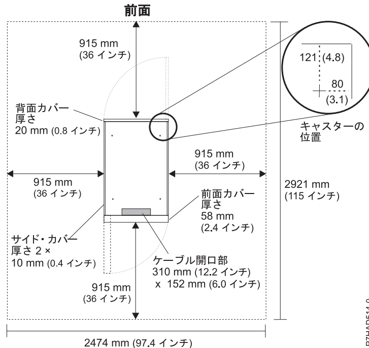
図 22. 7014-T00、7014-T42、および 0553 ラックの保守スペースとキャスター位置
