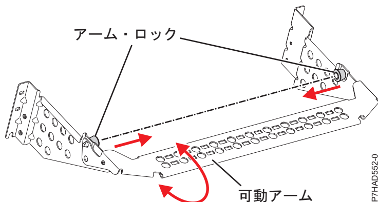
図 136. ケーブル管理ブラケット
