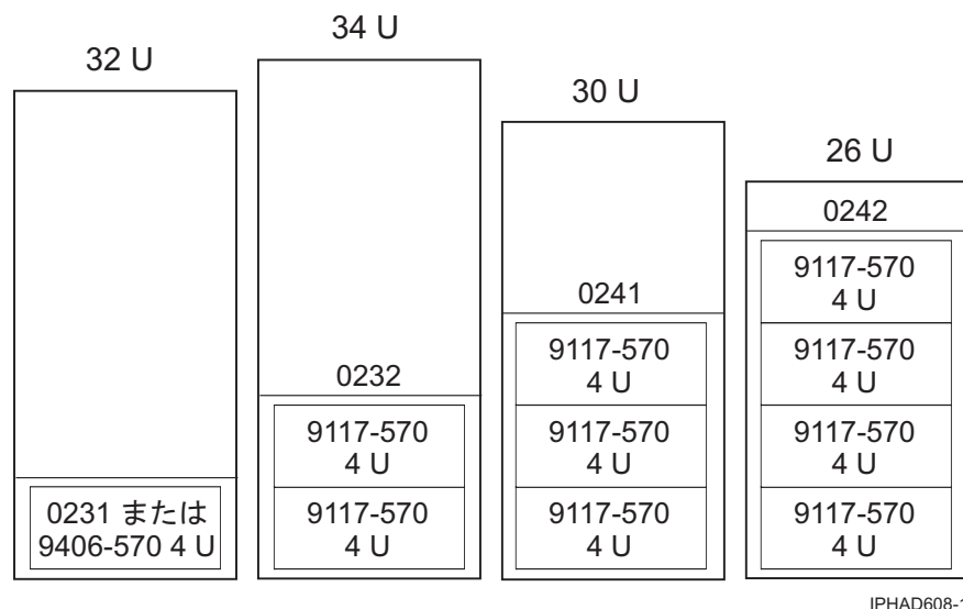
図 7. 570 のラック搭載
