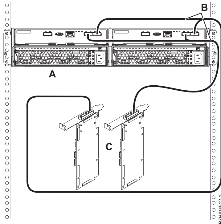
図 164. 2 つの SAS アダプターへの YO ケーブルを使用した 5887 ドロワーのモード 1 接続
