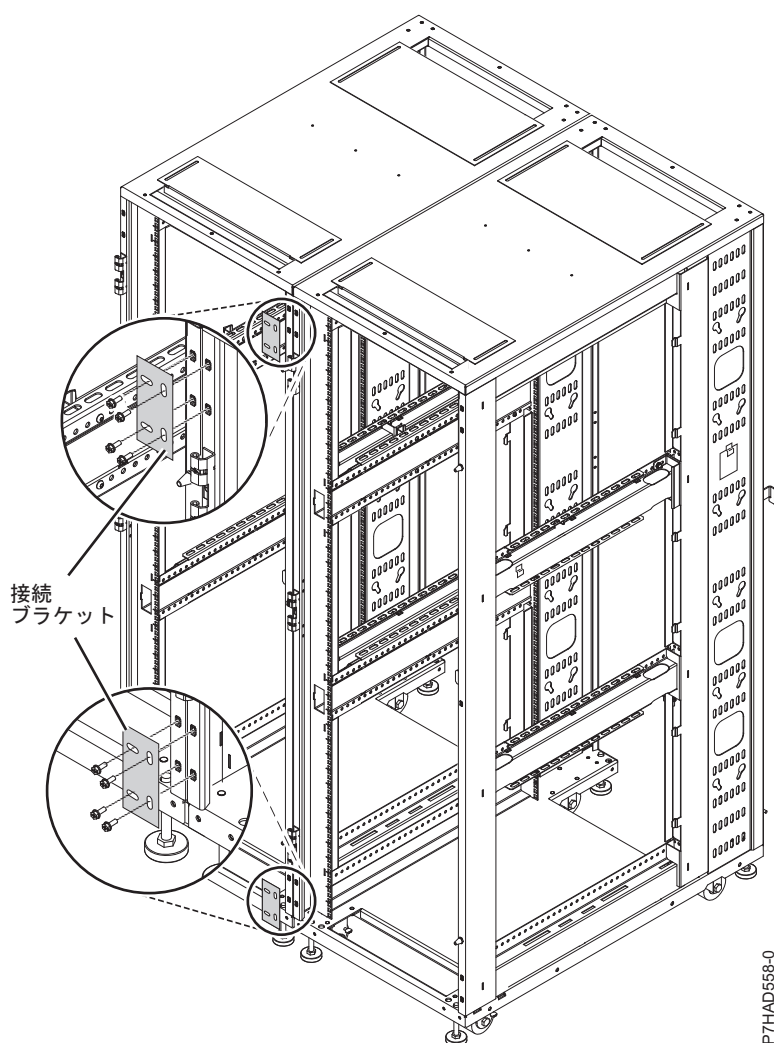
図 28. 接続ブラケット
