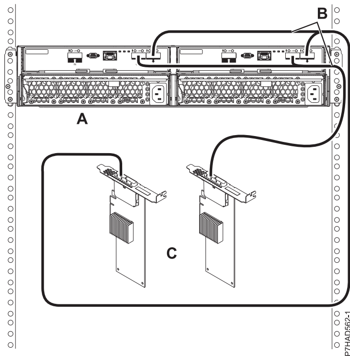
図 160. 2 つの SAS アダプターへの YO ケーブルを使用した 5887 ドロワーのモード 1 接続
