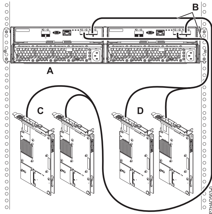
図 165. モード 2 接続を介して、2 ペアの FC 5805 または FC 5903 アダプターを 1 つの 5887 ドロワーに接続。
