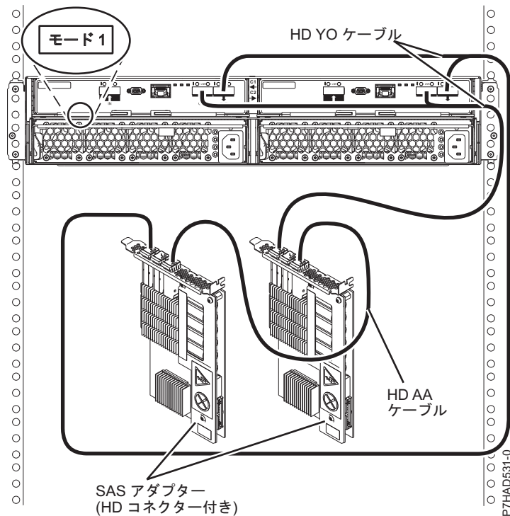
図 168. 2 つの SAS アダプターへの HD コネクターを使用した 5887 ドロワーのモード 1 接続
