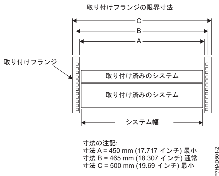
図 174. 取り付けフランジの限界寸法
