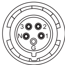
図 31. プラグ・ピン配列
