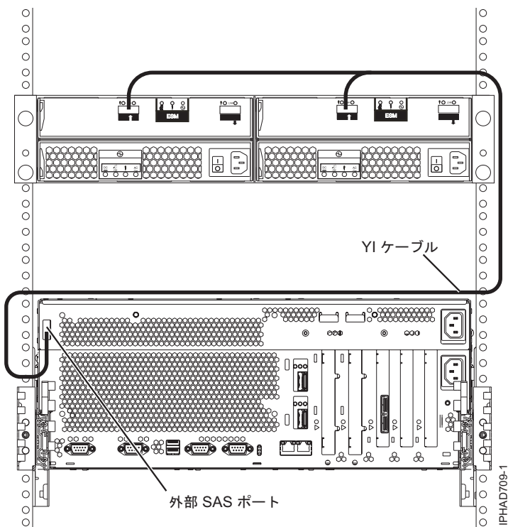
図 146. システム外部 SAS アダプター・ポートとディスク拡張ドロー間
