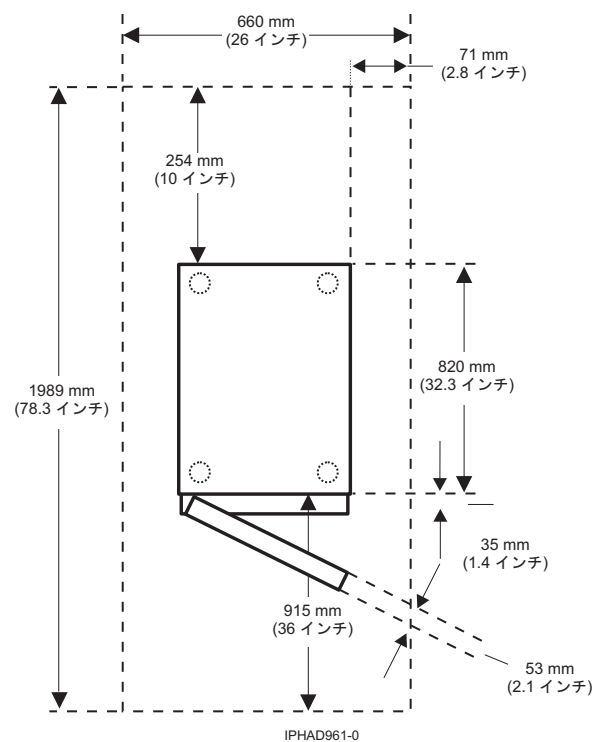
図 16. モデル 0554 および 7014-S11 平面図
