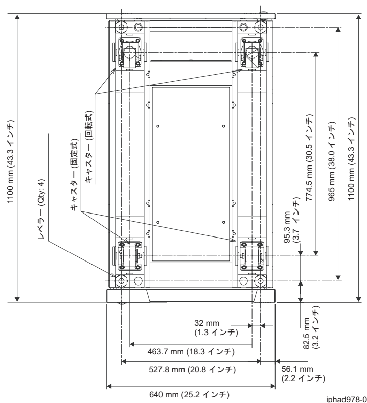
図 21. キャスターおよびレベラーの位置
