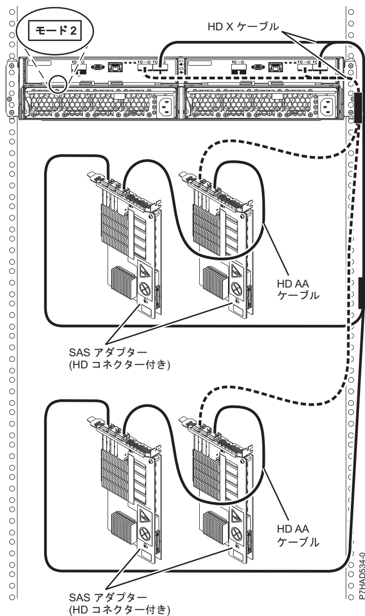
図 171. 2 ペアの SAS アダプターへの HD コネクターを使用した 5887 ドロワーのモード 2 接続
