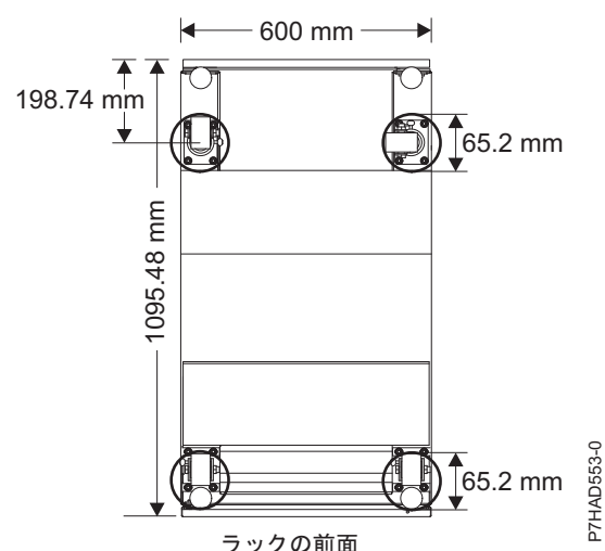
図 23. キャスターの位置
