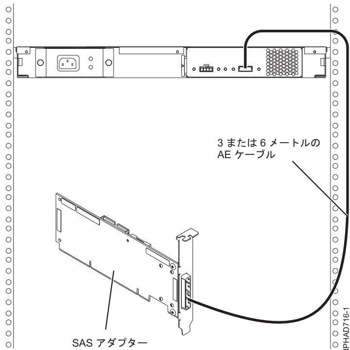
図 144. SAS アダプターとメディア拡張ドロワー間
