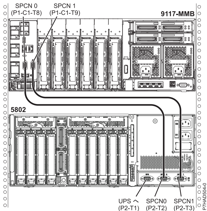
図 130. 8412-EAD、9117-MMB、9117-MMC、9117-MMD、9179-MHB、9179-MHC、9179-MHD、および 5208 または 5877 背面図のケーブル取り付け位置
