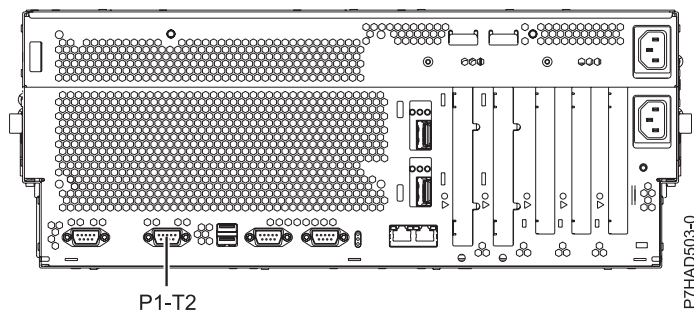
図 129. 8233-E8B および 8236-E8C の背面図とケーブル取り付け位置
