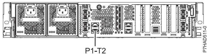
図 131. 8231-E2B、8231-E1C、8231-E1D、8231-E2C、8231-E2D、および 8268-E1D の背面図とケーブル取り付け位置
