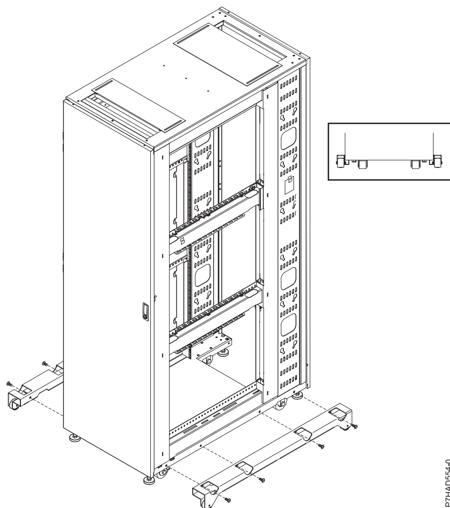
図 27. アウトリガーの位置
