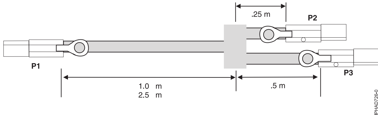
図 139. SAS 外付け YI ケーブル・アセンブリーのケーブルの長さ
