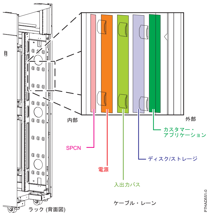
図 134. ケーブル管理ブリッジ LANCE
