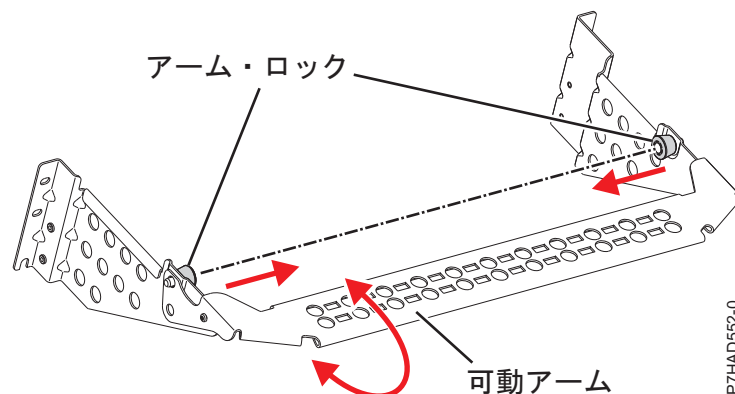
図 136. ケーブル管理ブラケット
