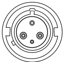
図 49. 電源コンセントのタイプ IEC 60309 2P+E
