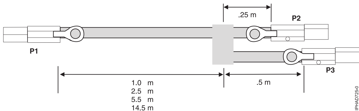
図 138. SAS 外付け YO ケーブル・アセンブリのケーブルの長さ
