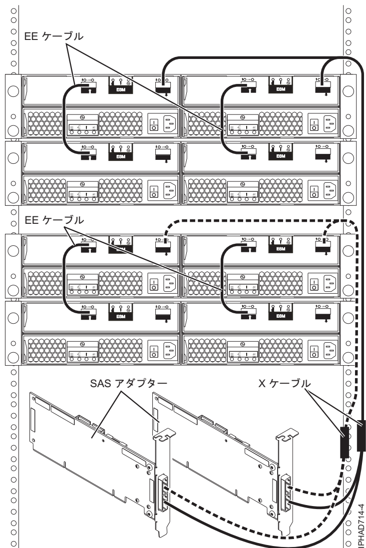
図 151. 2 つの SAS RAID アダプターと 4 つのディスク拡張ドロワー間 (マルチ・イニシエーター HA RAID 構成)
