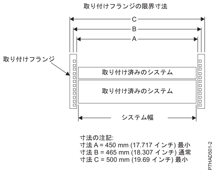
図 29. 取り付けフランジの限界寸法
