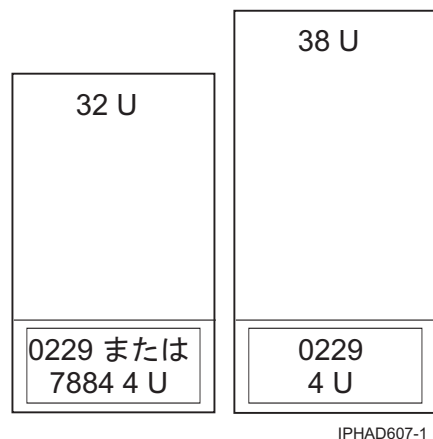
図 6. フィーチャー・コード 7884: 9406-520 および 9111-520 のラック搭載
