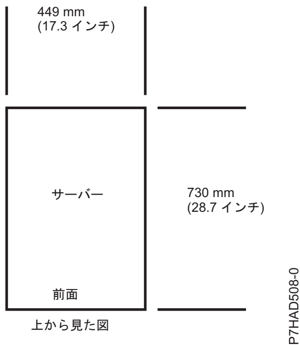
図 1. モデル 8202-E4B、8202-E4C、8202-E4D、8205-E6B、8205-E6C、および 8205-E6D の平面図 (ラック・マウント型サーバー)
