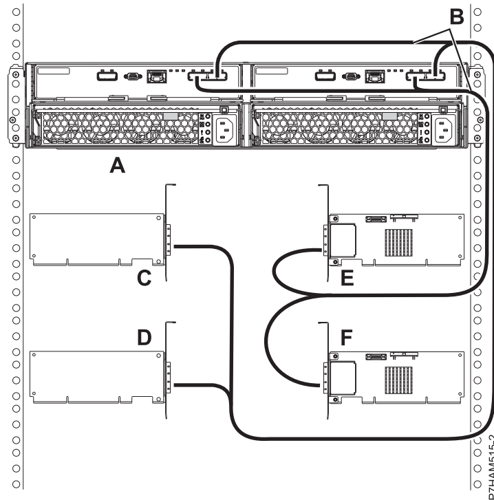
図 164. 4 つの単一 SAS アダプターへの X ケーブルを使用した 5887 ドロワーのモード 4 接続。
