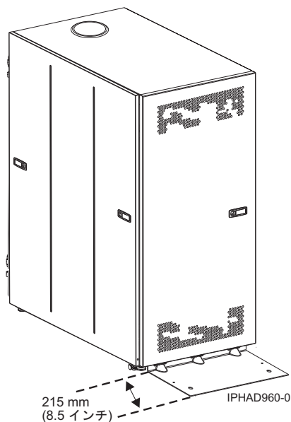
図 19. モデル 0555 および 7014-S25 (スタビライザー脚付属)
