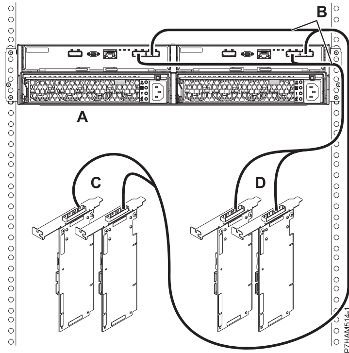
図 144. 2 ペアの SAS アダプターへの X ケーブルを使用した 5887 ドロワーのモード 2 接続
