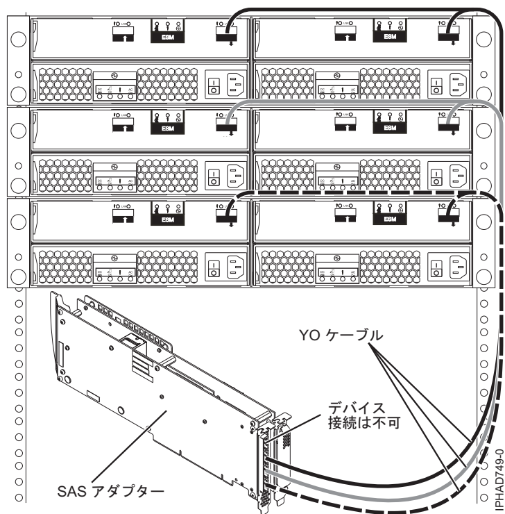
図 125. トライ・ポート SAS アダプターとディスク拡張ドロワー間
