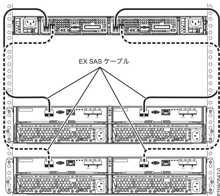
図 155. HD EX ケーブルを使用した、2 つの 5887 ドロワーから 1 つの EDR1 への接続
