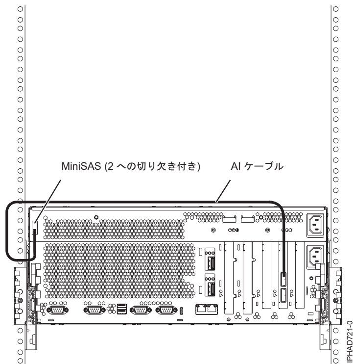
図 129. SAS アダプターと内部 SAS ディスク・スロット間 (システム外部 SAS ポートを使用)
