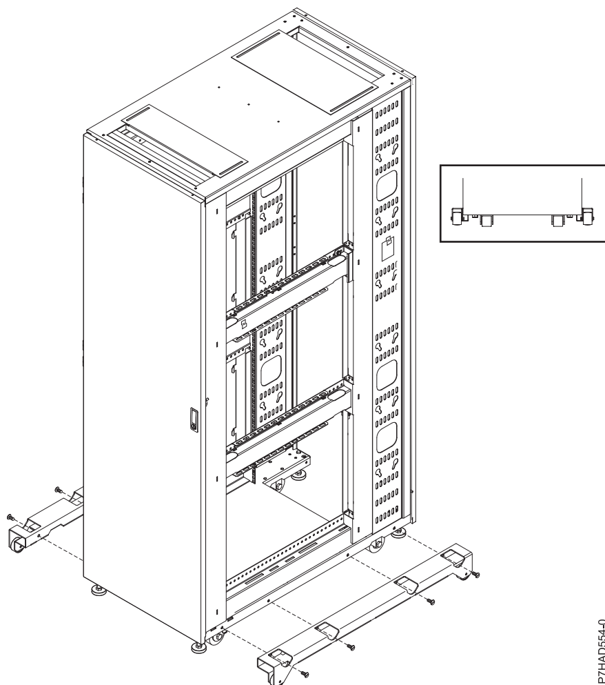
図 16. アウトリガーの位置
