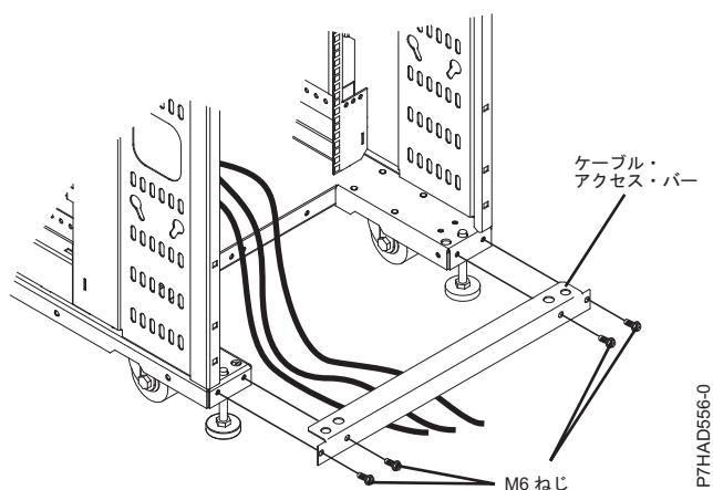
図 14. ケーブル・アクセス・バー
