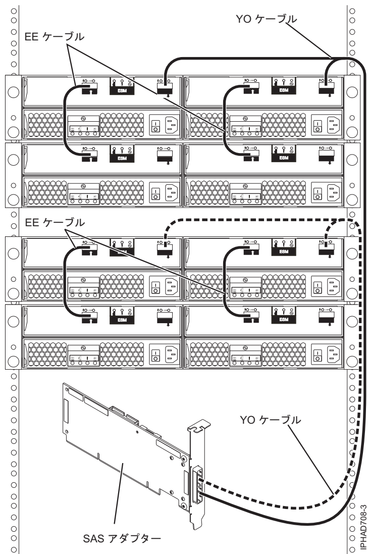
図 124. SAS アダプターと 4 つのディスク拡張ドロワー間
