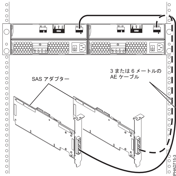
図 139. 2 つの RAID SAS アダプターと 1 つのディスク拡張ドロワー間 (マルチ・イニシエーター HA JBOD 構成)
