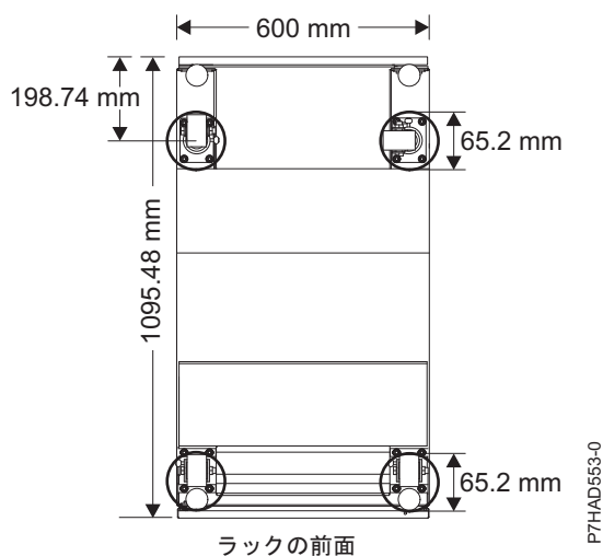
図 12. キャスターの位置
