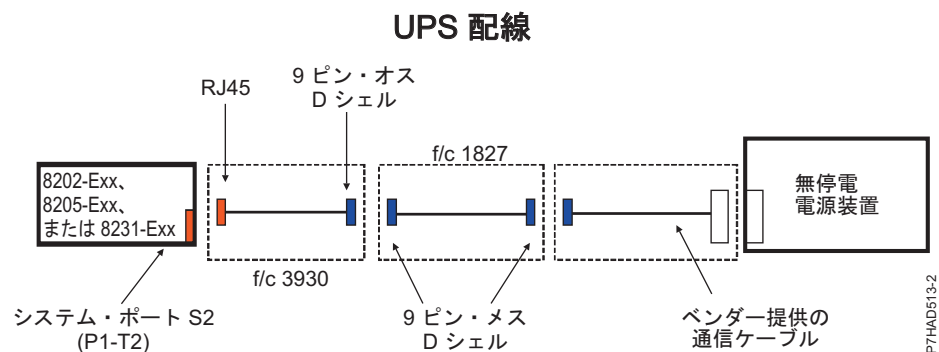
図 115. 8246-L1C、8246-L1S、8246-L2C、および 8246-L2S の無停電電源装置配線
