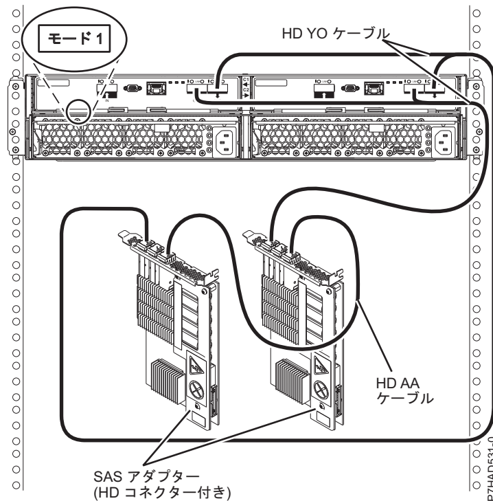
図 150. 2 つの SAS アダプターへの HD コネクターを使用した 5887 ドロワーのモード 1 接続
