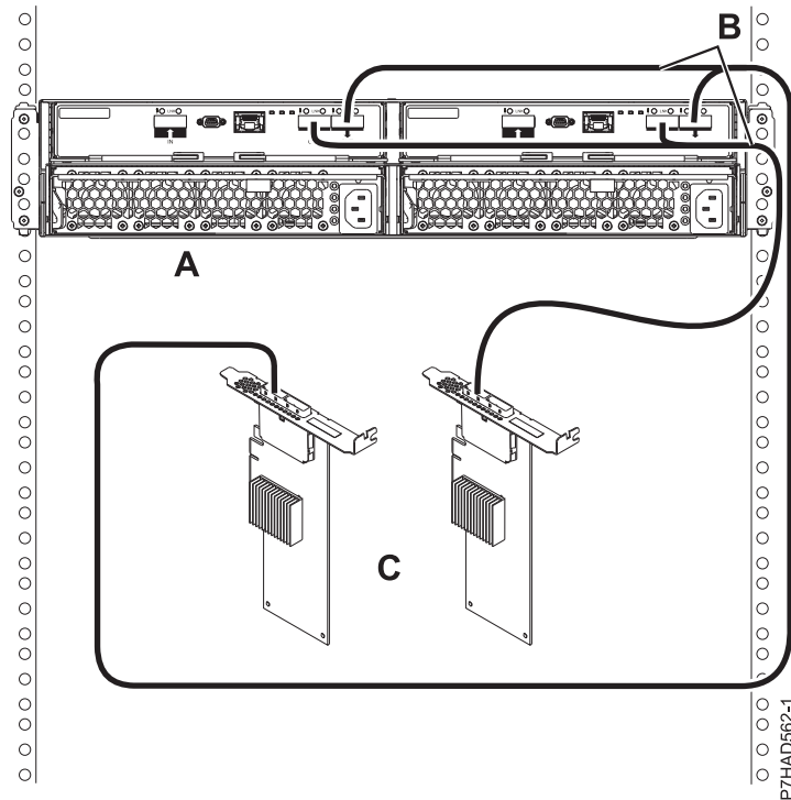
図 142. 2 つの SAS アダプターへの YO ケーブルを使用した 5887 ドロワーのモード 1 接続
