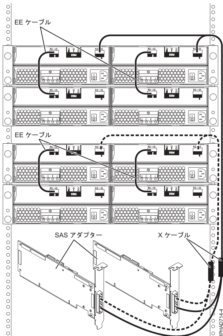
図 133. 2 つの SAS RAID アダプターと 4 つのディスク拡張ドロー間 (マルチ・イニシエーター HA RAID 構成)
