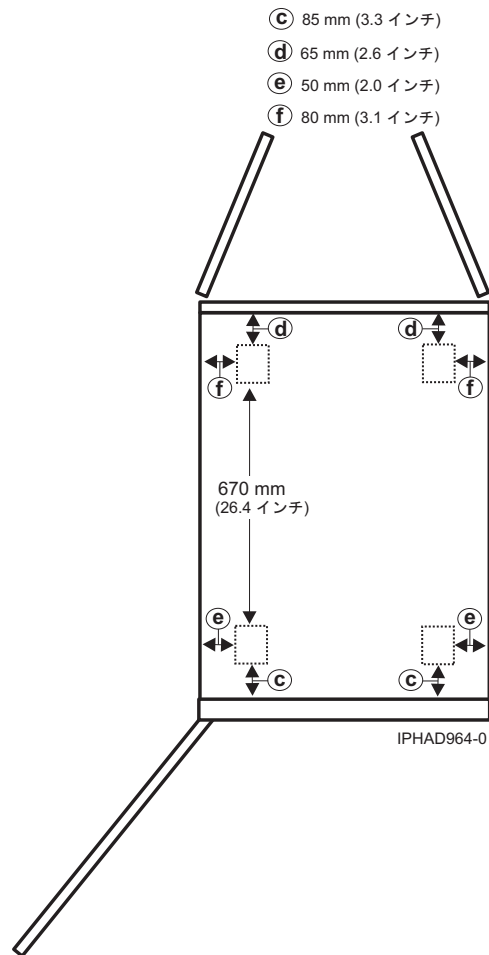
図 9. モデル 0555 および 7014-S25 のキャスター位置
