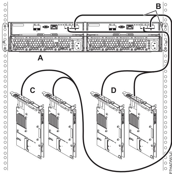
図 147. モード 2 接続を介して、2 ペアの FC 5805 または FC 5903 アダプターを 1 つの 5887 ドロワーに接続。
