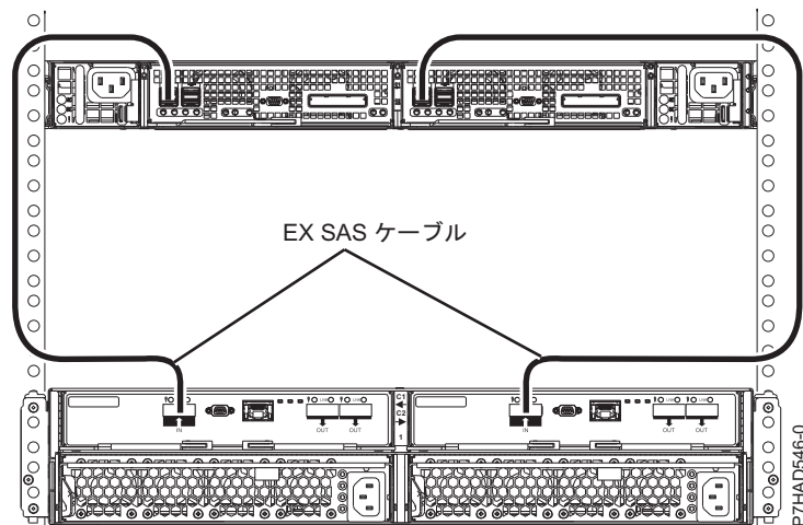
図 154. HD EX ケーブルを使用した、1 つの 5887 ドロワーから 1 つの EDR1 への接続
