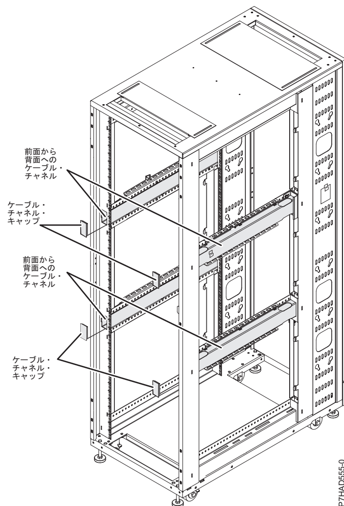
図 13. ラック内ケーブル接続
