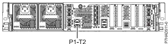
図 114. 、8246-L1C、8246-L1D、8246-L1S、8246-L1T、8246-L2C、8246-L2D、8246-L2S、および 8246-L2T の背面図とケーブル取り付け位置
