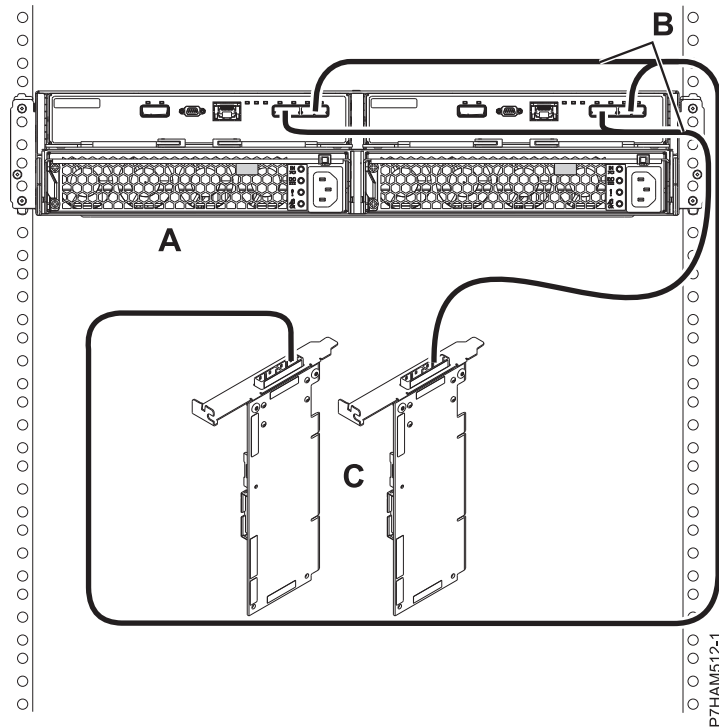
図 146. 2 つの SAS アダプターへの YO ケーブルを使用した 5887 ドロワーのモード 1 接続
