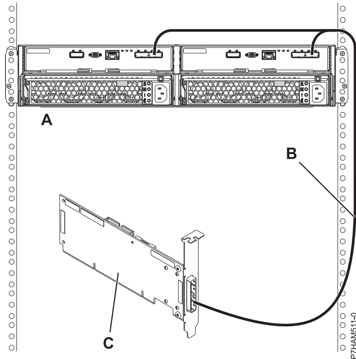
図 148. 単一の SAS アダプターへの YO ケーブルを使用した 5887 ドロワーのモード 1 接続
