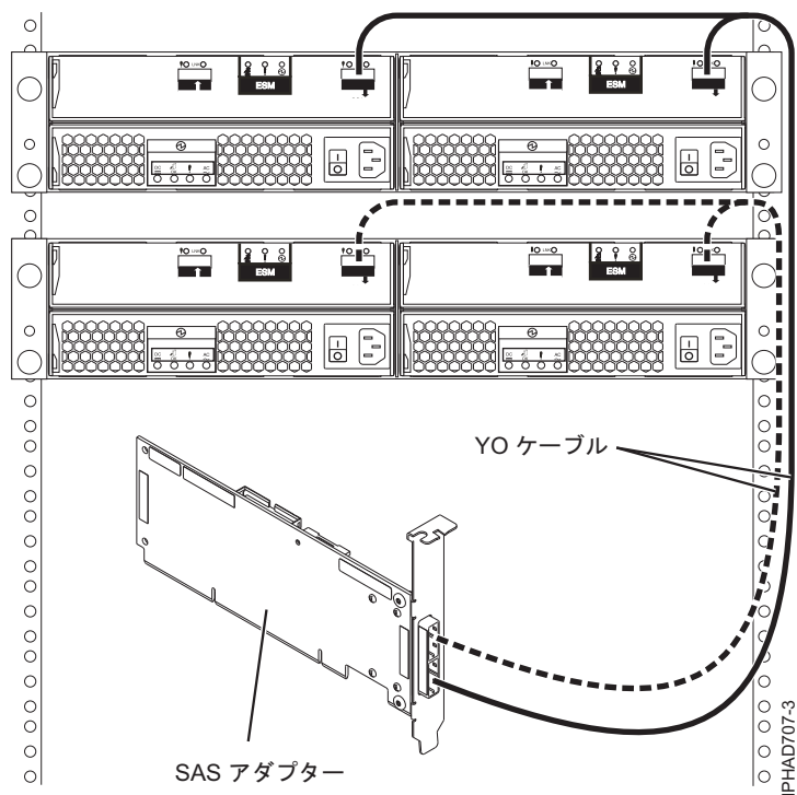
図 123. SAS アダプターと 2 つのディスク拡張ドロワー間
