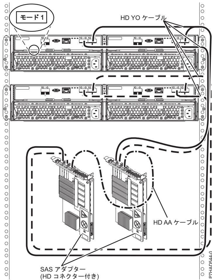
図 151. 2 つの SAS アダプターへの HD コネクターを使用した 2 つの 5887 ドロワーのモード 1 接続
