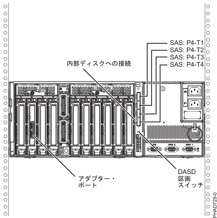
図 140. 2 つの RAID SAS アダプターと 1 つのディスク拡張ドロワー間 (マルチ・イニシエーター HA JBOD 構成)
