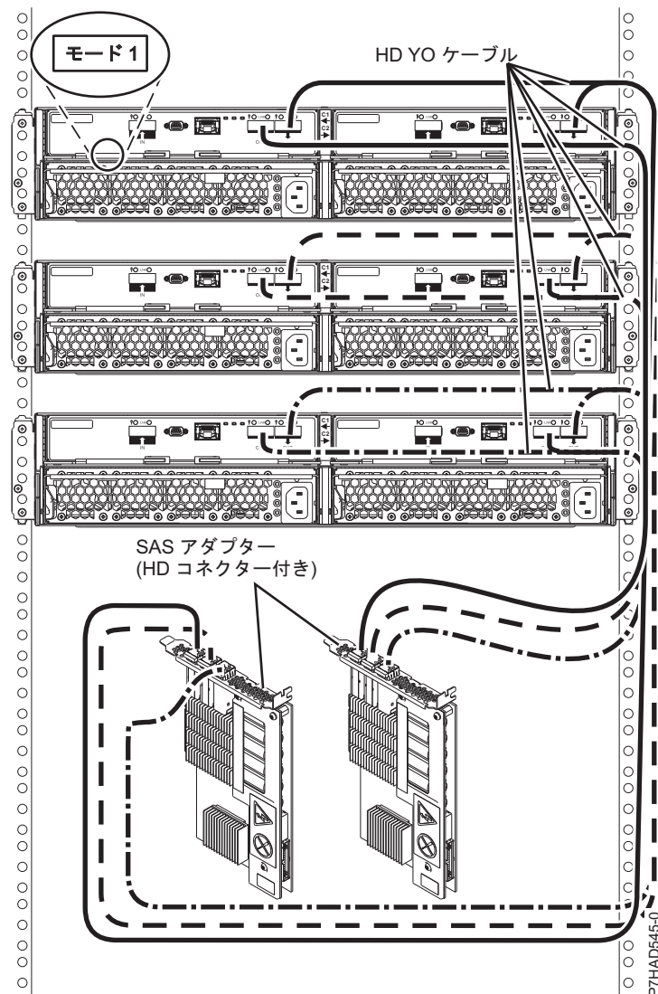
図 152. 2 つの SAS アダプターへの HD コネクターを使用した 3 つの 5887 ドロワーのモード 1 接続
