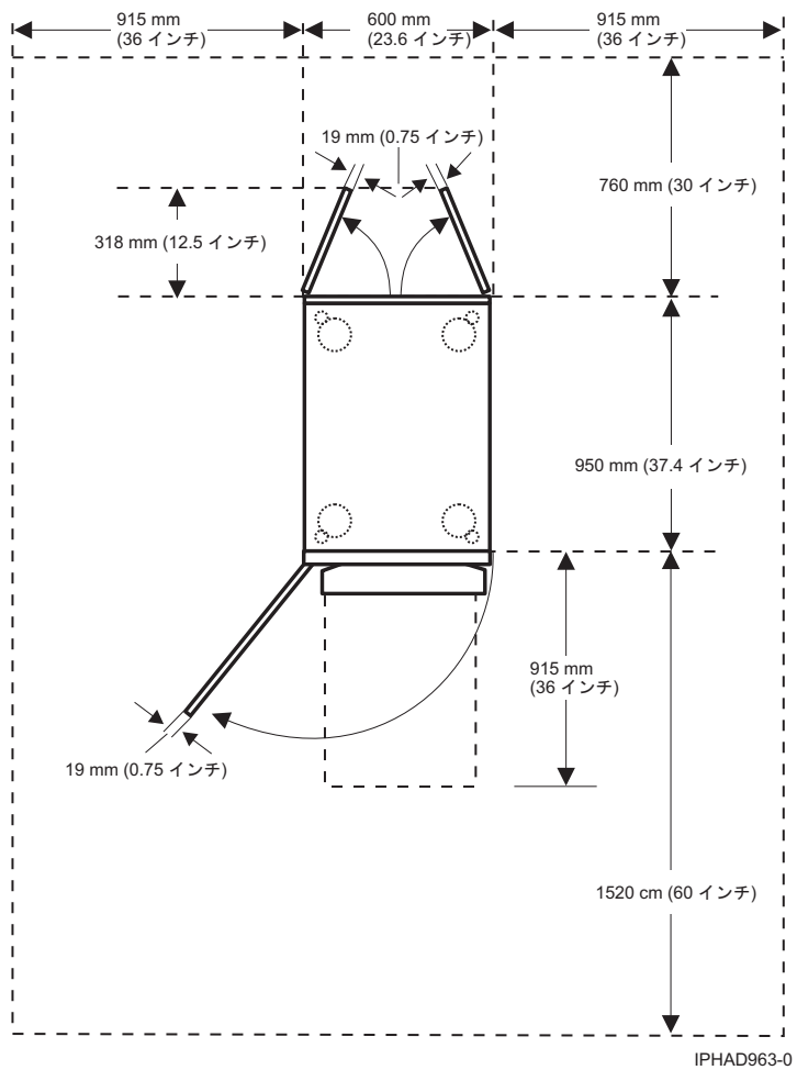
図 8. モデル 0555 および 7014-S25 平面図
