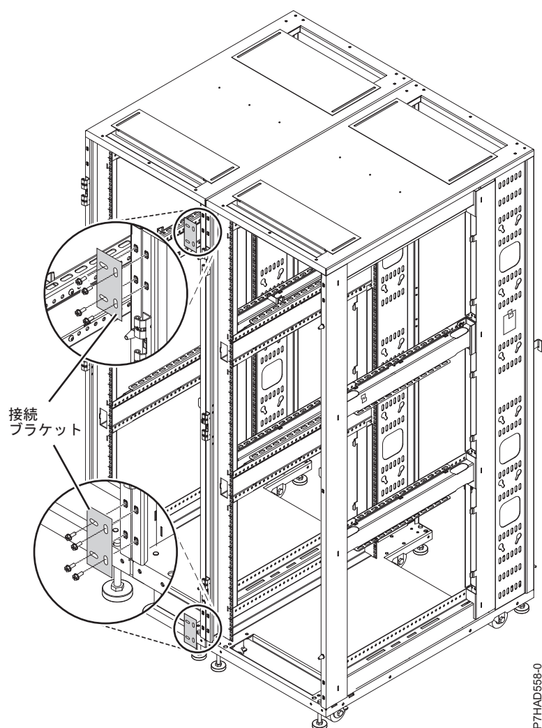
図 17. 接続ブラケット
