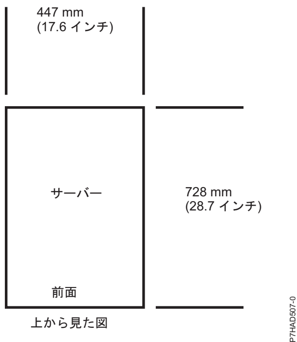
図 1. モデル 8246-L1C、8246-L1D、8246-L1S、8246-L1T、8246-L2C、8246-L2D、8246-L2S、および 8246-L2T の平面図 (ラック・マウント型サーバー)
