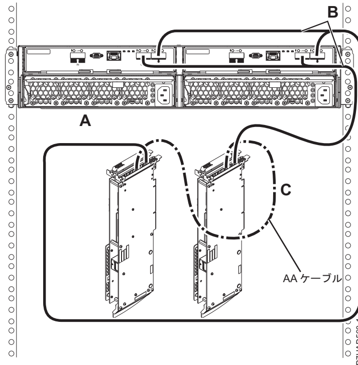
図 149. 2 つの SAS アダプターへの YO ケーブルを使用した 5887 ドロワーのモード 1 接続
