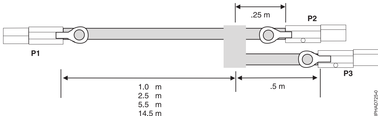
図 120. SAS 外付け Y0 ケーブル・アセンブリのケーブルの長さ
