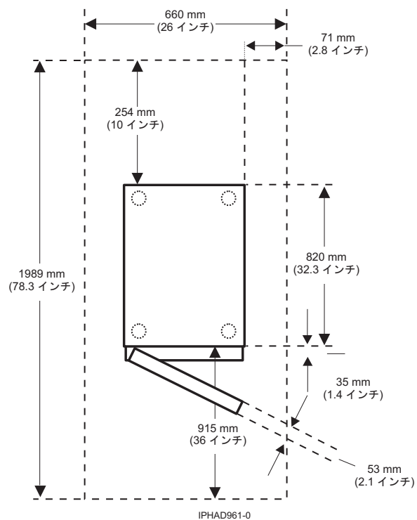
図 5. モデル 0554 および 7014-S11 平面図
