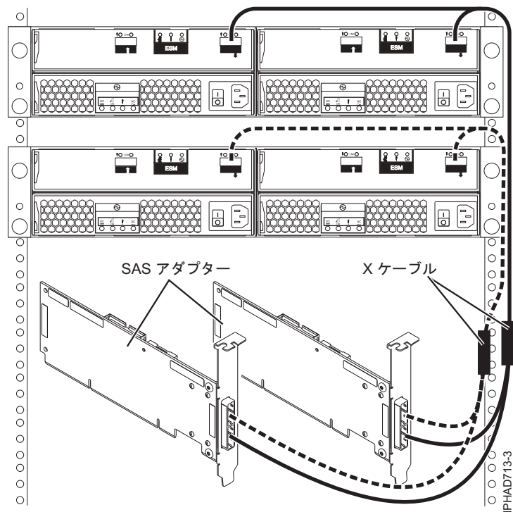
図 132. 2 つの SAS RAID アダプターと 2 つのディスク拡張ドロワー間 (マルチ・イニシエーター HA RAID 構成)
