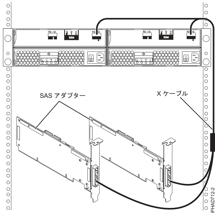
図 131. 2 つの SAS RAID アダプターと 1 つのディスク拡張ドロワー間 (マルチ・イニシエーター HA RAID 構成)
