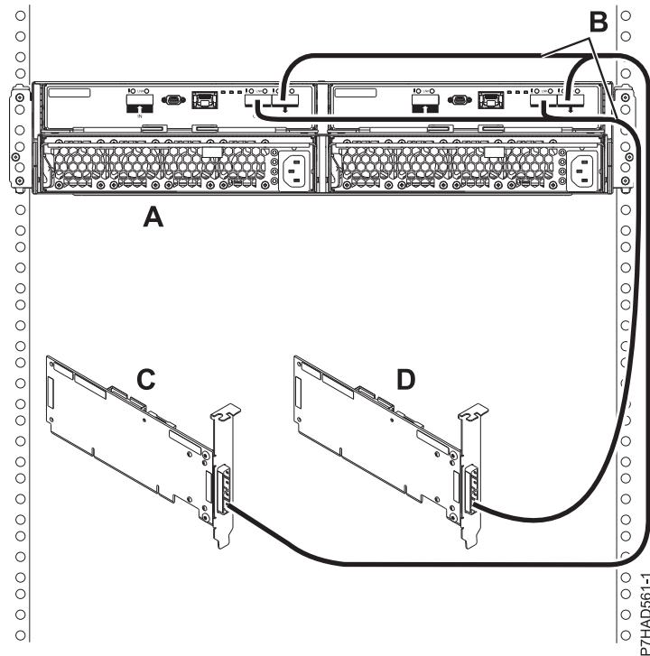
図 143. 2 つの単一 SAS アダプターへの YO ケーブルを使用した 5887 ドロワーのモード 2 接続
