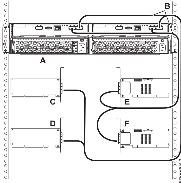
図 145. 4 つの単一 SAS アダプターへの X ケーブルを使用した 5887 ドロワーのモード 4 接続。
