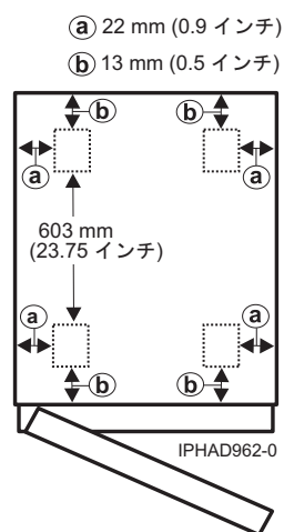
図 6. モデル 0554 および 7014-S11 のキャスター位置
