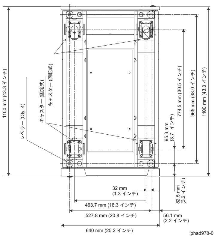
図 10. キャスターおよびレベラーの位置
