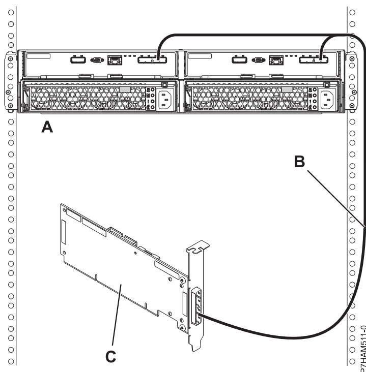
図 141. 単一の SAS アダプターへの YO ケーブルを使用した 5887 ドロワーのモード 1 接続
