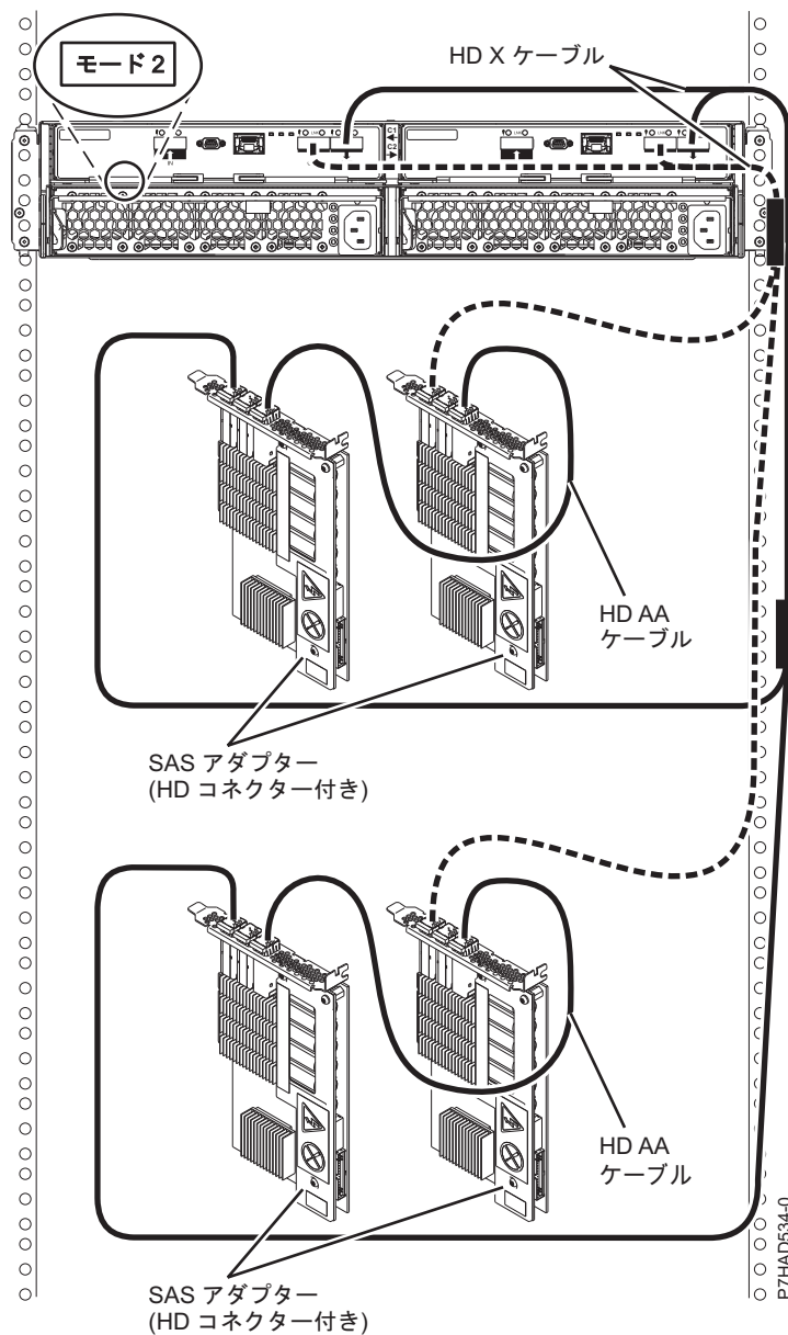
図 153. 2 ペアの SAS アダプターへの HD コネクターを使用した 5887 ドロワーのモード 2 接続
