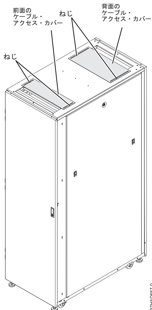
図 15. ケーブル・アクセス・カバー
