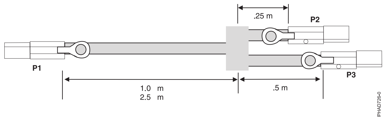
図 121. SAS 外付け Y1 ケーブル・アセンブリのケーブルの長さ
