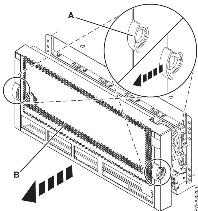
図 5. 前面カバーの取り外し
