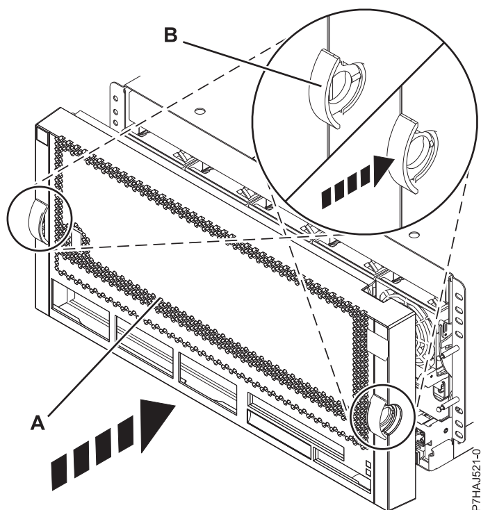
図 6. 前面カバーの取り付け
