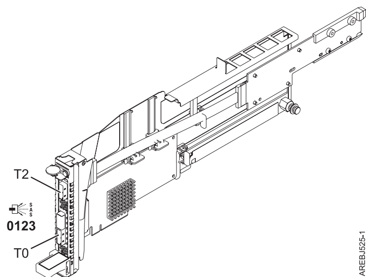
図 11. CCIN 57B9 PCIe x8 外付け Dual-x4 3 Gb SAS アダプターおよびケーブル・カード
