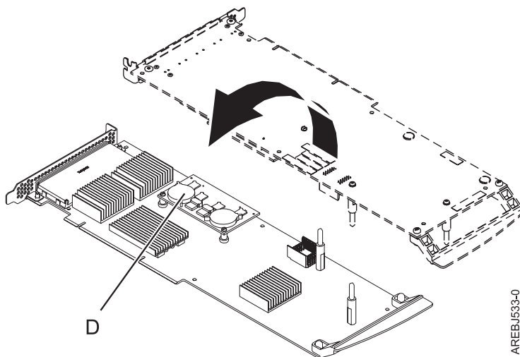
図 43. キャッシュ・ディレクトリー・カード
