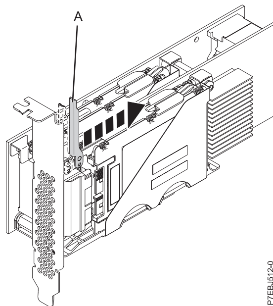
図 48. アダプター・テール・ストックから離れる方向にレバーを押し
