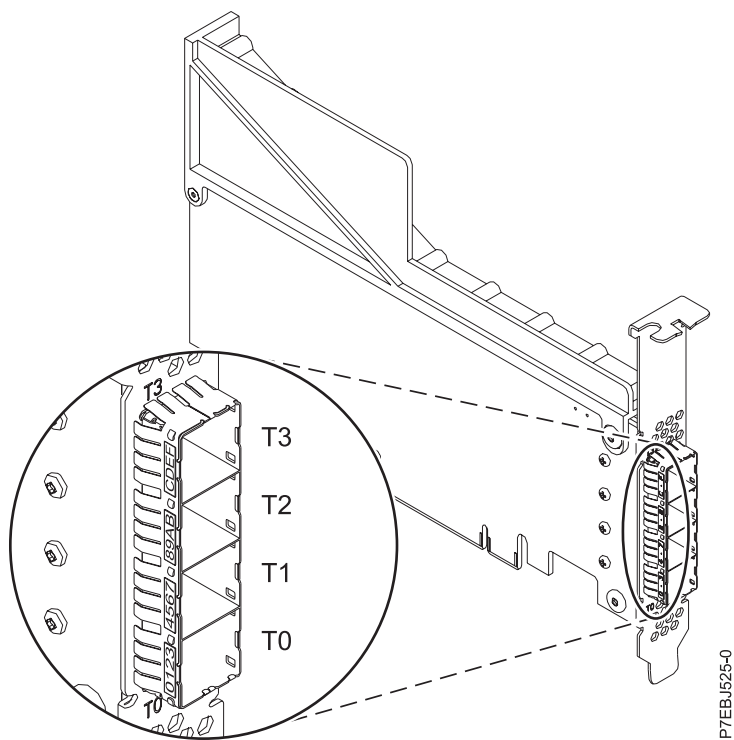
図 22. CCIN 57B4 PCIe3 RAID SAS アダプター・クワッド・ポート 6 Gb x8、2 ユニット
