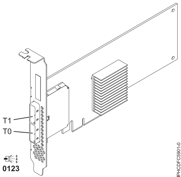
図 9. CCIN 57B3 PCIe x8 外付け Dual-x4 3 Gb SAS アダプター
