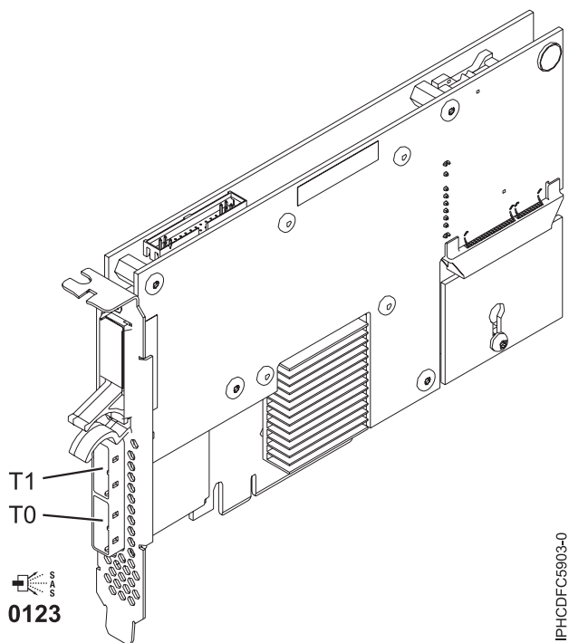
図 8. CCIN 574E PCIe x8 Ext Dual-x4 3 Gb SAS RAID アダプター (ディスク/メディア・バックプレーン)
