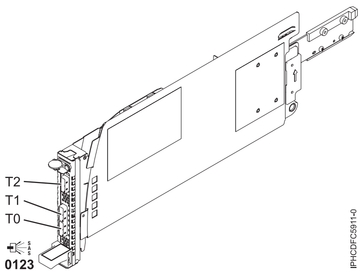
図 12. CCIN 57BA PCIe x8 外付け Dual-x4 3 Gb SAS アダプターおよびケーブル・カード
