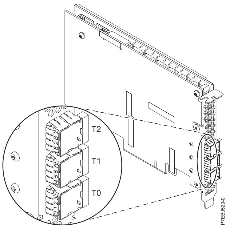
図 18. CCIN 57B5 PCIe2 1.8 GB キャッシュ RAID SAS アダプター 3 ポート 6 Gb
