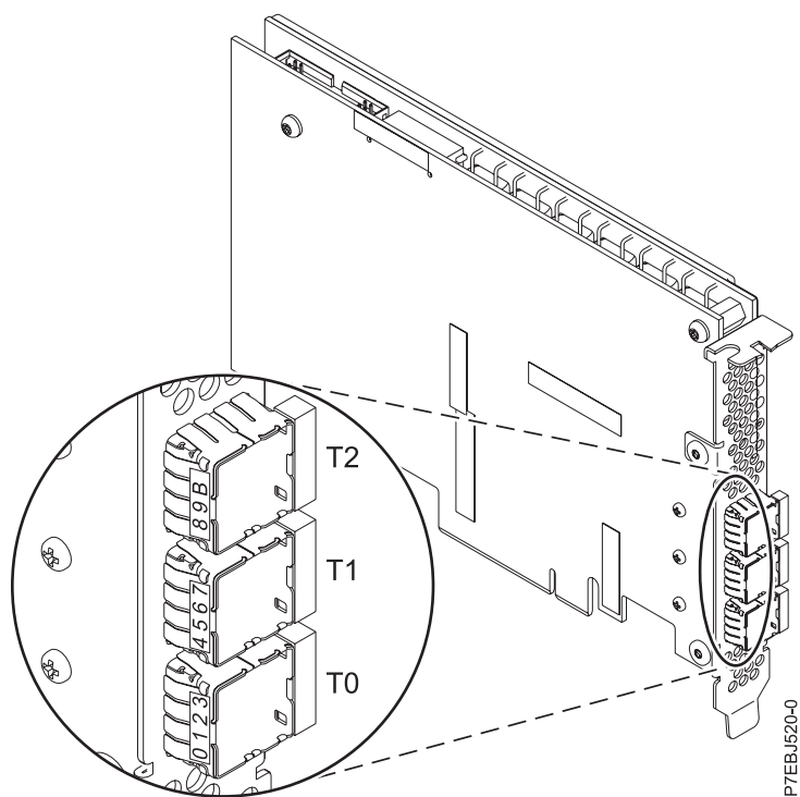
図 21. CCIN 57BB PCIe2 1.8 GB キャッシュ RAID SAS アダプター 3 ポート 6 Gb
