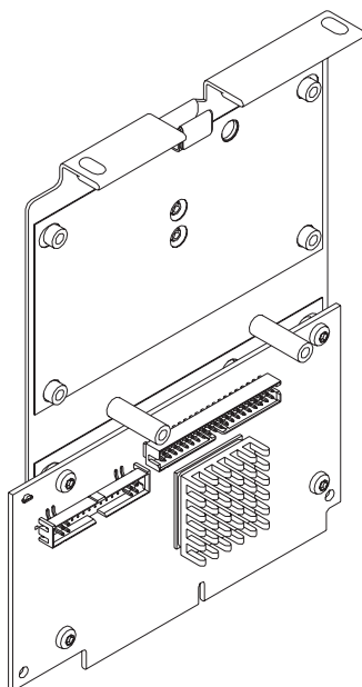
図 6. CCIN 2BE0 PCI-X266 プレーナー 3 Gb SAS アダプター
