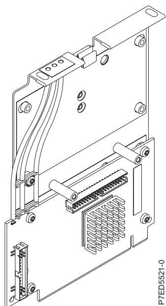
図 17. CCIN 2B4F PCIe x4 内部 3Gb SAS RAID アダプター
