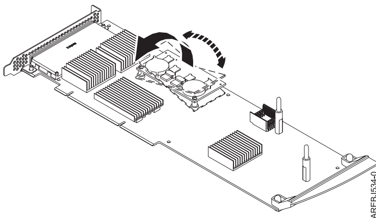
図 44. コネクタの取り外し
