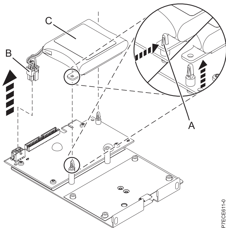
図 38. キャッシュ・バッテリーの取り外し
