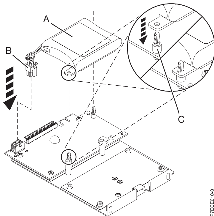
図 39. キャッシュ・バッテリーの再取り付け
