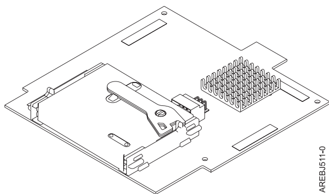
図 10. CCIN 57B7 プレーナー補助キャッシュ
