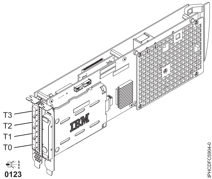
図 3. CCIN 572F PCI-X266 外付け Tri-x4 3 Gb SAS RAID アダプターおよび CCIN 575C PCI-X266 補助キャッシュ・アダプター
