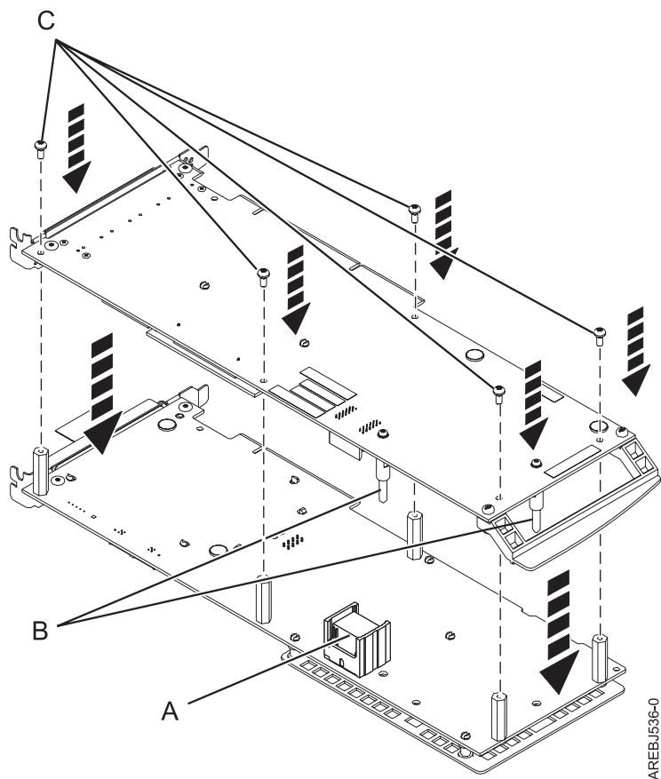
図 45. カードの再組み立て
