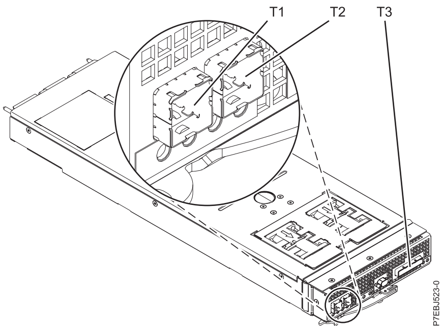
図 19. CCIN 57C3 PCIe2 3.1 GB キャッシュ RAID SAS エンクロージャー 6 Gb x8
