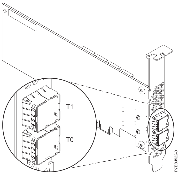
図 20. CCIN 57C4 PCIe2 RAID SAS アダプター・デュアル・ポート 6 Gb
