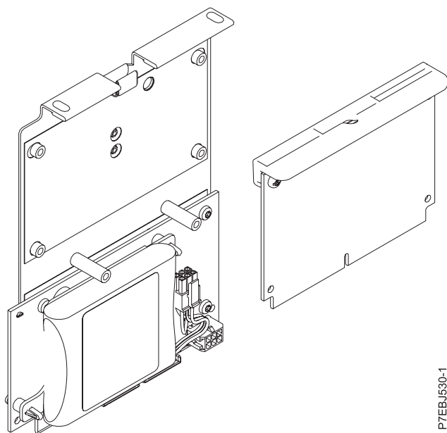
図 5. CCIN 2BE1 PCI-X266 プレーナー 3 Gb SAS アダプター
