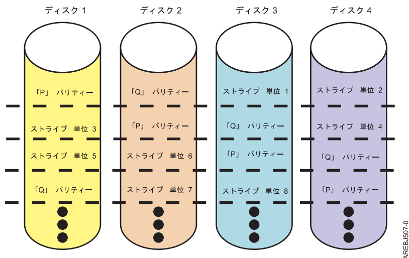
図 29. RAID 6
