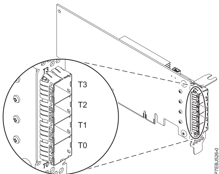
図 23. CCIN 57B4 PCIe3 RAID SAS アダプター・クワッド・ポート 6 Gb x8、4 ユニット
