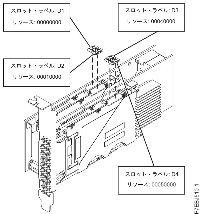
図 14. CCIN 57CD PCIe SAS RAID および 3 Gb x8 SSD アダプター
