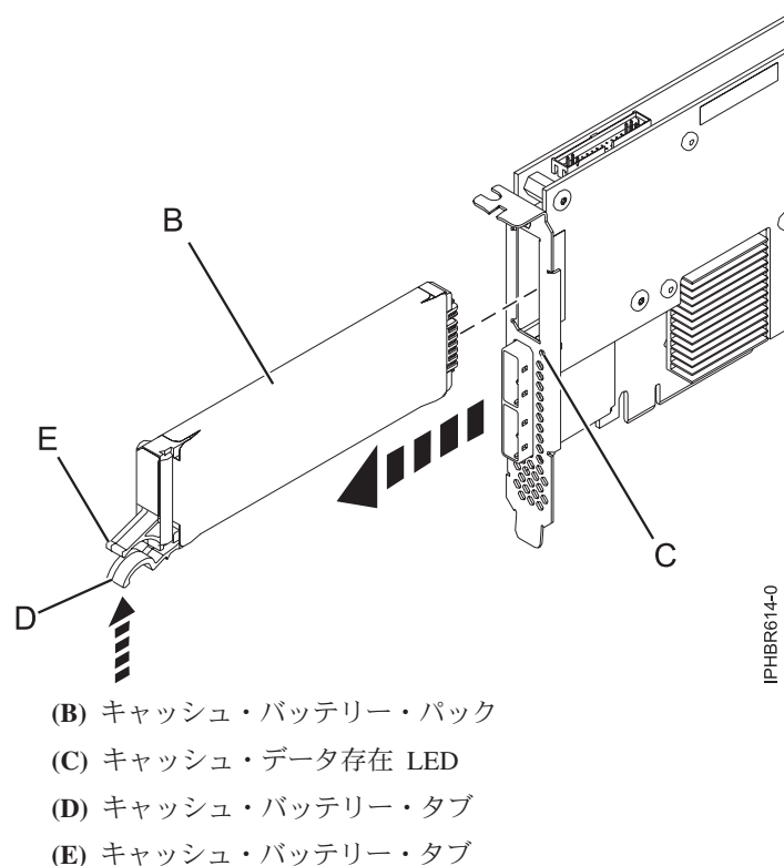
図 35. 574E キャッシュ・バッテリーの取り替え
