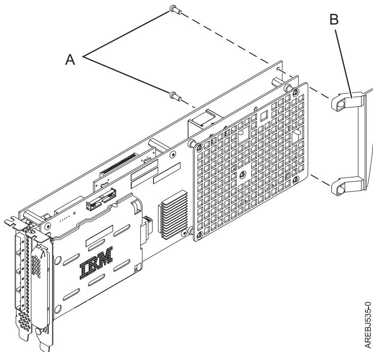
図 46. カセット・アダプター・ハンドルの接続
