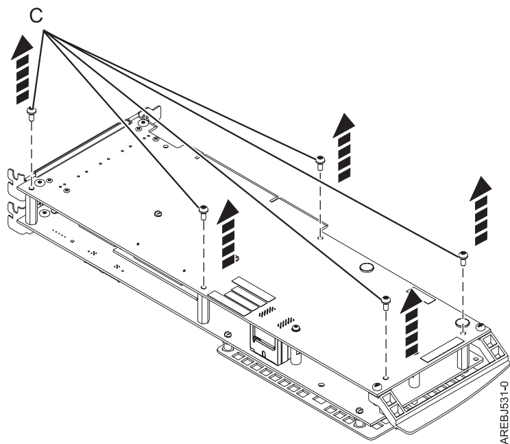
図 41. 572F/575C カード・セット・アダプター上のねじの位置
