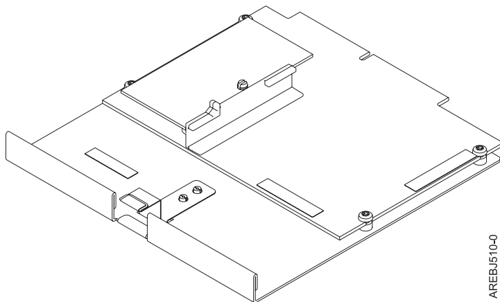
図 4. CCIN 57B8 プレーナー RAID イネーブルメント・カード
