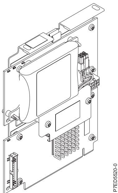
図 16. CCIN 2B4C PCIe x4 内部 3 Gb SAS アダプター
