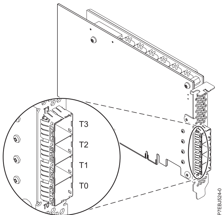
図 24. CCIN 57CE PCIe3 12 GB キャッシュ RAID SAS アダプター・クワッド・ポート 6 Gb x8
