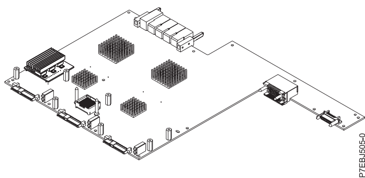
図 13. CCIN 57C7 PCI Express x8 プレーナー 3 Gb SAS アダプター (175 MB キャッシュ RAID - デュアル IOA インタープリメント・カード付き)
