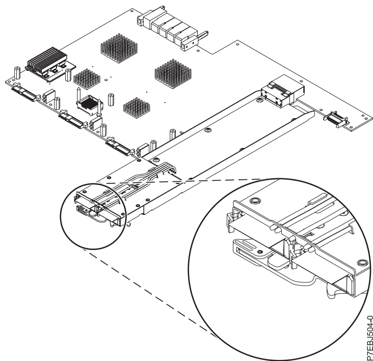
図 15. CCIN 57CF PCI Express x8 ブレーナー 3 Gb SAS RAID アダプター(175 MB キャッシュ RAID - デュアル IOA イネーブルメント・カード付き)
