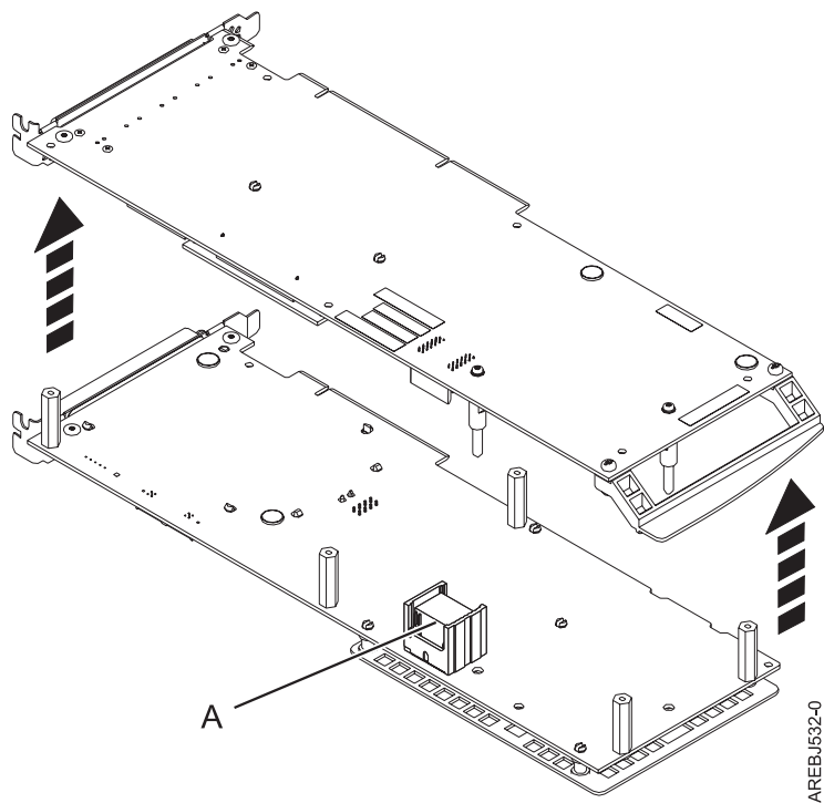
図 42. 572F/575C カード・セット・アダプター上の相互接続コネクタの位置
