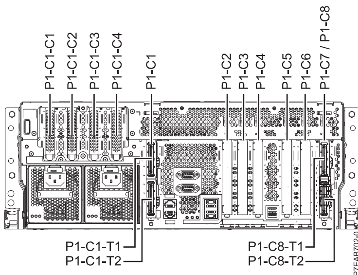
図 4. ロケーション・コード付き PCI スロットを示すシステムの背面図
