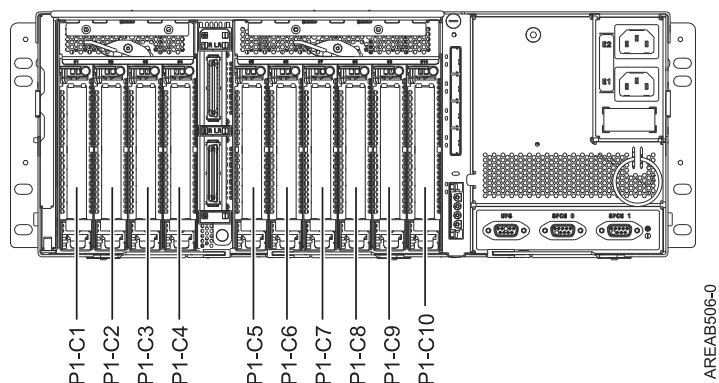
図 6. 背面図： 次の図に、拡張装置の背面を示します。
