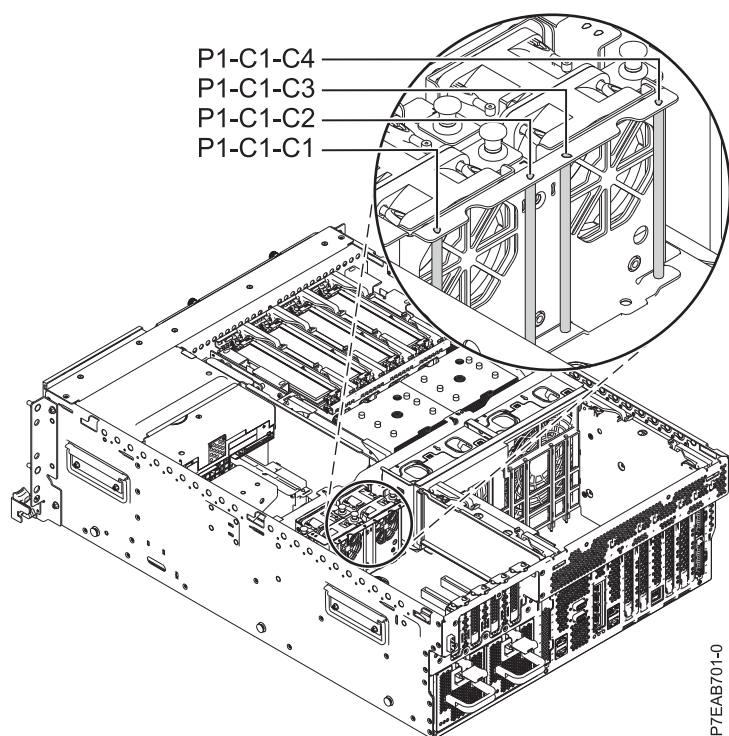
図 3. 8202-E4B および 8205-E6B システムの PCI ライザー拡張とロケーション・コード
