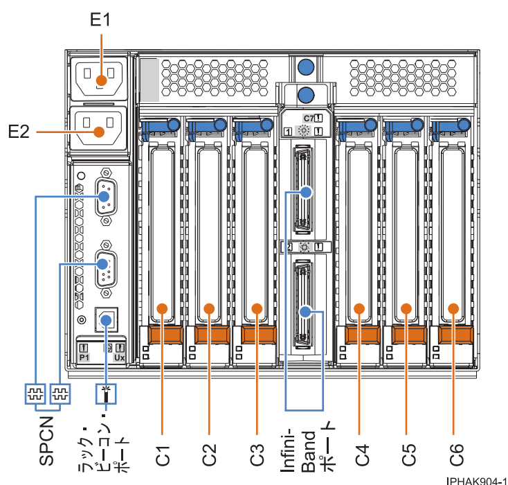
図 5. 背面図
