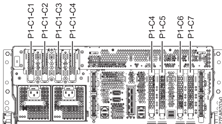
図 1. PCI スロットのロケーション・コード付きの 8202-E4B および 8205-E6B システムの背面図
