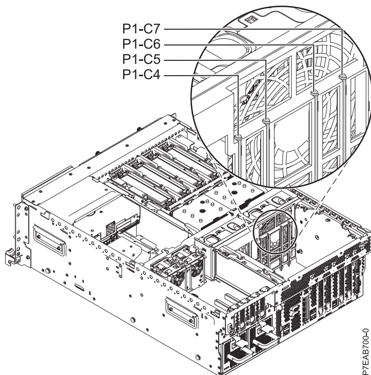
図 2. 8202-E4B システムおよび 8205-E6B システムの PCI スロットのロケーション・コード
