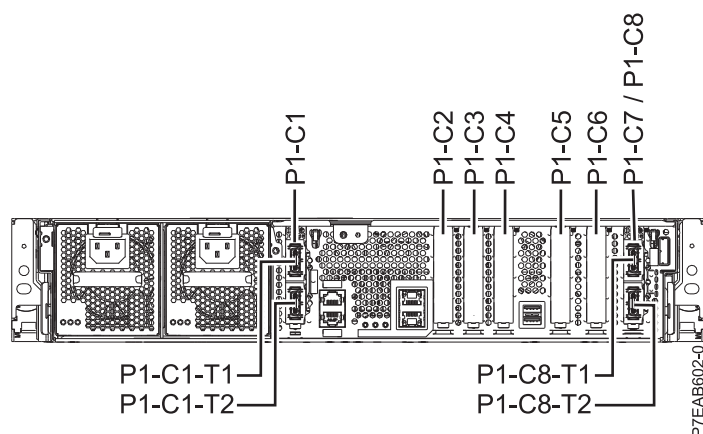
図 1. ロケーション・コード付きのシステムの背面図
