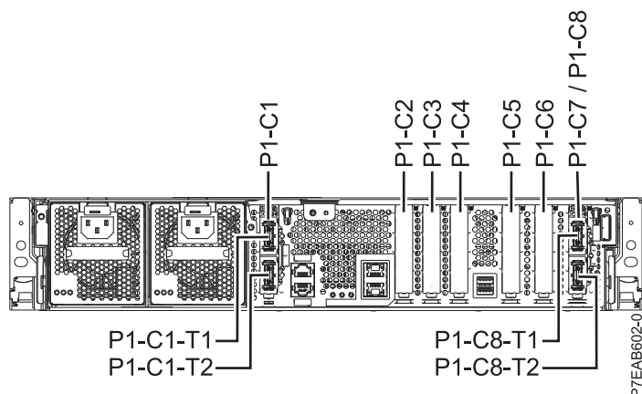
図 2. ロケーション・コード付きのシステムの背面図
