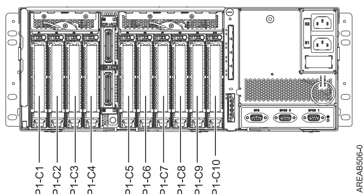
図 3. 背面図: 次の図に、拡張装置の背面を示します。
