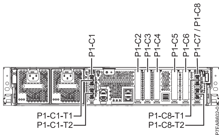
図 3. ロケーション・コード付きのシステムの背面図
