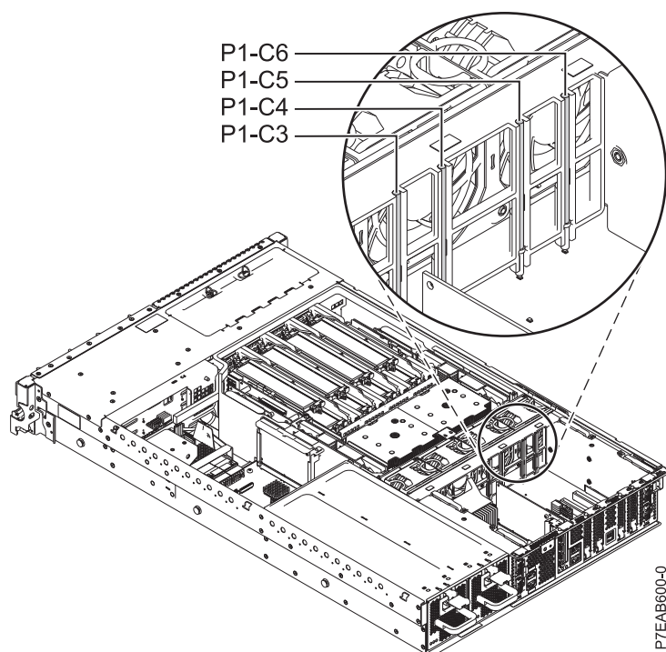
図 1. PCI スロットのロケーション・コード付きの 8231-E2B の背面図
