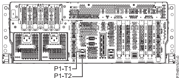
2. ábra: 8202-E4B és 8205-E6B modellek csatlakoztatása
