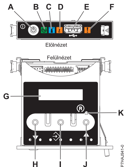
4. ábra: Vezérlőpanel
