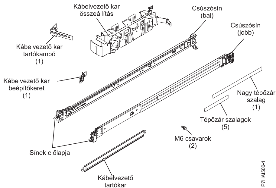
14. ábra: Alkatrészeleltár
