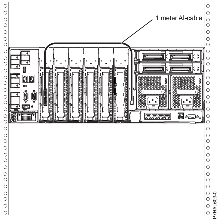
147. ábra: SAS csatoló összekapcsolása belső SAS lemez bővítőhelyekkel a rendszer külső SAS portján keresztül.
