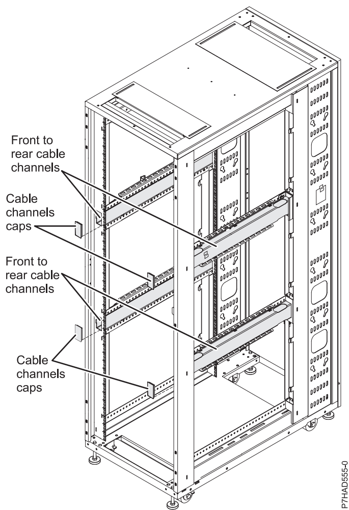
24. ábra: Kábelezés a rack szekrényen belül
