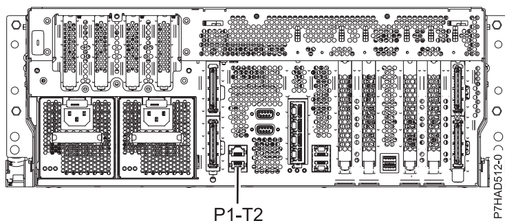
132. ábra: 8202-E4B, 8202-E4C, 8202-E4D, 8205-E6B, 8205-E6C, and 8205-E6D hátulnézete kábelbeszerelési helyel
