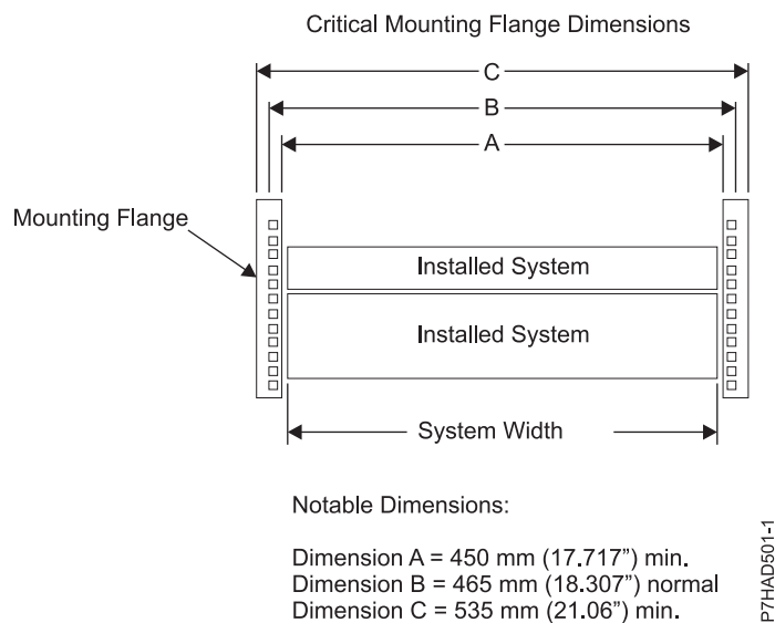
29. ábra: Kritikus beszerelési peremméreteket
