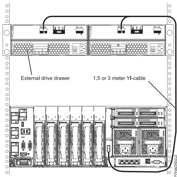
146. ábra: Külső SAS csatoló port összekapcsolása lemez bővítőfiókkal (9117-MMB és 9179-MHB modellek)
