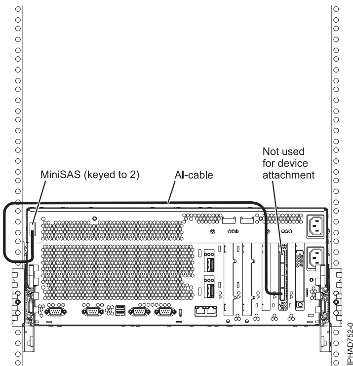
148. ábra: Lemez bővítőfiókokhoz csatlakoztatott FC5904 vagy FC5908 csatoló
