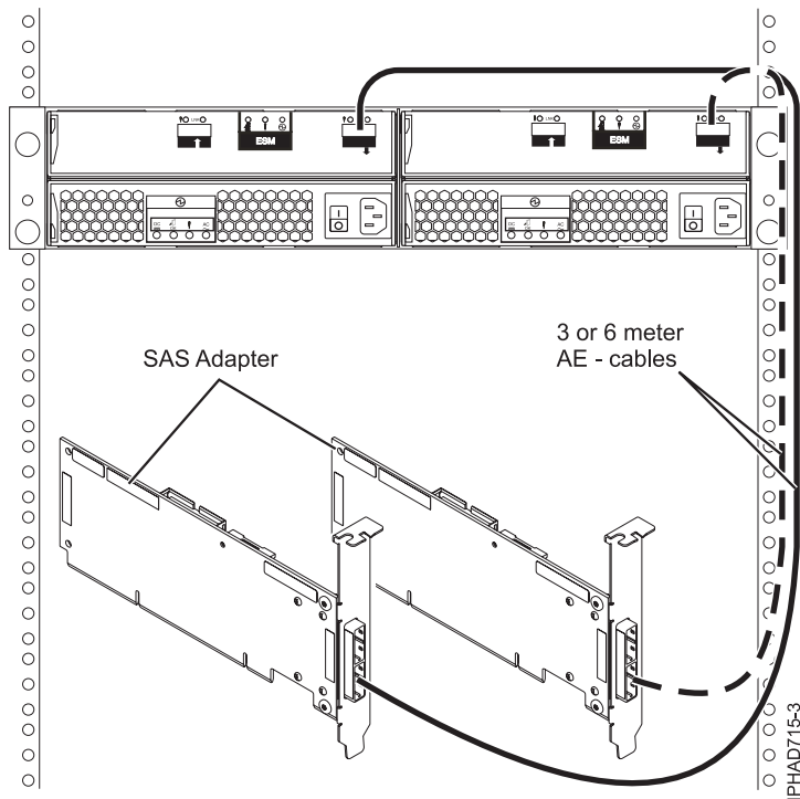
157. ábra: Két RAID SAS csatoló összekapcsolása egy lemez bővítőfiókkal több kezdeményezés HA JBOD konfigurációban
