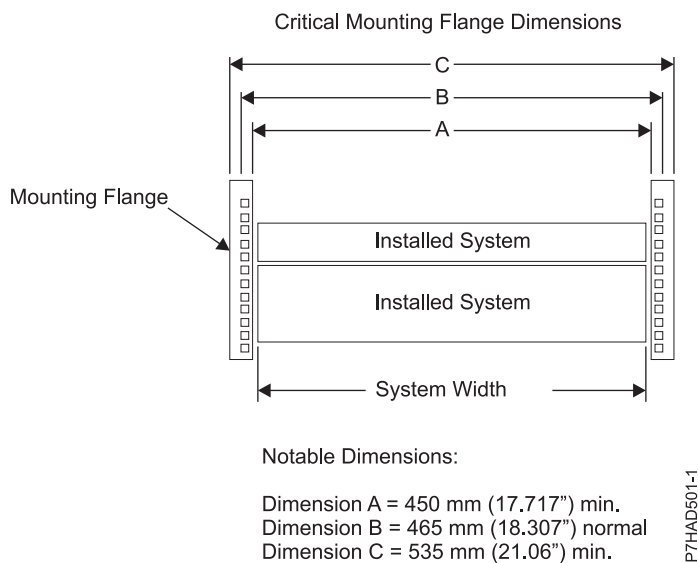
29. ábra: Kritikus beszerelési peremméretek
