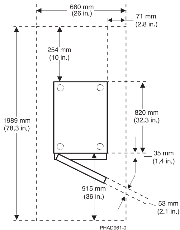
16. ábra: 0554 és 7014-S11 modell tervezési nézete
