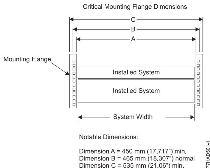
174. ábra: Kritikus beszerelési peremmérete
