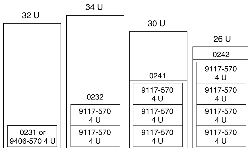
7. ábra: 570 rack szekrényben
