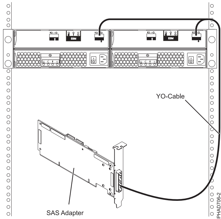
141. ábra: SAS csatoló összekapcsolása egy lemez bővítőfiókkal
