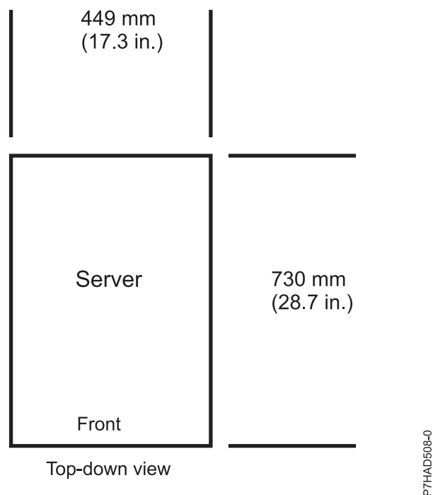
1. ábra: 8202-E4B, 8202-E4C, 8202-E4D, 8205-E6B, 8205-E6C és 8205-E6D modell tervezési nézete (rackbe szerelt szerverek)
