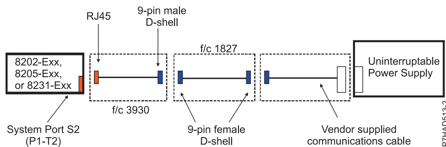
134. ábra: Szünetmentes tápegység vezetékezése a 8202-E4B, 8202-E4C, 8205-E6B, 8205-E6C, 8231-E2B, 8231-E1C, 8231-E1D, 8231-E2C, 8231-E2D, and 8268-E1D
