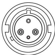
109. ábra: IEC 60309 2P+E dugaszolóaljzat típus
