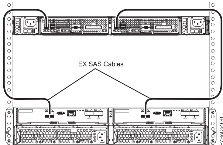
173. ábra: Egy 5887 fiók csatlakoztatása HD EX vezetékkel egy EDR1-hez
