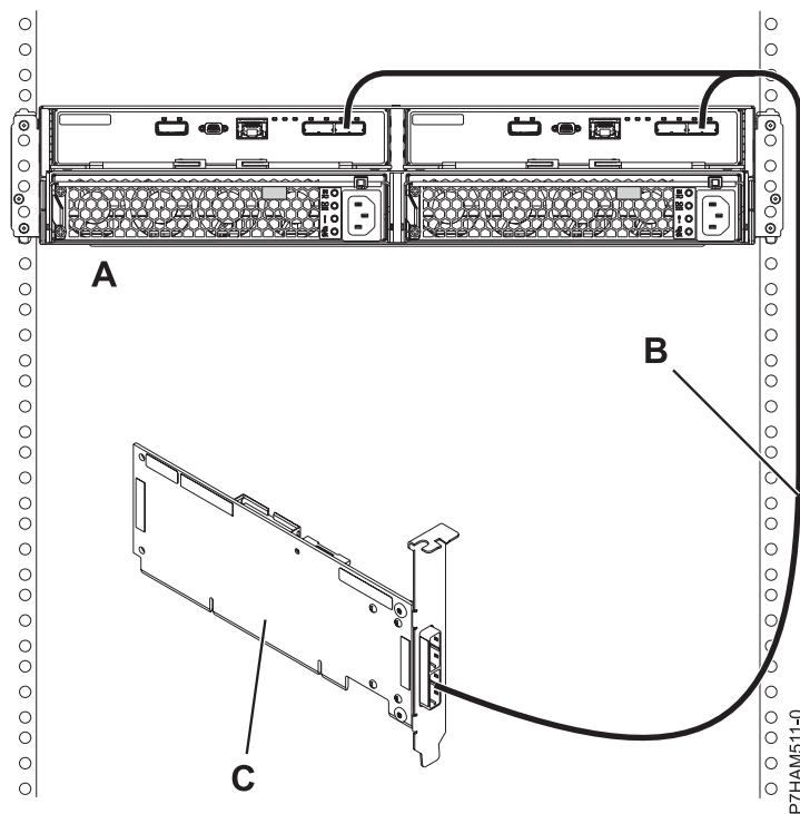
160. ábra: Egy 5887 fiók 1. módú csatlakoztatása egy SAS adapterhez egy YO kábel használatával
