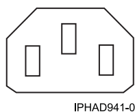
75. ábra: 15-ös dugasztípus
