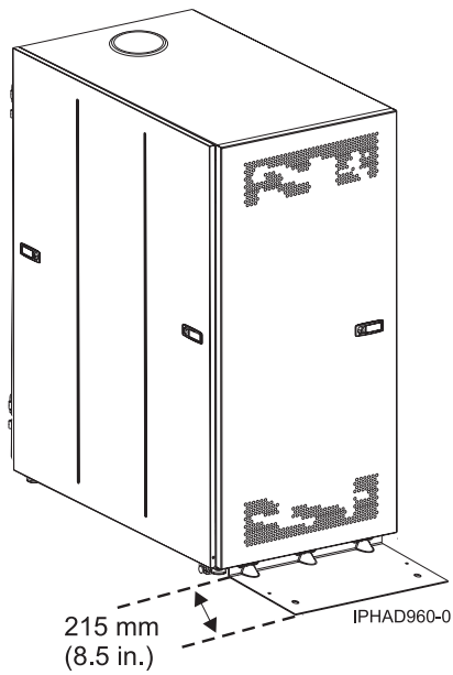
19. ábra: 0555 és 7014-S25 modell stabilizáló lábbal
