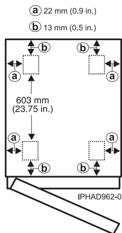
18. ábra: 0554 és 7014-S11 modell görgőhelyei
