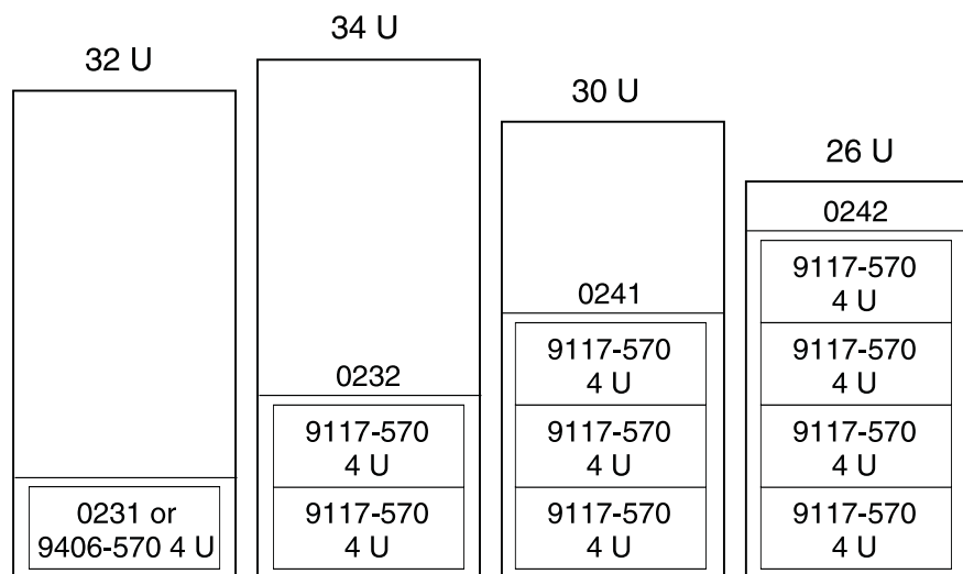
8. ábra: 570 rack szekrényben
