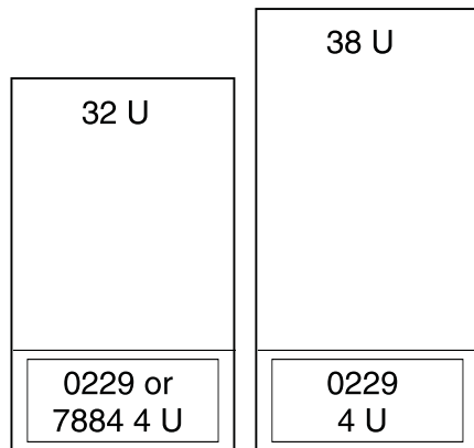
6. ábra: 7884-es termékkód: 9406-520 és 9111-520 egy rack szekrényben
