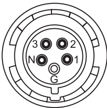
32. ábra: Csatlakozó kihúzása
