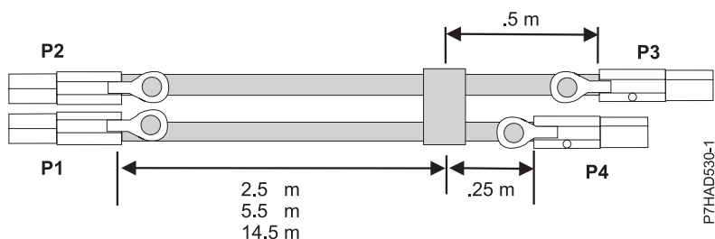
138. ábra: SAS külső X-kábel összeállítási kábelhosszak
