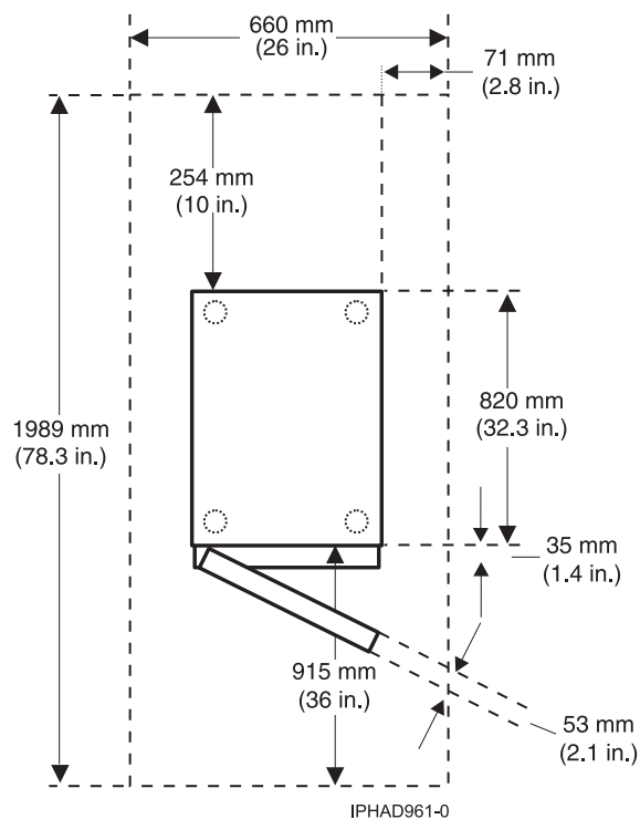
17. ábra: 0554 és 7014-S11 modell tervezési nézete
