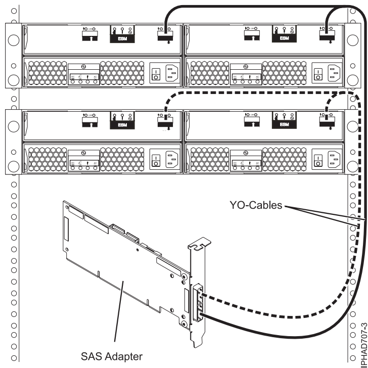
142. ábra: SAS csatoló összekapcsolása két lemez bővítőfiókkal
